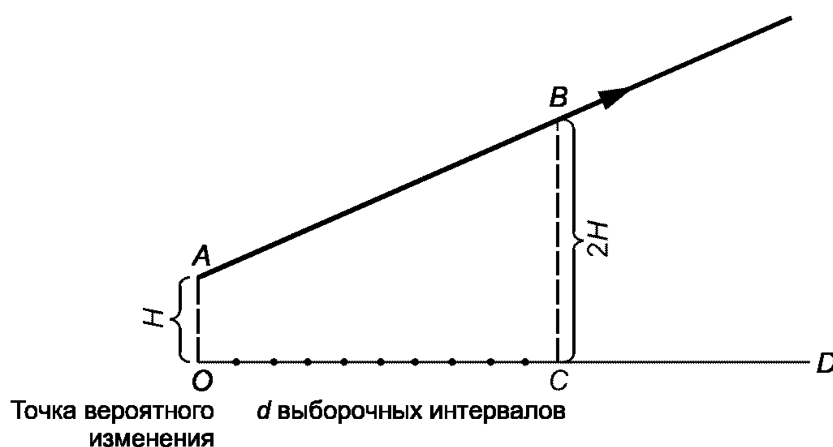
Рисунок Г.1 — Построение локальной разрешающей линии
