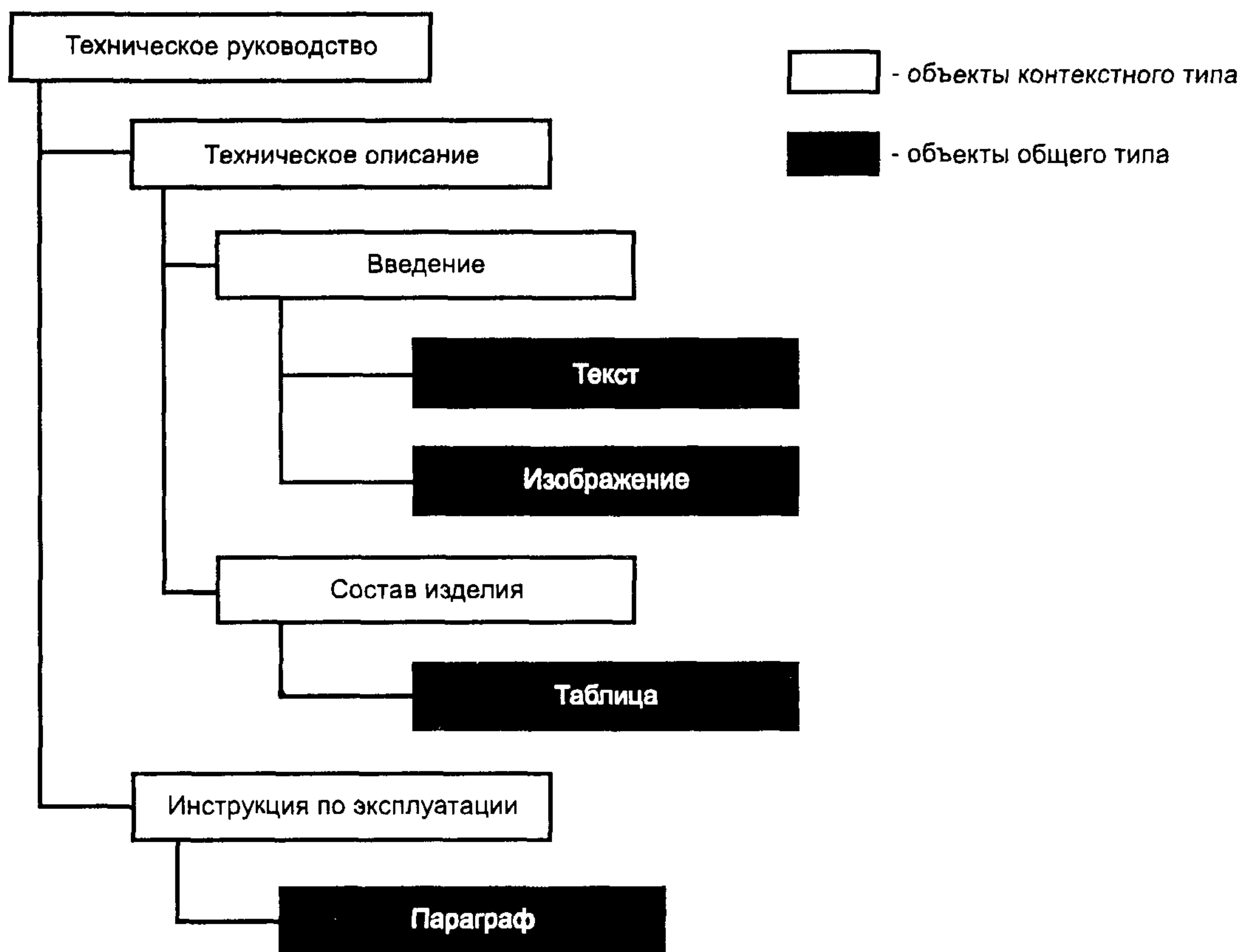
Рисунок 1 — Логическая структура базы данных
