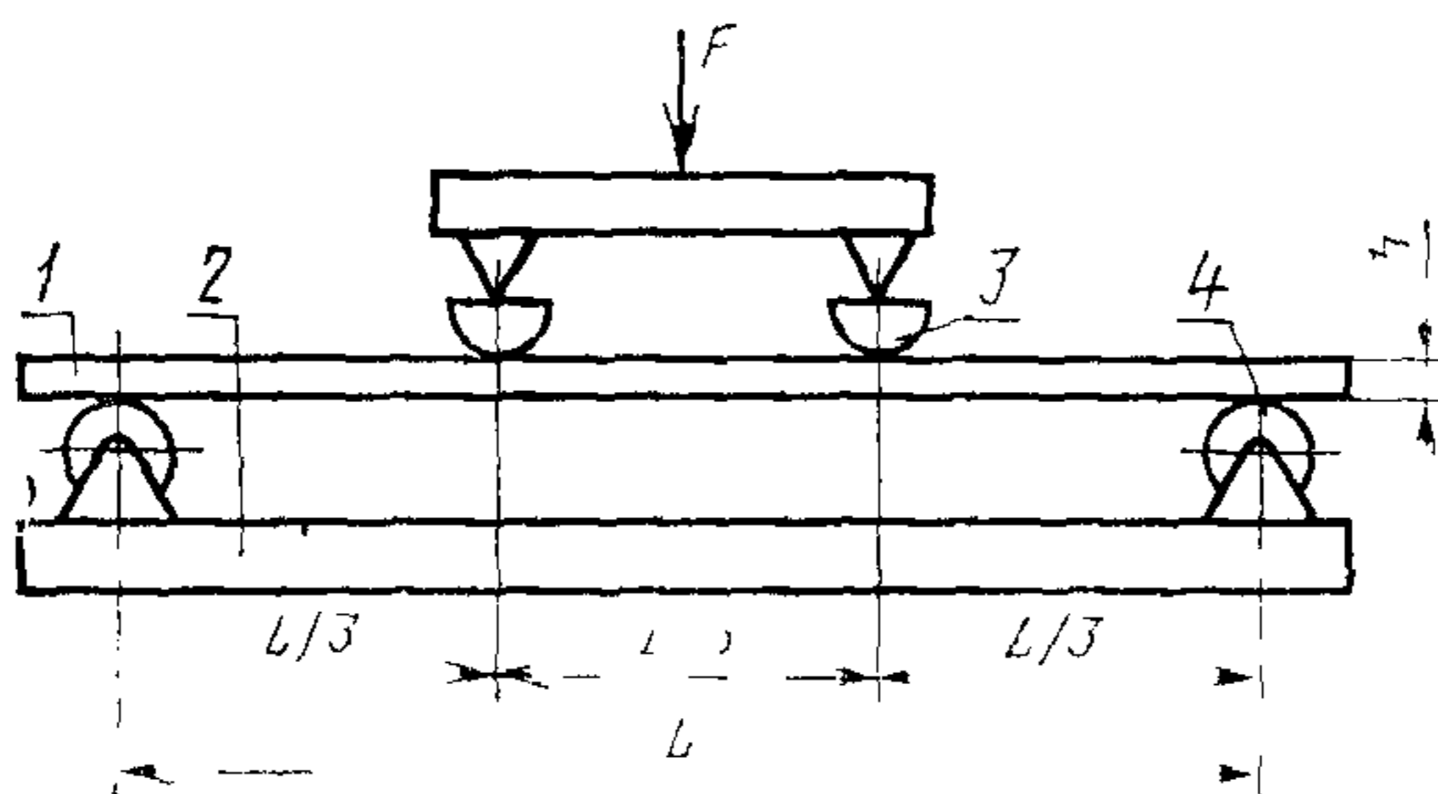
1—образец, 2—основание, 3—нагружающий элемент; 4—опора
