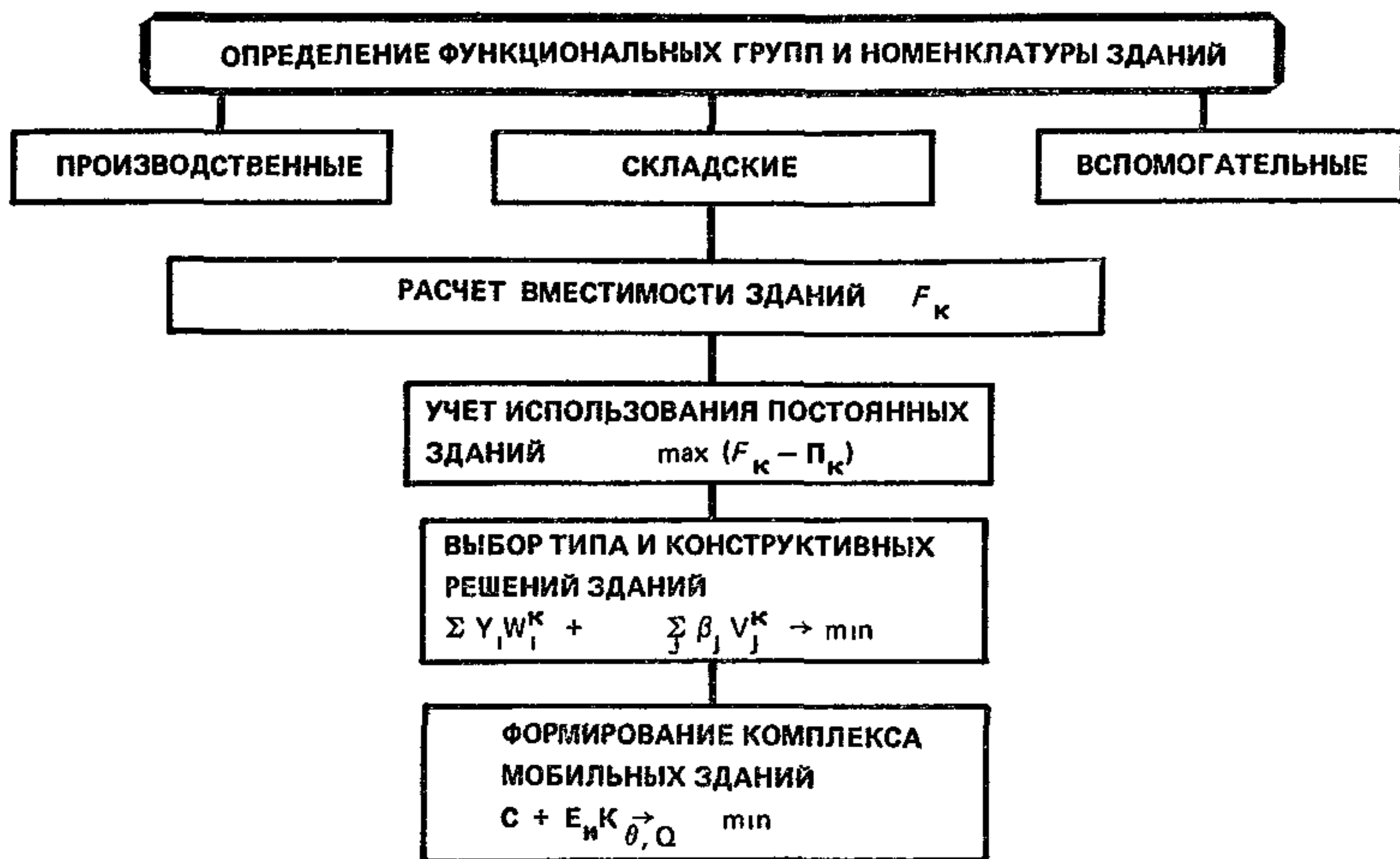
Рис. 1. Схема определения параметров комплекса мобильных (инвентарных) зданий
