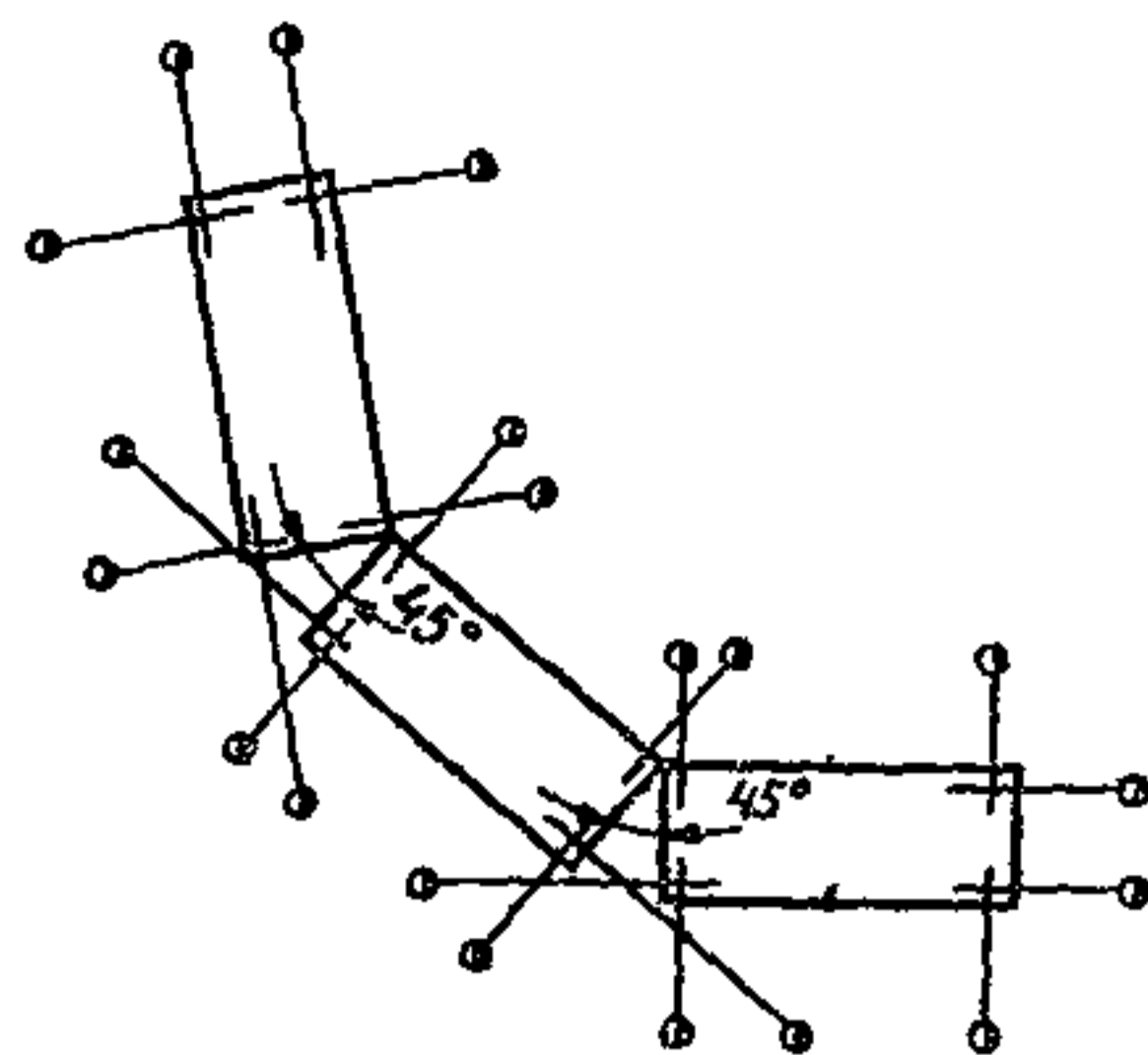
Рис. 11. Схема размещения знаков закрепления основных осей при строительстве зданий, примыкающих друг к другу под углом 45^\circ
