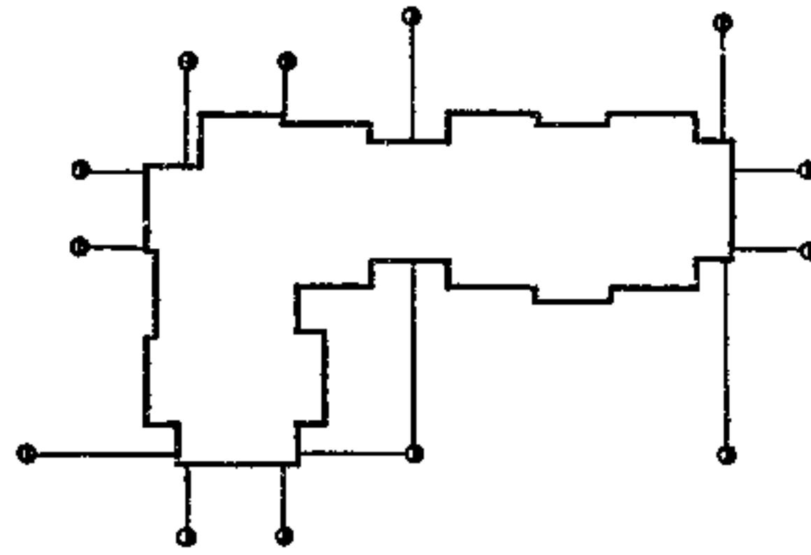
Рис. 7. Схема размещения знаков закрепления основных, промежуточных осей при строительстве зданий г-образной формы
