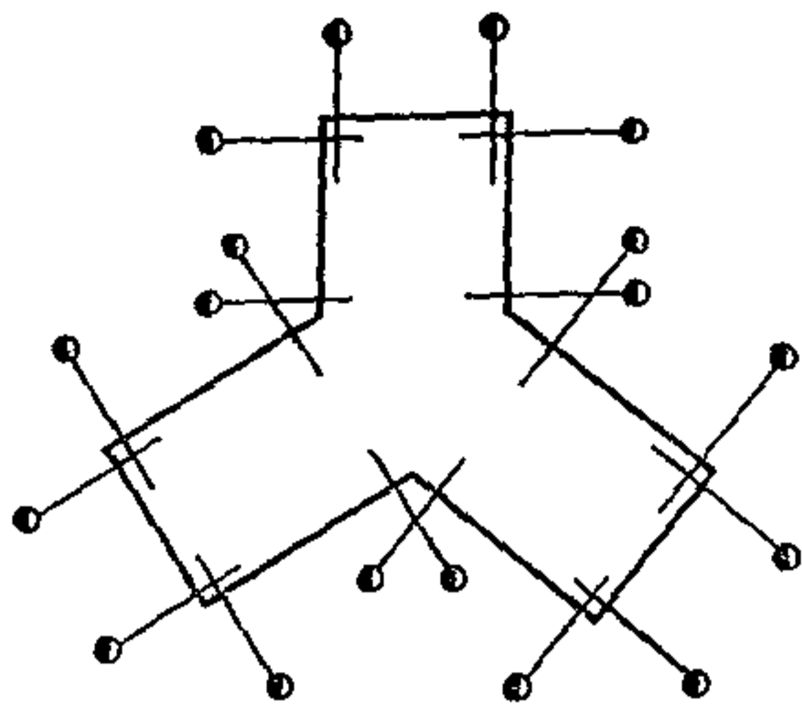
Рис. 10. Схема размещения знаков закрепления основных осей при строительстве зданий «башенной» конфигурации
