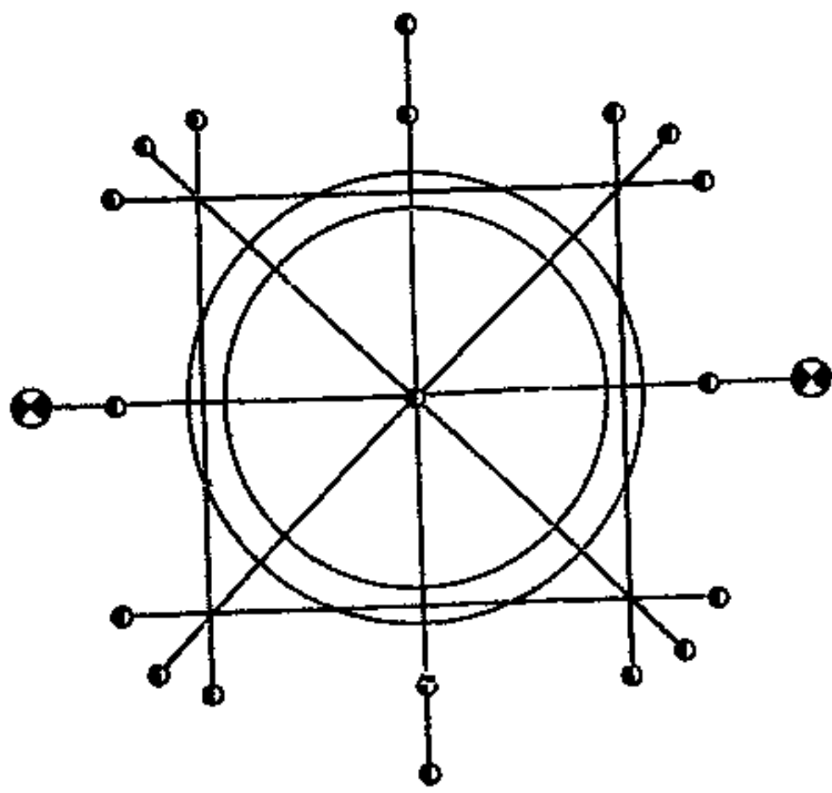
Рис. 6. Схема размещения знаков закрепления главных и основных осей при строительстве зданий круглой конфигурации
