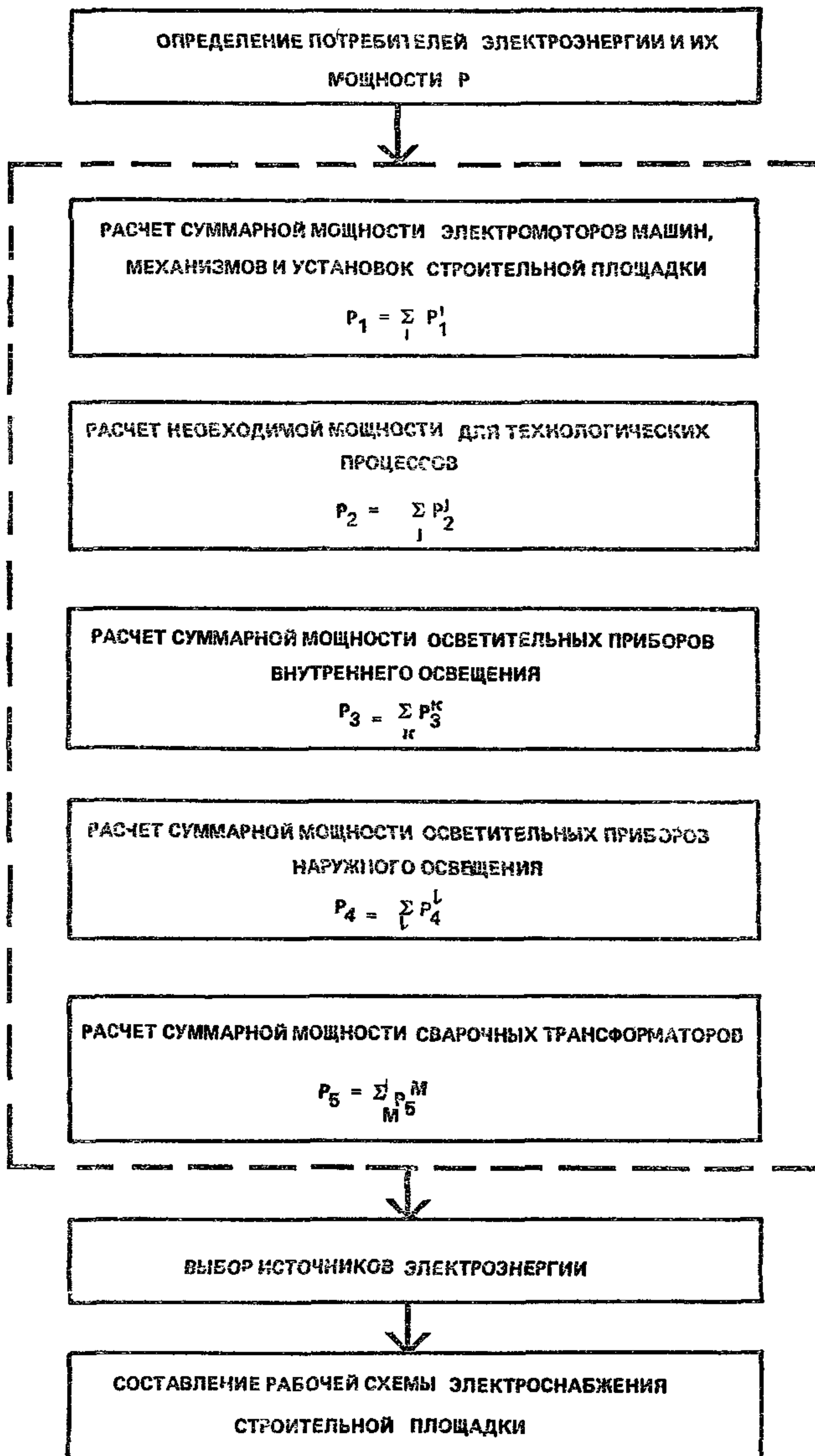
Рис. 2. Блок-схема электроснабжения строительной площадки
