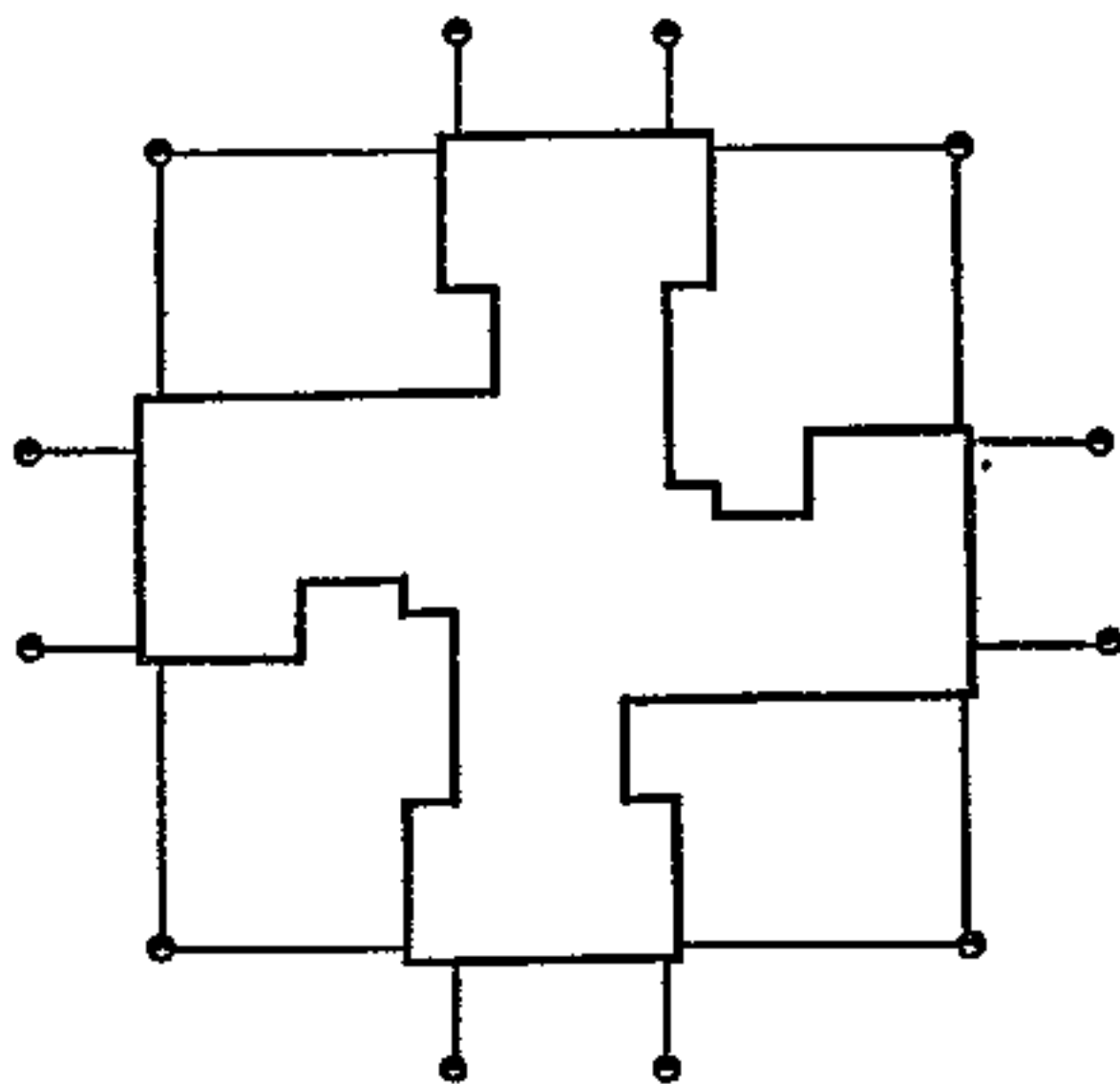
Рис. 8. Схема размещения знаков закрепления основных осей при строительстве зданий крестообразной конфигурации
