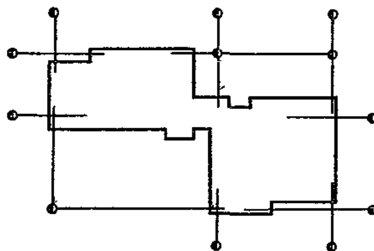
Рис. 9. Схема размещения знаков закрепления основных осей при строительстве зданий точечной конфигурации
