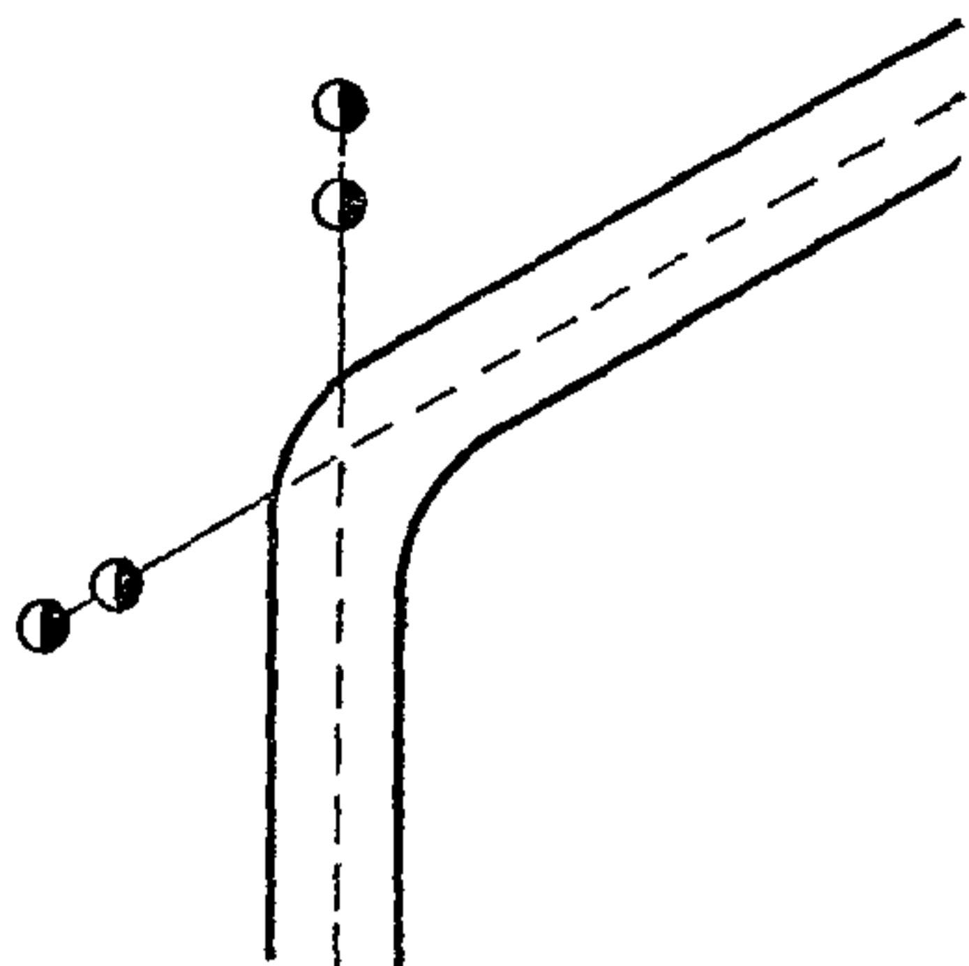
Рис. 13. Схема размещения знаков главных разбивочных осей углов поворота линейных сооружений
