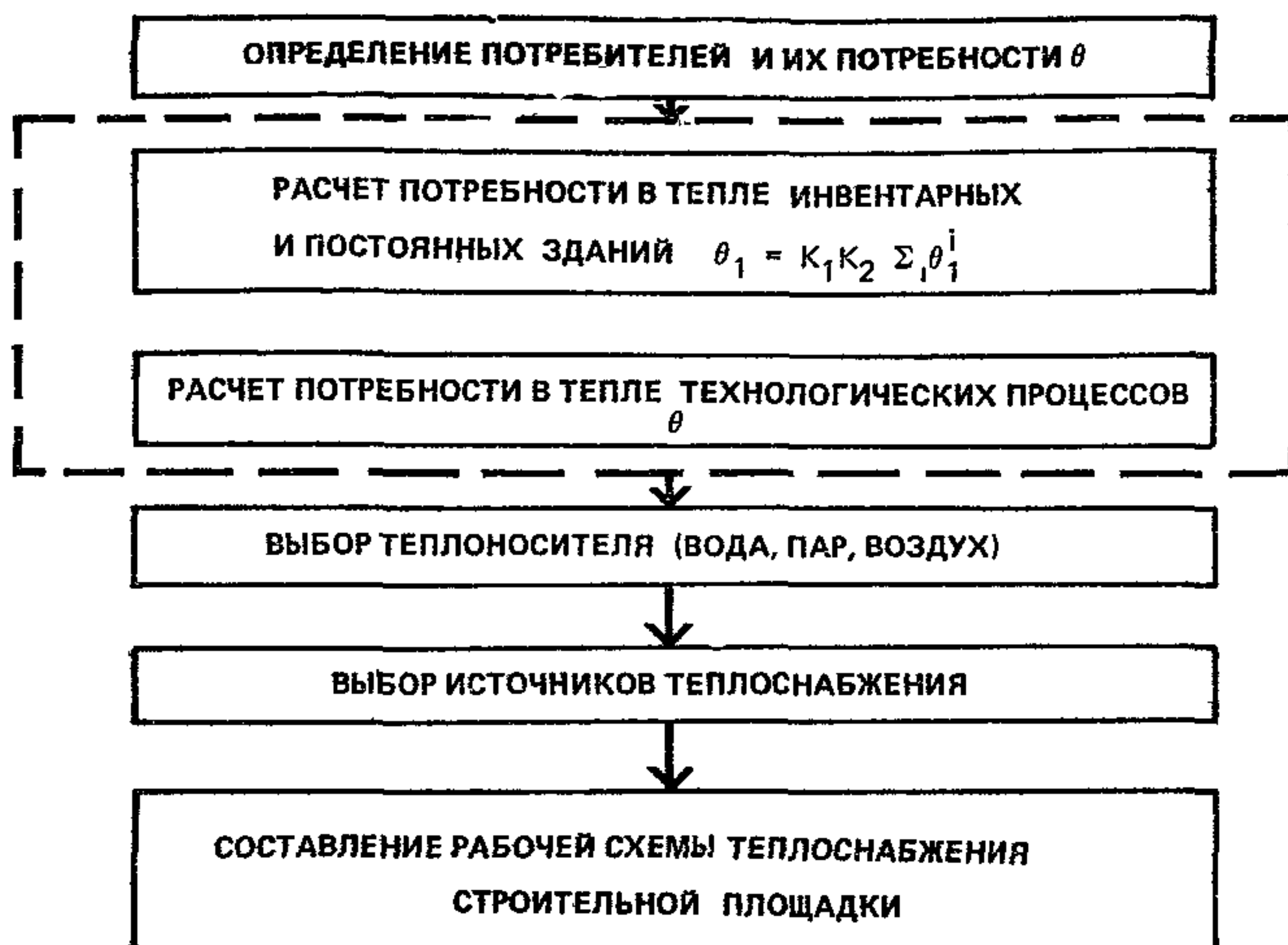
Рис. 4. Блок-схема теплоснабжения строительной площадки
