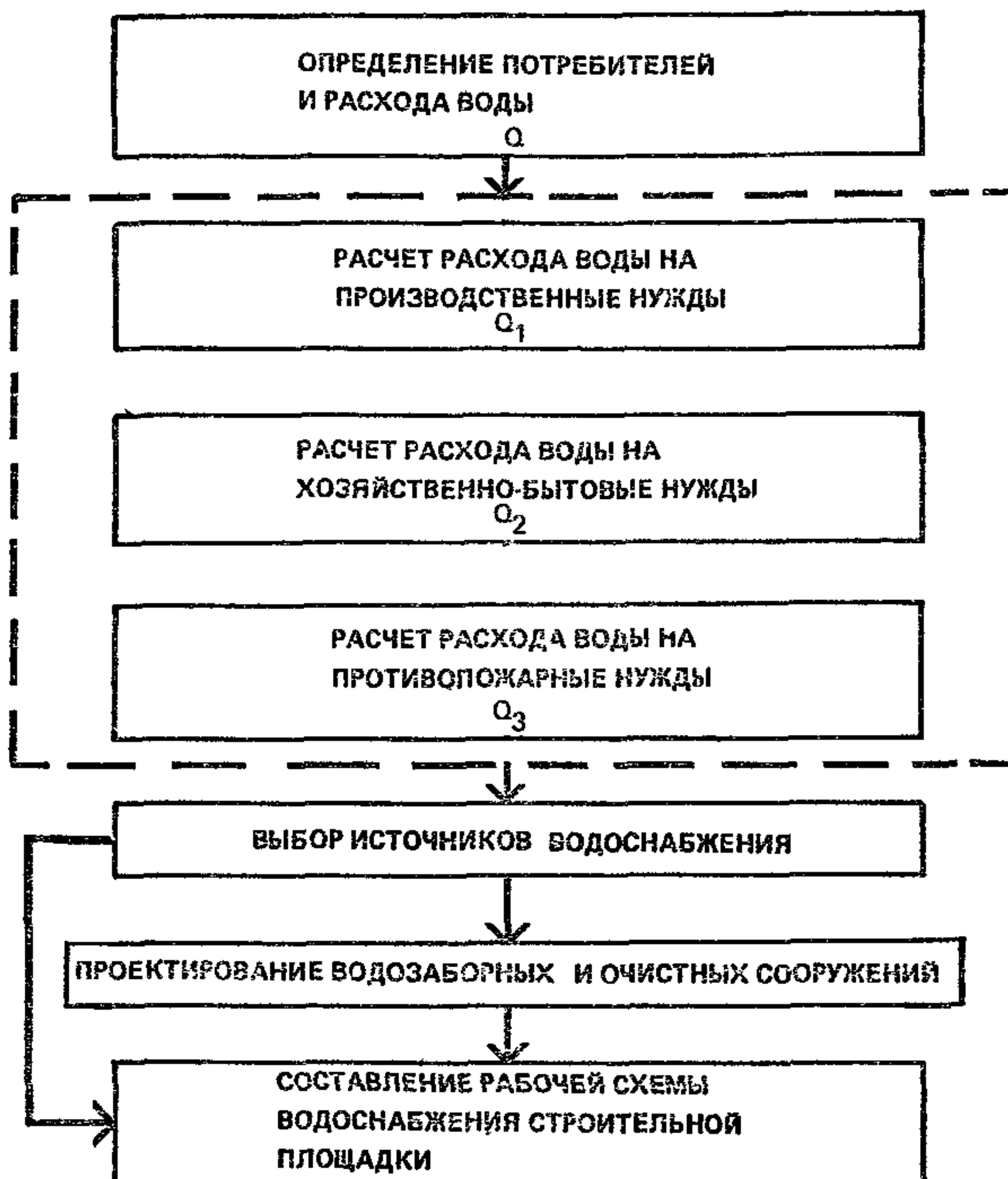
Рис. 3. Блок-схема водоснабжения строительной площадки
