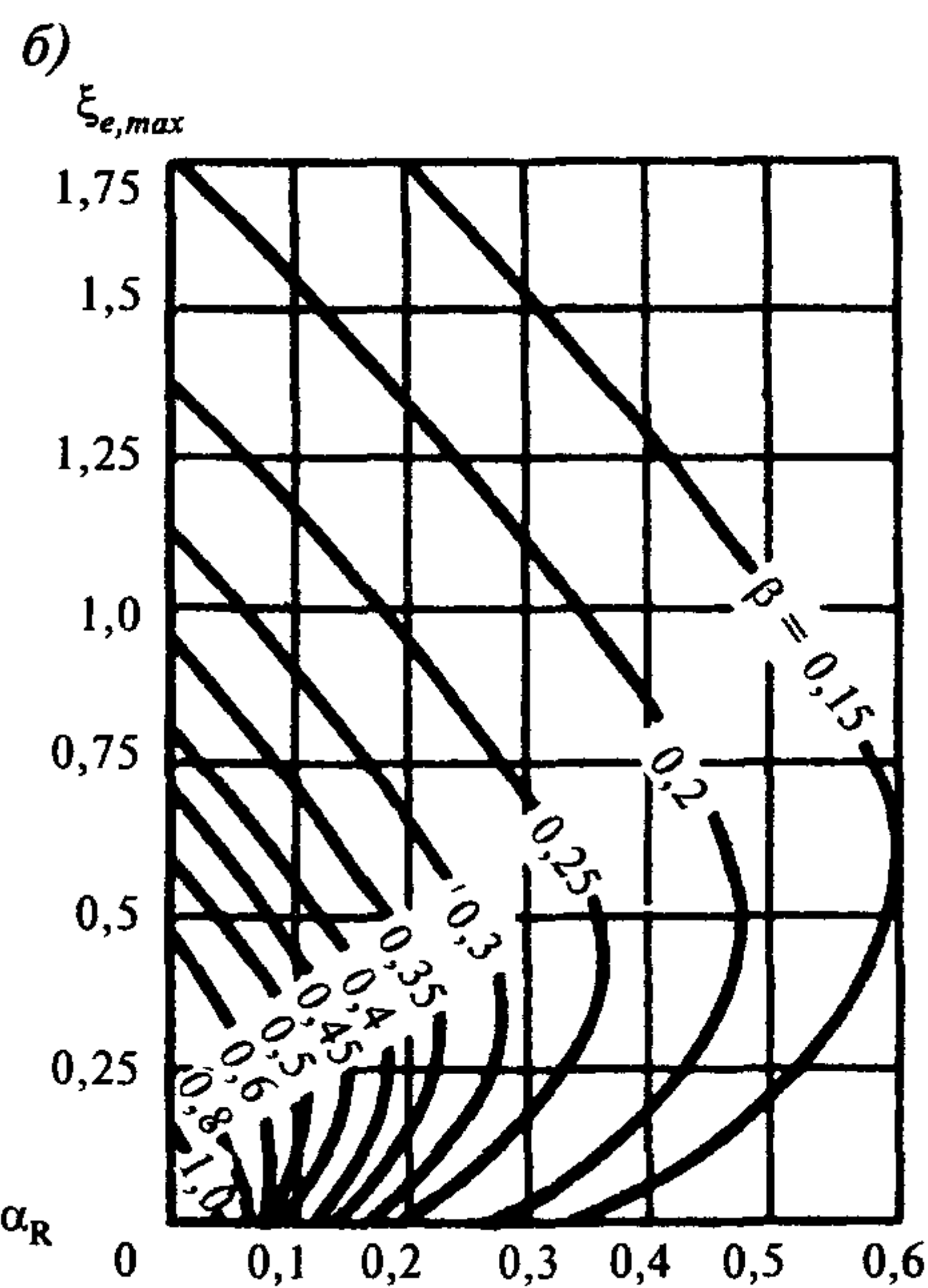
Черт. 3. Графики для определения коэффициентов:
