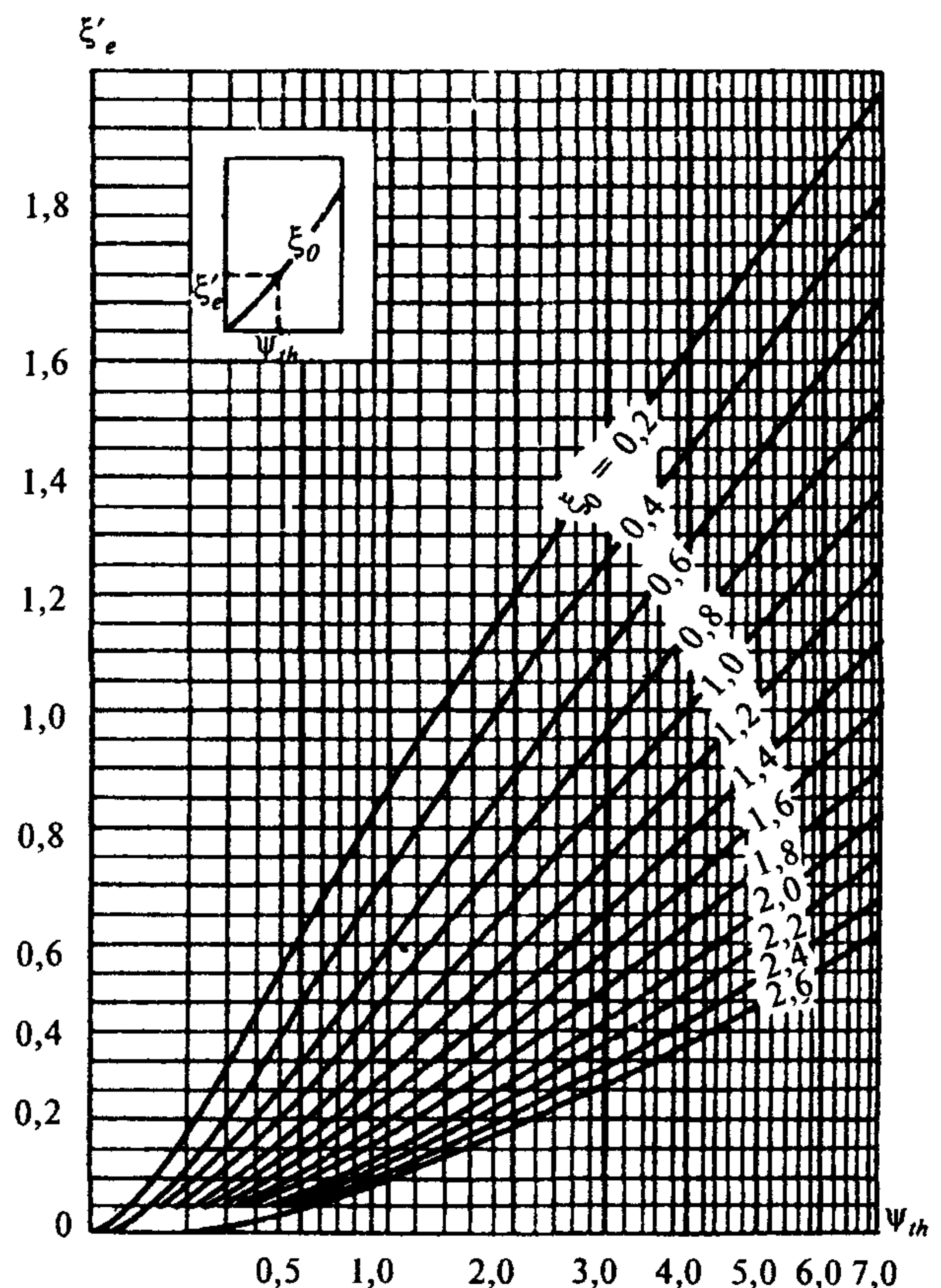
Черт. 6. Графики для определения коэффициента \xi'_e
