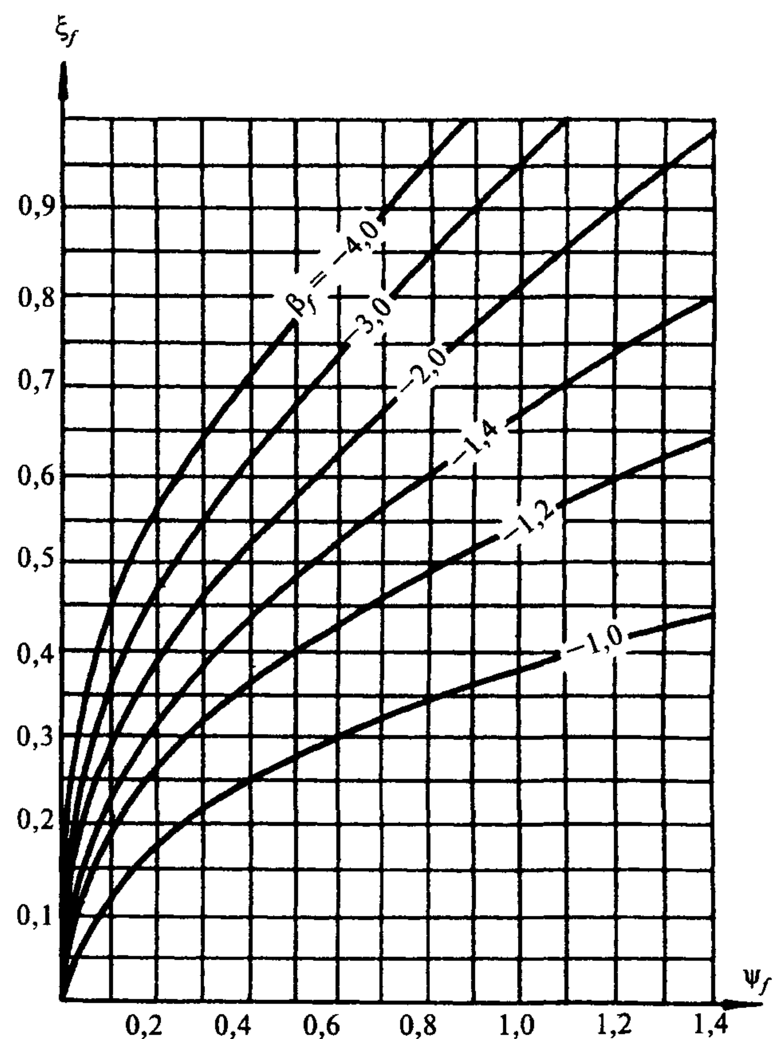
Черт. 1. Графики для определения коэффициента \beta_f
