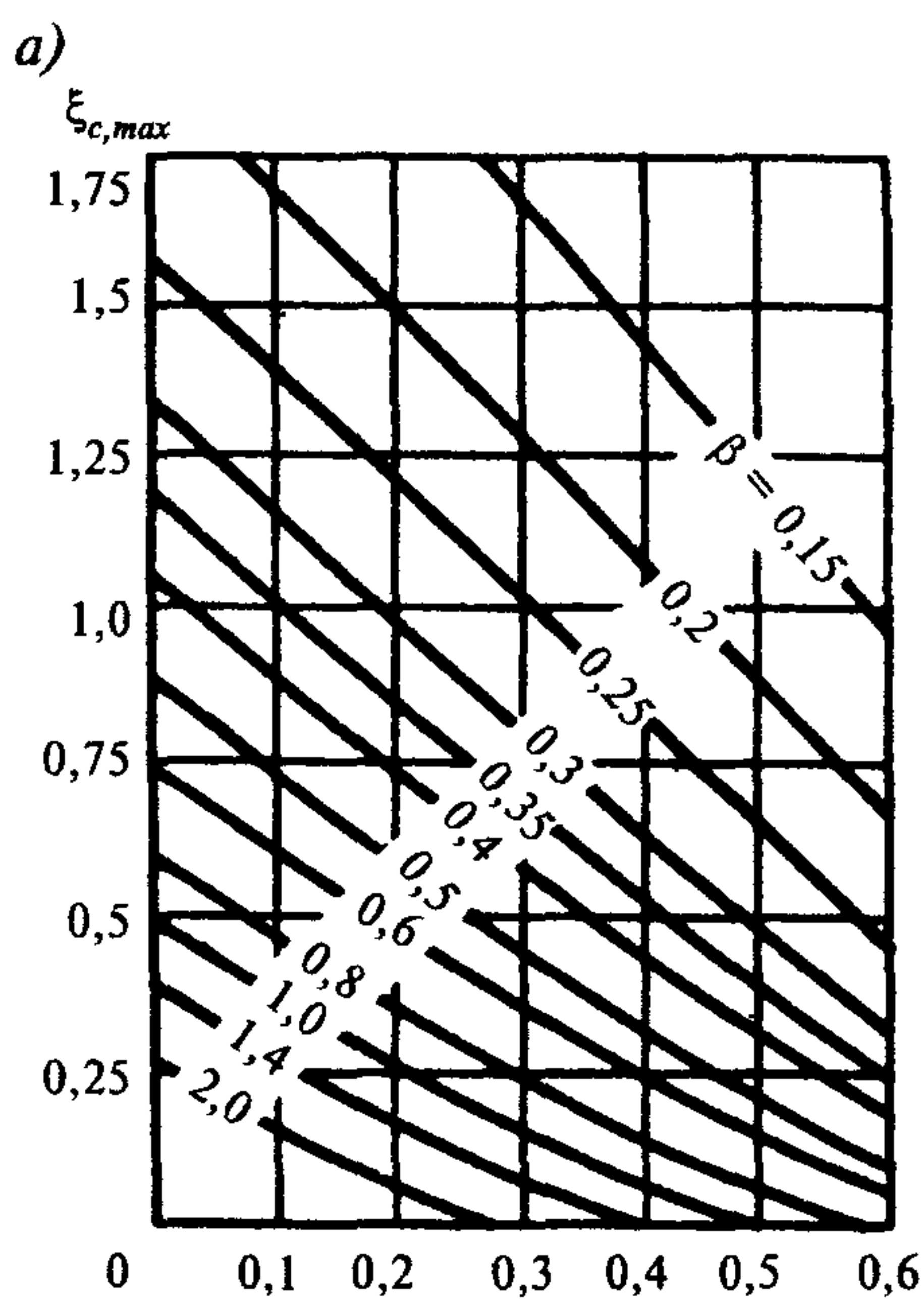
Черт. 1. Графики для определения коэффициентов \xi_c и k_c
