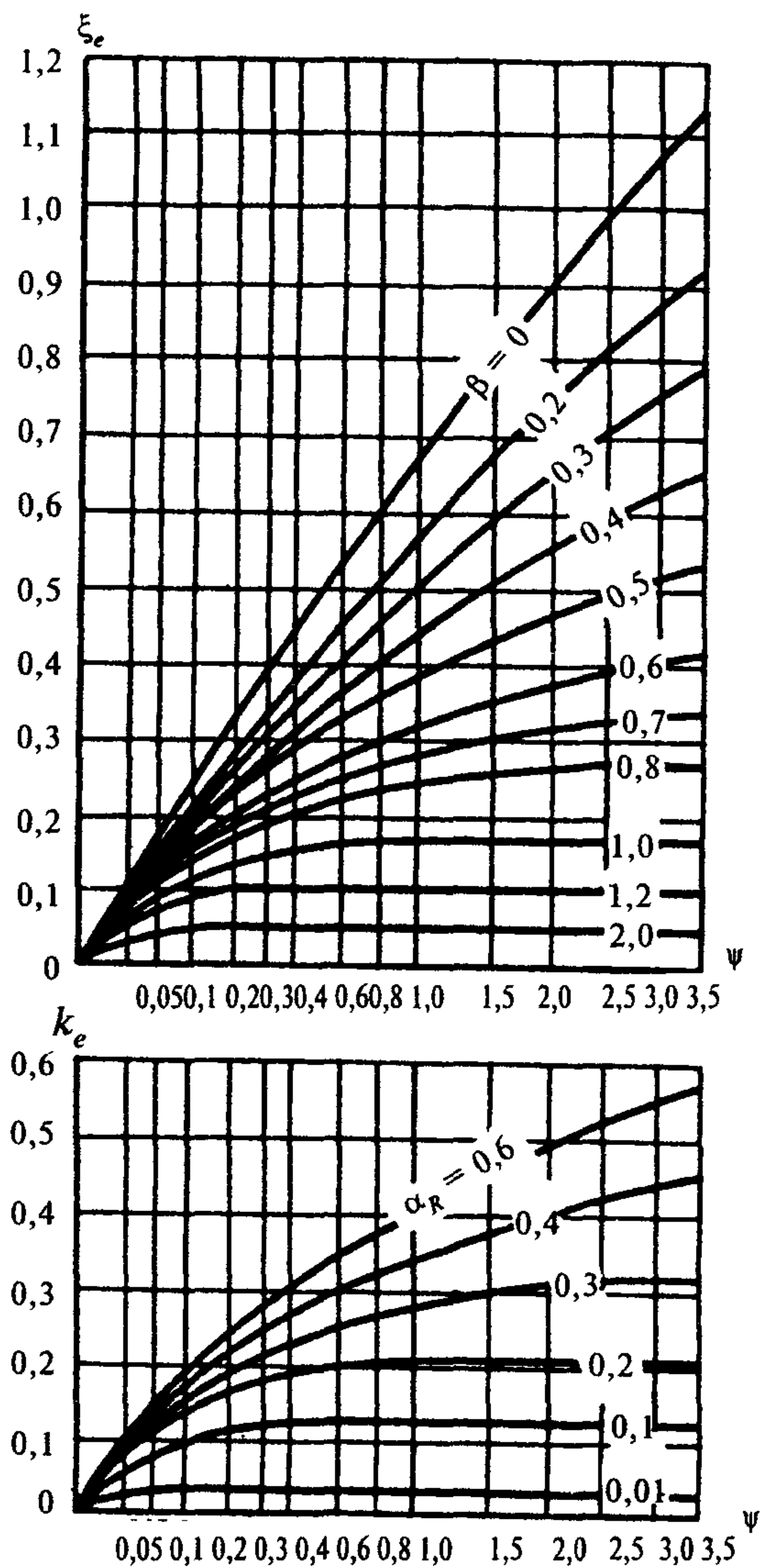
Черт. 2. Графики для определения коэффициентов \xi_e и k_e
