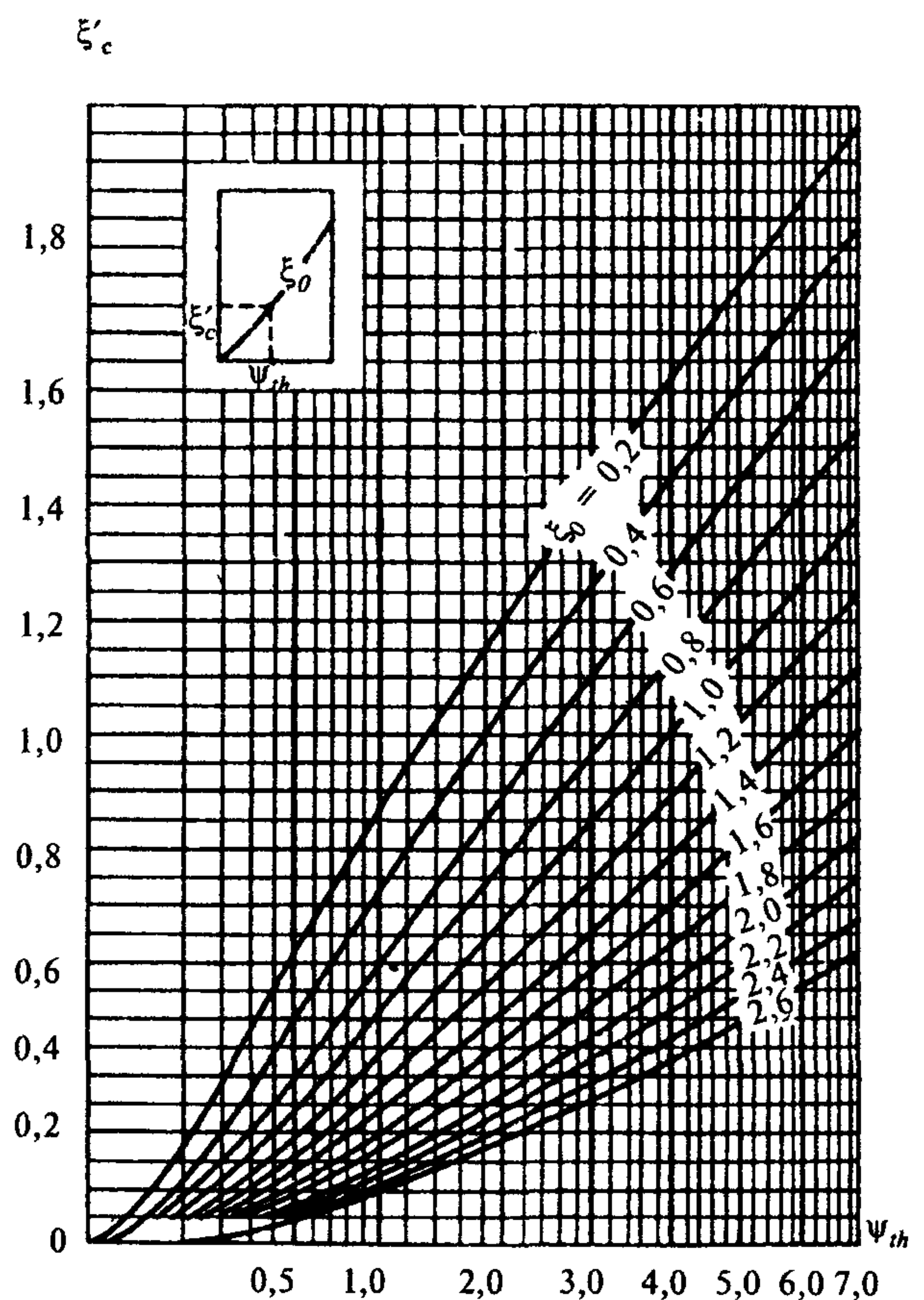
Черт. 5. Графики для определения коэффициента \xi'_c
