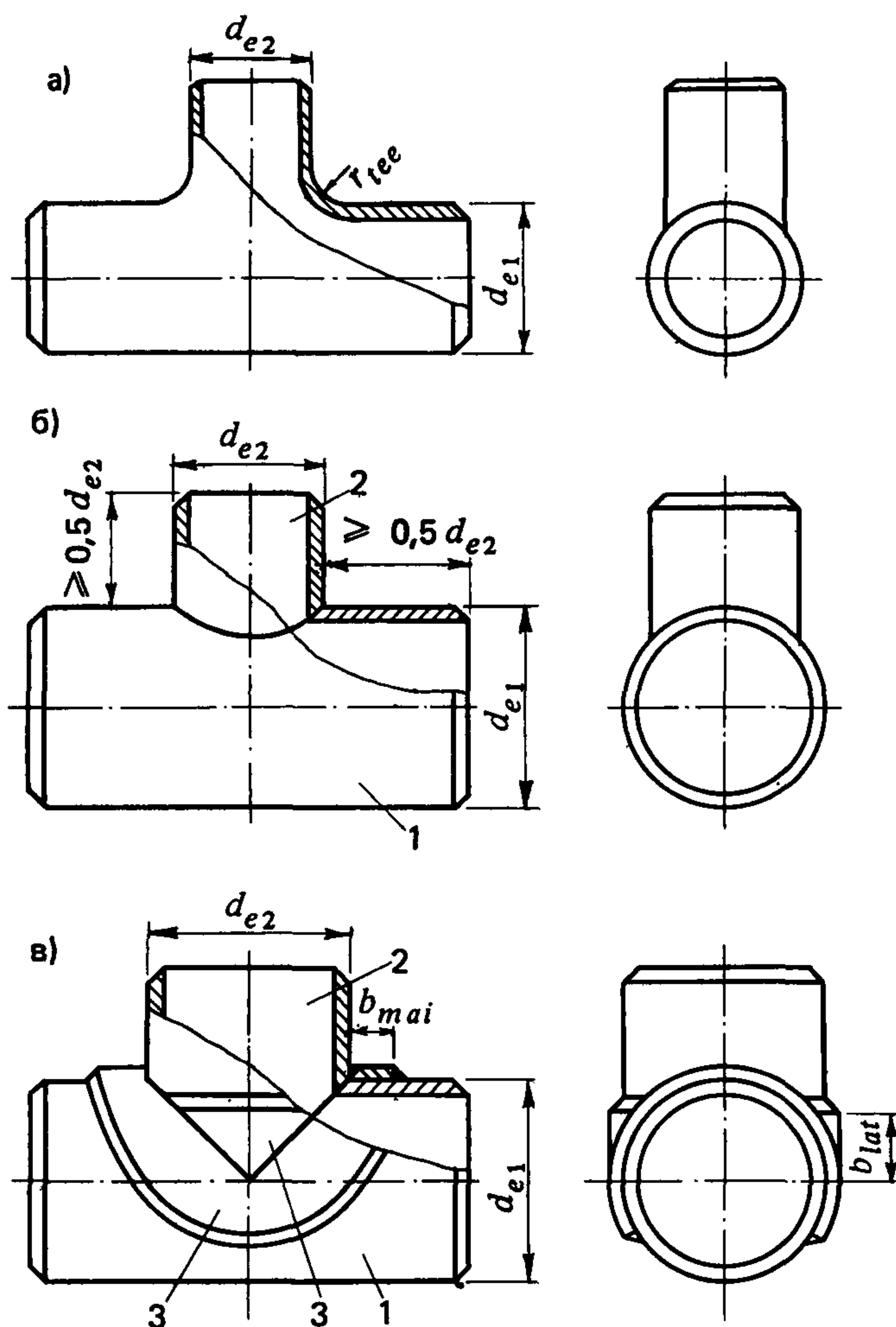
Черт. 1. Тройники
