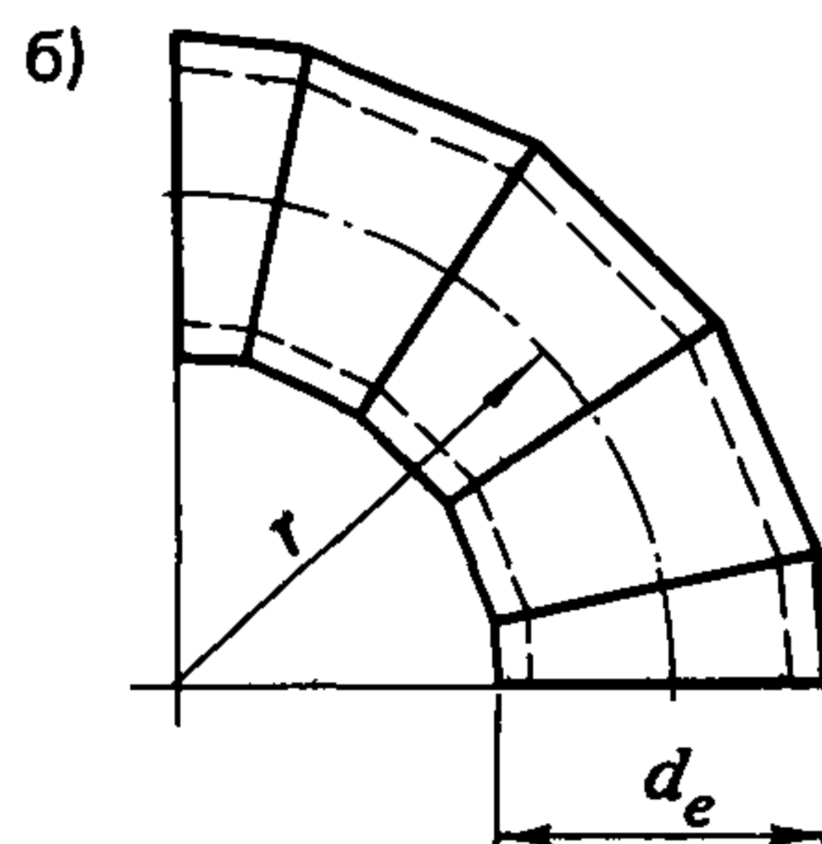
Черт. 4. Отводы
