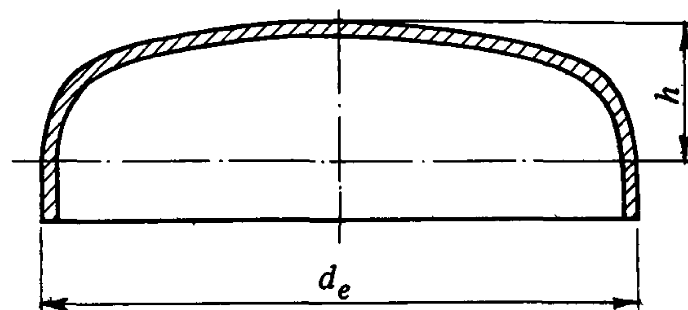
Черт. 3. Заглушка эллиптическая
