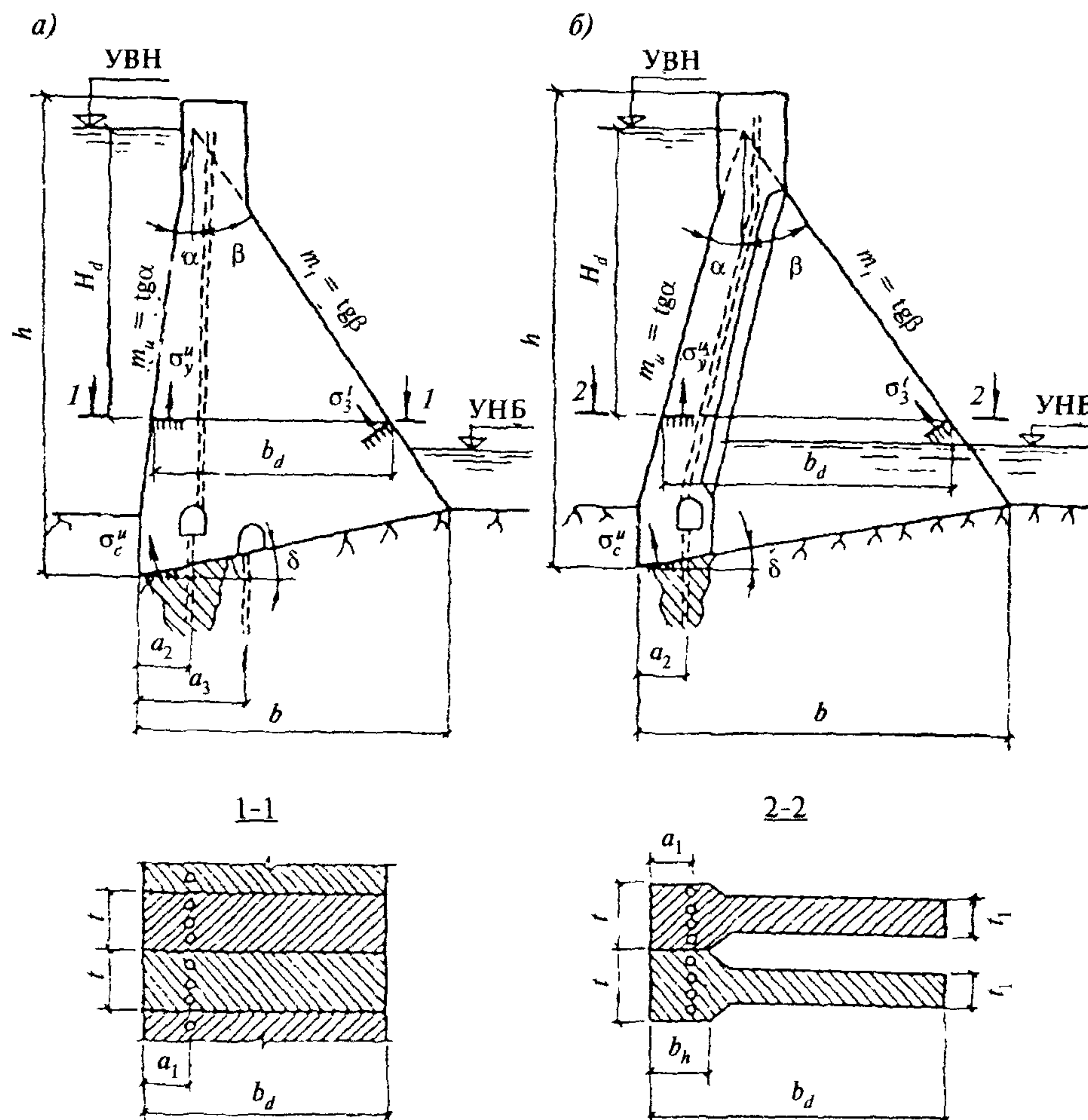
Черт. 10. Обозначения к расчету плотины на прочность
