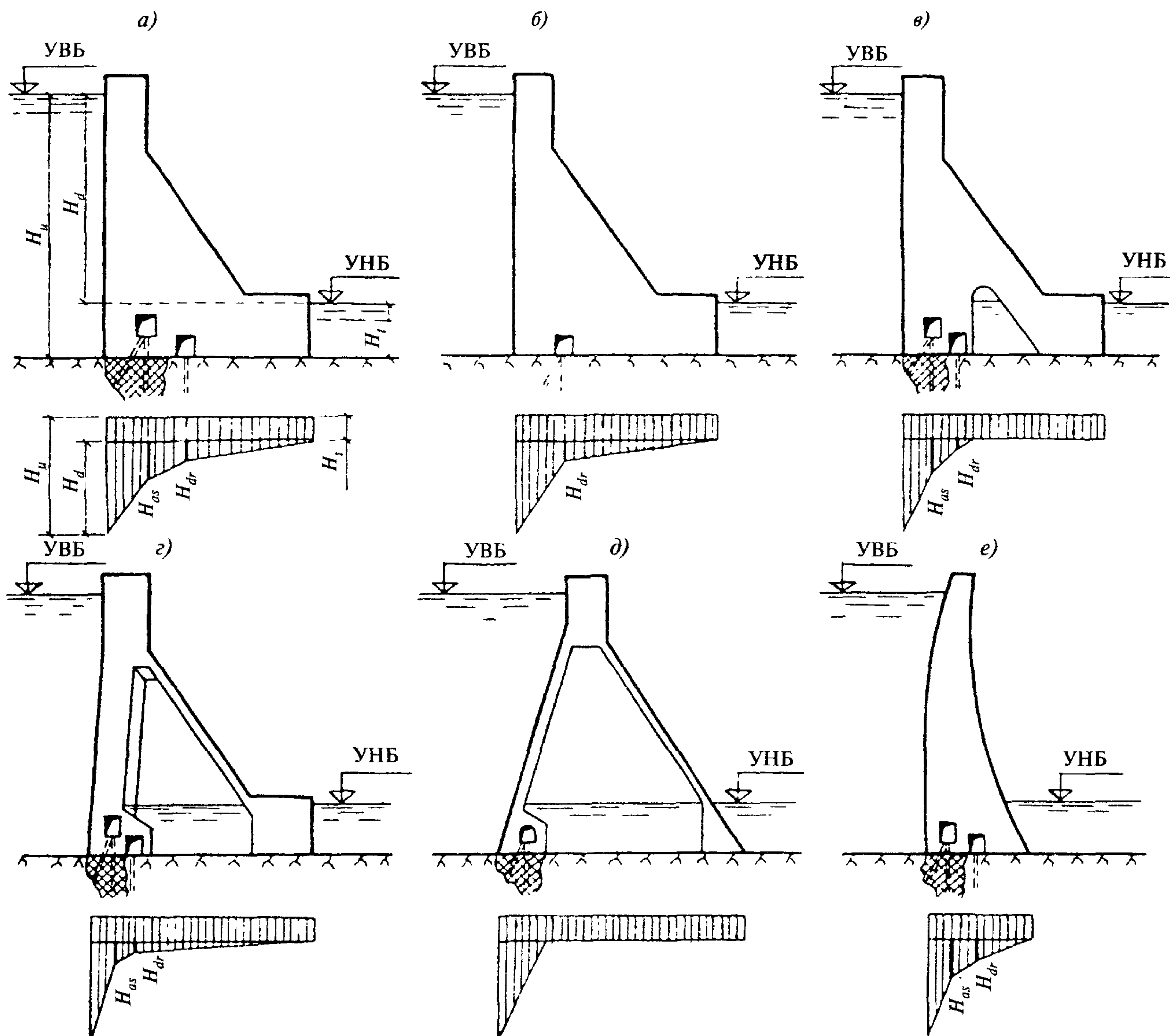
Черт. 7. Эпюры пьезометрического напора по подошве плотины
