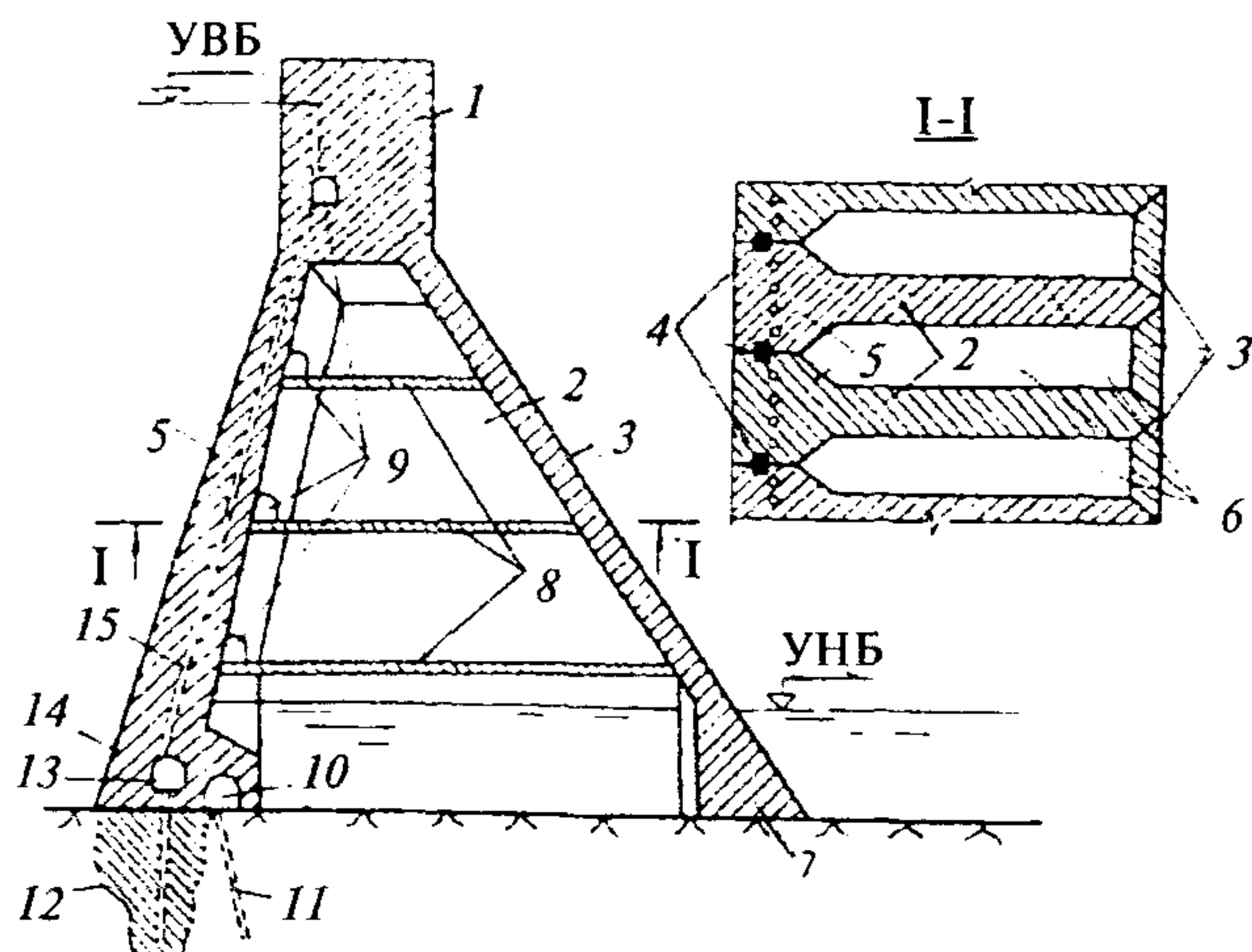
Черт. 11. Отдельные части и элементы массивно-контрфорсной плотины
