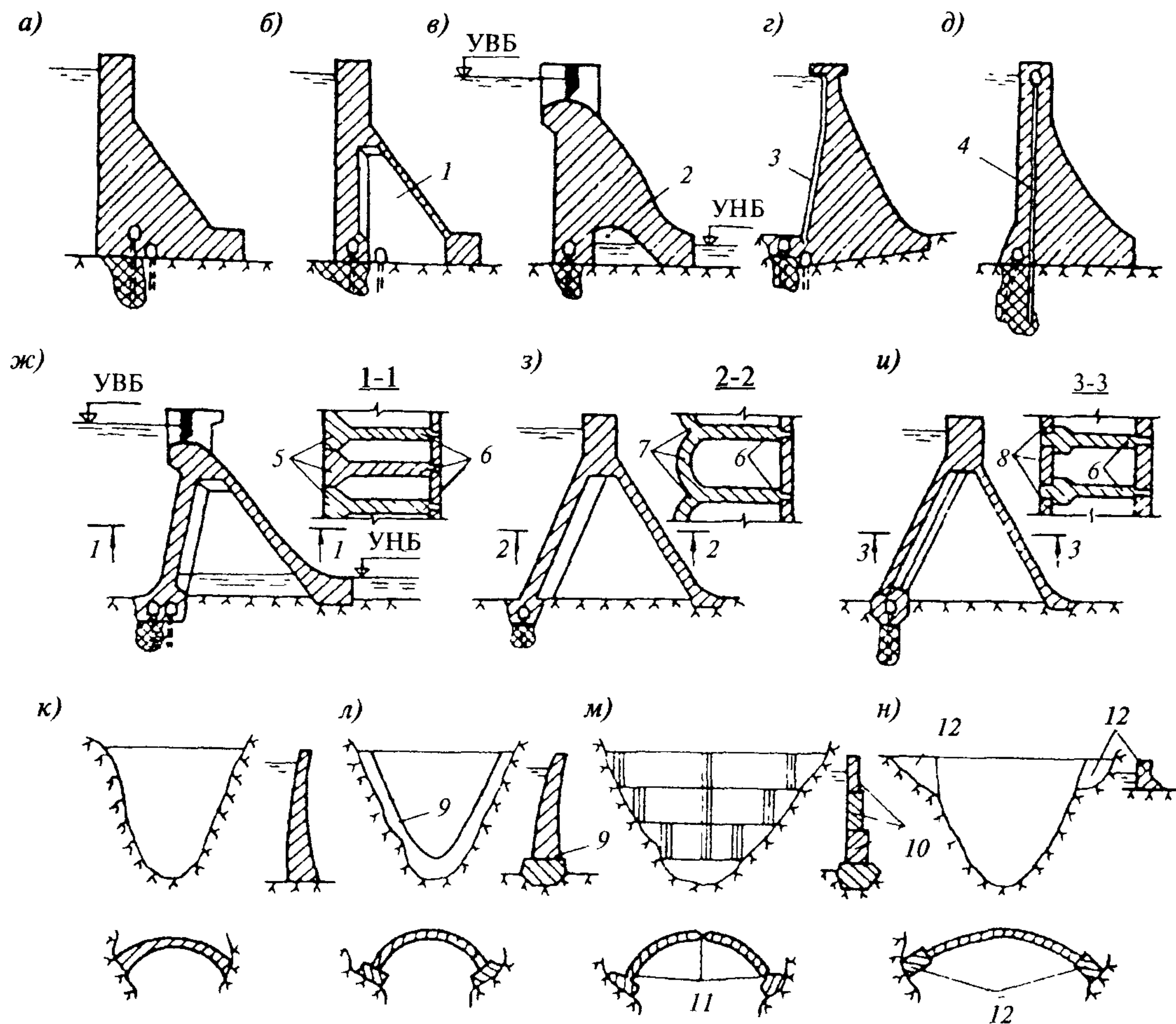
Черт. 1. Основные виды плотин на скальных основаниях
