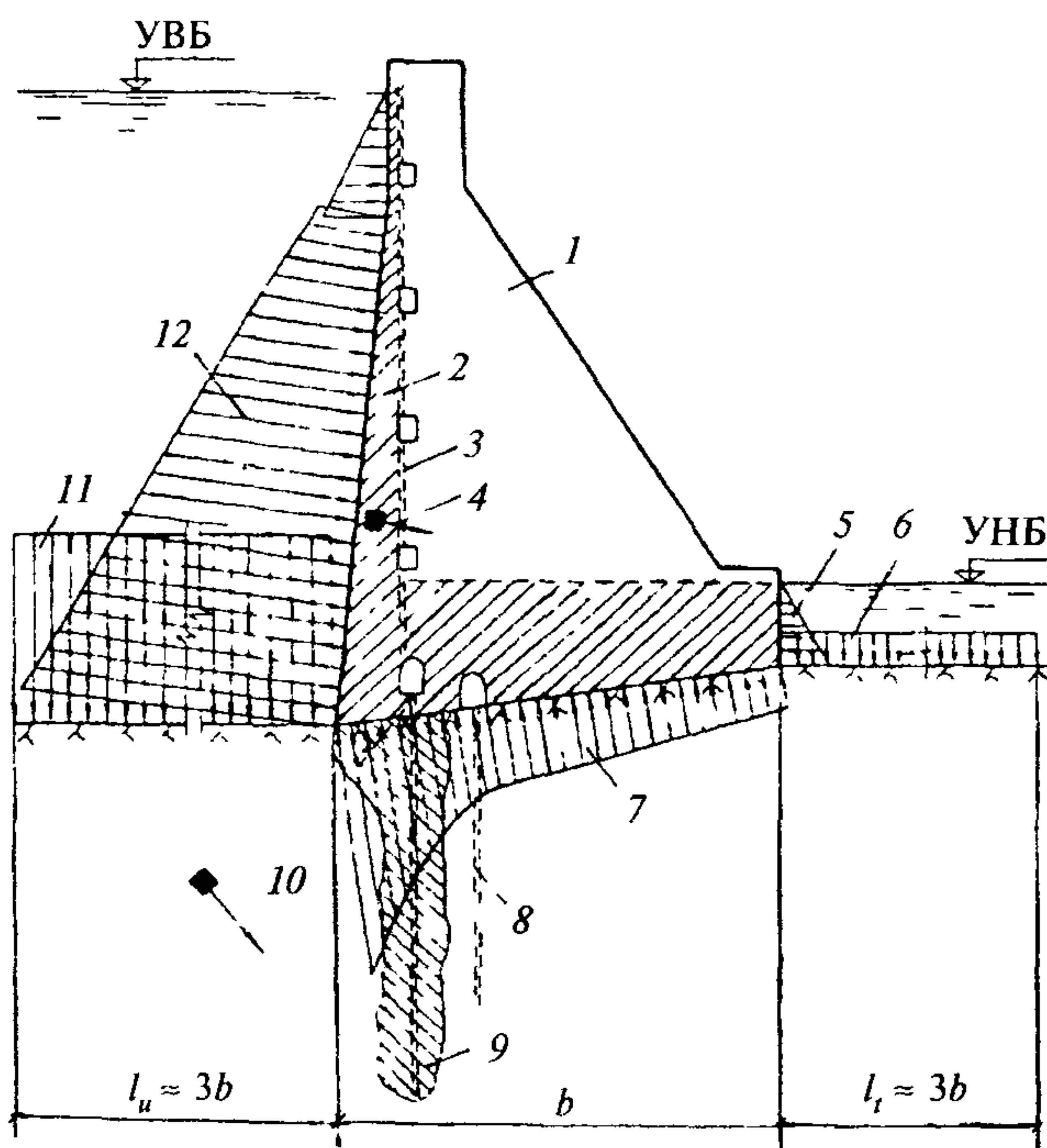
Черт. 6. Схема силового воздействия воды
