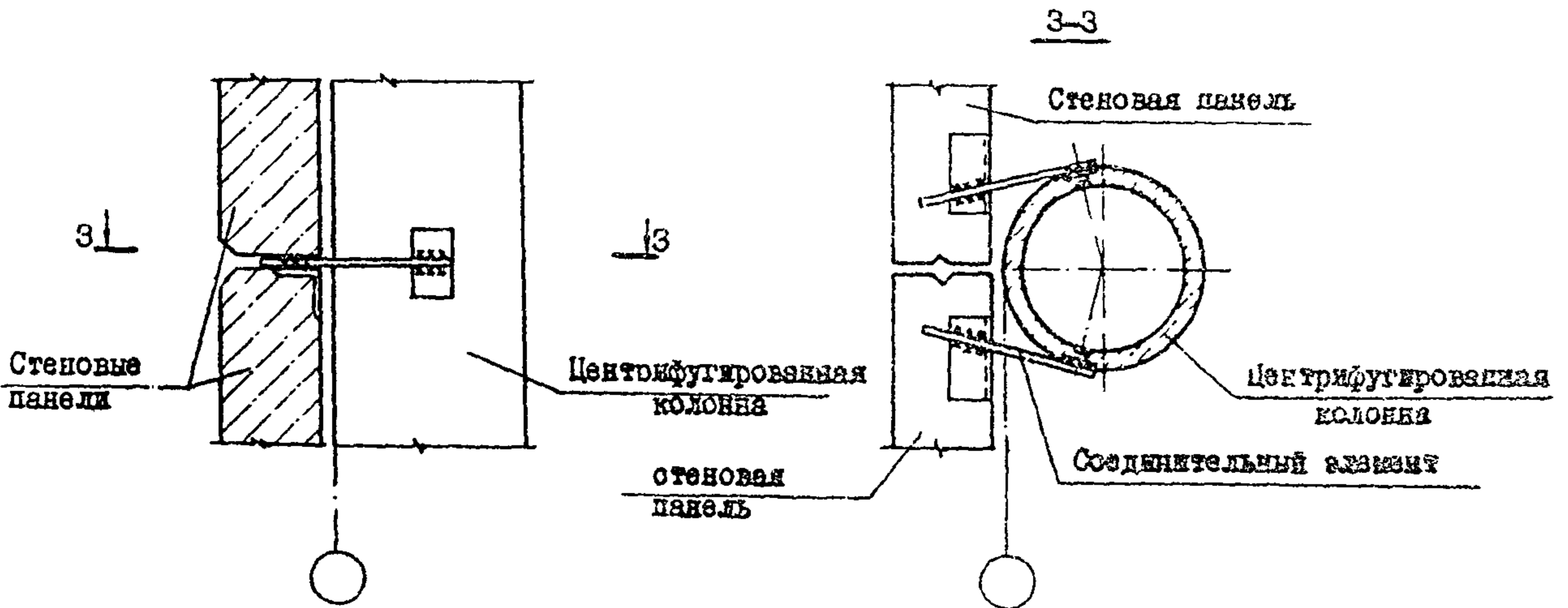
Сопряжение стеновых панелей с центрифугированной колонной
