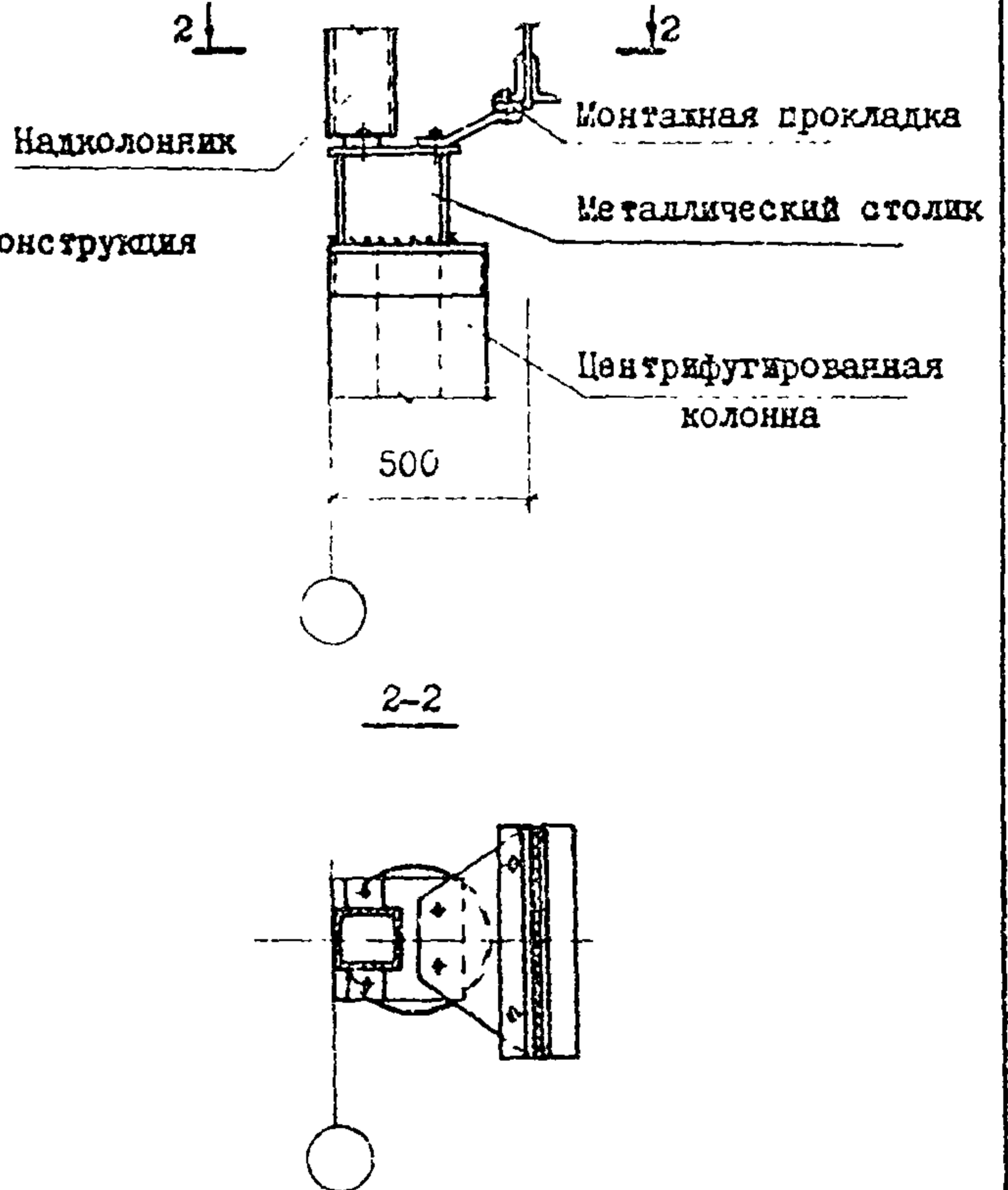
Сопряжение стеновых панелей с центрифугированной колонной
