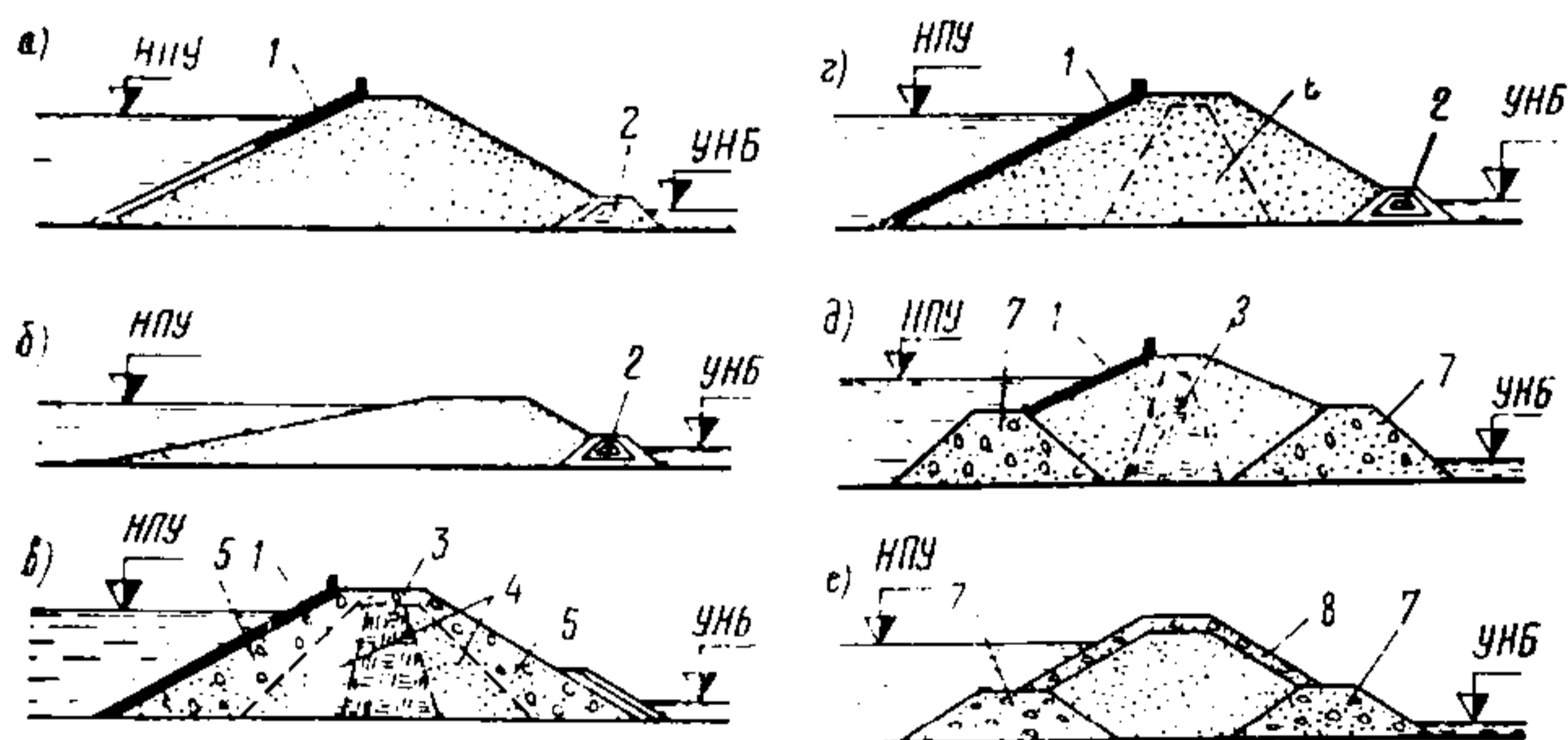
Рис. 4. Виды намывных плотин
