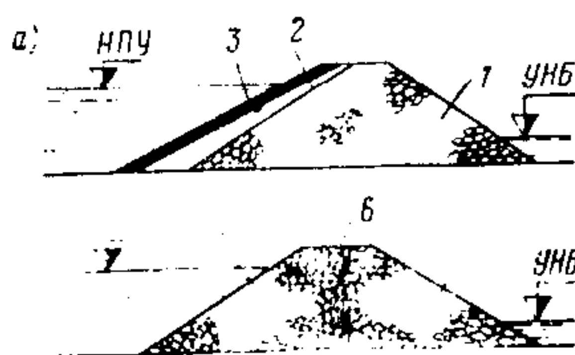
Рис. 8. Виды каменнонабросных плотин
