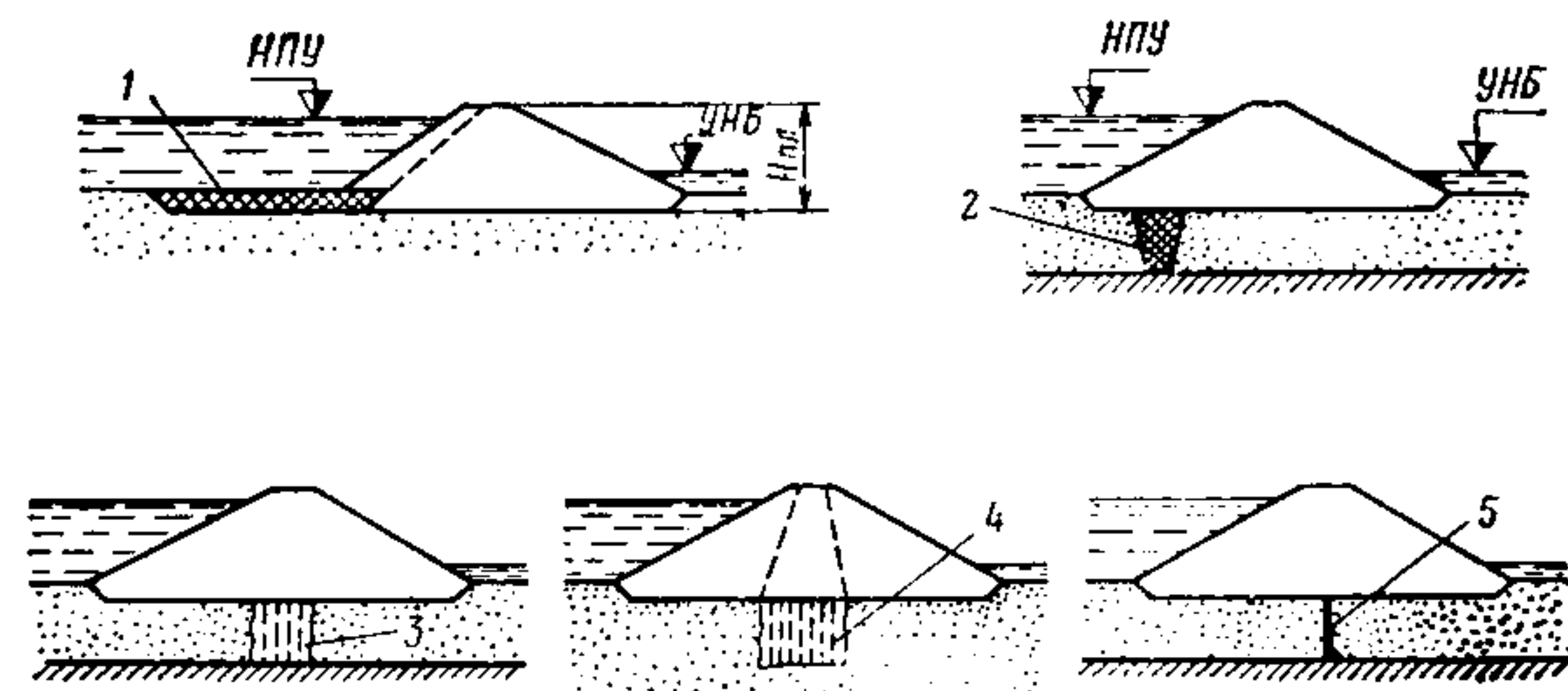
Рис. 2. Конструкции противофильтрационных устройств в основании 1 — понур; 2 — зуб; 3 — инъекционная завеса; 4 — то же, висячая; 5 — диафрагма (стенка, шпунт)
