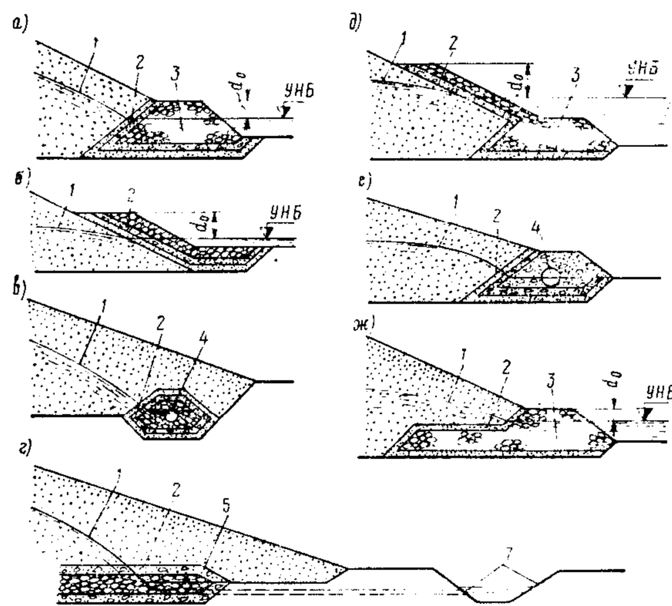
Рис. 3. Схемы основных видов дренажа а — дренажный банкет; б — наклонный дренаж; в — трубчатый дренаж; г — горизонтальный дренаж; д, е, ж — комбинированный тип дренажа; 1 — кривая депрессии; 2 — обратный фильтр; 3 — банкет; 4 — труба; 5 — дренажная лента; 6 — отводящая труба; 7 — отводящая канава
