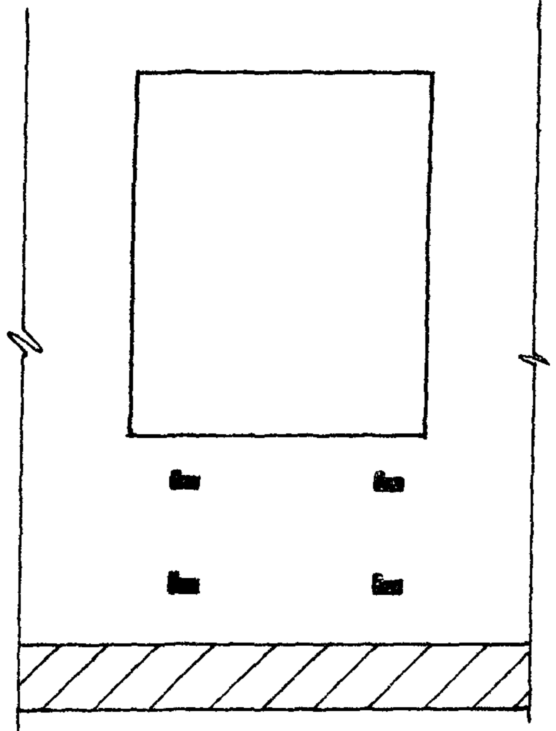
Пристрелка кронштейнов к стене строительным-монтажным пистолетом
