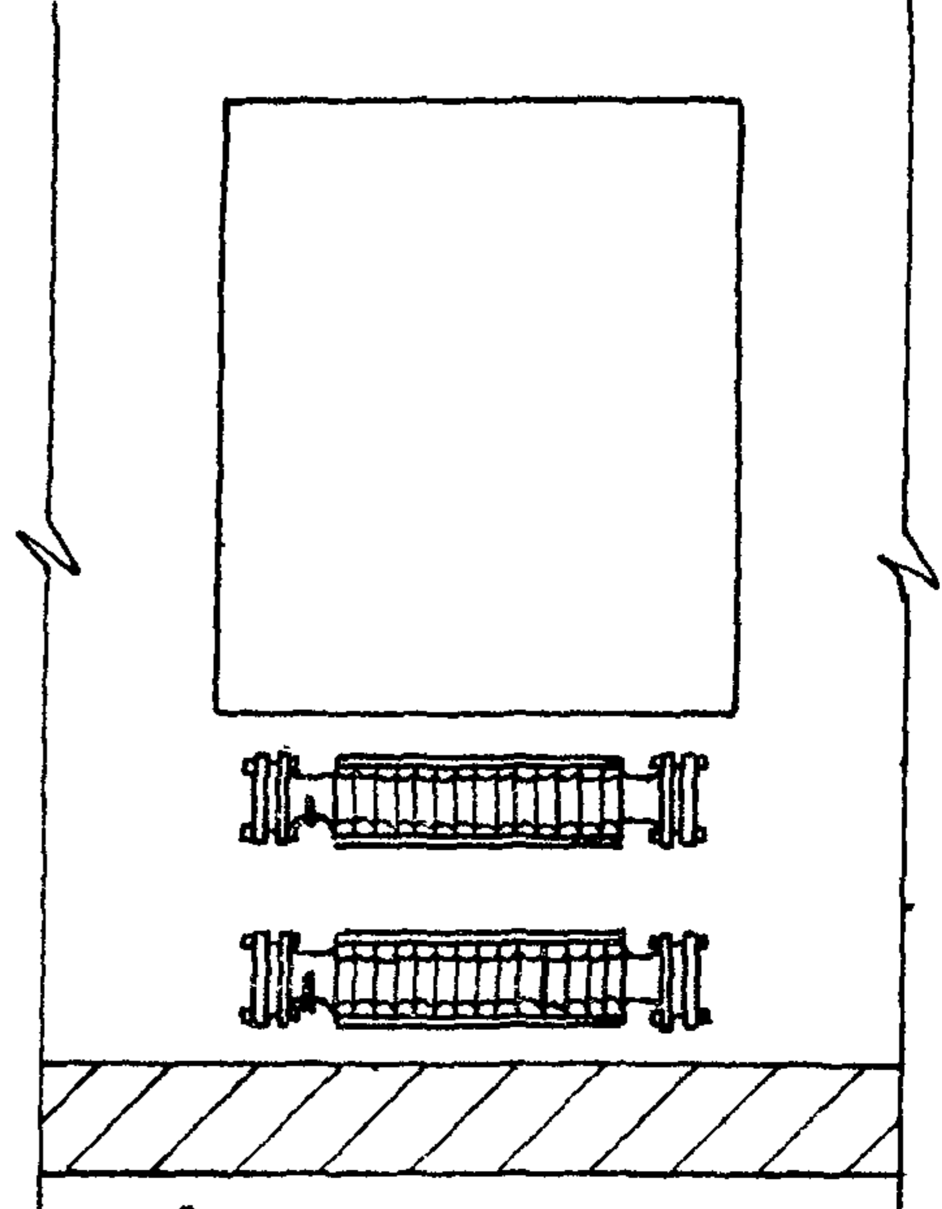
Навеска ребристых труб с фланцами и выверка по уровню
