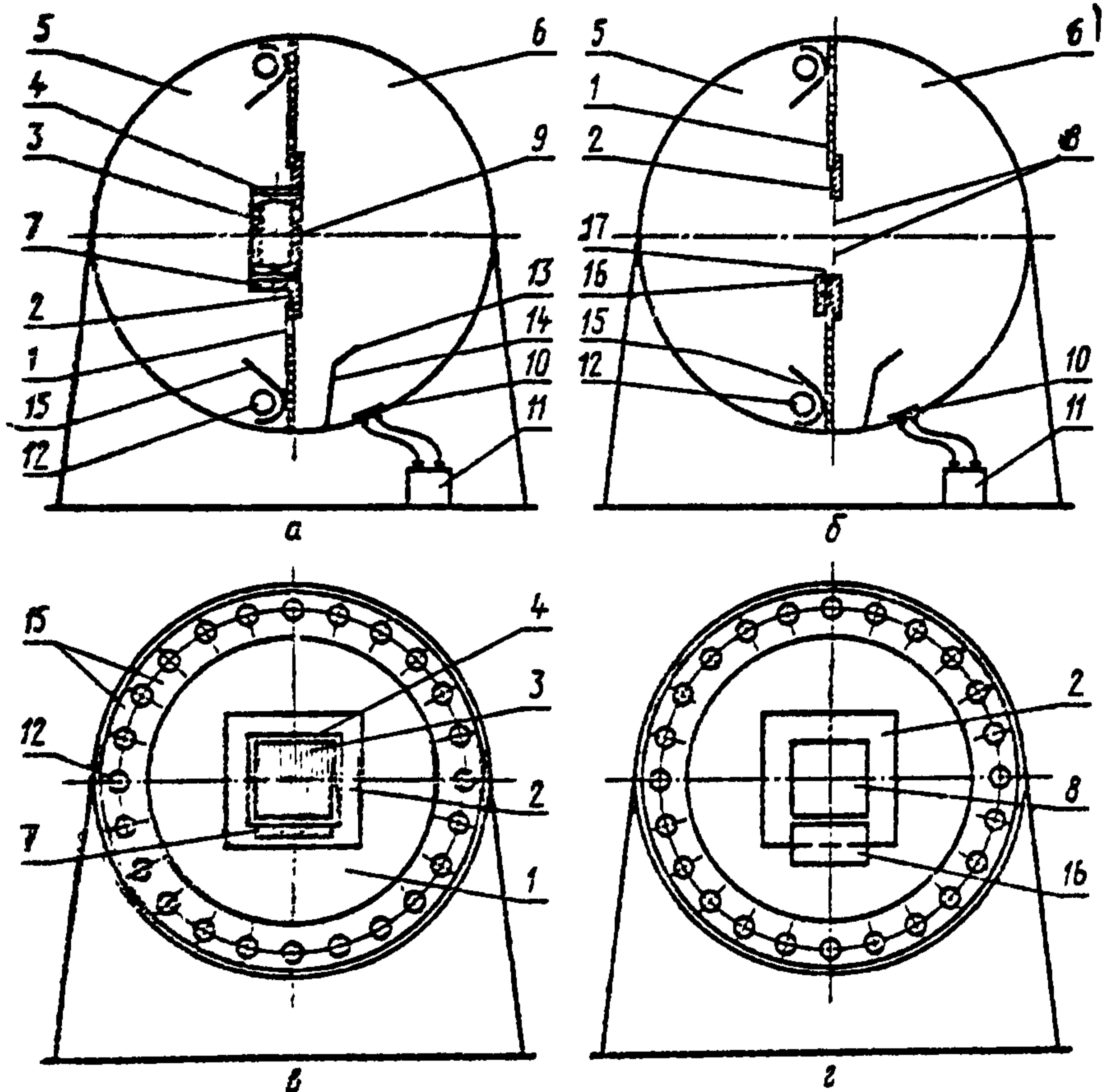
Схема диффузометра
