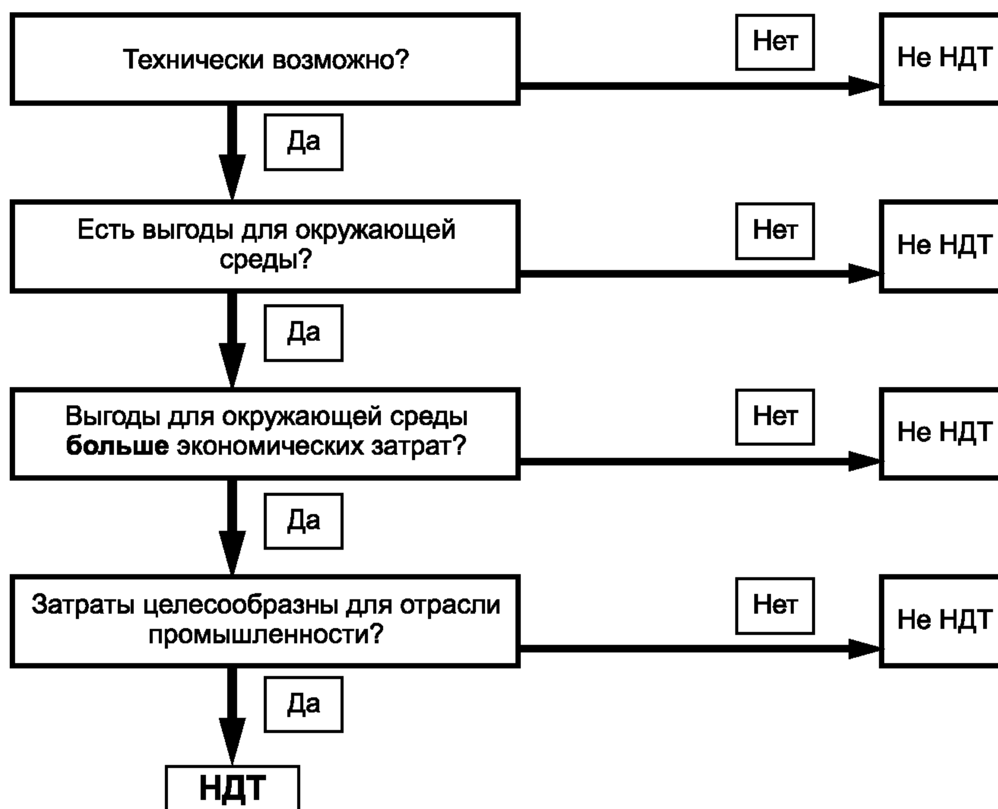
Рисунок 1 — Логический подход для принятия решения по НДТ
