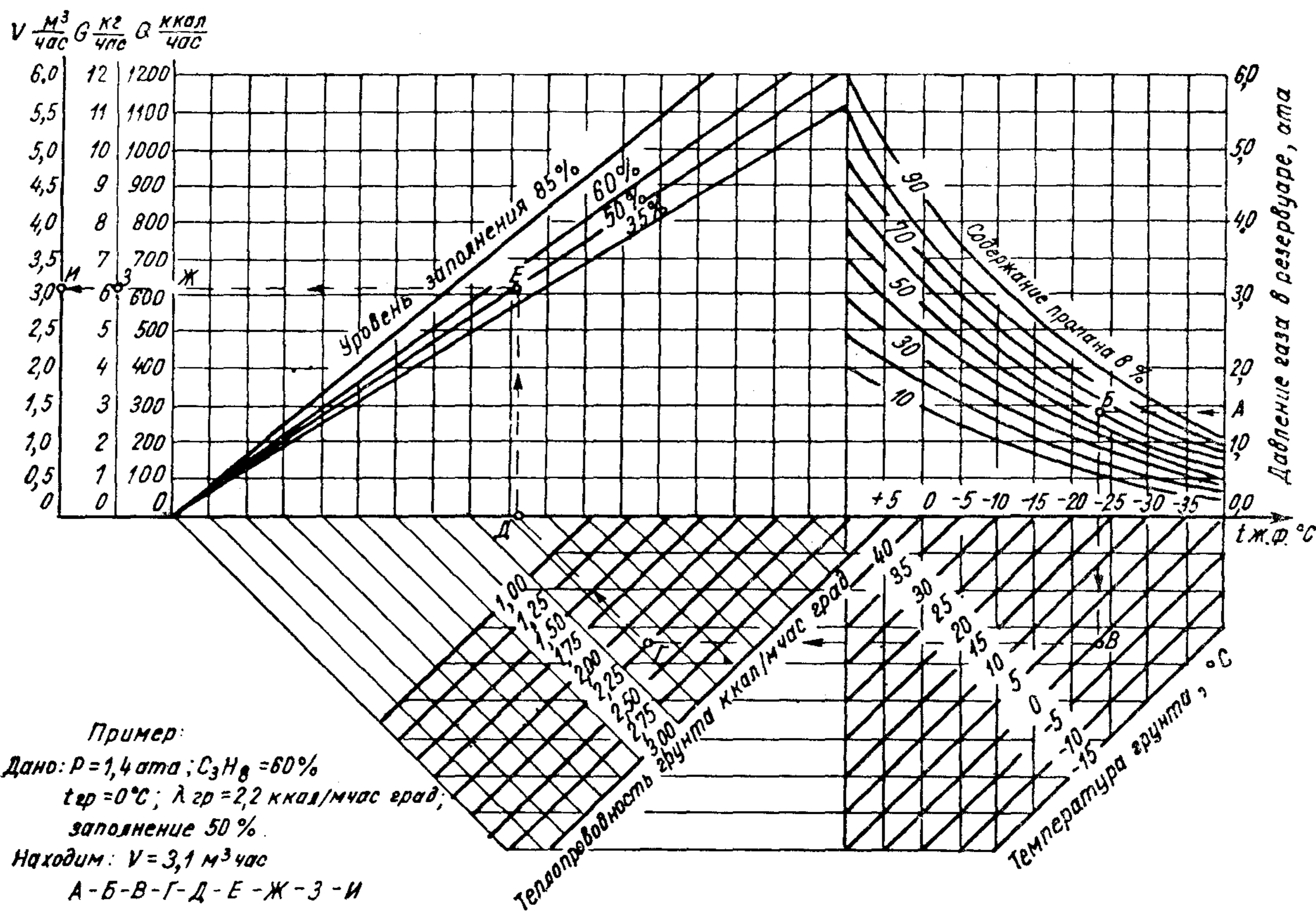
Номограмма для определения производительности резервуара (подземного) сжиженного газа объемом 4,4 м 3
