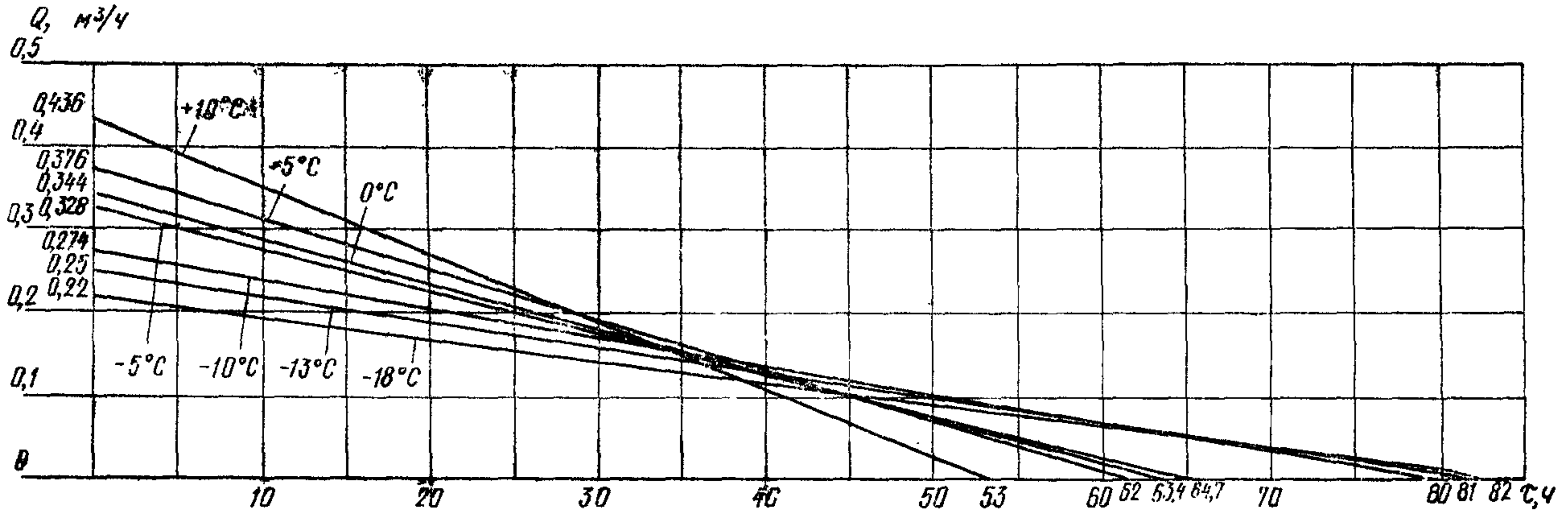
Рис. 1. Зависимость производительности однобаллонной установки от времени испарения
