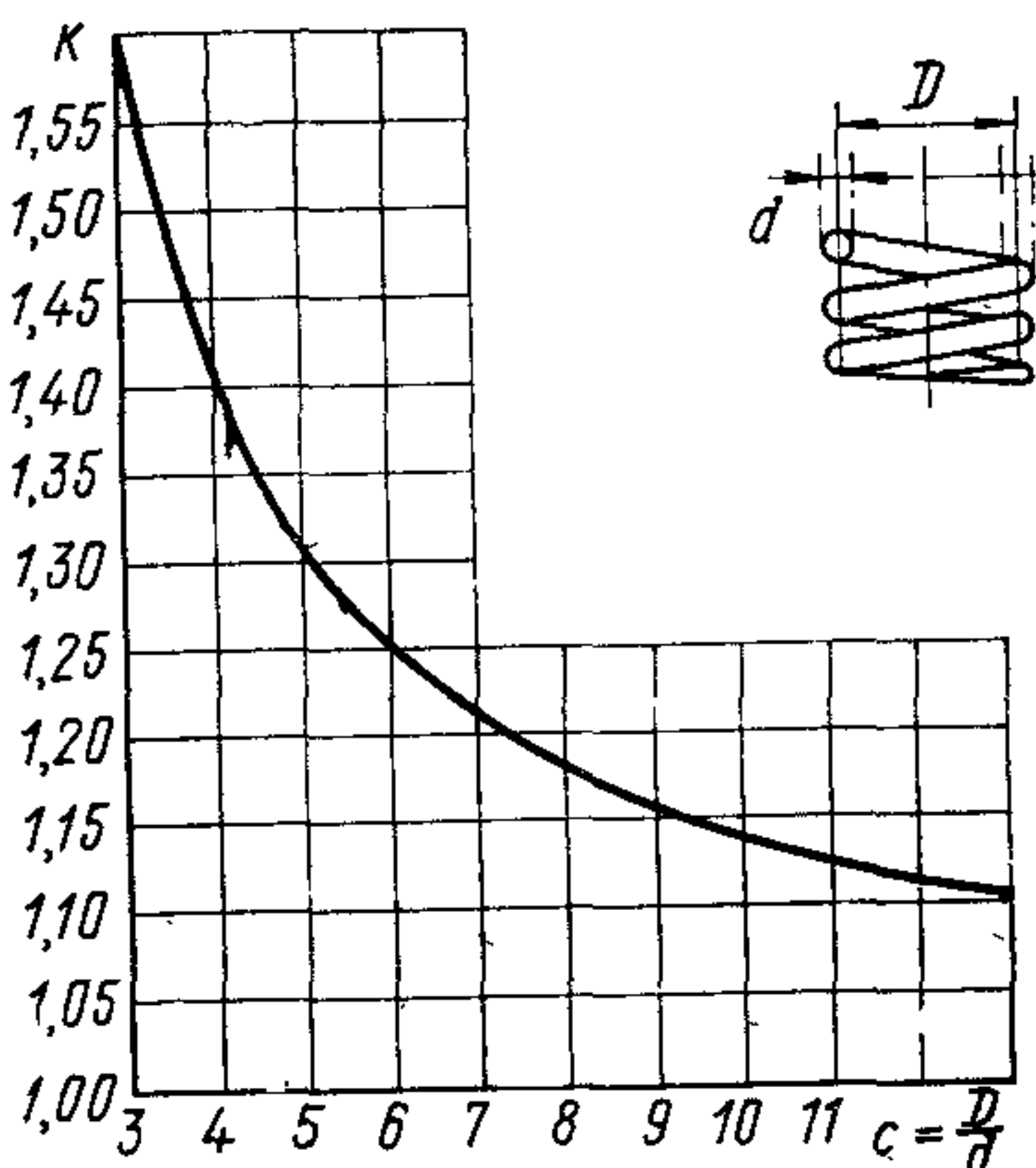
Рис. 5.1. График определения коэффициента k
