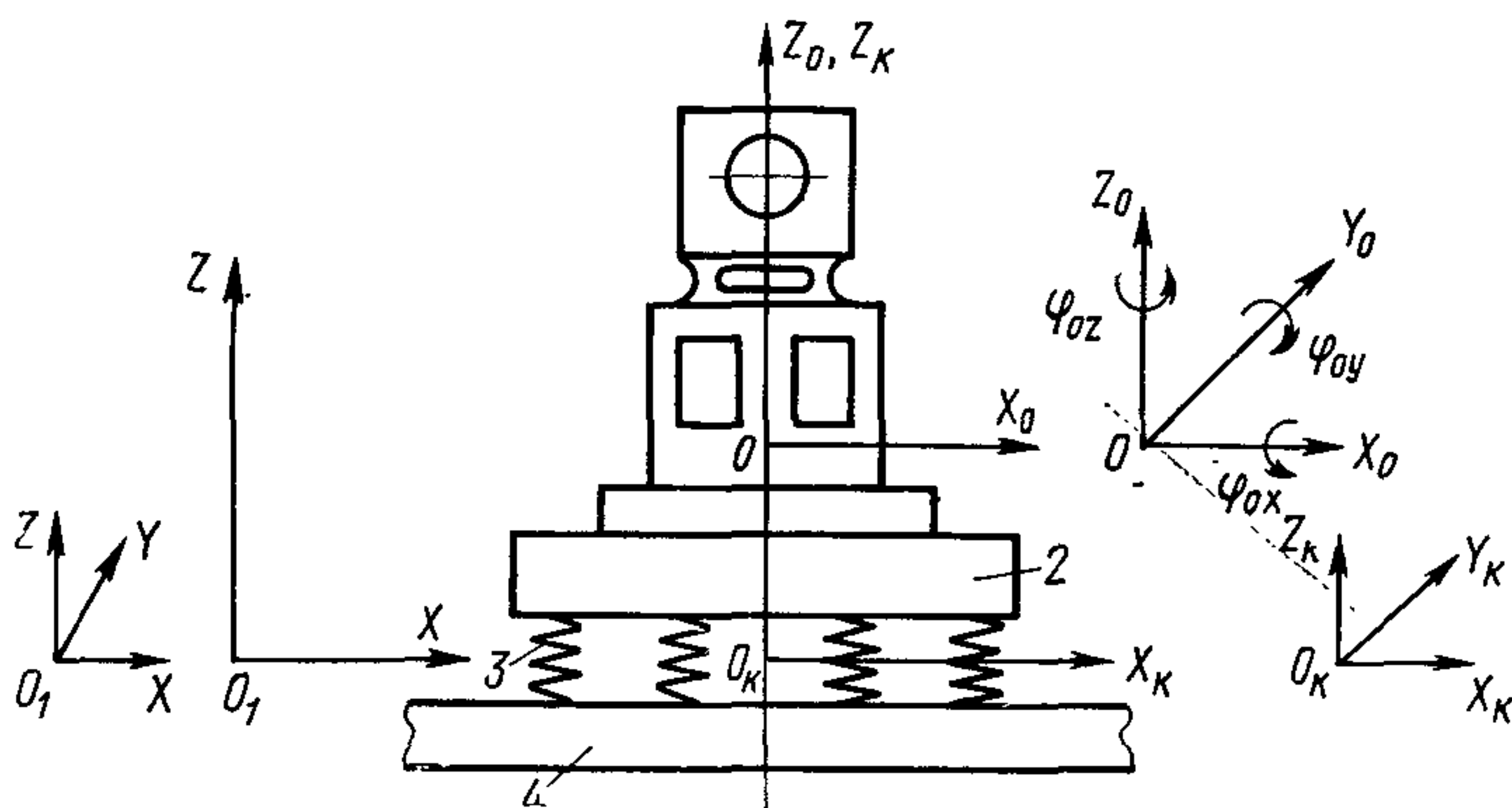
Рис. 2.2. Схема расположения осей координат, принимаемая при расчете виброизоляции машин
