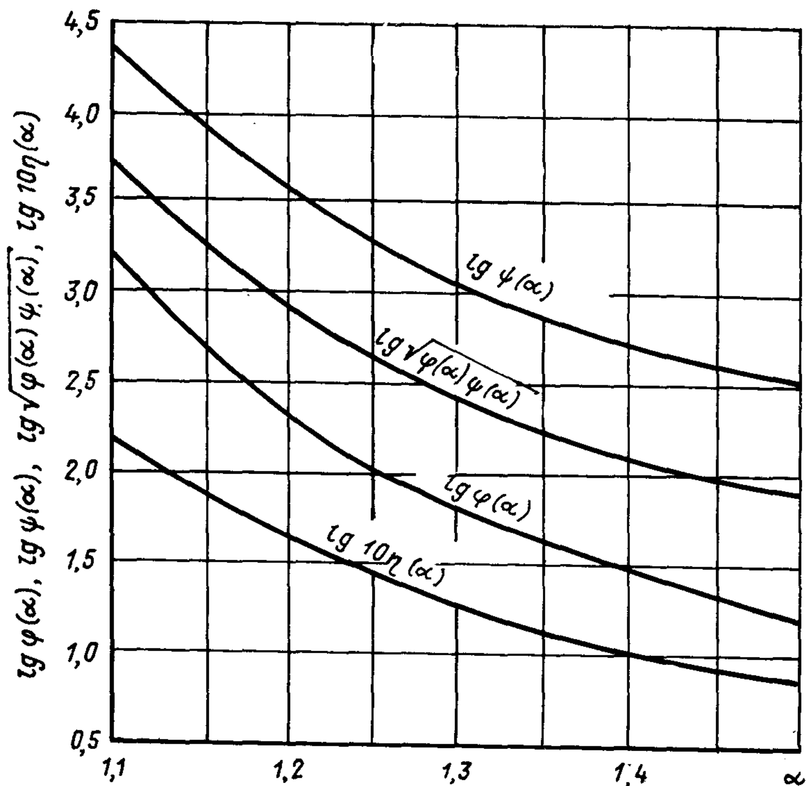
Рис. 6.5. Графики к расчету демпфера с двухкомпонентной жидкостью
