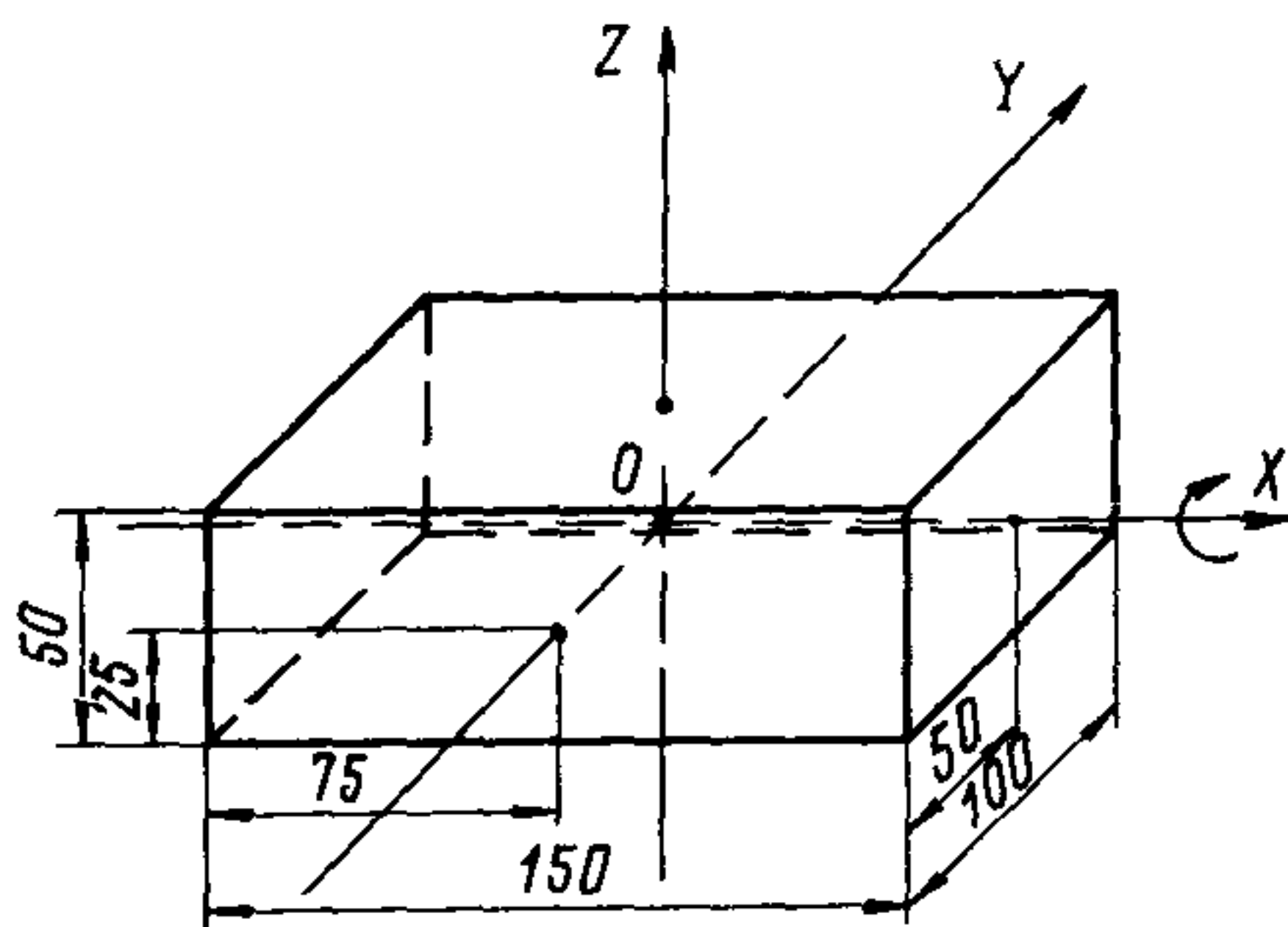
Рис. 9. К примеру расчета пассивной виброизоляции. Общий вид объекта и расположение координатных осей O — центр тяжести объекта (размеры даны в см)
