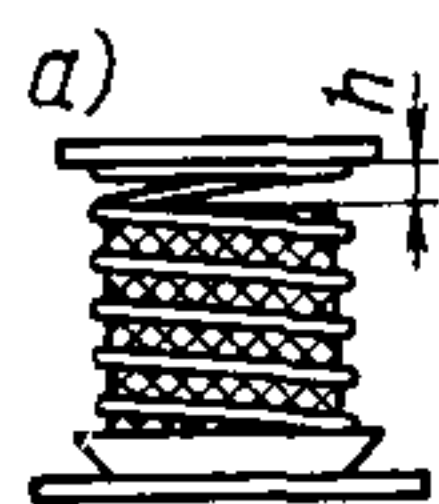
Рис. 5.8. Схемы комбинированных пружинно-пластмассовых виброизоляторов
