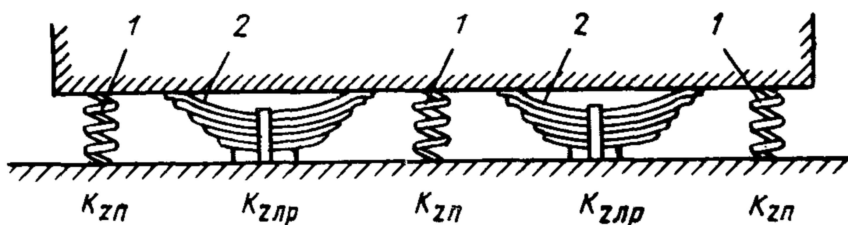
Рис. 3.2. Схема комбинированного виброизолятора при параллельном соединении пружин и листовых рессор 1 — пружины; 2 — листовые рессоры
