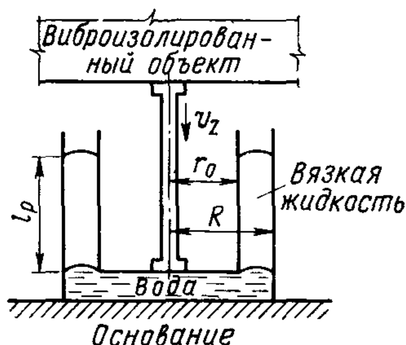
Рис. 6.4. Схема демпфера вязкого трения с двухкомпонентной жидкостью
