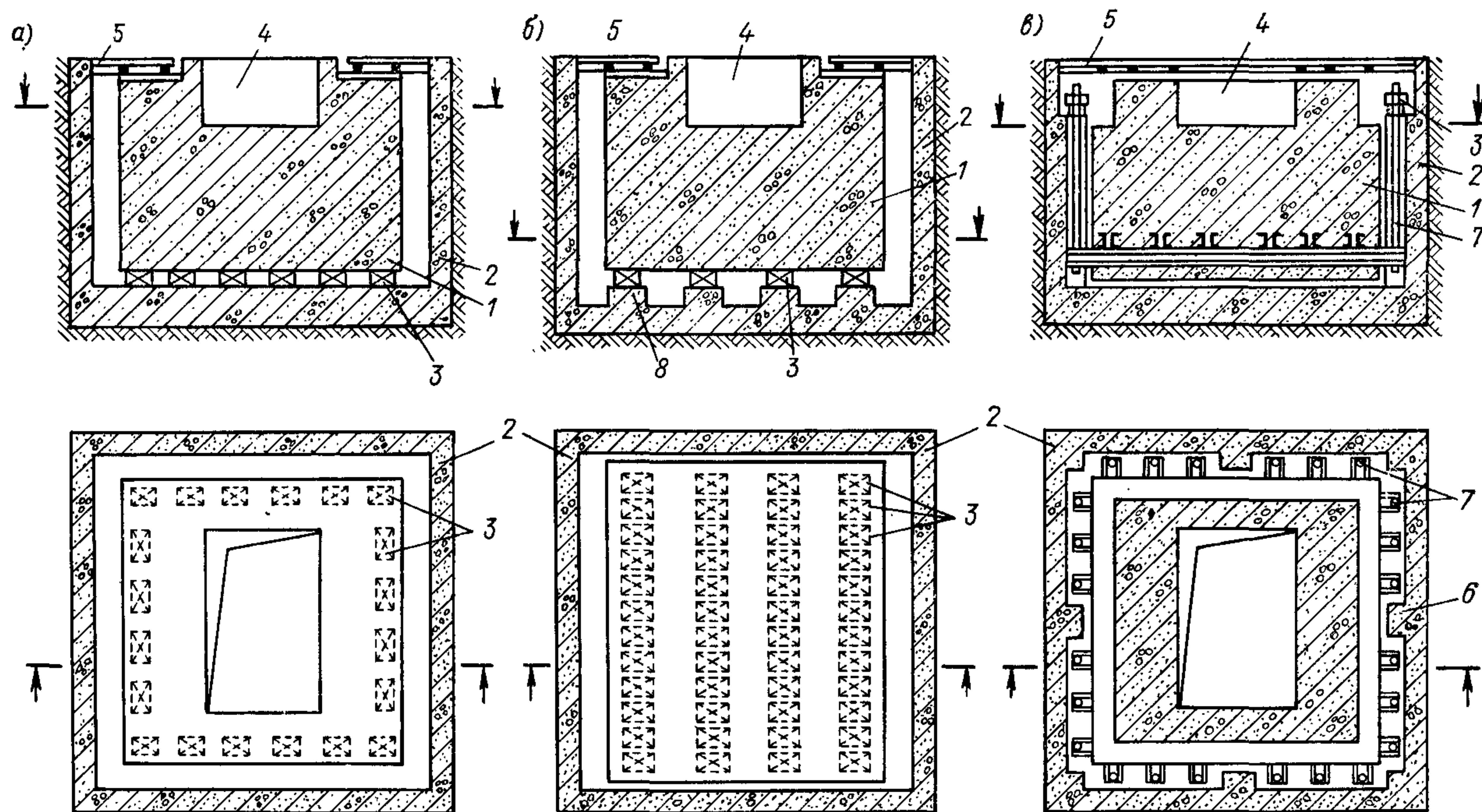
Рис. 3.1. Варианты выполнения виброизоляции под молоты
