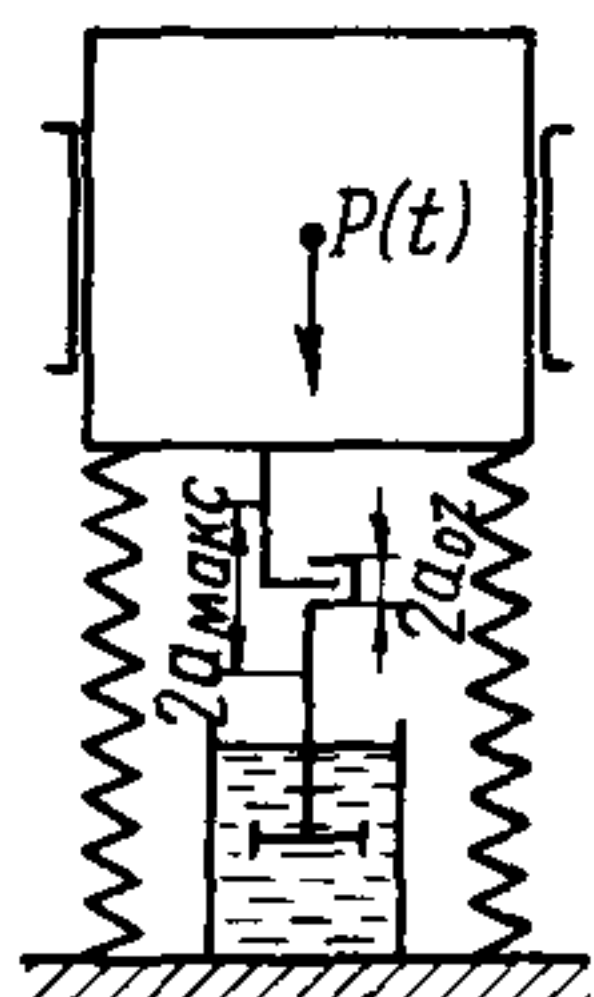
Рис. 6.6. Схема включения демпфера вязкого трения в пуско-остановочных режимах
