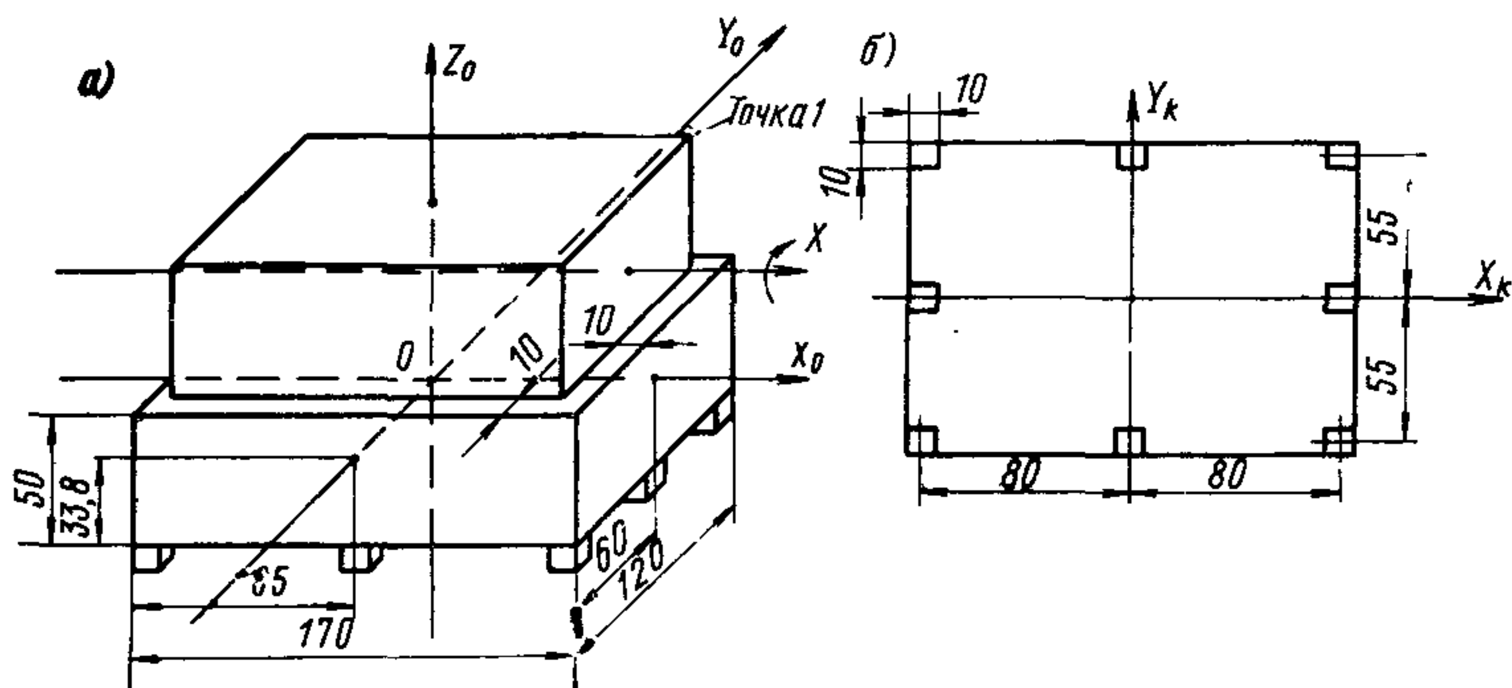
Рис. 10. К примеру расчета пассивной виброизоляции
