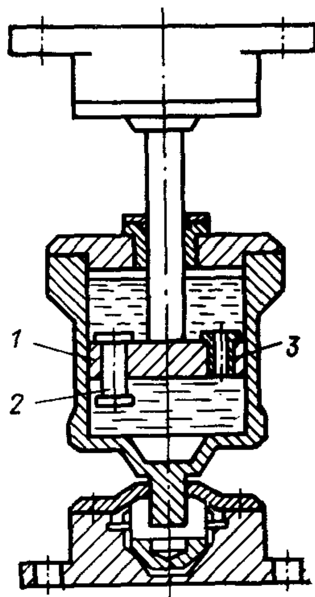
Рис. 6.8. Демпфер вязкого трения со свободным ходом
