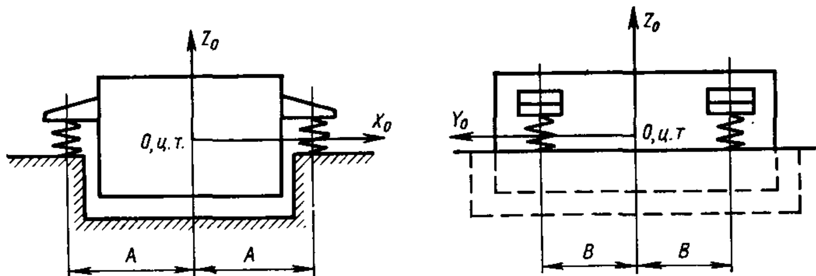
Рис. 1. Схема виброизоляции с симметричным расположением упругих элементов относительно плоскостей X_0Z_0 , X_0Y_0 , Y_0Z_0
