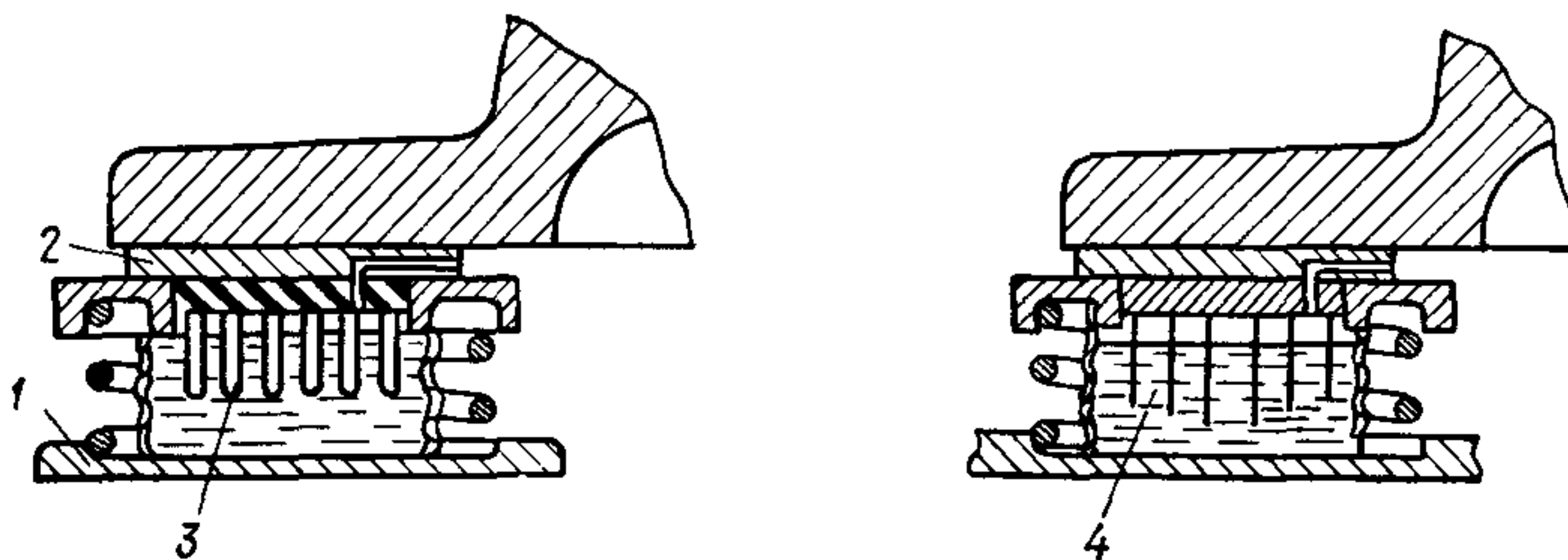
Рис. 6.2. Схемы различных конструктивных решений элементов трения
