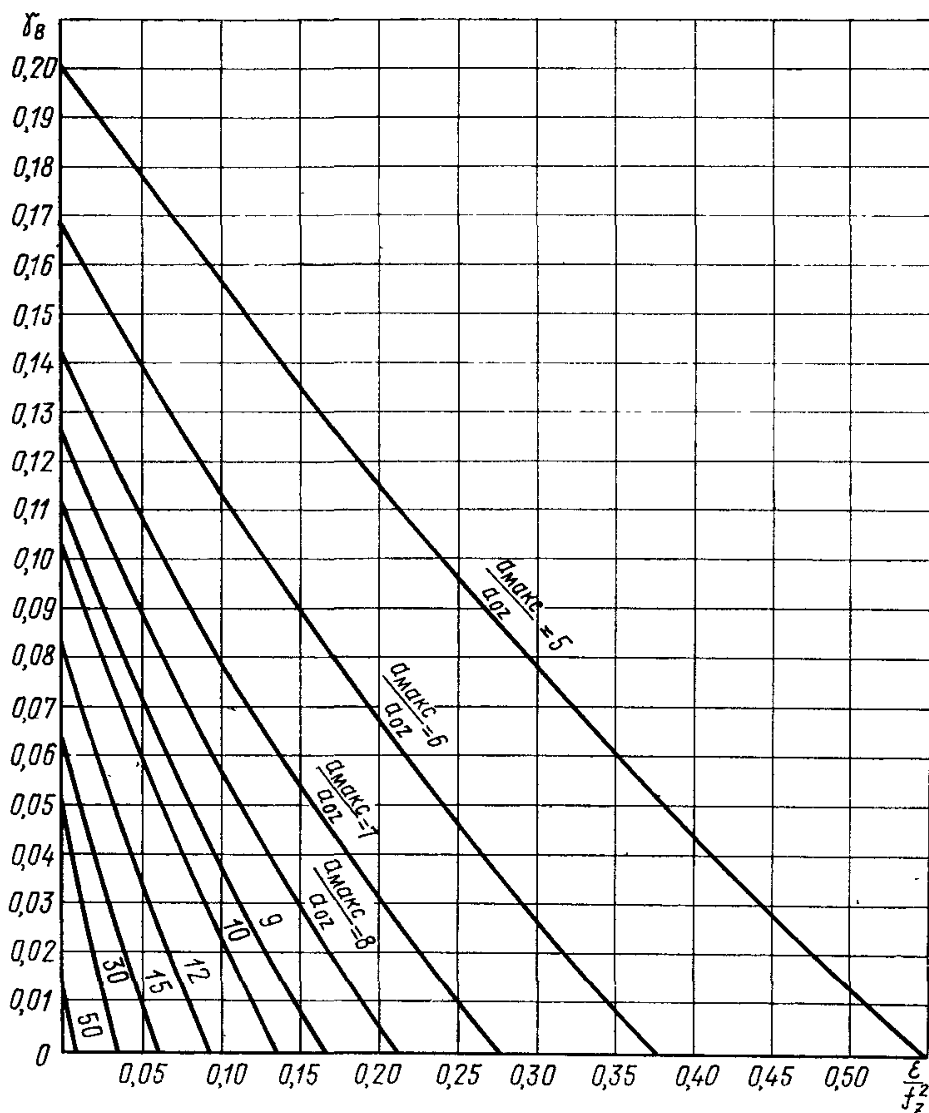
Рис. 2.4. График для определения требуемой величины коэффициента неупругого сопротивления \gamma_v , характеризующего затухание виброизоляции
