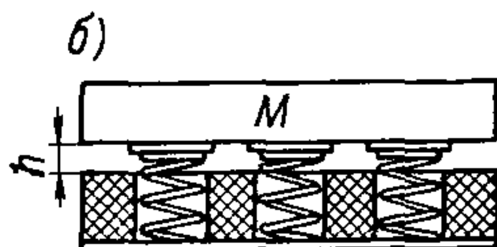
Рис. 5.8. Схемы комбинированных пружинно-пластмассовых виброизоляторов
