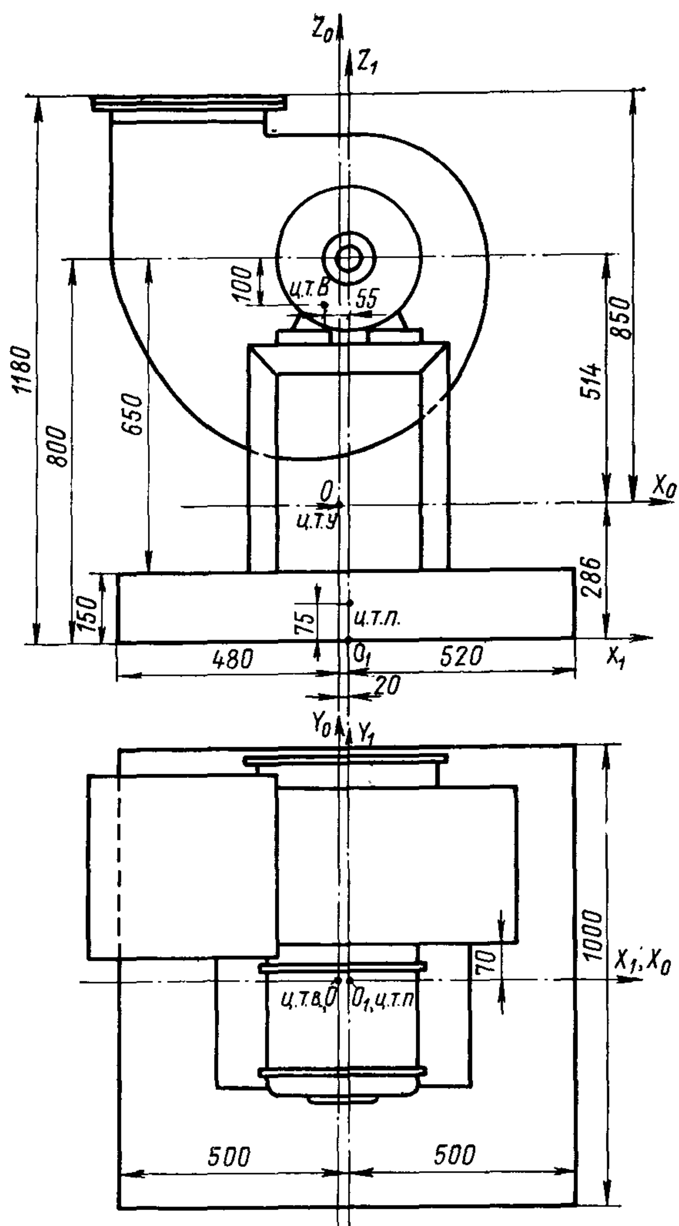
Рис. 5. Эскиз вентилятора, установленного на железобетонную плиту
