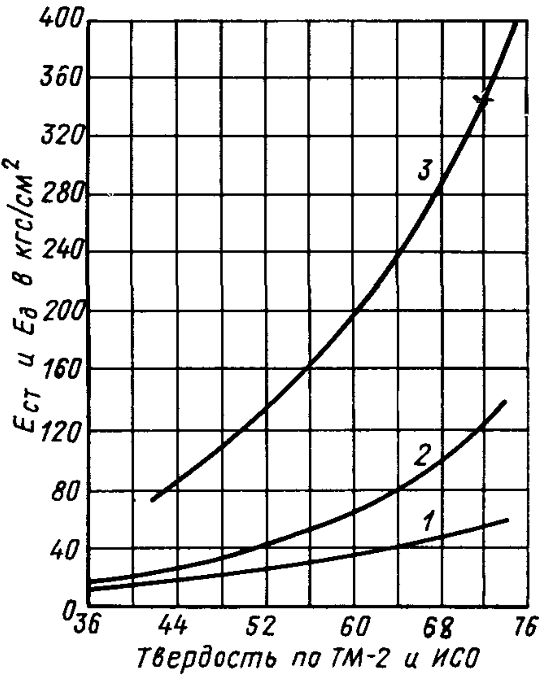
Рис. 5.4. Статические (1) и динамические (2) модули упругости резины на натуральном каучуке и E_d резины на синтетических каучуках (3)
