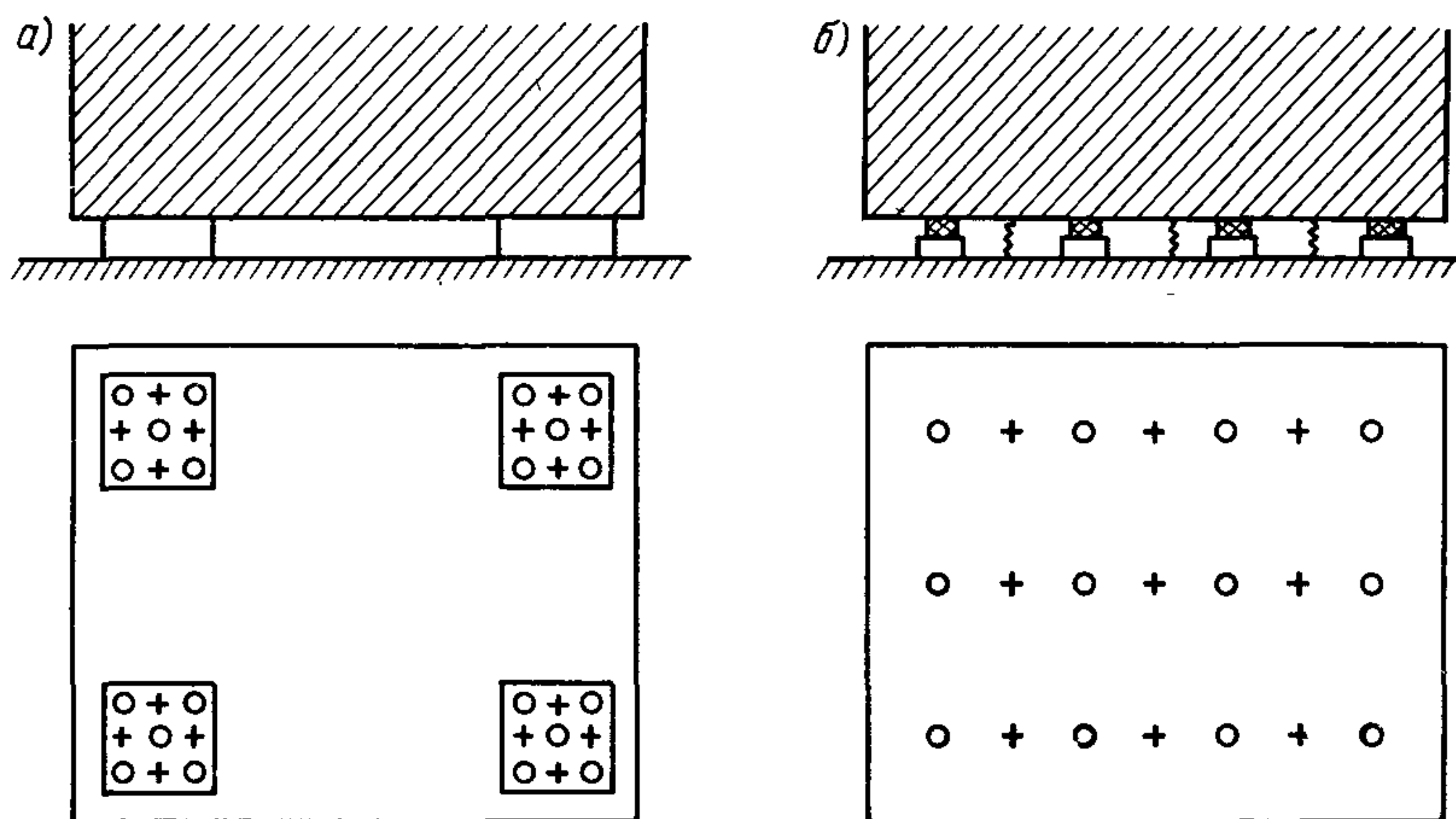
Рис. 5.5. Схемы комбинированных виброизоляторов из пружин и резиновых элементов
