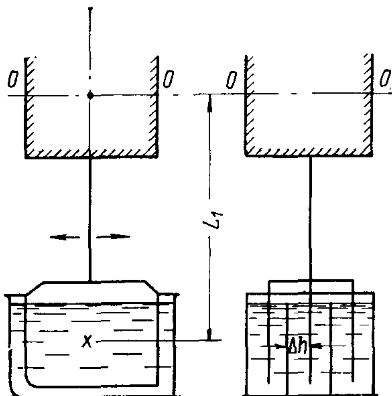
Рис. 6.3. Демпфер вязкого трения
