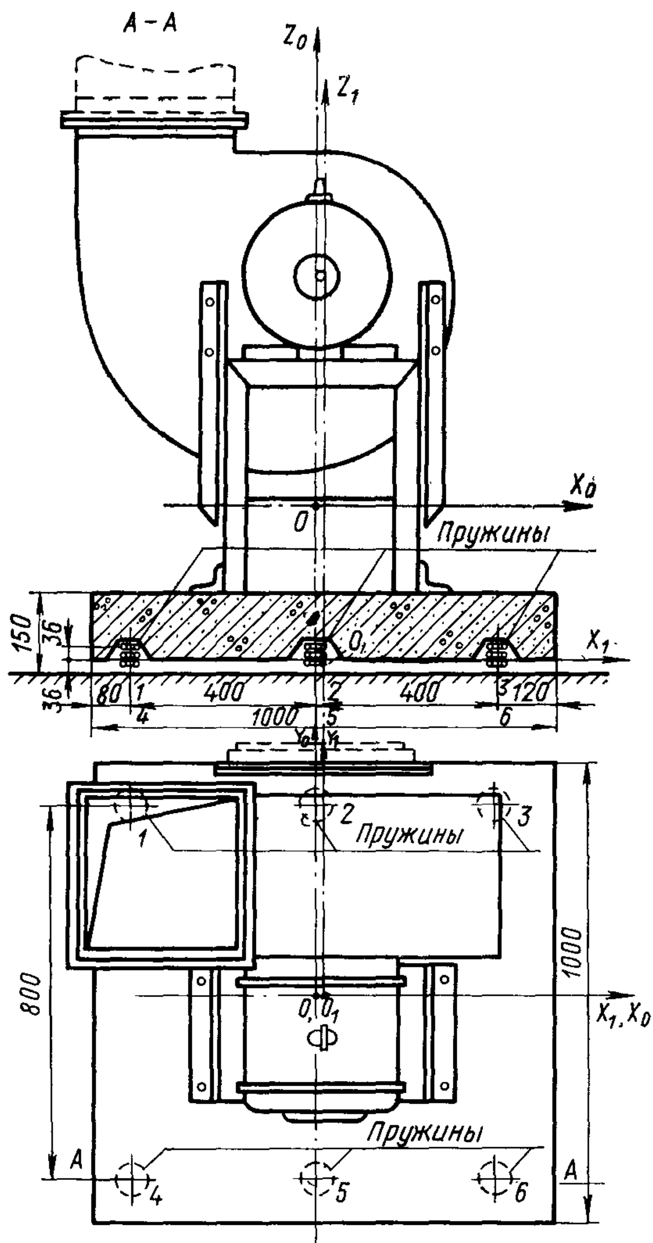
Рис. 6. Схема расположения пружинных вибро- изоляторов
