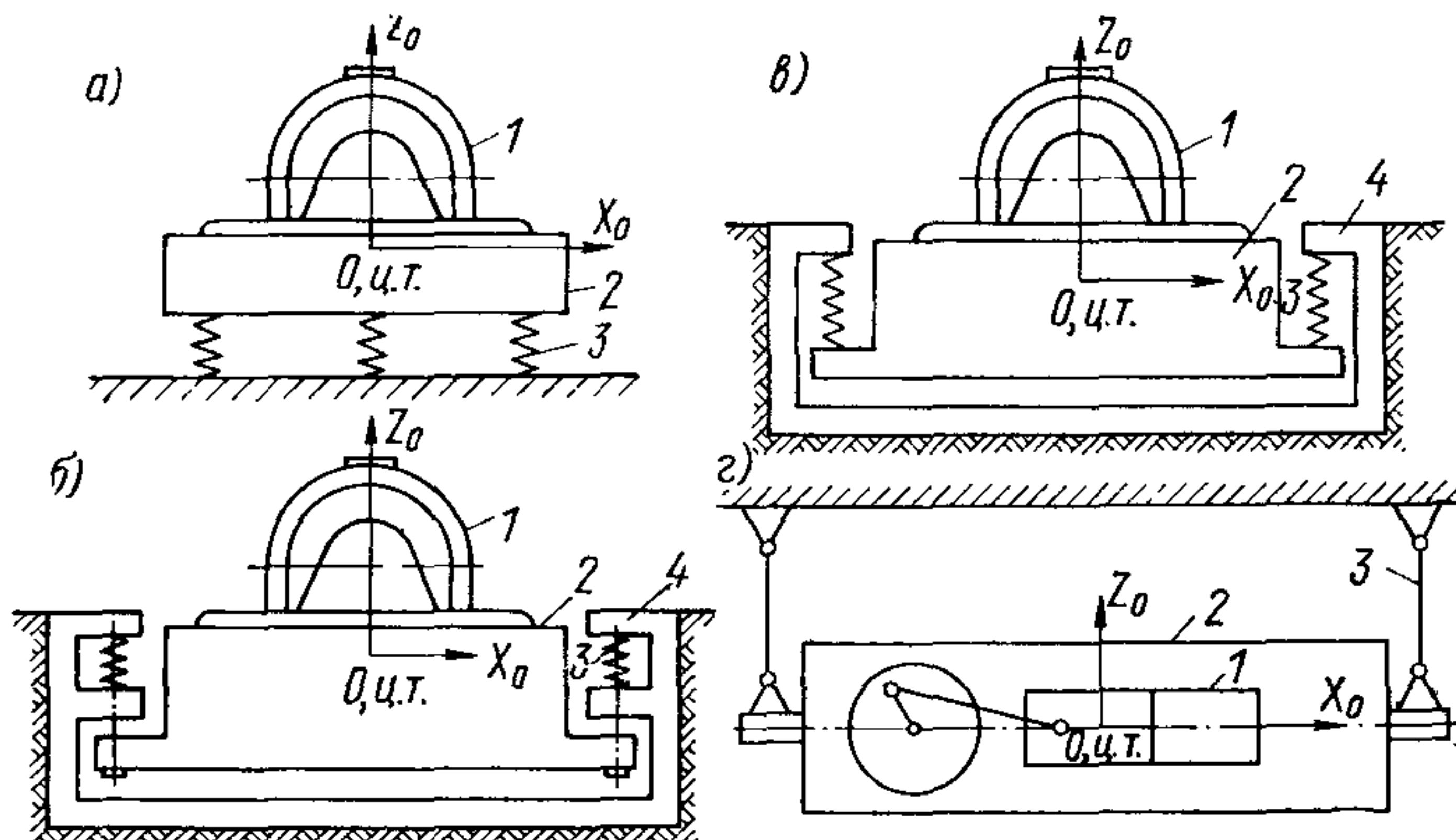
Рис. 2.1. Схемы виброизоляции машин
