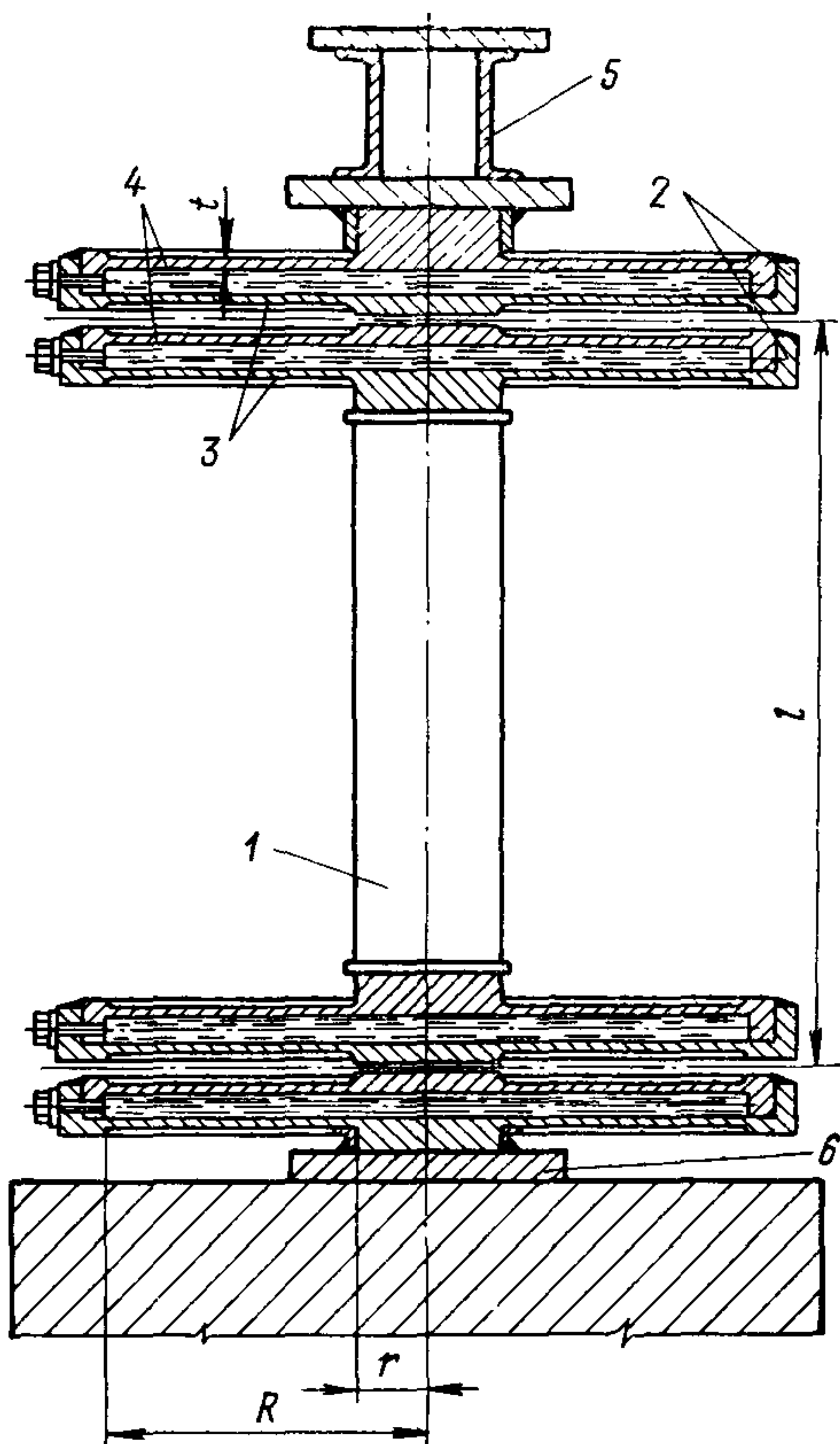
Рис. 5.9. Схема опорного виброизолятора с гидрошарнирами:
