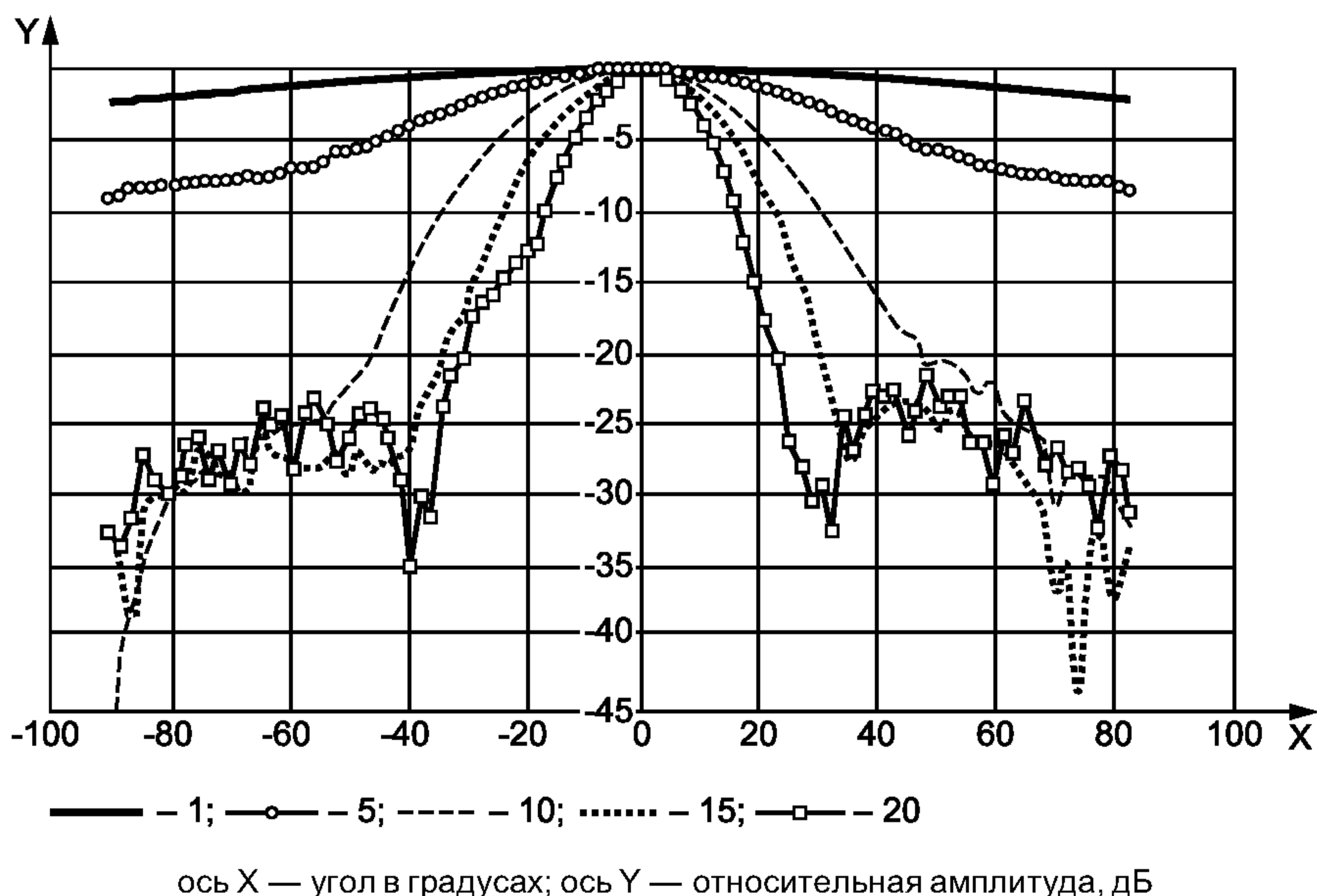
Рисунок А.2 — Характеристики направленности 0,2 мм — зондового гидрофона
