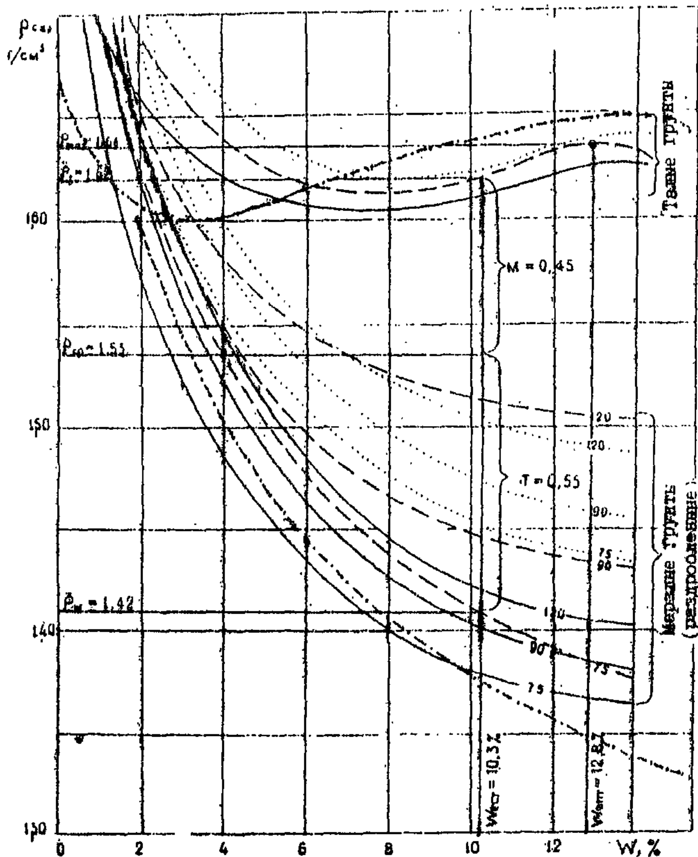
Рис. 1. Зависимость уплотняемости песчаных грунтов в талом и мерзлом состояниях \rho_{сж} от влажности W при различной энергии уплотнения:
