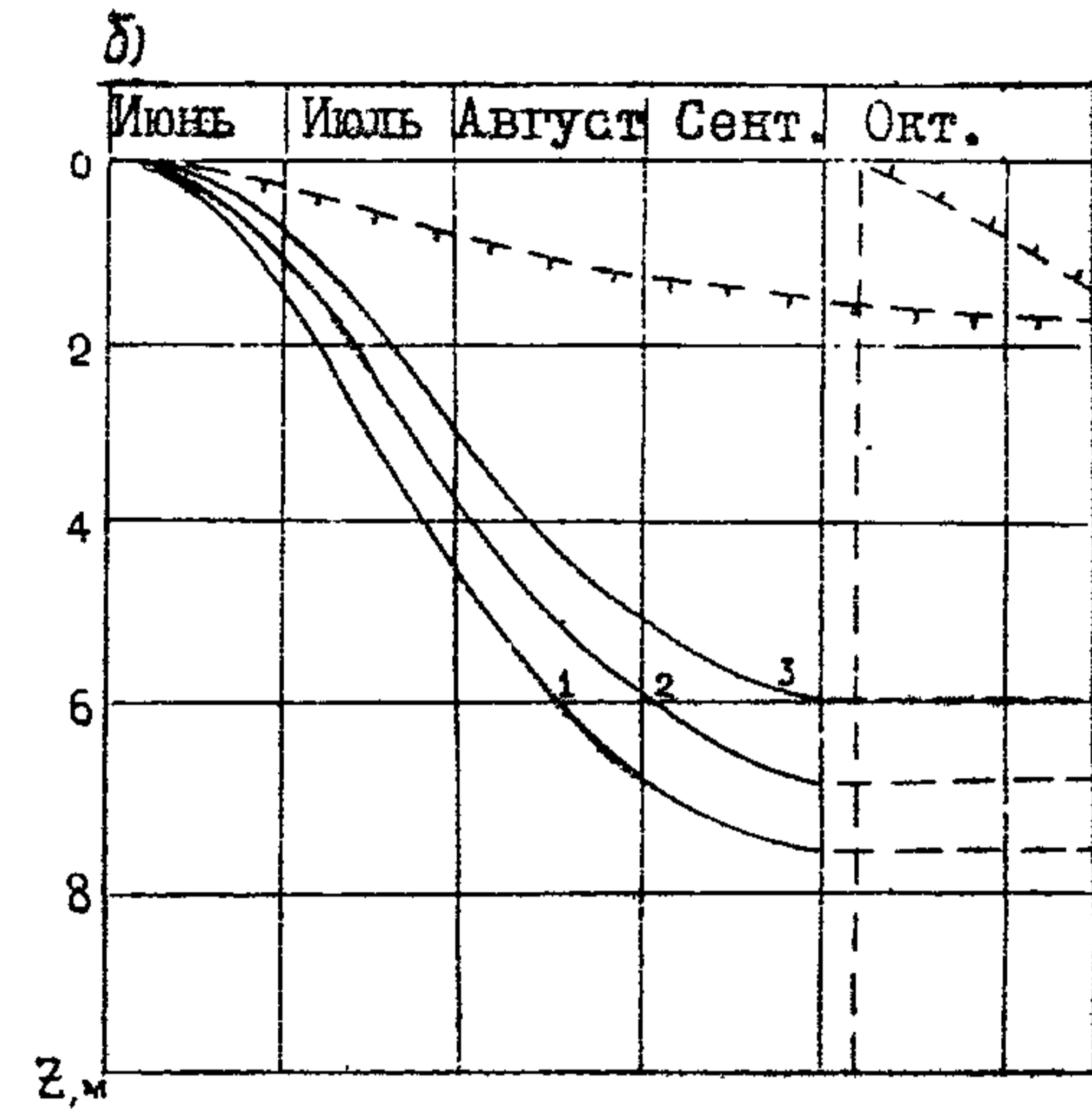
Рис. 3. Графики протаивания песчаного твердомерзлого грунта при радиационно-послойной разработке в районе Ямбурга: а, б - мерзлый песчаный грунт с суммарной влажностью соответственно 25 и 30%; 1, 2, 3 - см. на рис. 2
