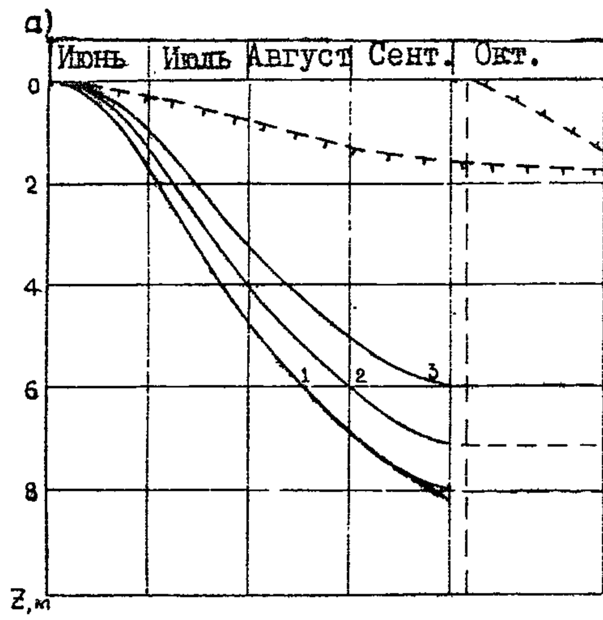
Рис. 3. Графики протаивания песчаного твердомерзлого грунта при радиационно-послойной разработке в районе Ямбурга: а, б - мерзлый песчаный грунт с суммарной влажностью соответственно 25 и 30%; 1, 2, 3 - см. на рис. 2
