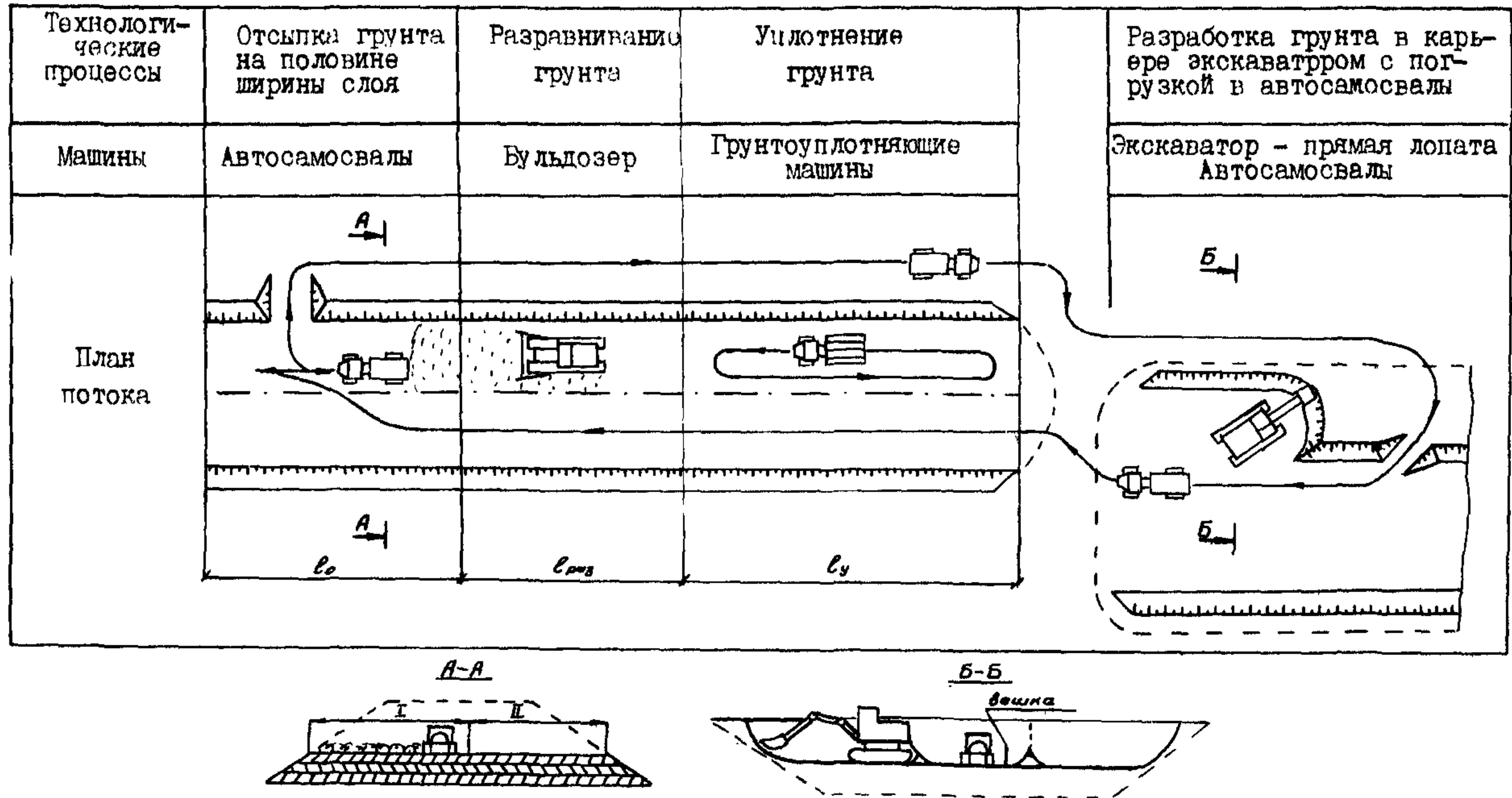
Рис. 3.1. Схема отсыпки насыпи автосамосвалами с разработкой грунта в карьере экскаватором-прямая лопата (с кольцевой ездой автосамосвалами): I—зона отсыпки слоя насыпи; II—зона движения груженых автосамосвалов
