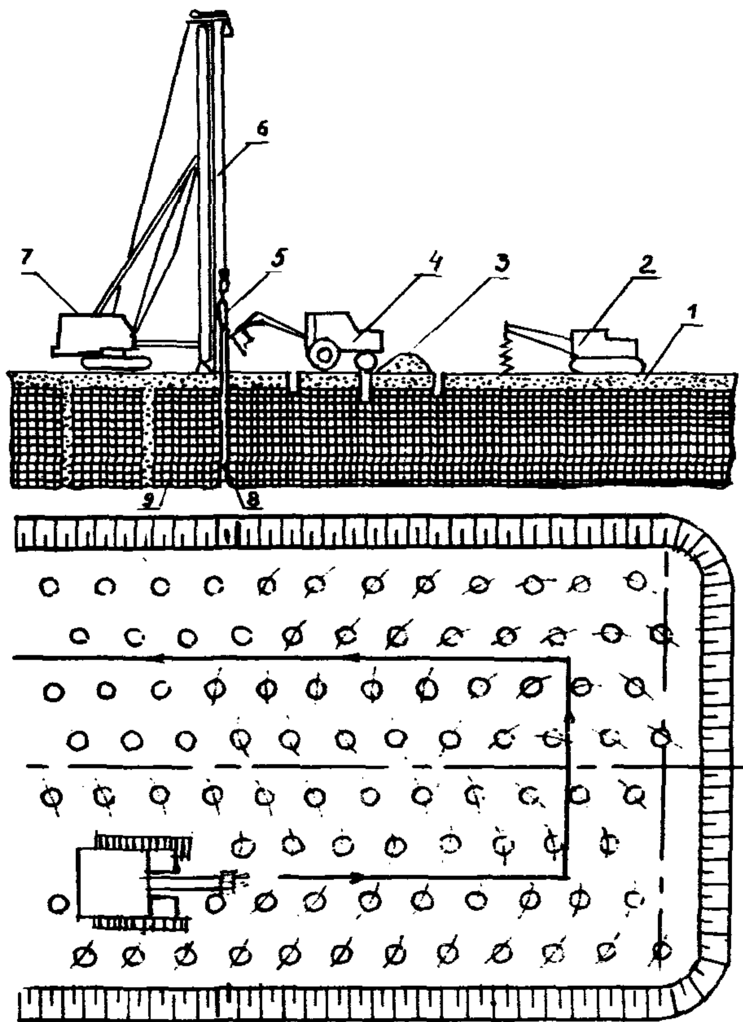
Рис. 6.4. Технологическая схема устройства вертикальных песчаных дрен:
