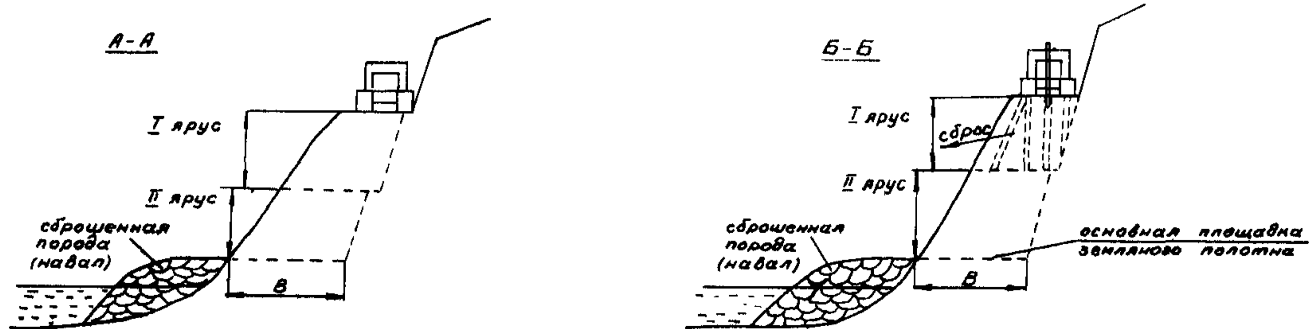
Рис. 3.13. Технологическая схема разработки полувыемок на косогорах при взрывах на сброс
