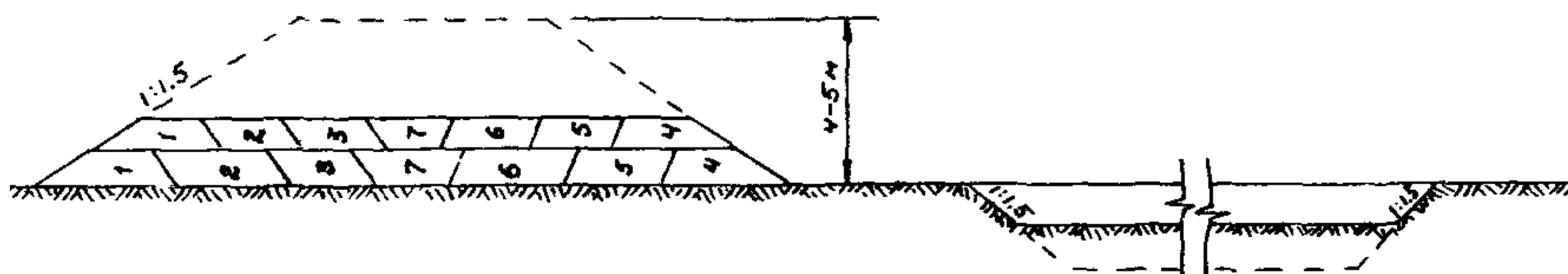
Рис. 3.7. Схема отсыпки насыпей прицепными скреперами из резерва
