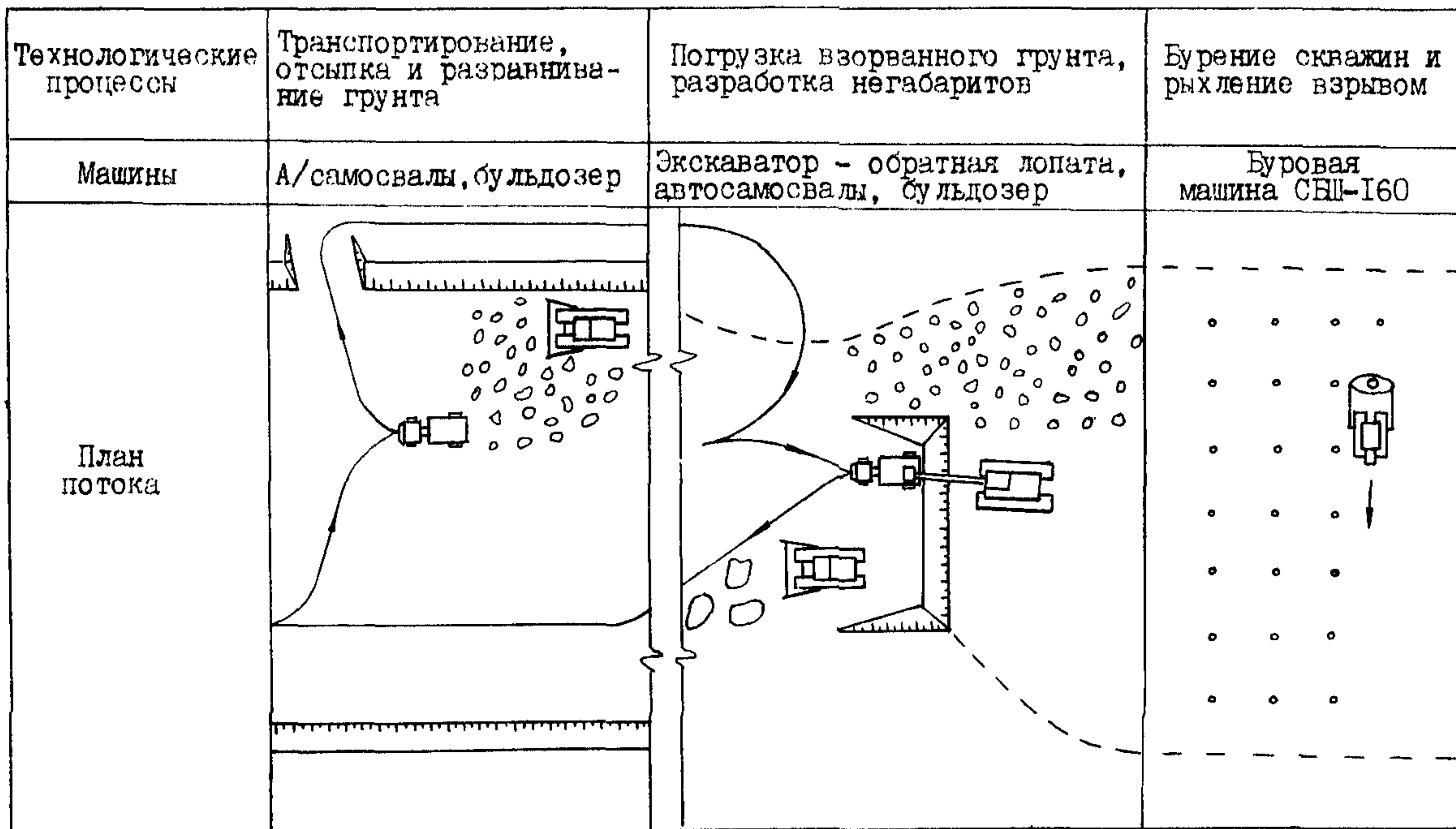
Рис. 3.11. Технологическая схема разработки выемки в скальных грунтах
