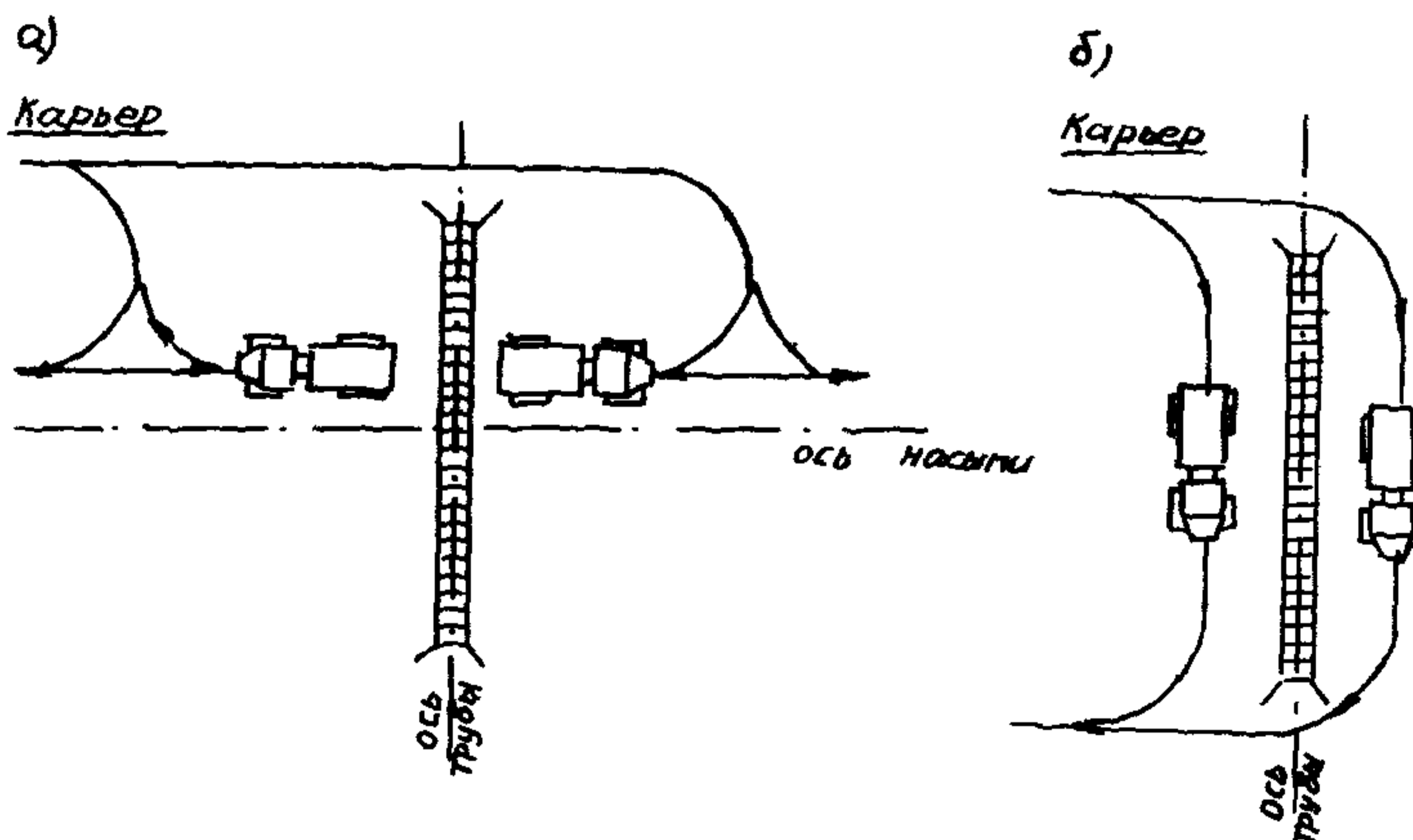
Рис. 9.8. Схемы движения самосвалов при засыпке труб: а—вдоль оси насыпи; б—с кольцевым движением
