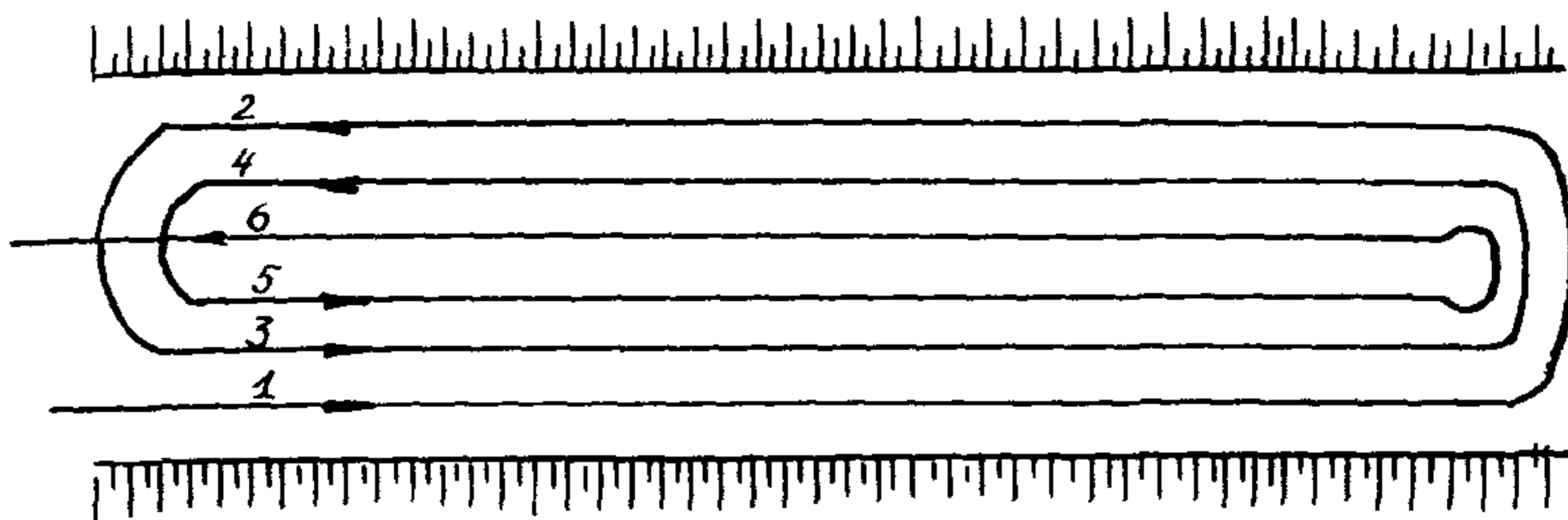
Рис. 9.3. Технологическая схема уплотнения грунта по всей ширине земляного полотна грунтоуплотняющей машиной: 1—6—последовательность проходов
