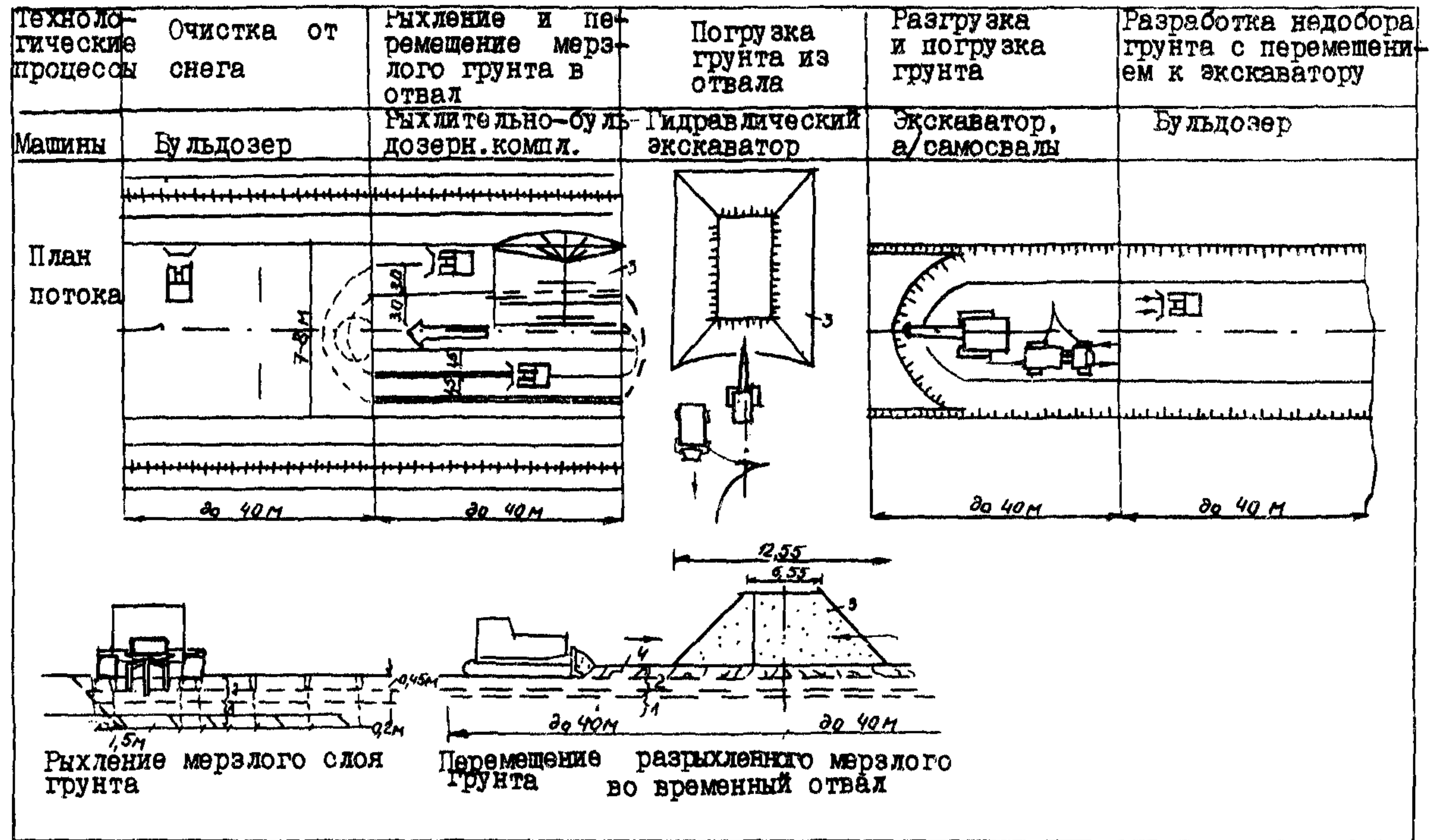
Рис. 5.2. Схема производства работ при разработке грунта в зимних условиях: 1—талый грунт; 2—мерзлый грунт; 3—временный отвал мерзлого грунта; 4—разрыхленный грунт
