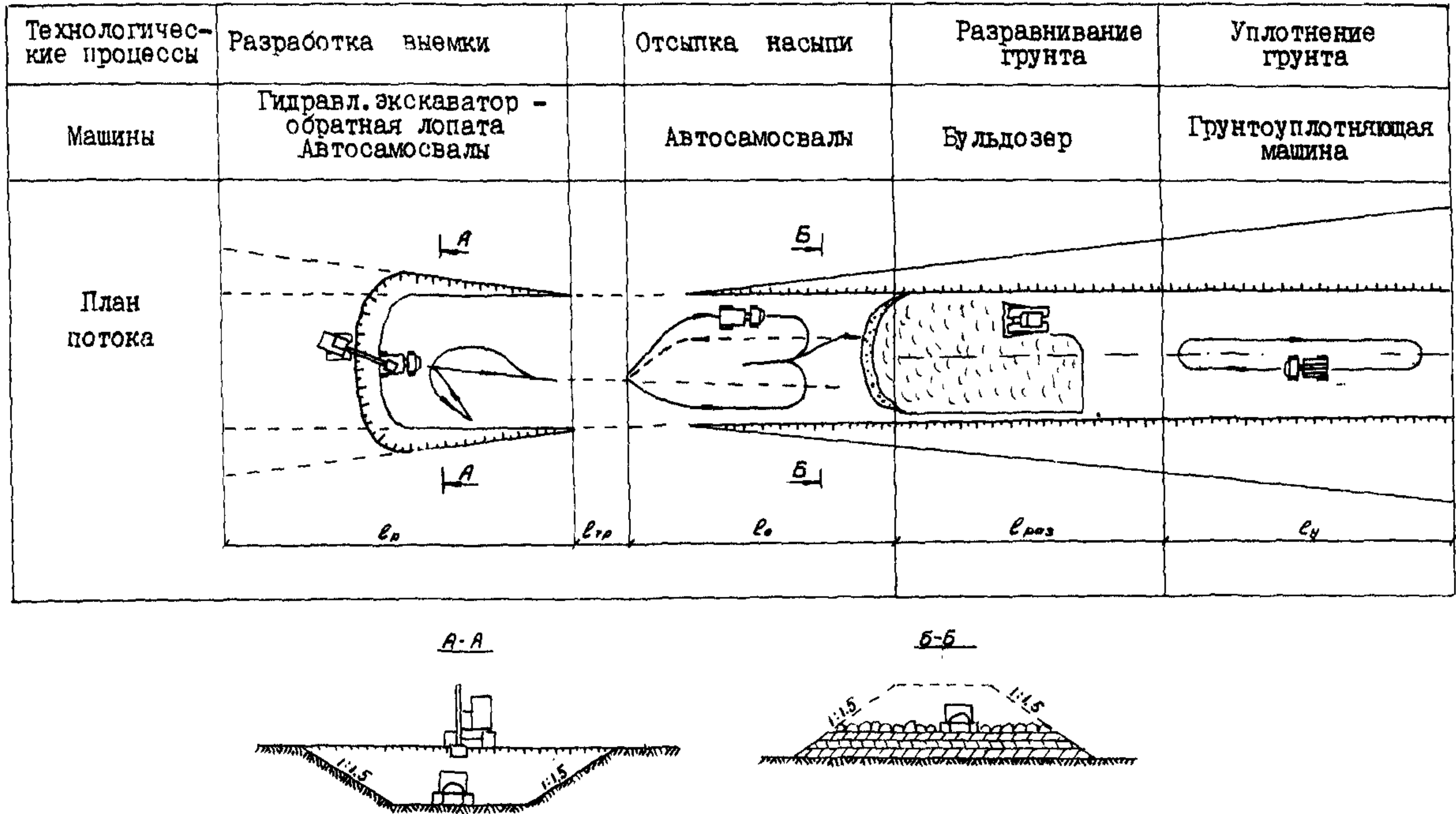
Рис. 3.2. Схема разработки выемки экскаватором-обратная лопата и отсыпки насыпи автосамосвалами (с разворотом автосамосвалов на насыпи)
