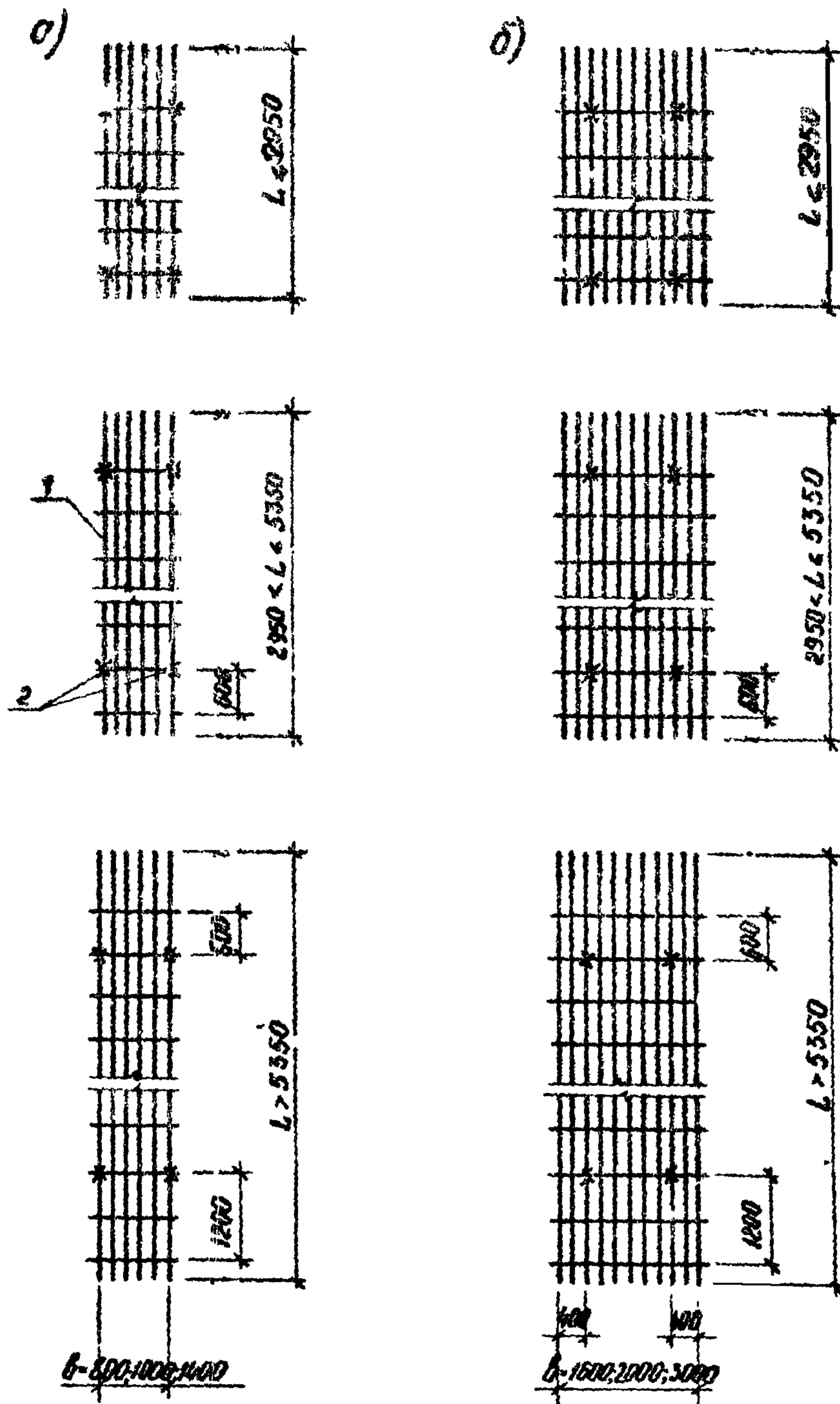
Рис. 1 Схема строповки сеток
