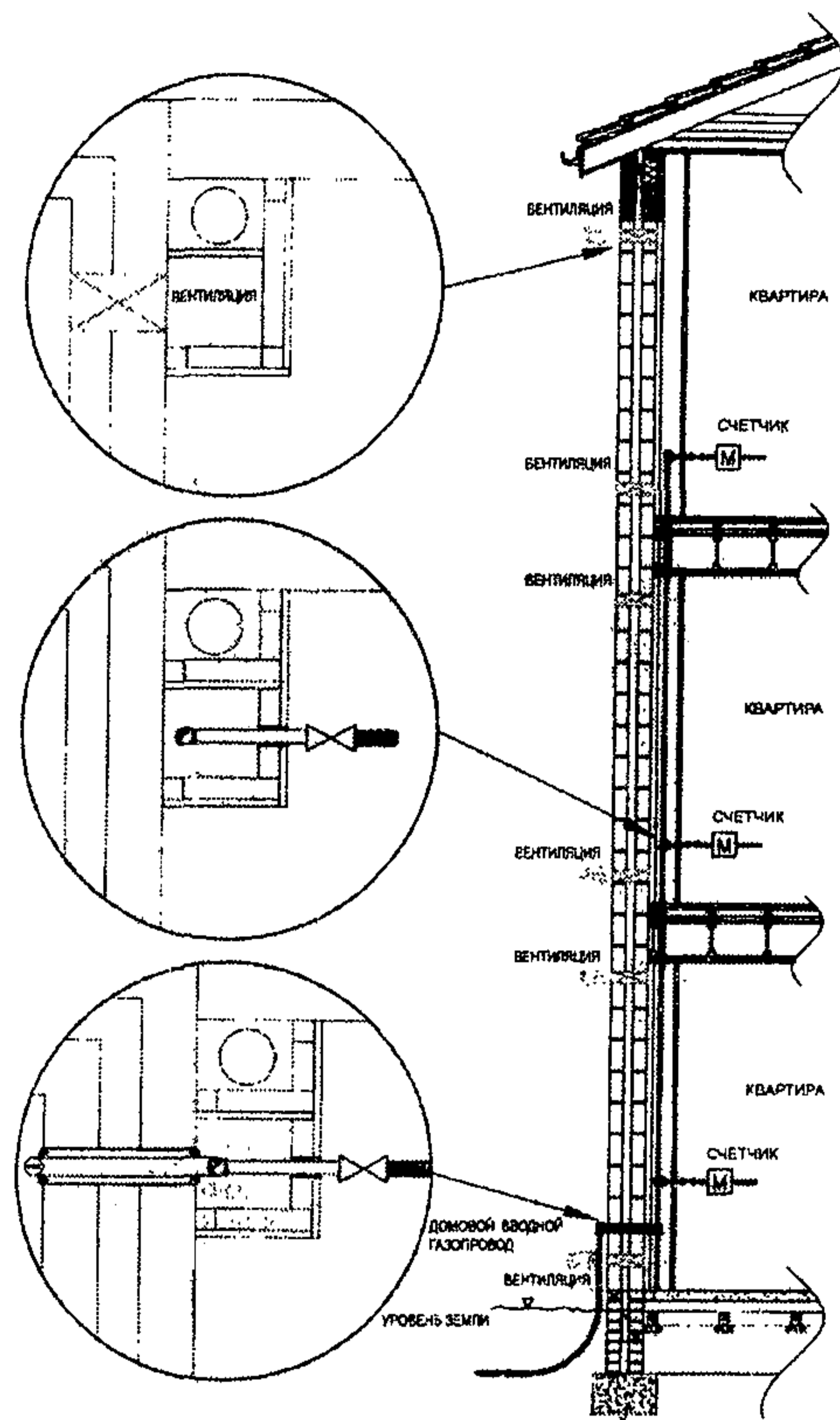
Рисунок Г.1 — Газопровод в вентилируемой штрабе
