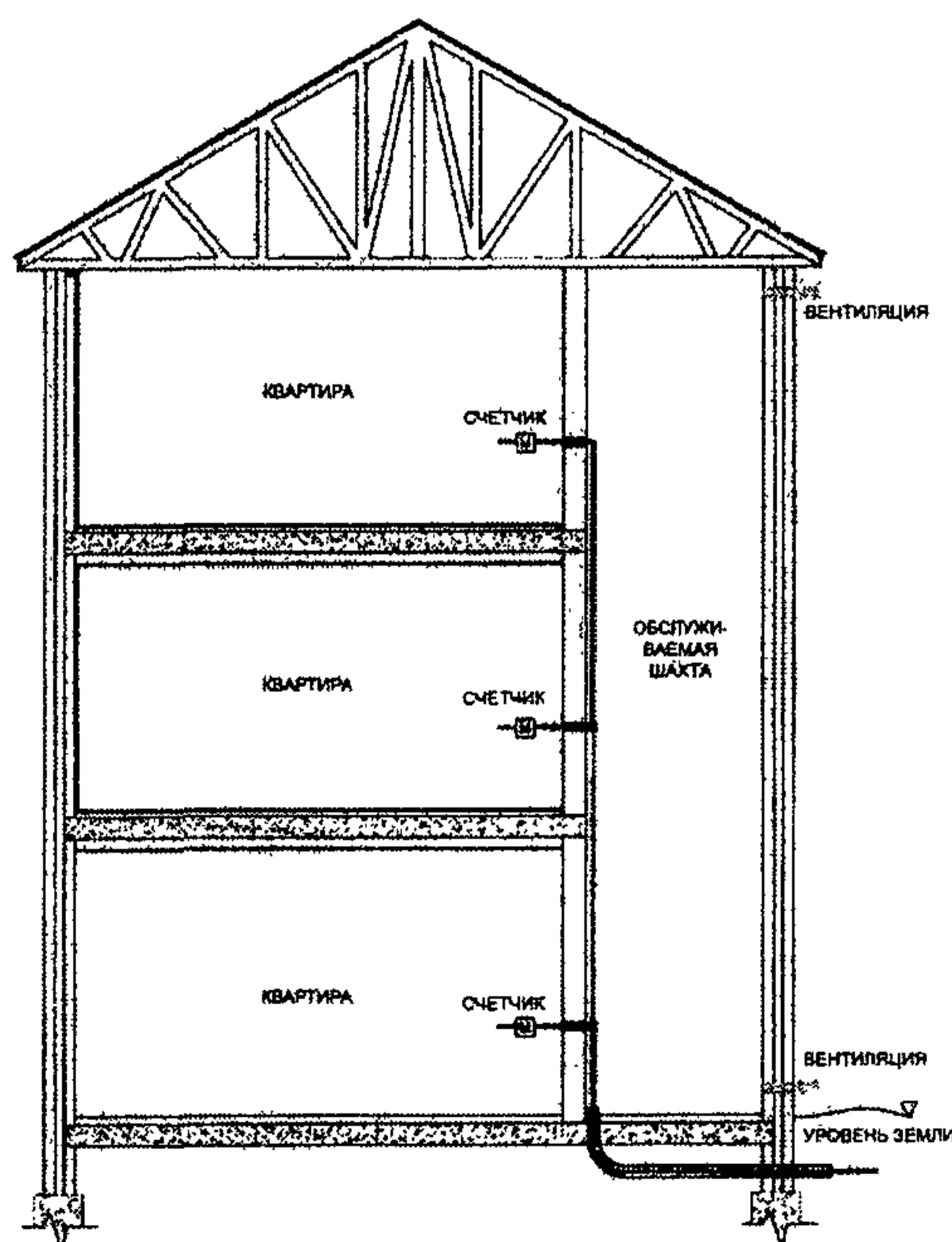
Рисунок Г.2 — Газопровод в вентилируемой шахте
