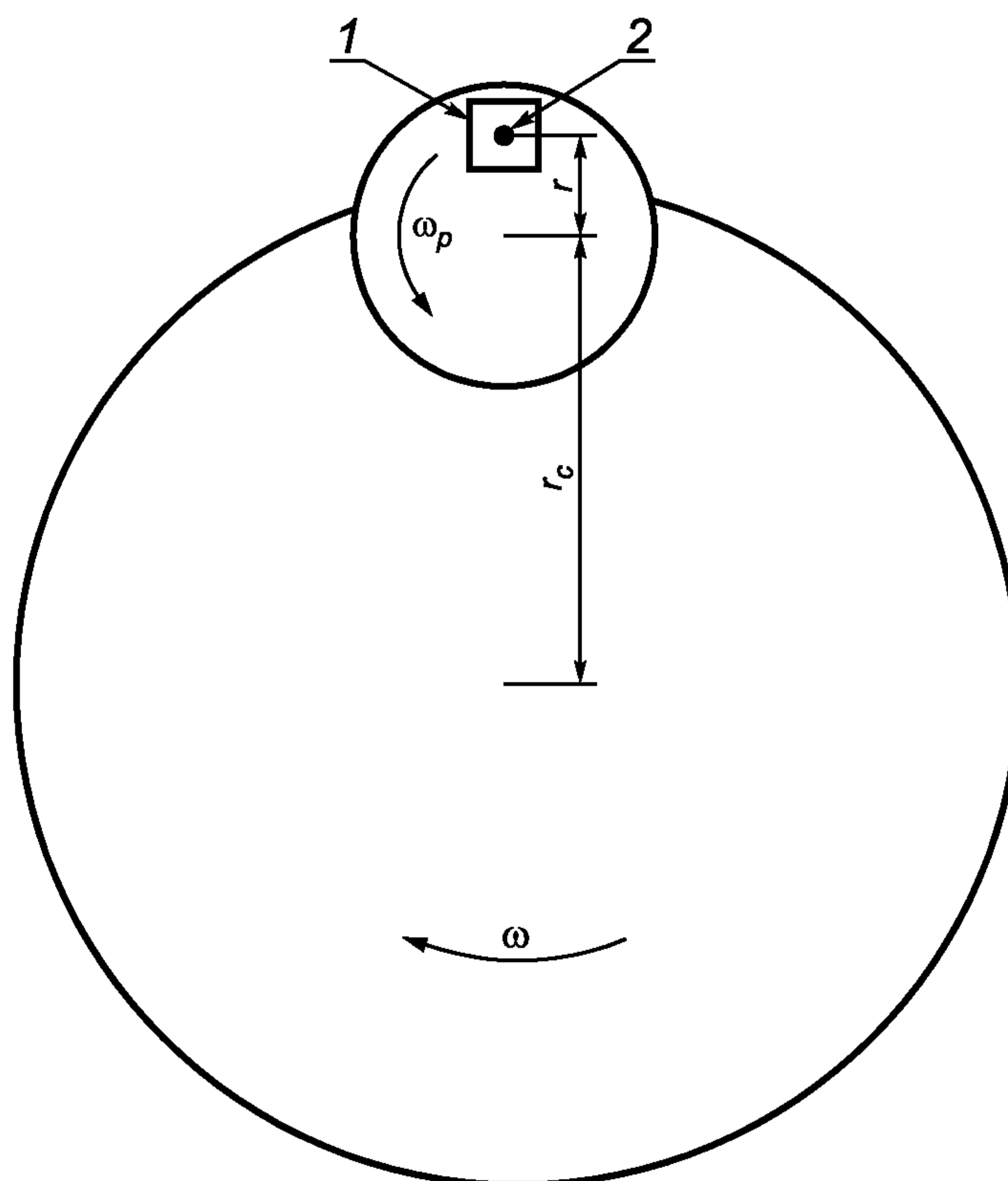
1 — испытуемый преобразователь; 2 — центр тяжести сейсмической массы преобразователя
