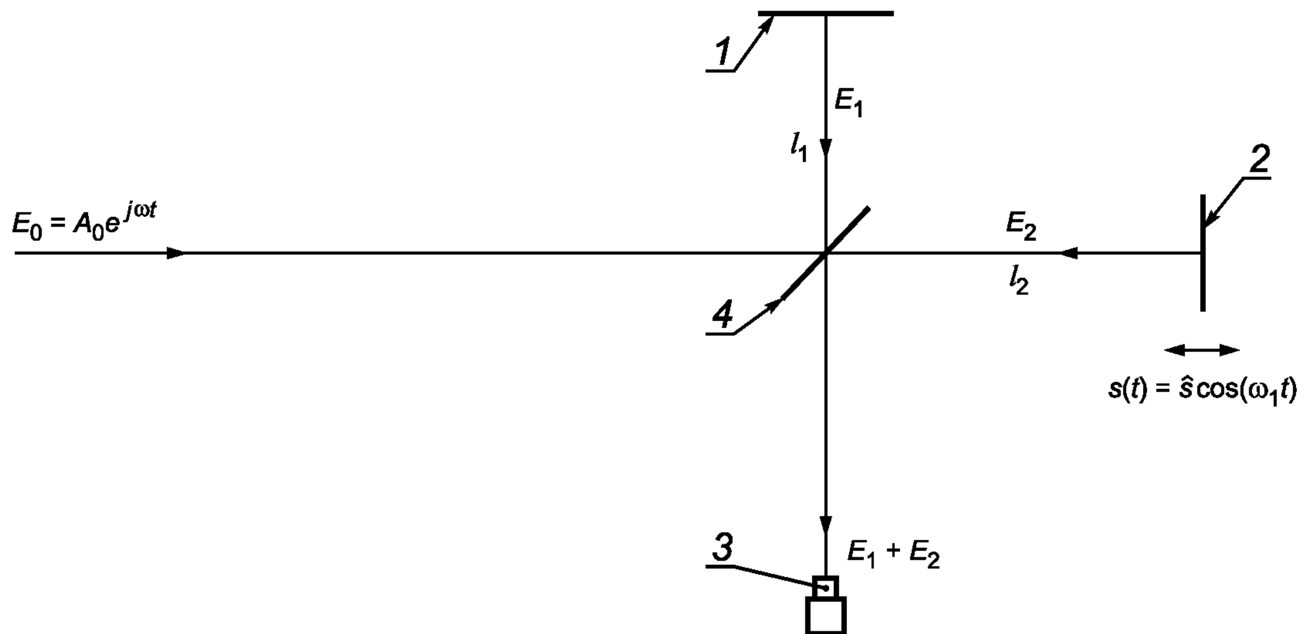
1 — зеркало 1; 2 — зеркало 2; 3 — фотодетектор; 4 — разделитель луча
