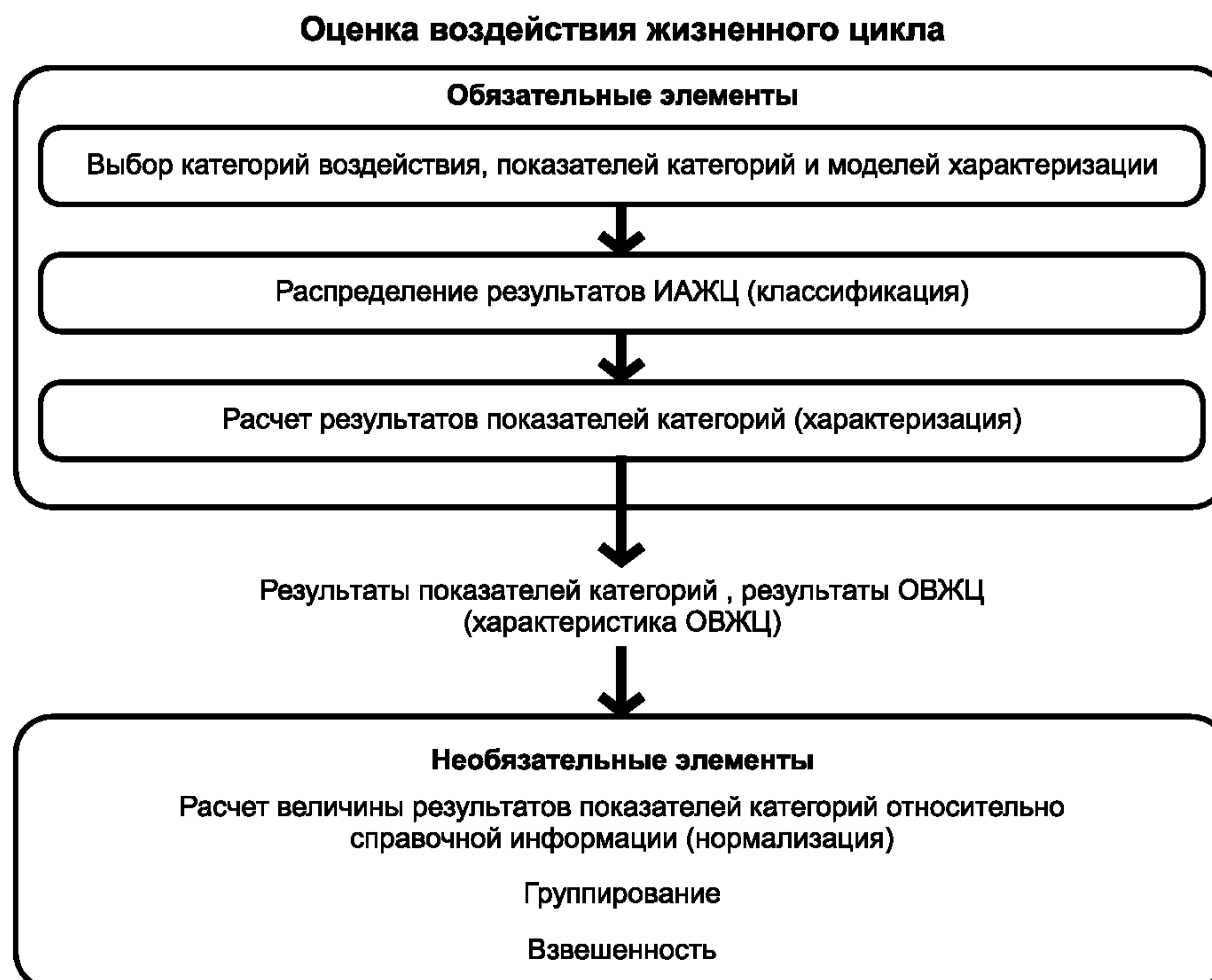
Рисунок 4 — Элементы стадии ОВЖЦ
