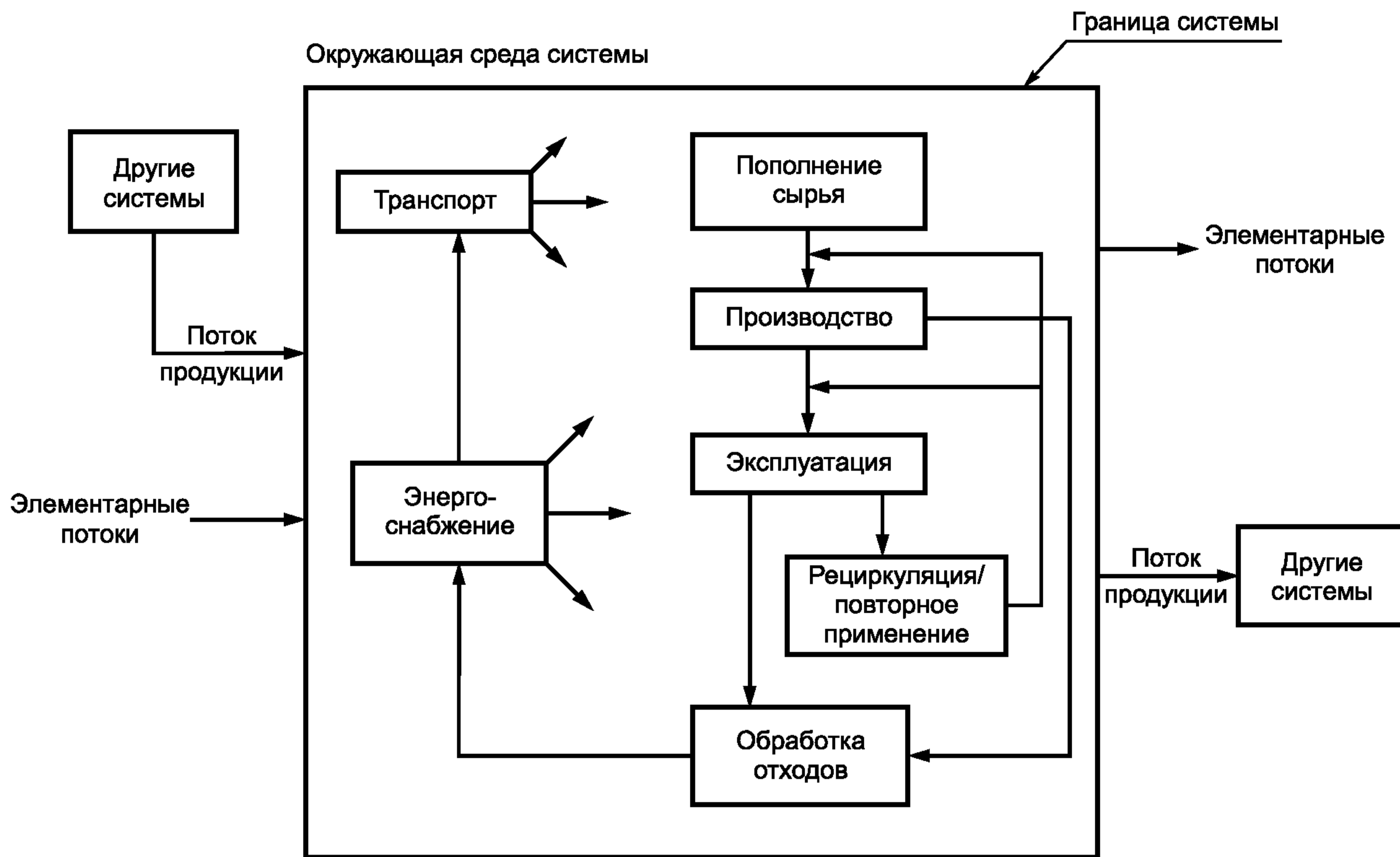
Рисунок 2 — Пример производственной системы для ОЖЦ
