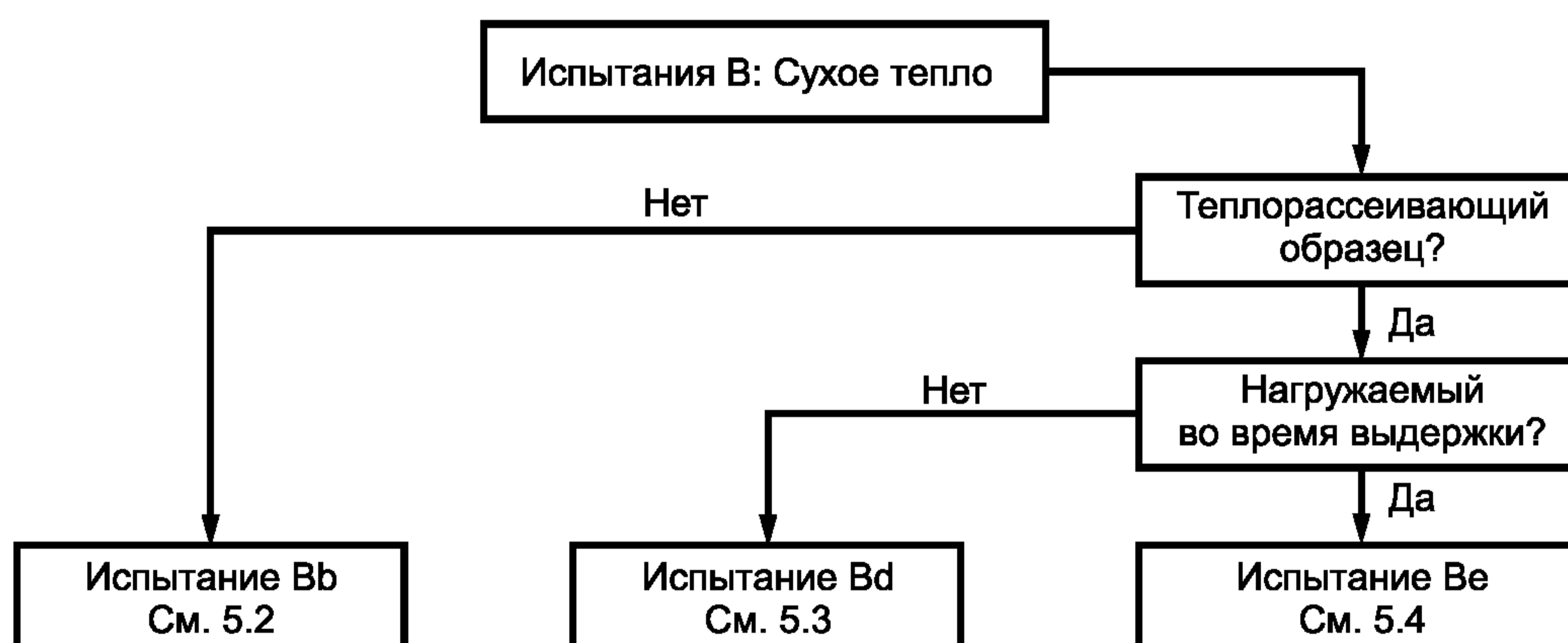
Рисунок 1 — Блок-схема испытаний В: Сухое тепло
