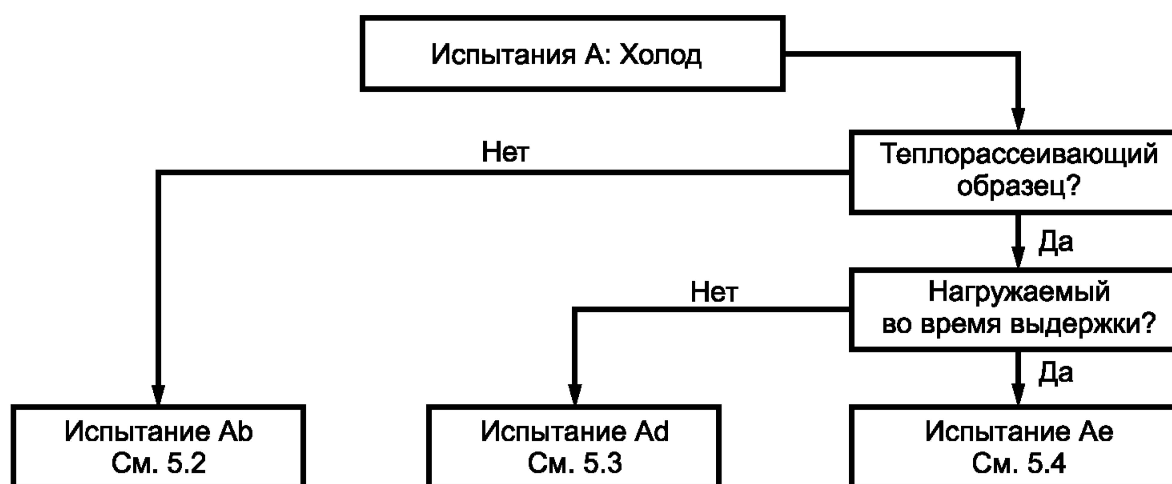
Рисунок 1 — Блок-схема испытаний А: Холод
