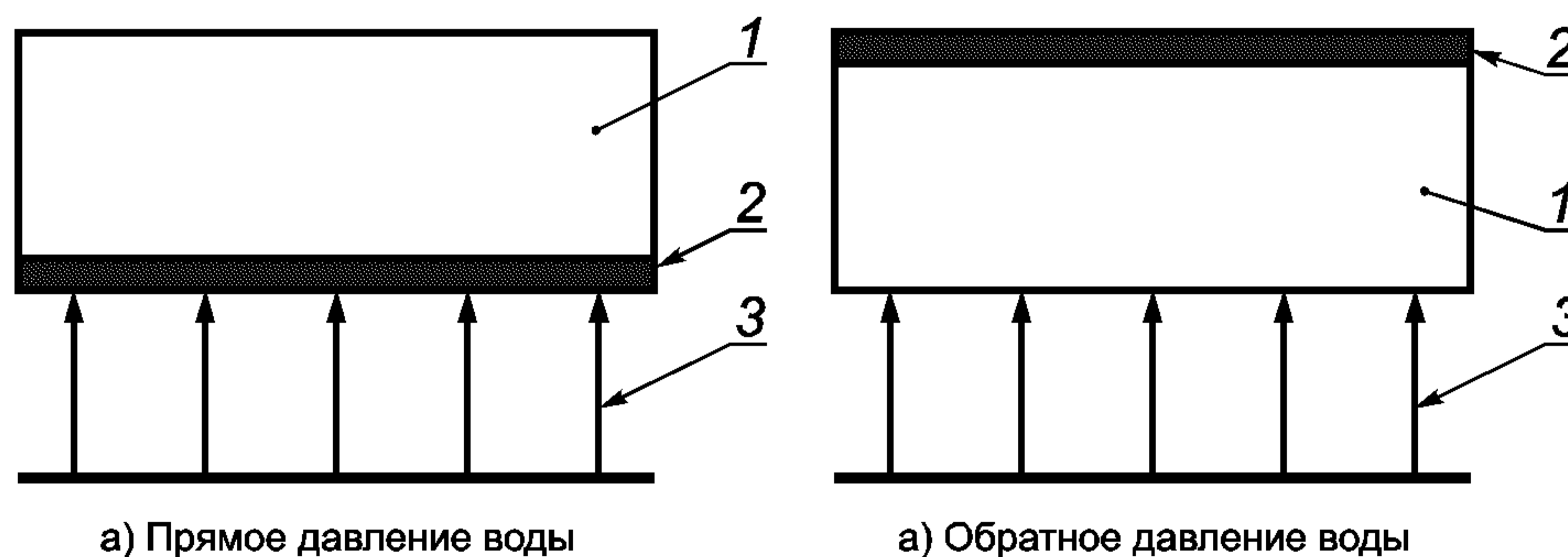
1 — испытуемый образец; 2 — защитное покрытие; 3 — направление подачи воды
