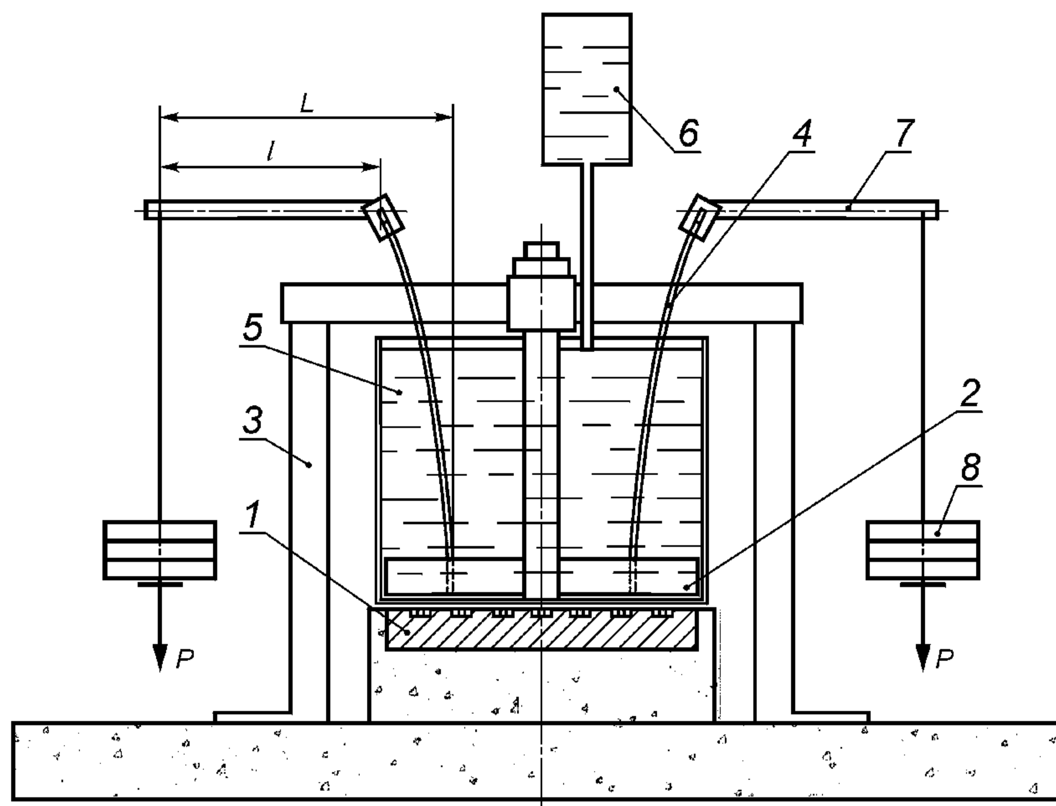
L — горизонтальная проекция плеча действующей силы P ; l — длина рычага; P — сила, действующая на испытуемый образец, подвергая его изгибу; 1 — нагревательный элемент; 2 — плита с отверстиями для крепления испытуемого образца; 3 — рама для жесткой подвески плиты и устойчивости установки; 4 — испытуемый образец; 5 — емкость для коррозионного раствора; 6 — дозатор воды; 7 — рычаг; 8 — груз
