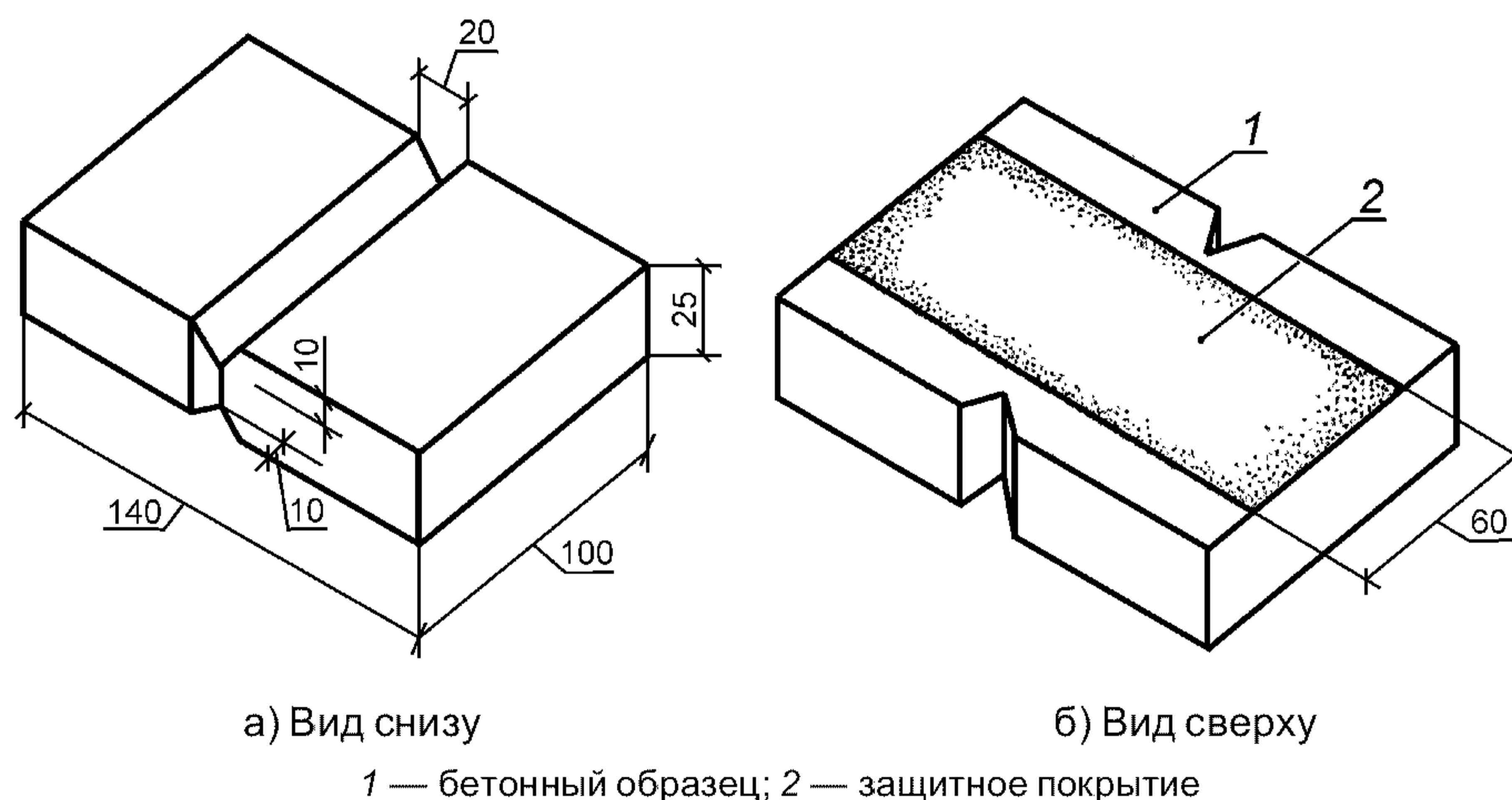
Рисунок 7 — Общий вид образца для определения трещиностойкости
