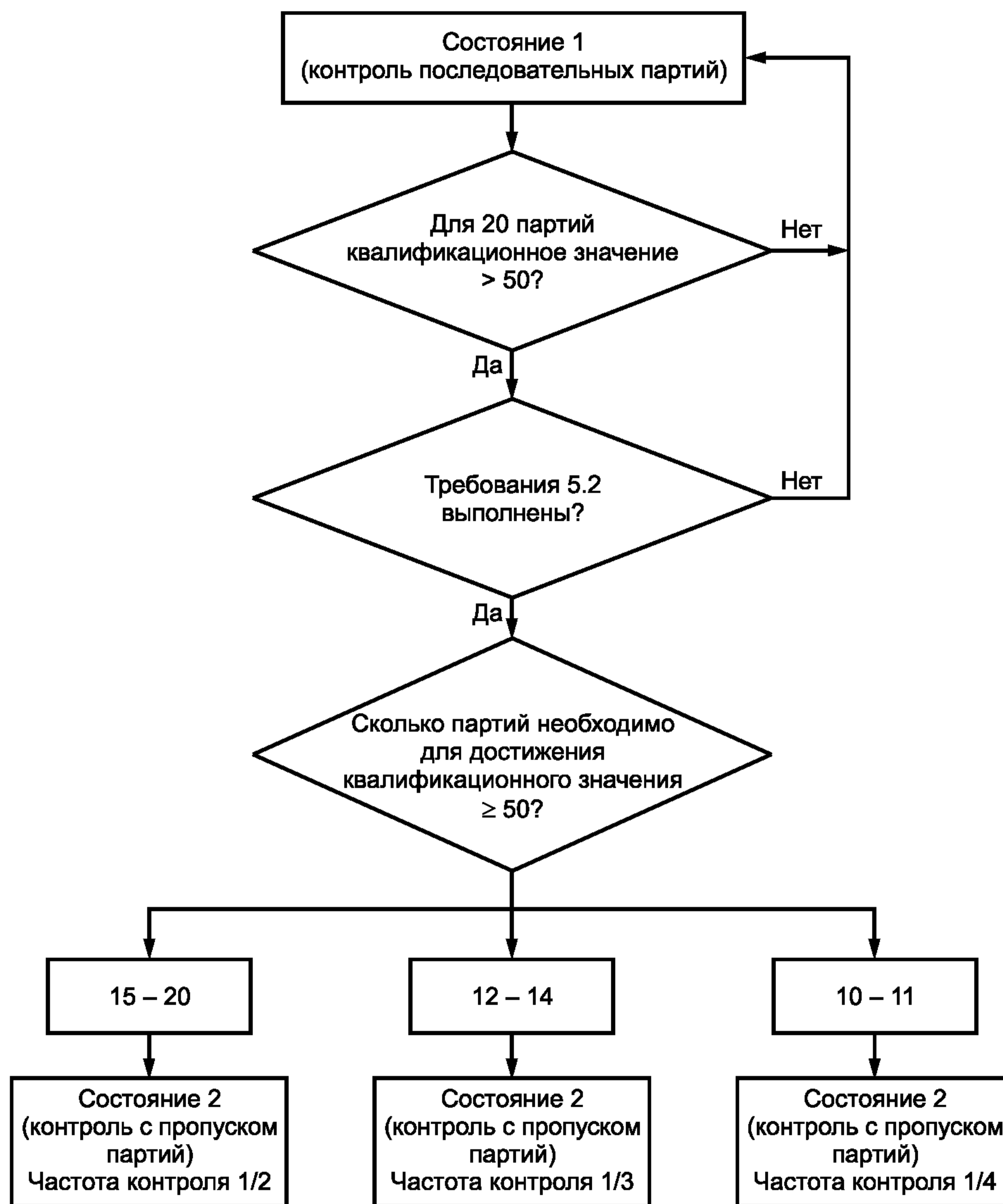
Рисунок 2 — Блок-схема определения начальной частоты контроля
