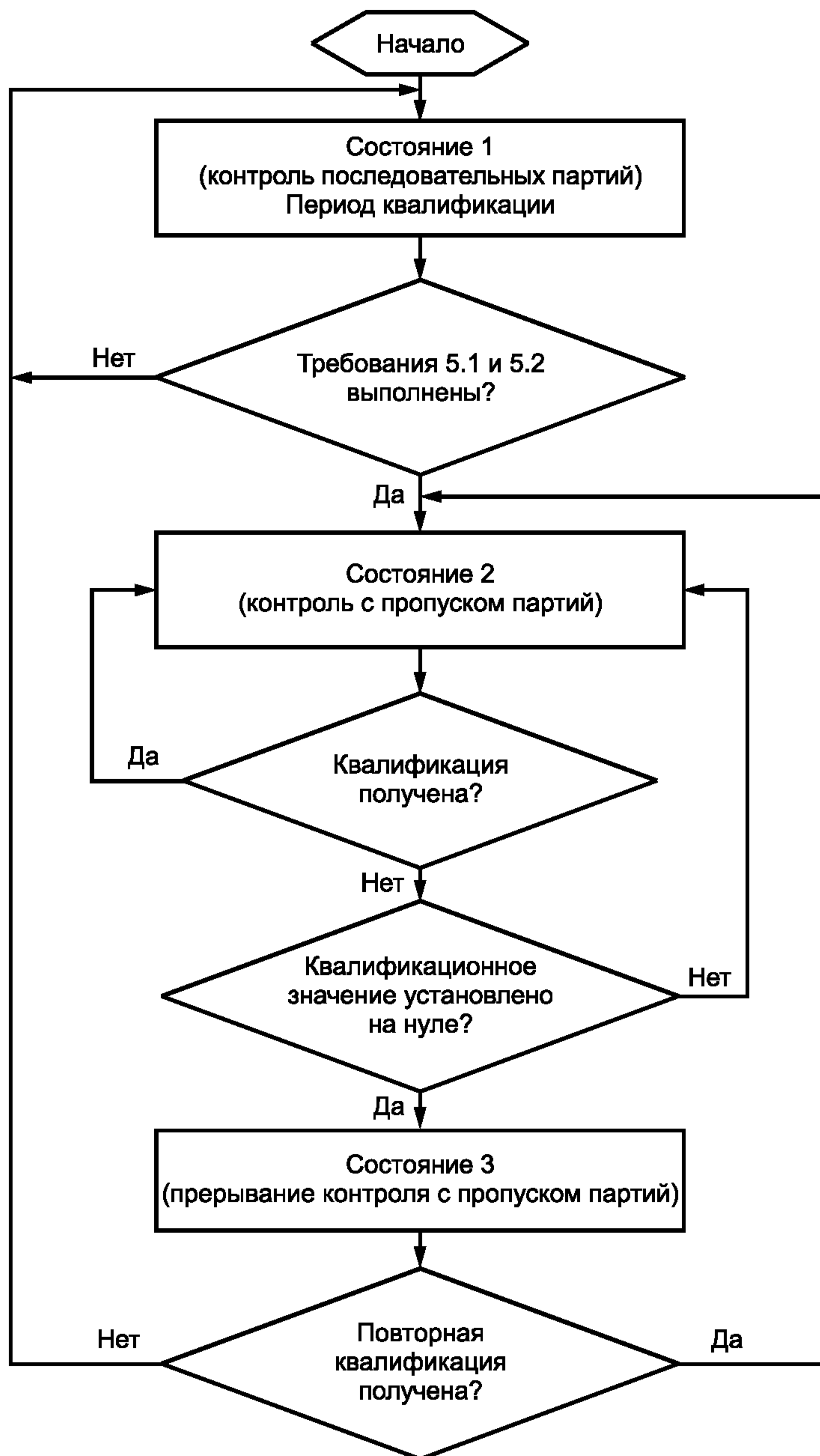
Рисунок 1 — Блок-схема процедуры контроля с пропуском партий
