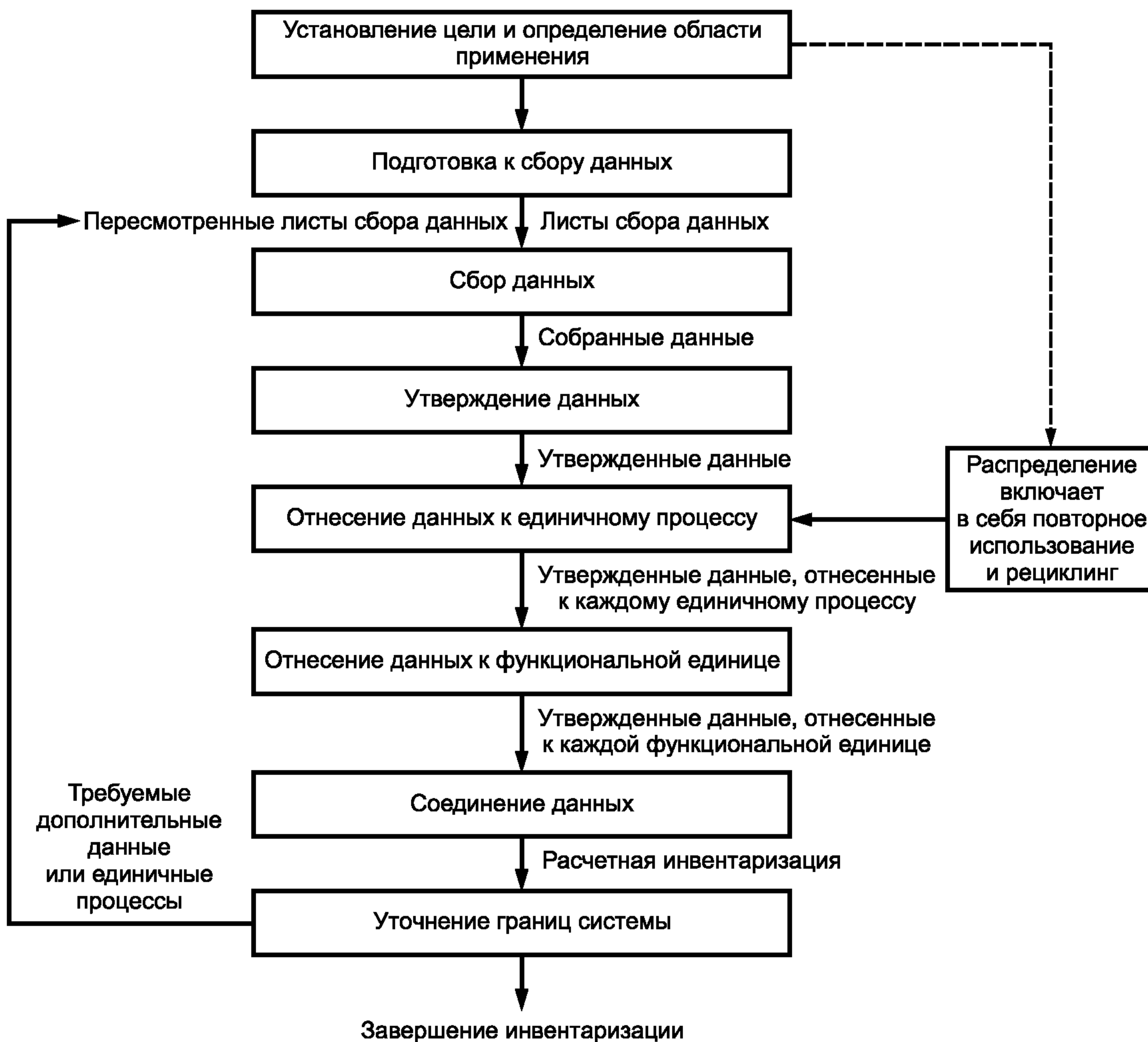
Рисунок 1 — Упрощенные процедуры инвентаризационного анализа
