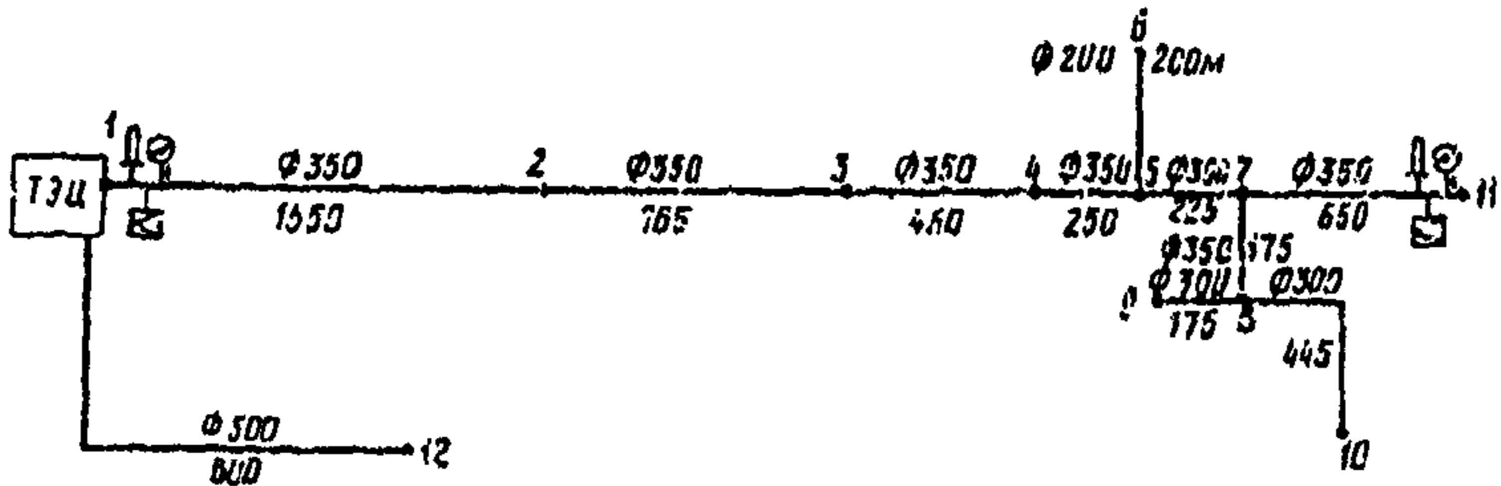
Рис. 3. Схема паропроводов:
