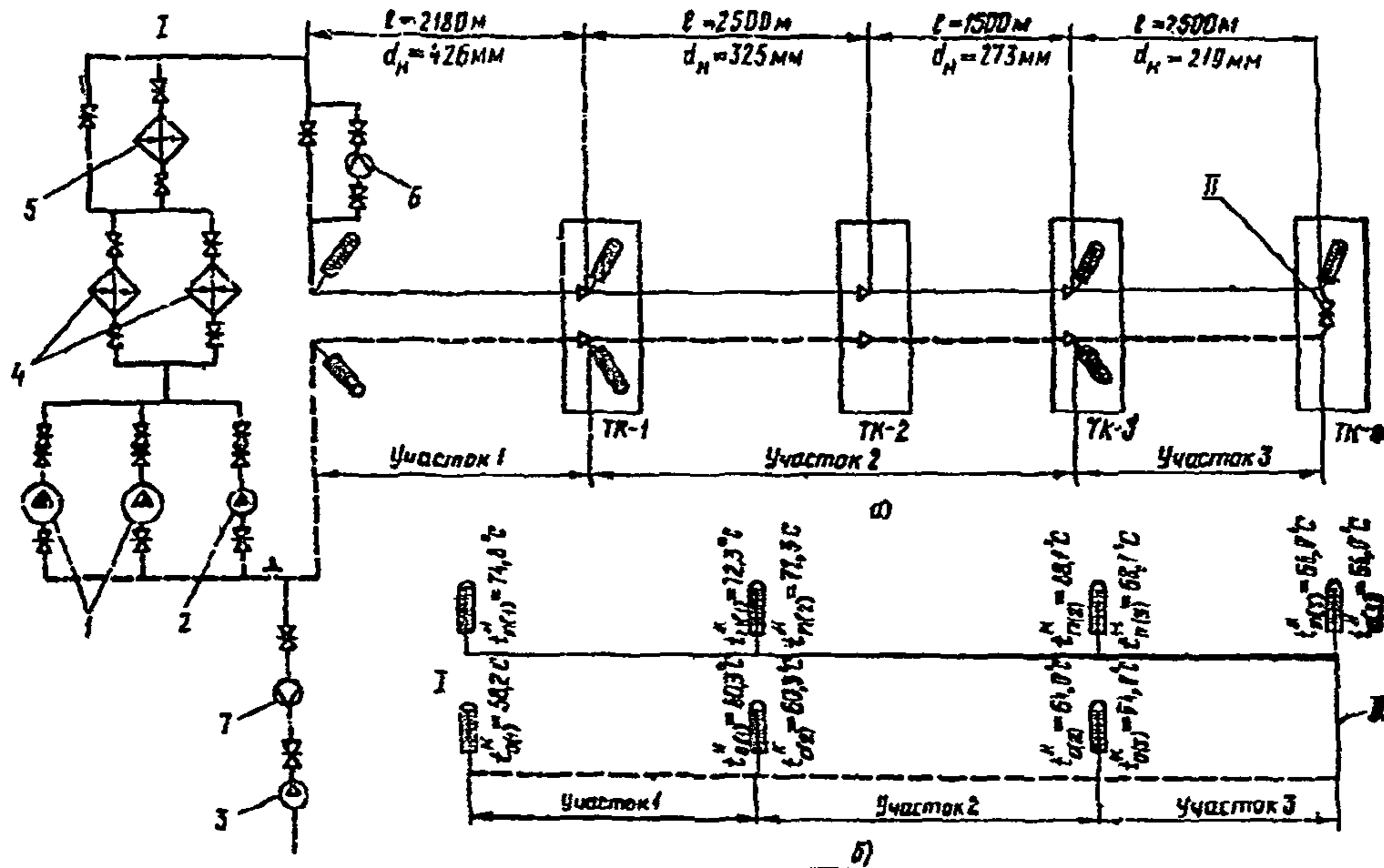
Рис. I. Схема испытываемого циркуляционного кольца:
