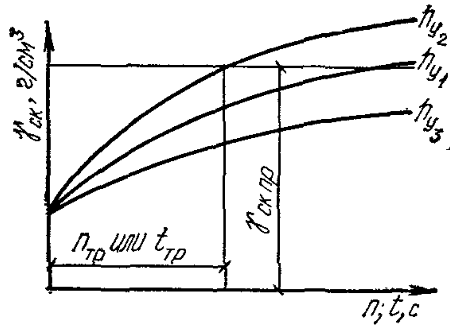
Рис. 3. Зависимость плотности скелета грунта \gamma_{ск} от числа проходов (ударов) n или времени уплотнения t для различных толщин уплотненных слоев
