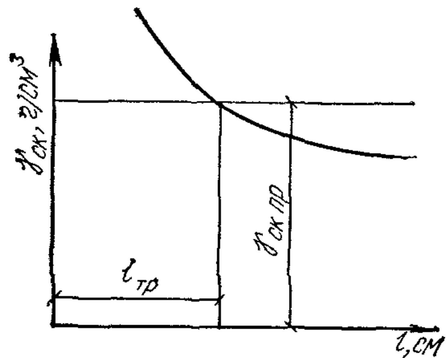
Рис. 4. Зависимость плотности скелета грунта \gamma_{ск} от расстояния между осями скважин l
