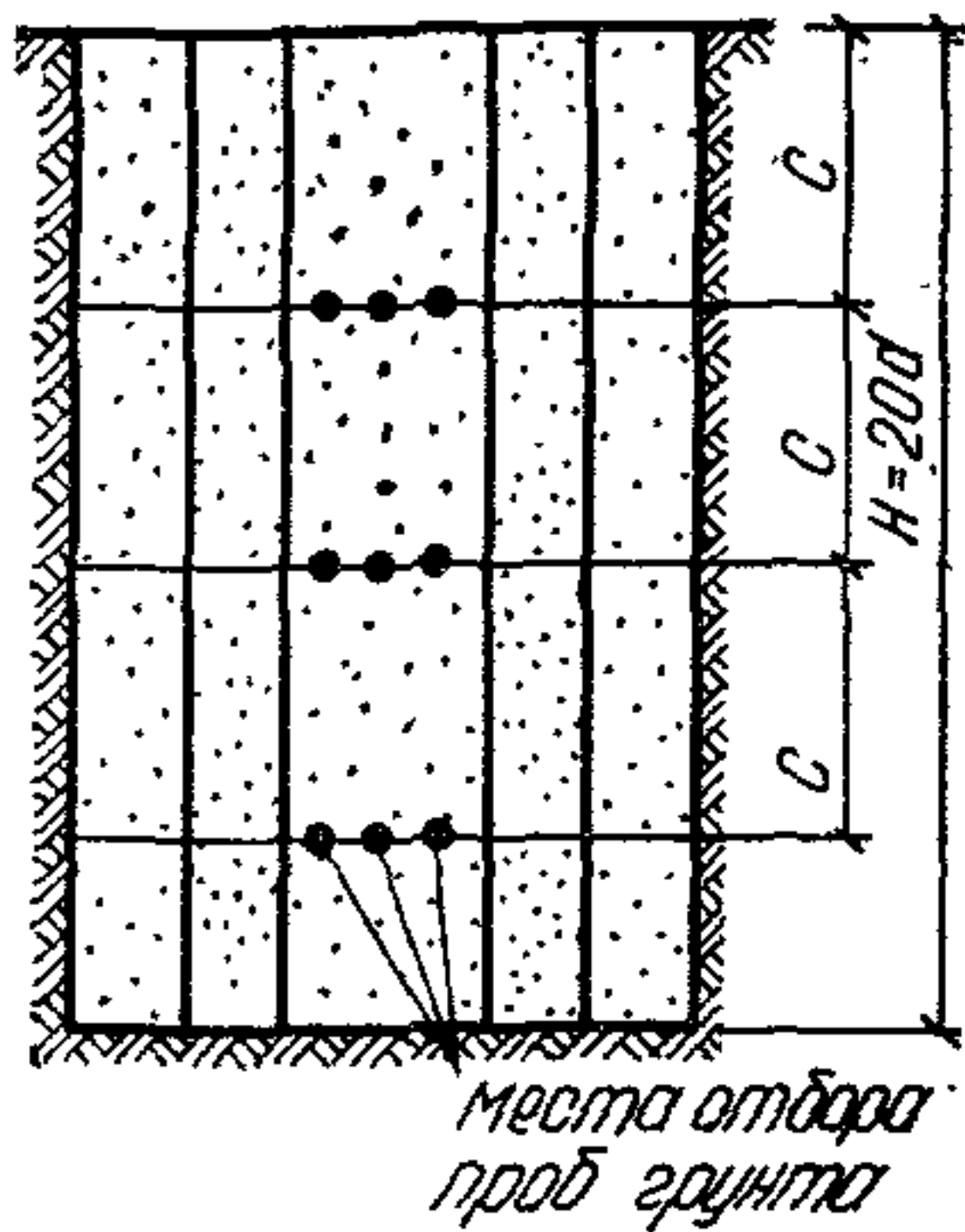
Рис. 2. Схема опытного участка для глубинного уплотнения и места отбора проб грунта A — длина и ширина участка; d — диаметр скважины (рабочего органа); d_y — диаметр зоны уплотненного грунта; l — расстояние между осями скважин; C — расстояние от поверхности до места отбора проб и между точками отбора проб грунта ( C=5d ); H — глубина откапываемого шурфа ( H=20d )
