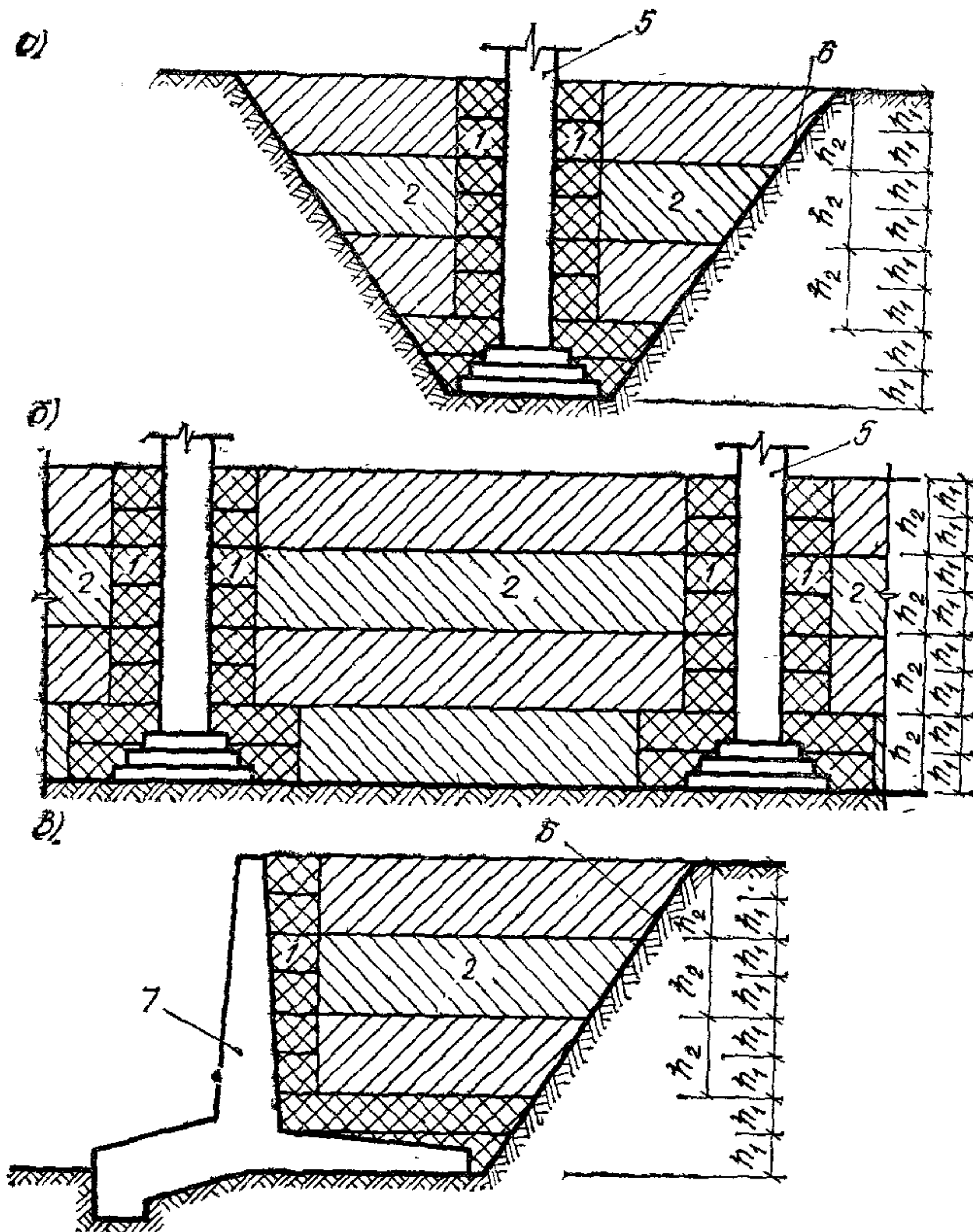
Рис. 1. Виды стесненных мест для обратных засыпок грунта
