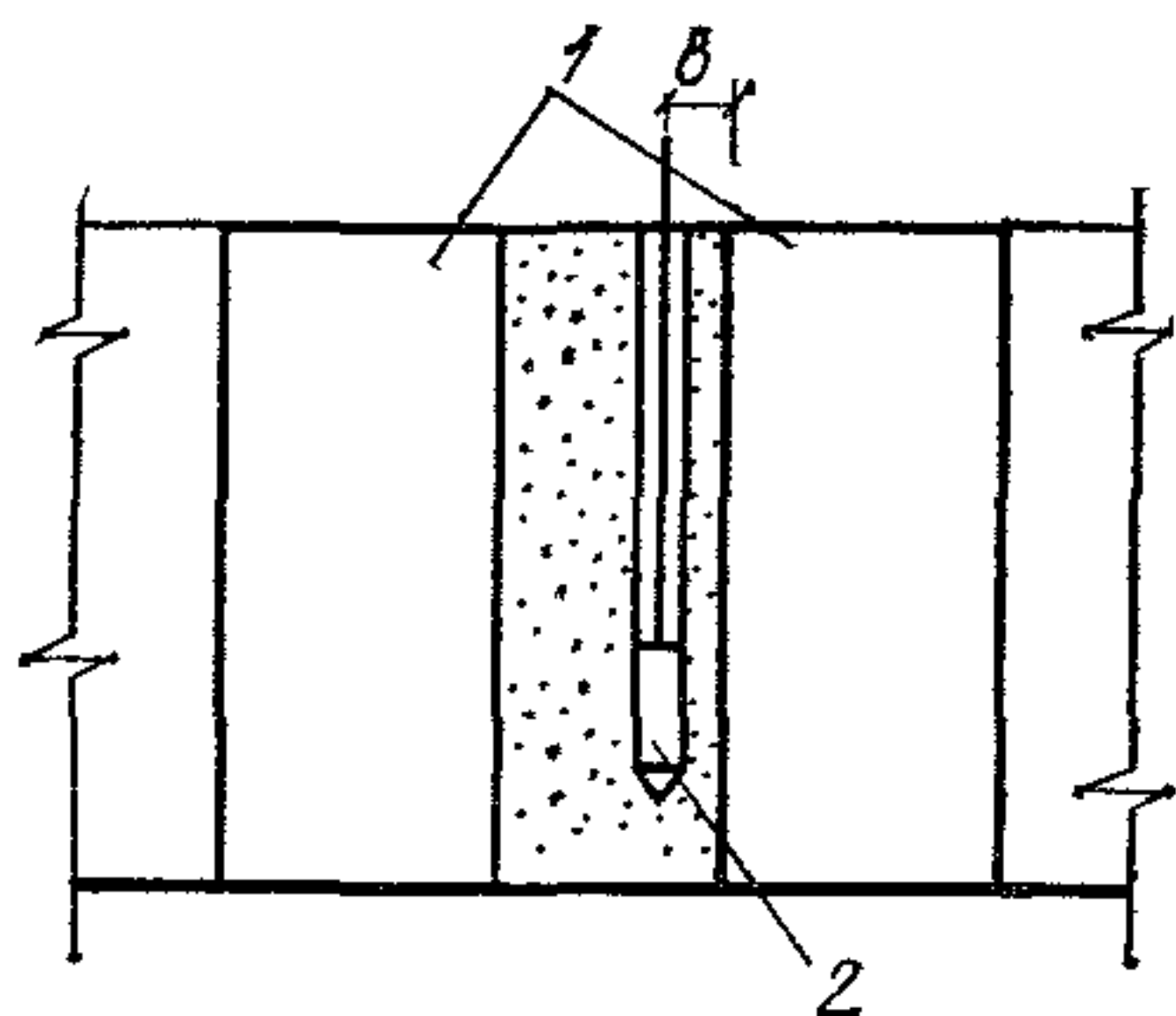
Рис. 7. Схема работы уплотняющих рабочих органов машин и механизмов вблизи строительных конструкций при глубинном уплотнении
