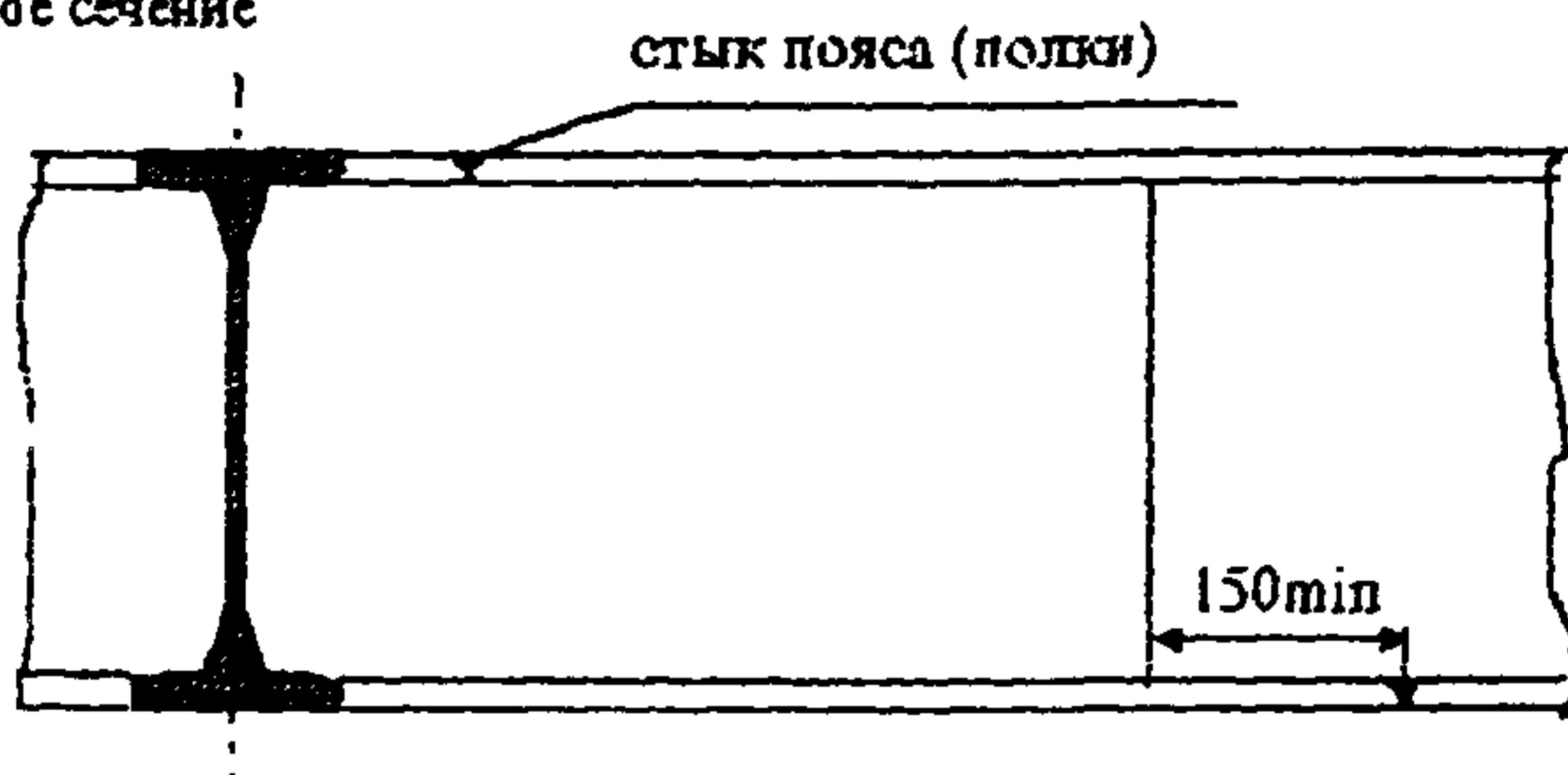
рисунк 1. Расположение сварных стыков в металлоконструкциях коробчатого и двутаврового сечения
