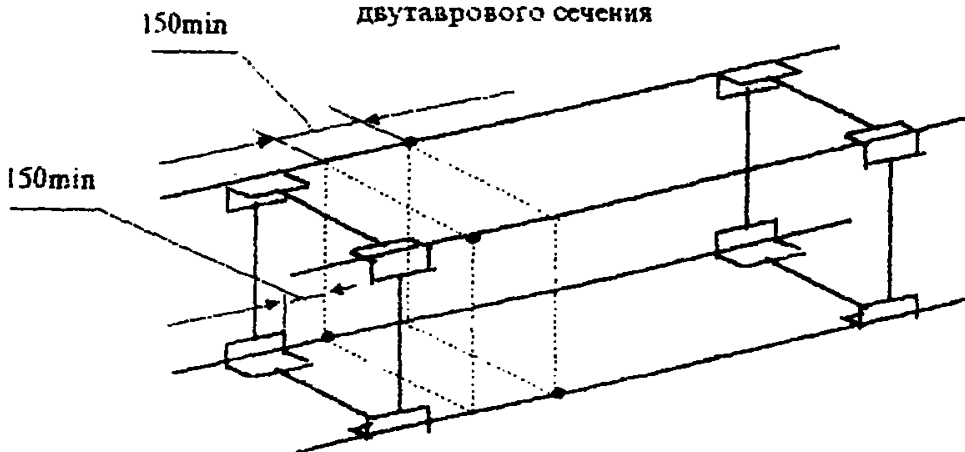
рисунк 2. Расположение сварных стыков в решетчатых металлоконструкциях
