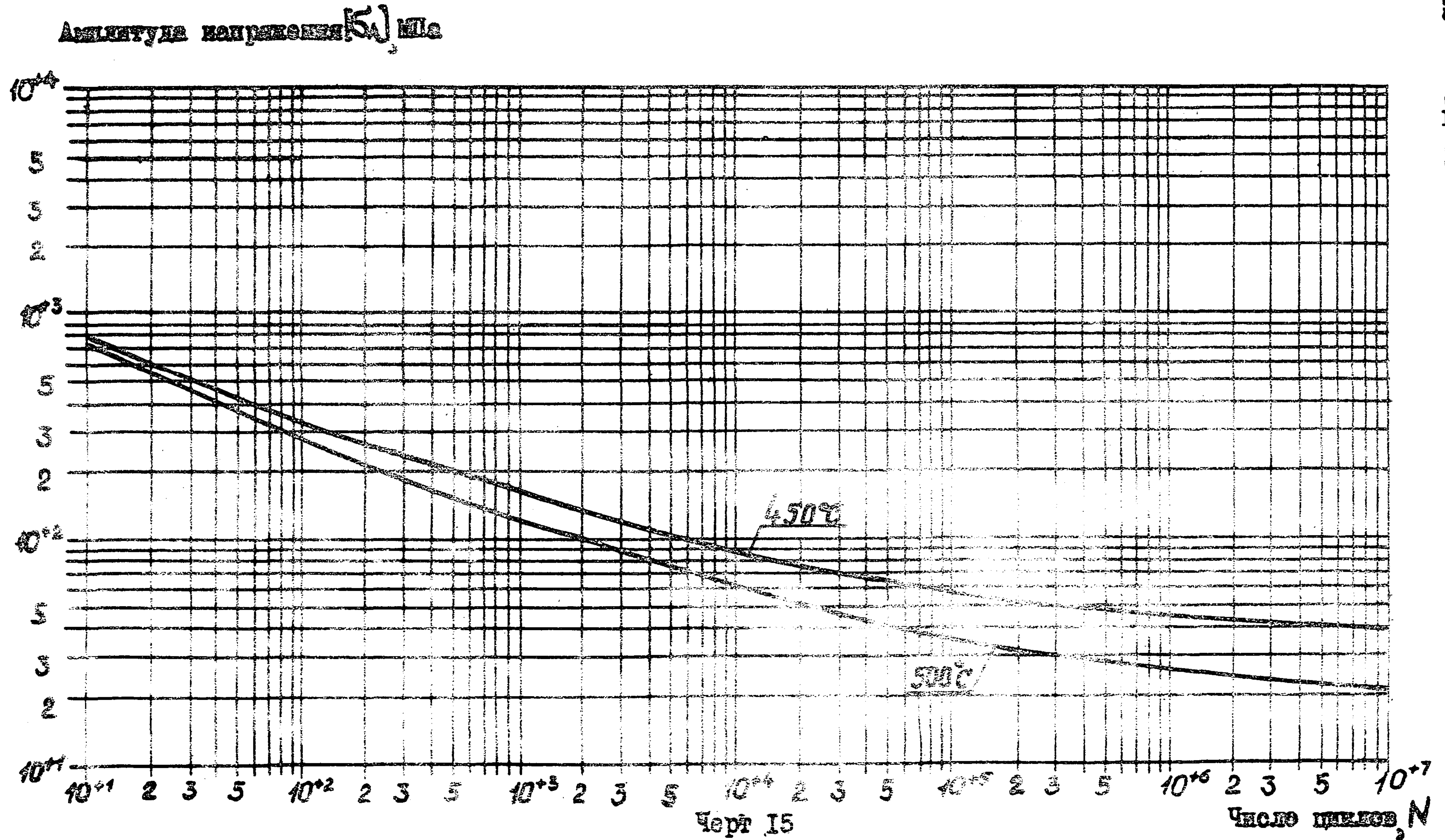
Расчетные кривые усталости для низколегированных и коррозионностойких аустенитных сталей при длительности нагружения \sim 2 \cdot 10^6 ч
