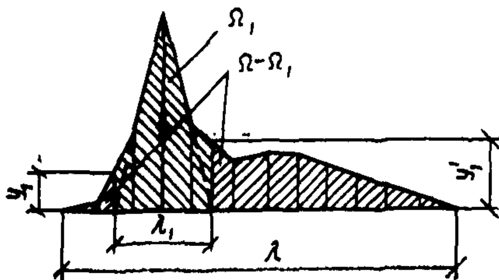
Рис. 2. Линия влияния криволинейного очертания
