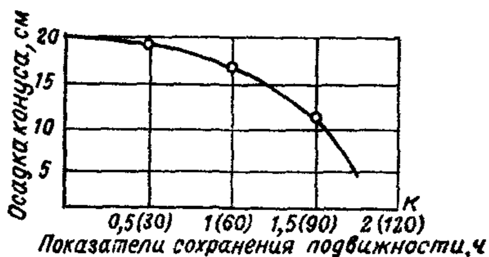
Показатель сохранения подвижности бетонной смеси
