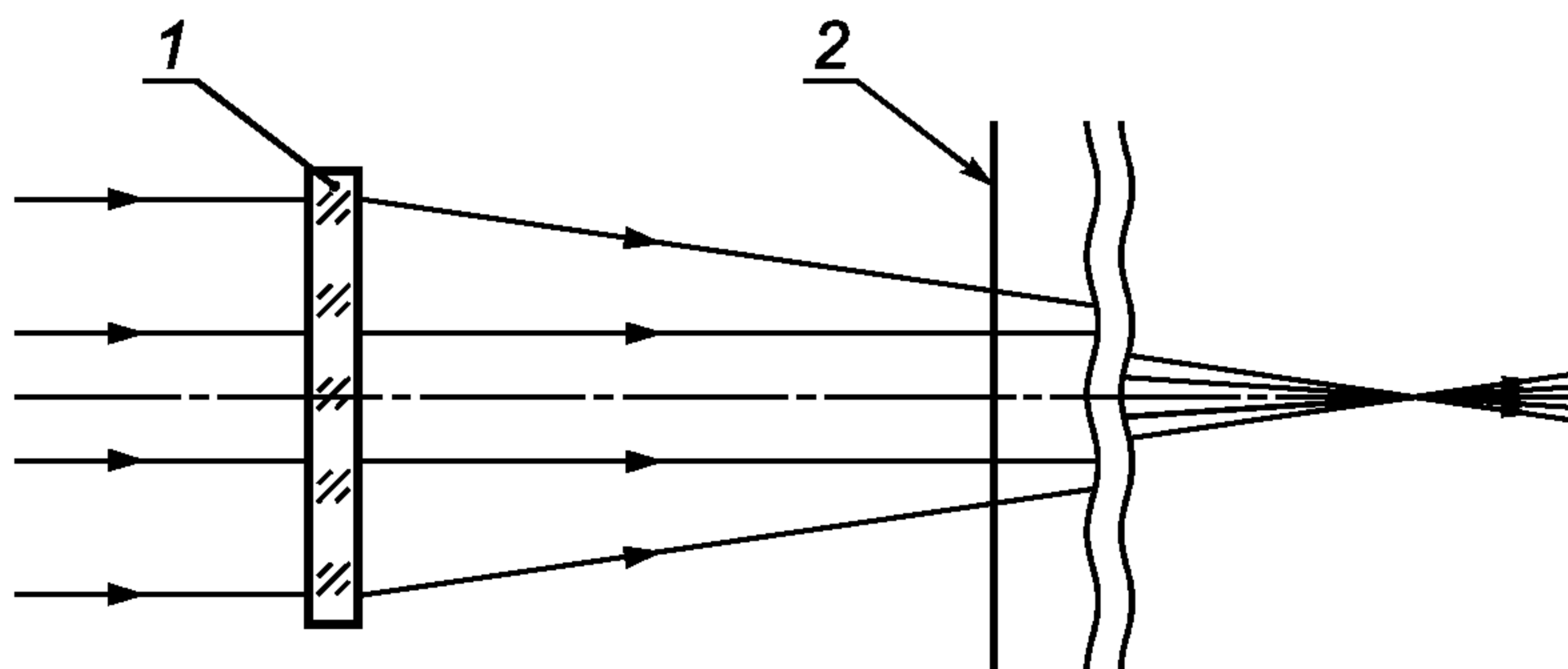
1 — испытуемое очковое стекло; 2 — плоскость измерений
