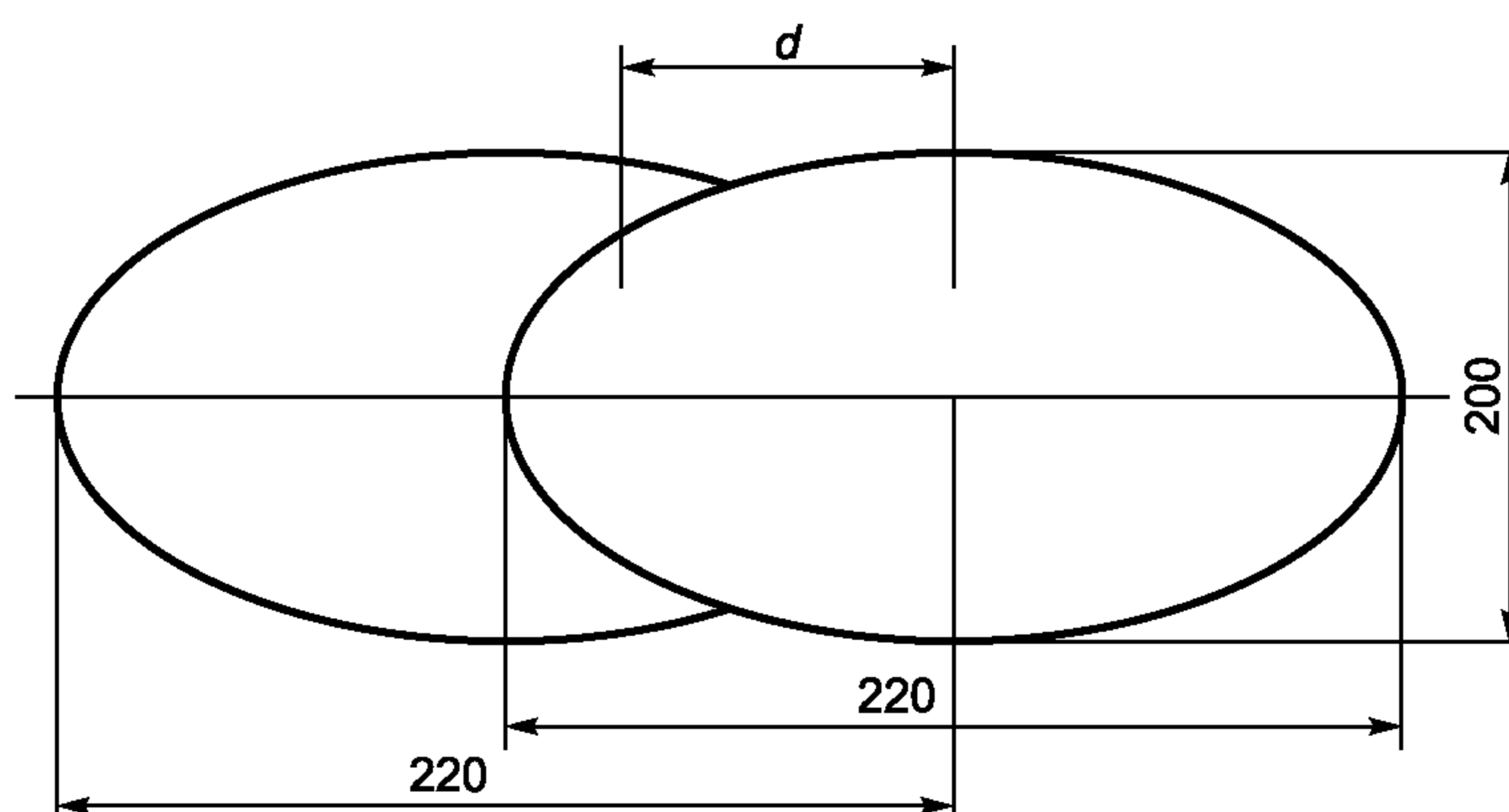
Рисунок 5 — Контрольные эллипсы для измерения поля зрения
