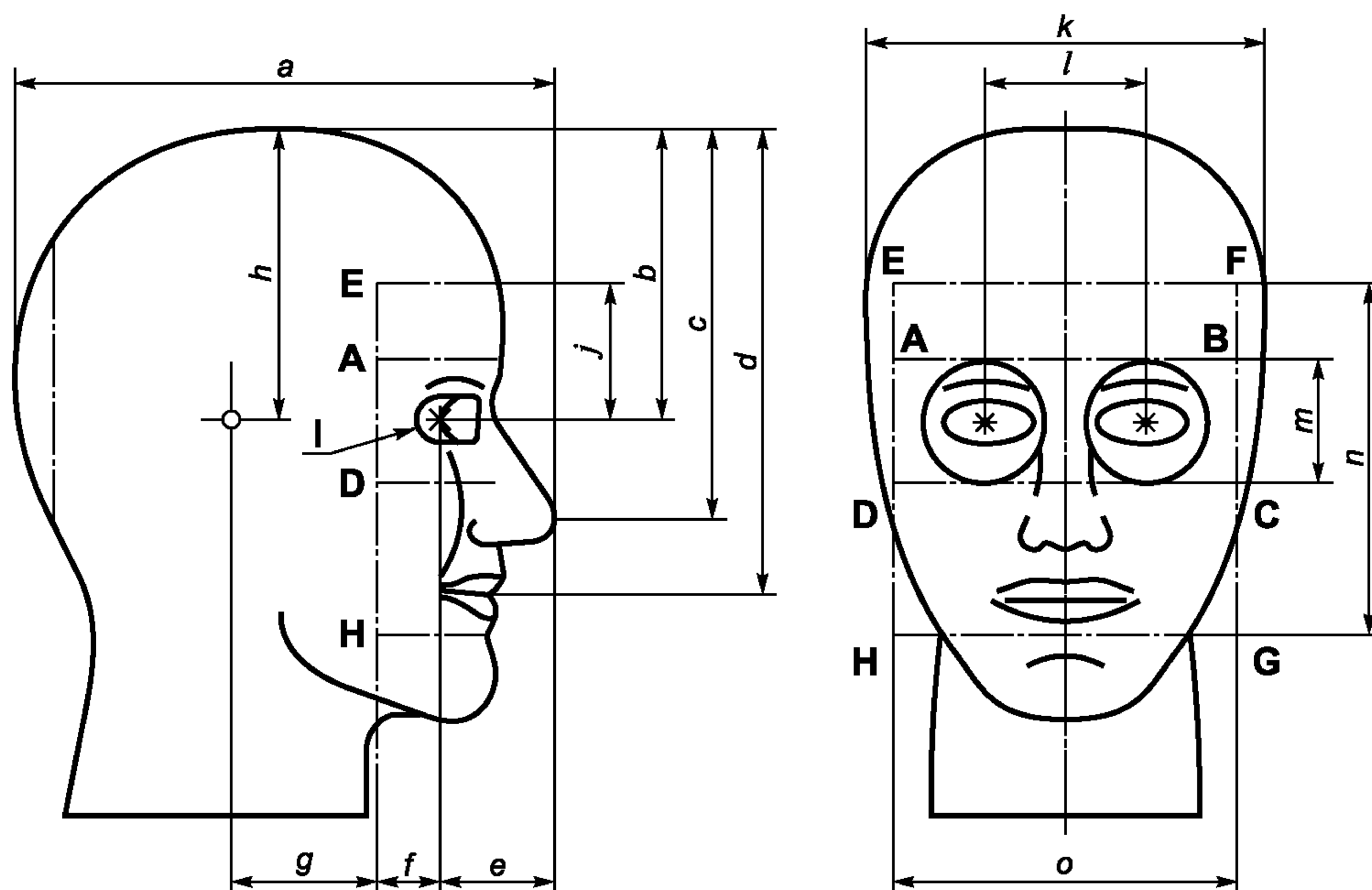
Рисунок А.1 — Тип контрольного макета головы человека
