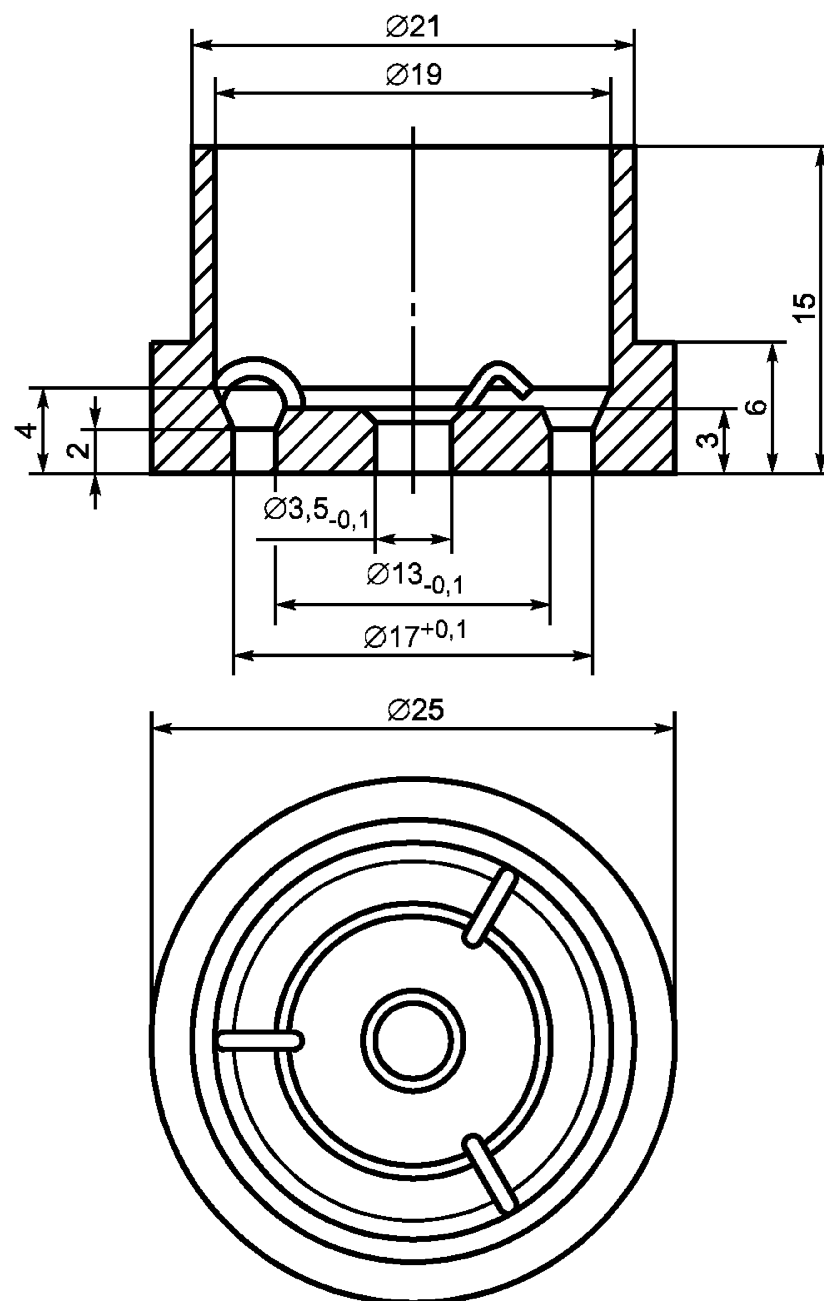
Рисунок 18 — Выходное сопло контейнера
