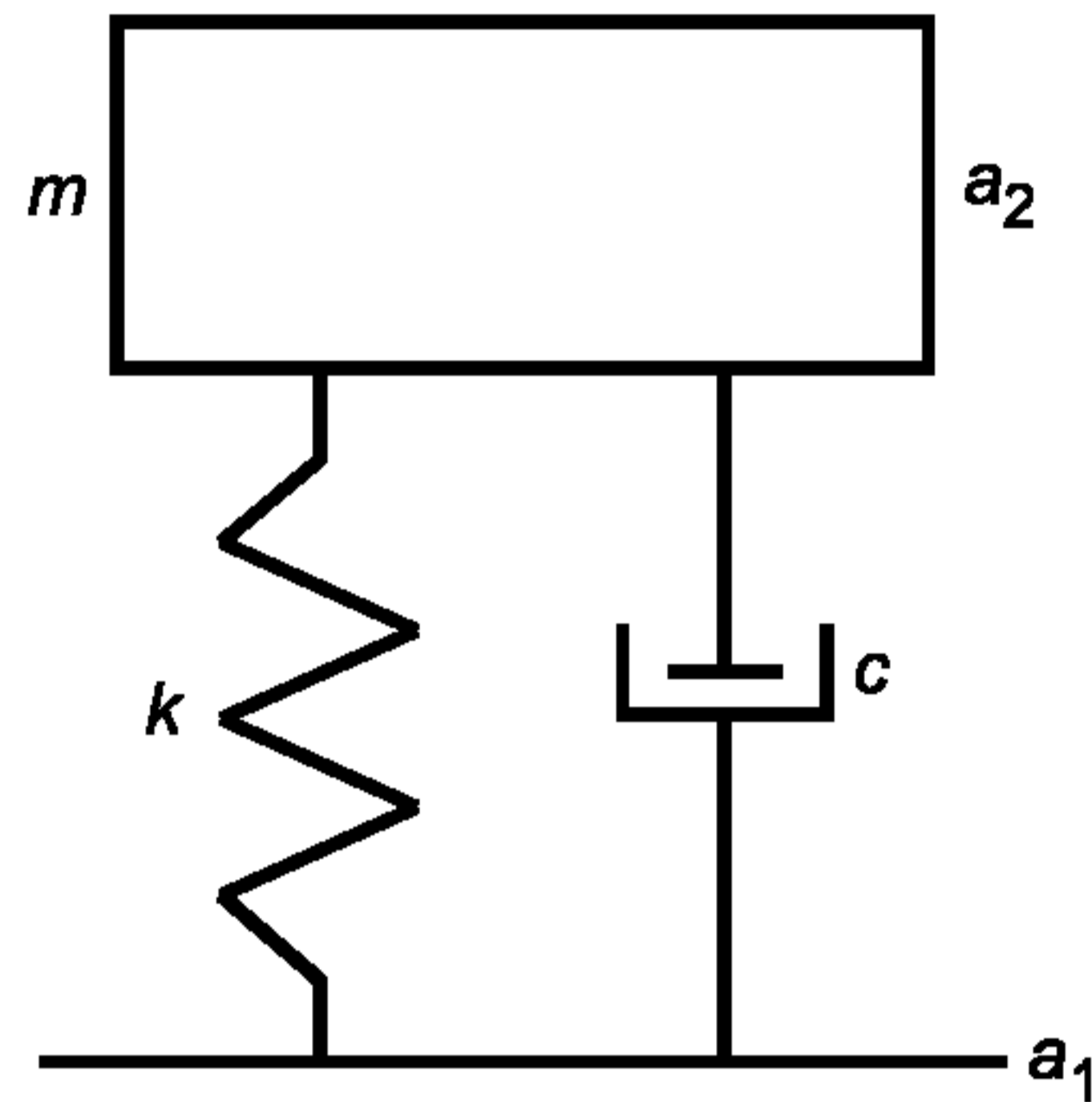
Рисунок А.1 — Система с одной степенью свободы
