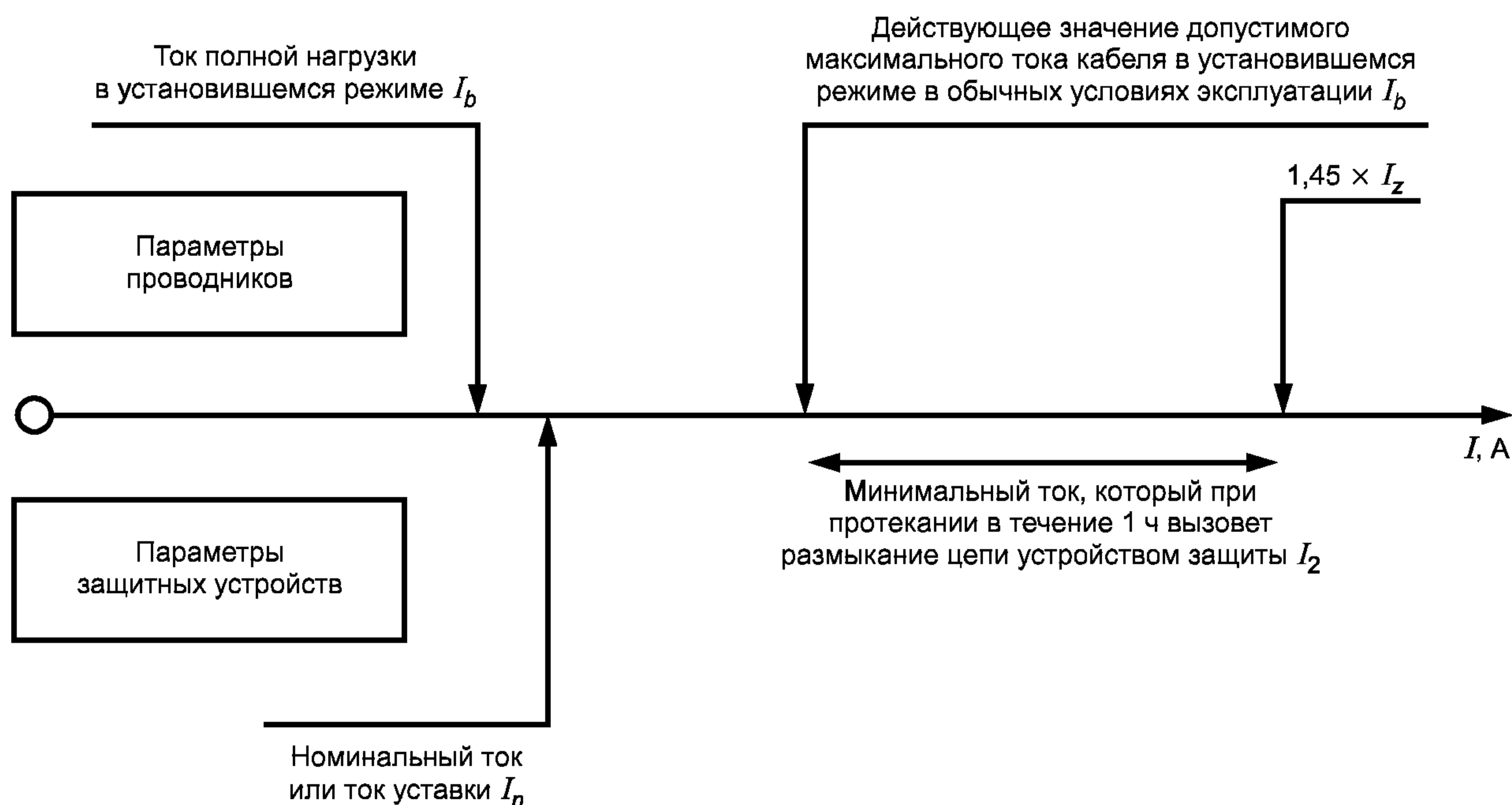
Рисунок D.2 — Параметры проводников и защитных устройств
