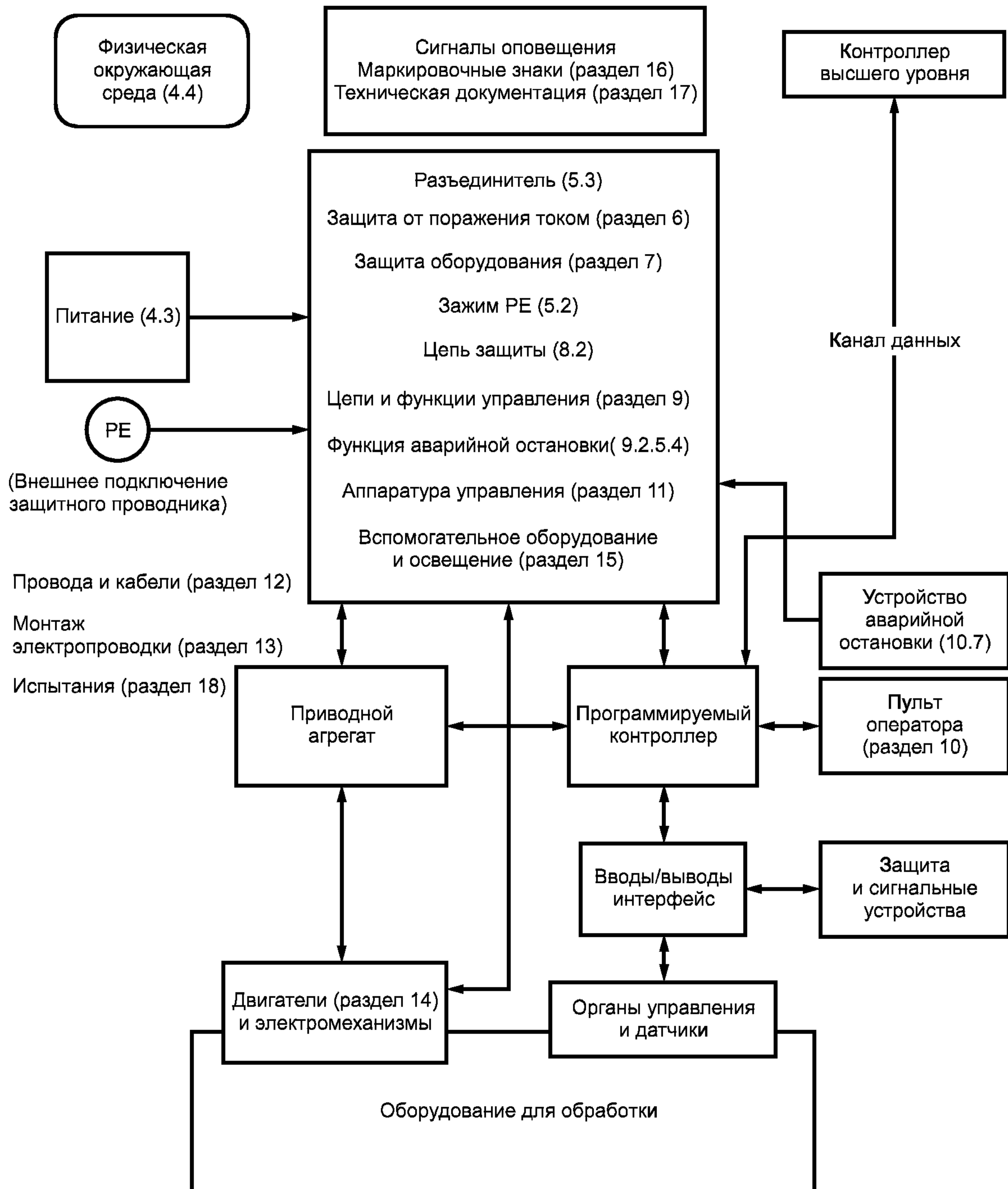
Рисунок 1 — Функциональная схема типовой машины
