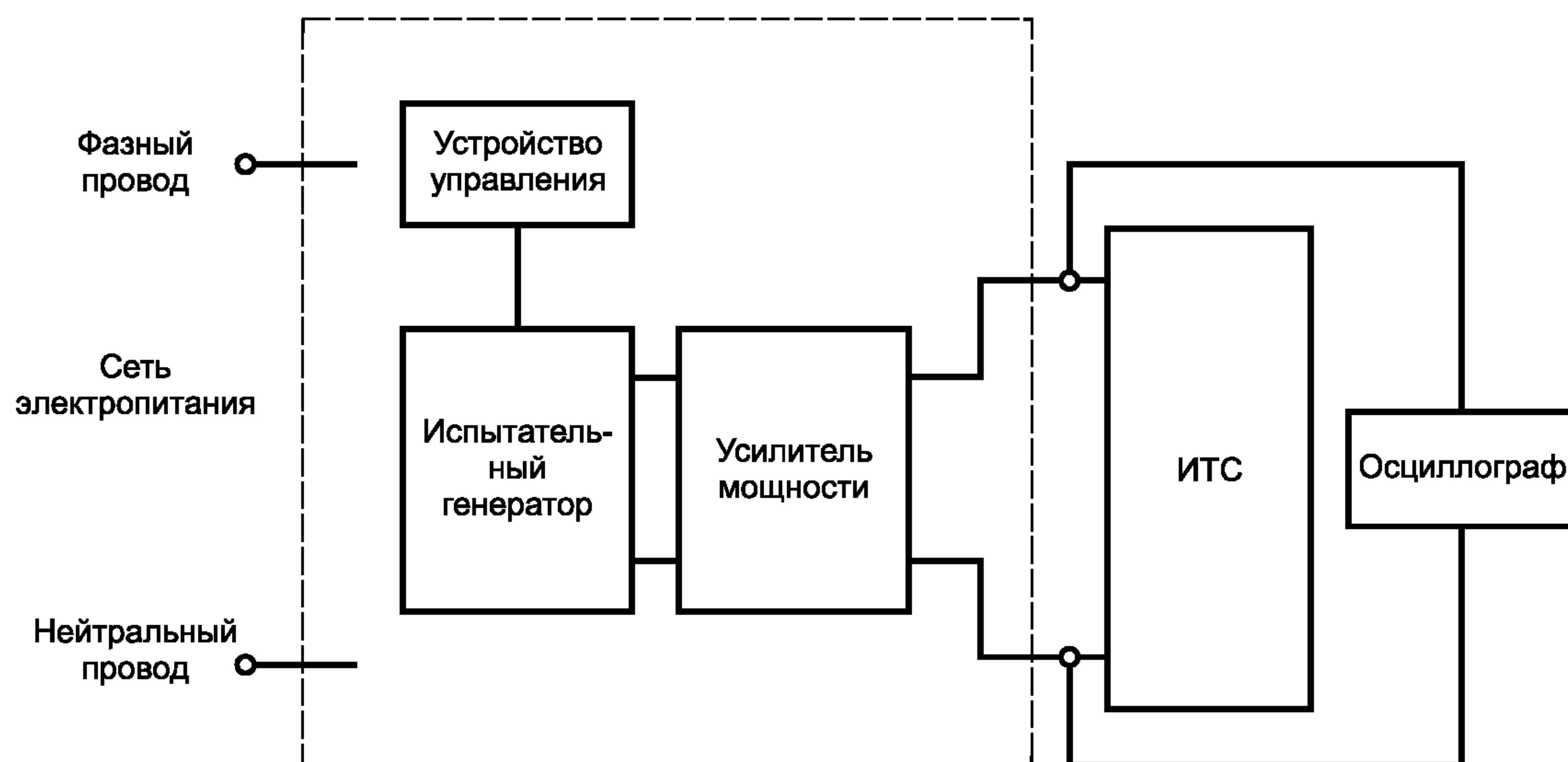
б) Схема испытаний с использованием усилителя мощности
