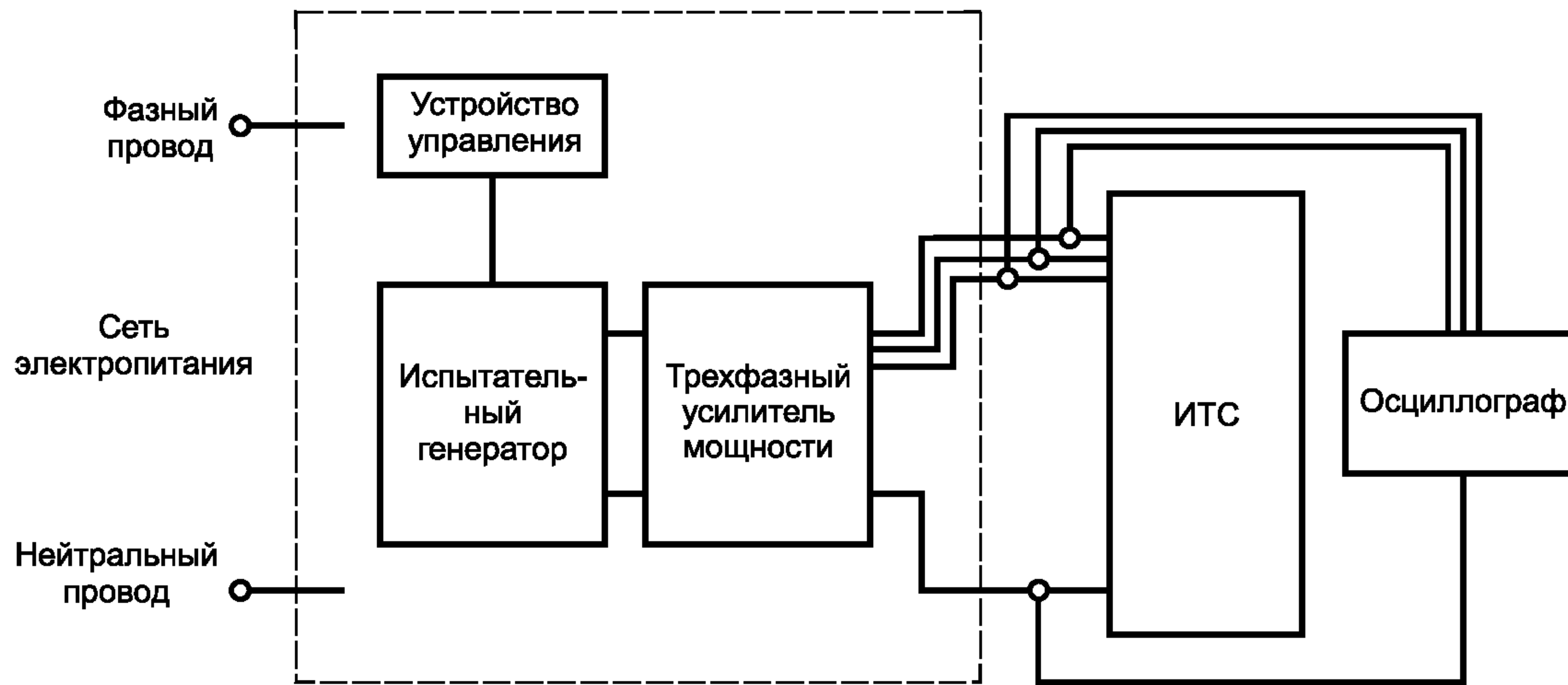
Рисунок В.2 — Схема установки для испытаний трехфазных систем при воздействии провалов, кратковременных прерываний и изменений напряжения электропитания
