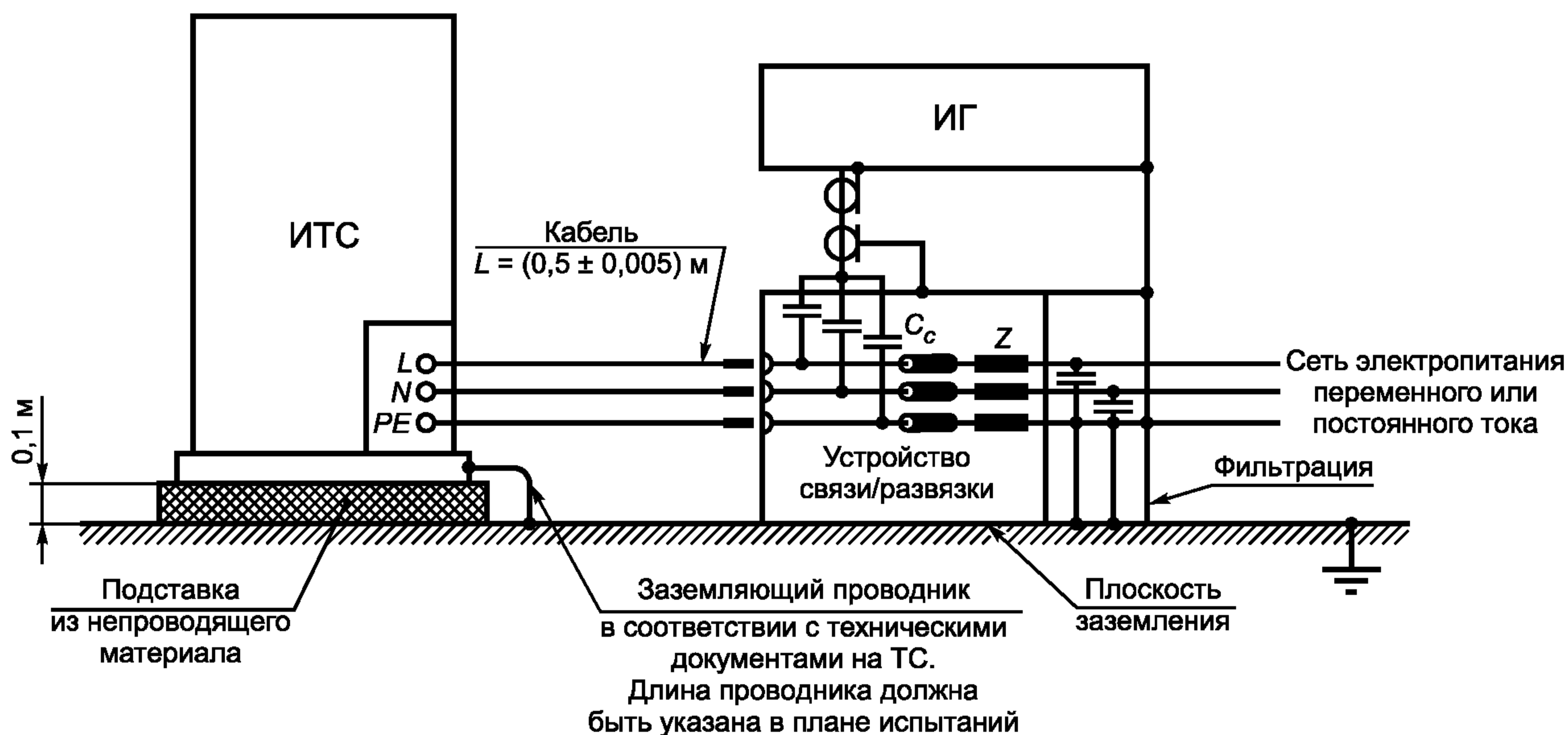
Рисунок 8 — Пример установки для испытания оборудования в стойке
