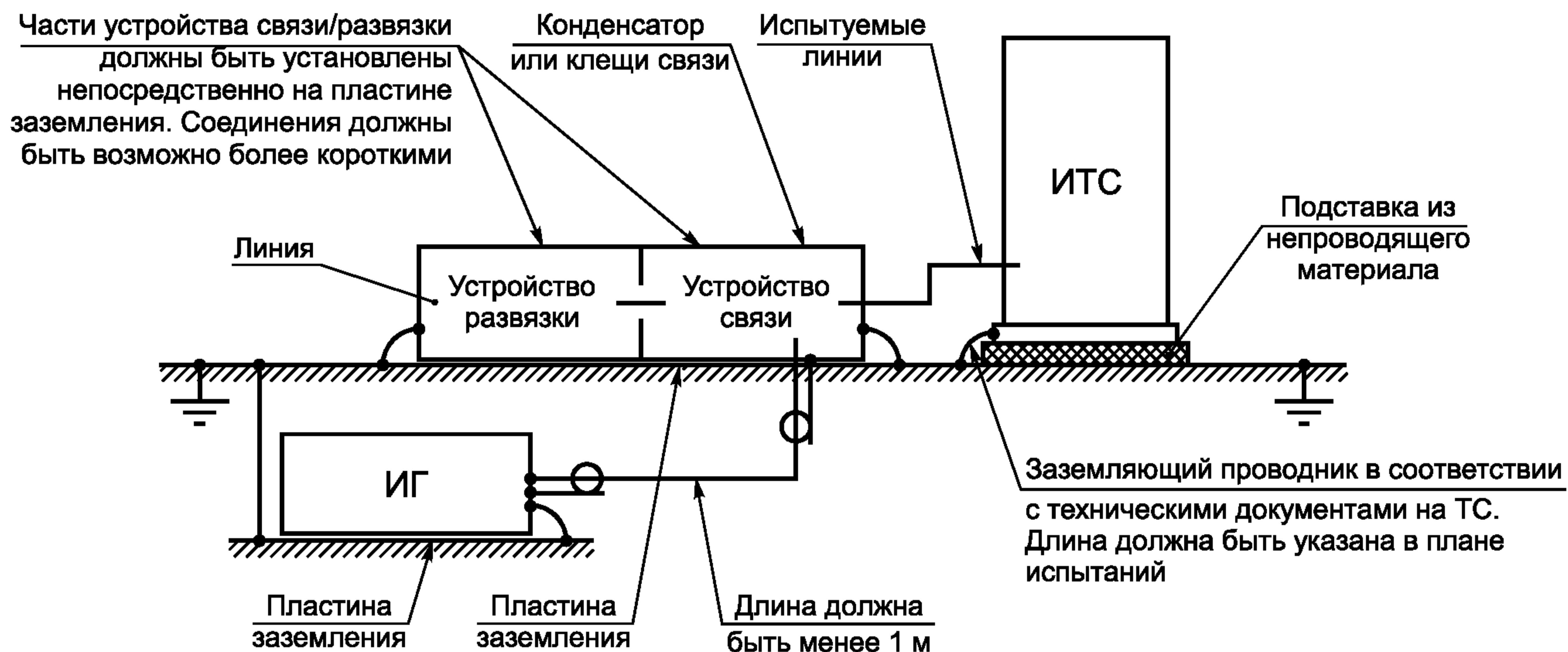
Рисунок 6 — Схема испытаний ТС на устойчивость к НИП
