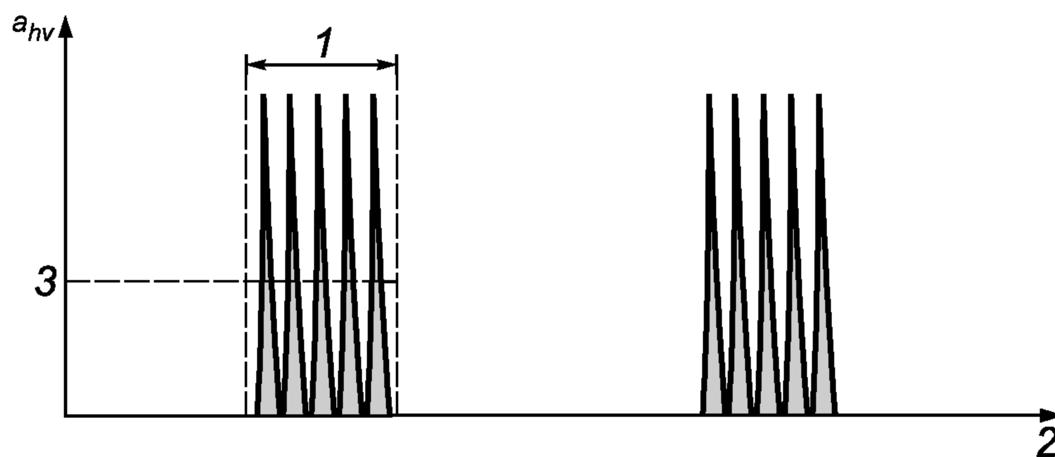
1 — длительность измерений; 2 — время; 3 — a_{hv,measured}
