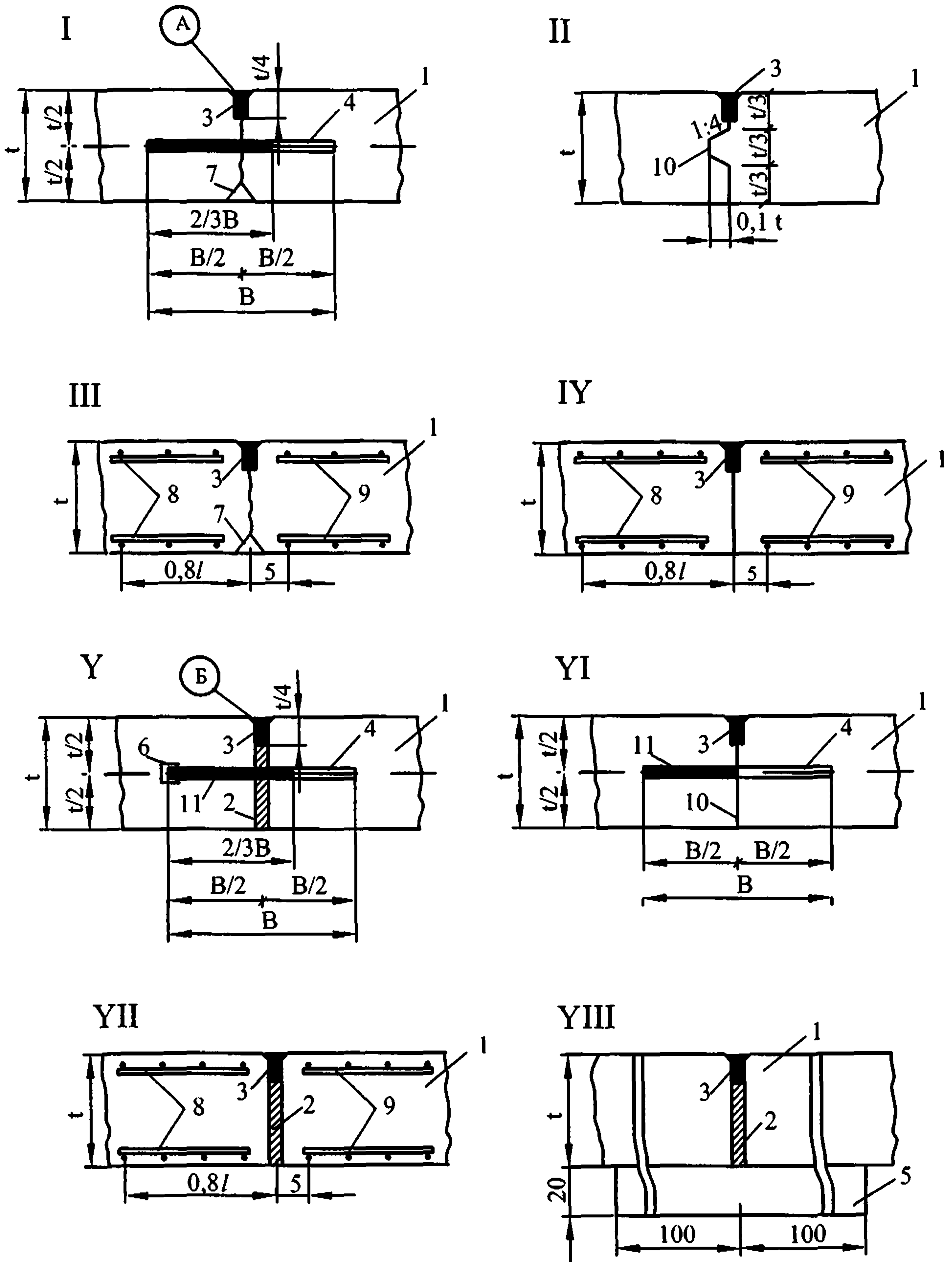
Рис.4.1. Схемы конструкций деформационных швов
