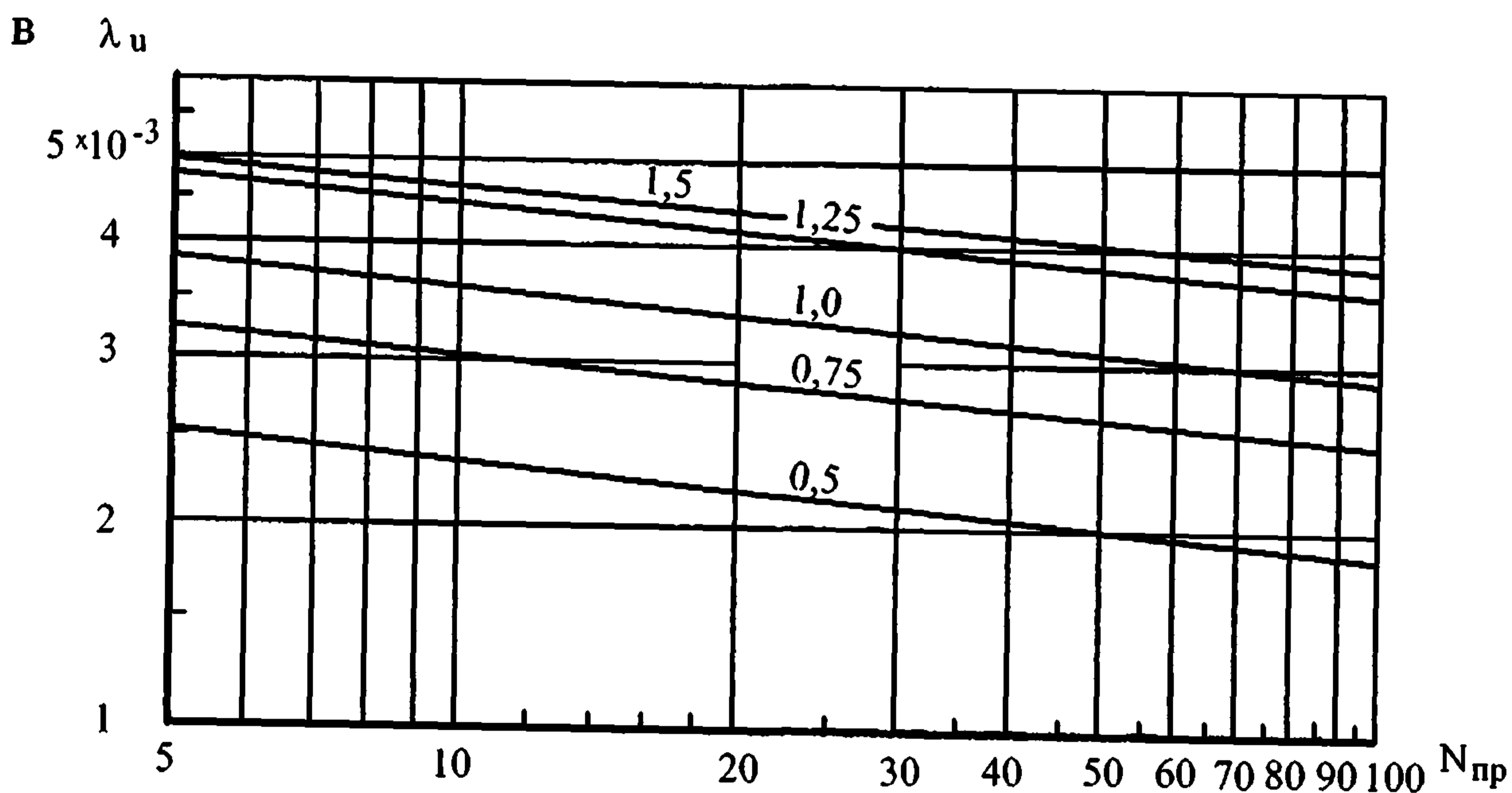
Рис.12.2. Графики предельных относительных прогибов нежестких аэродромных покрытий, устраиваемых на грунтах:
