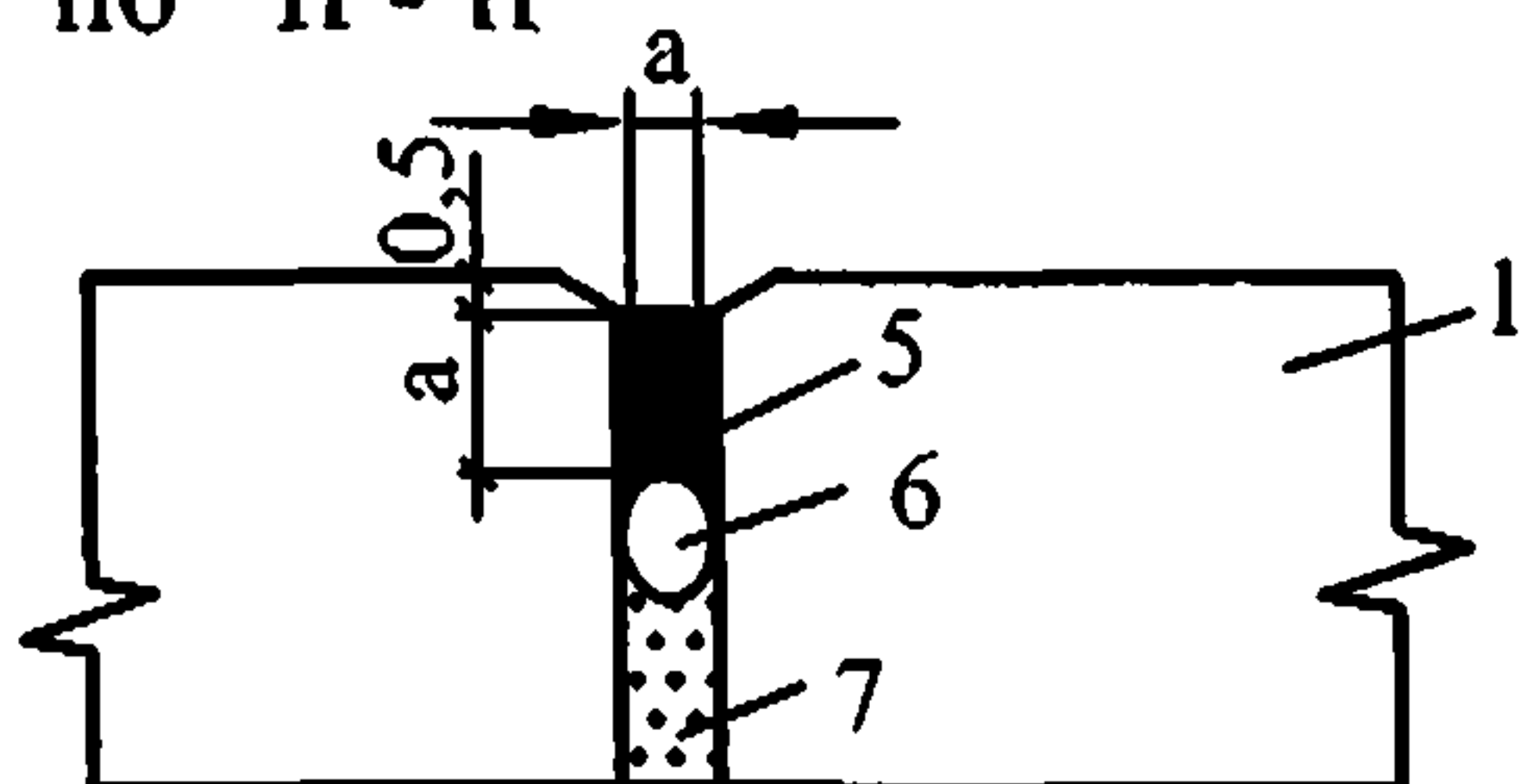
Рис.4.3. Швы в сборном покрытии из плит типа ПАГ
