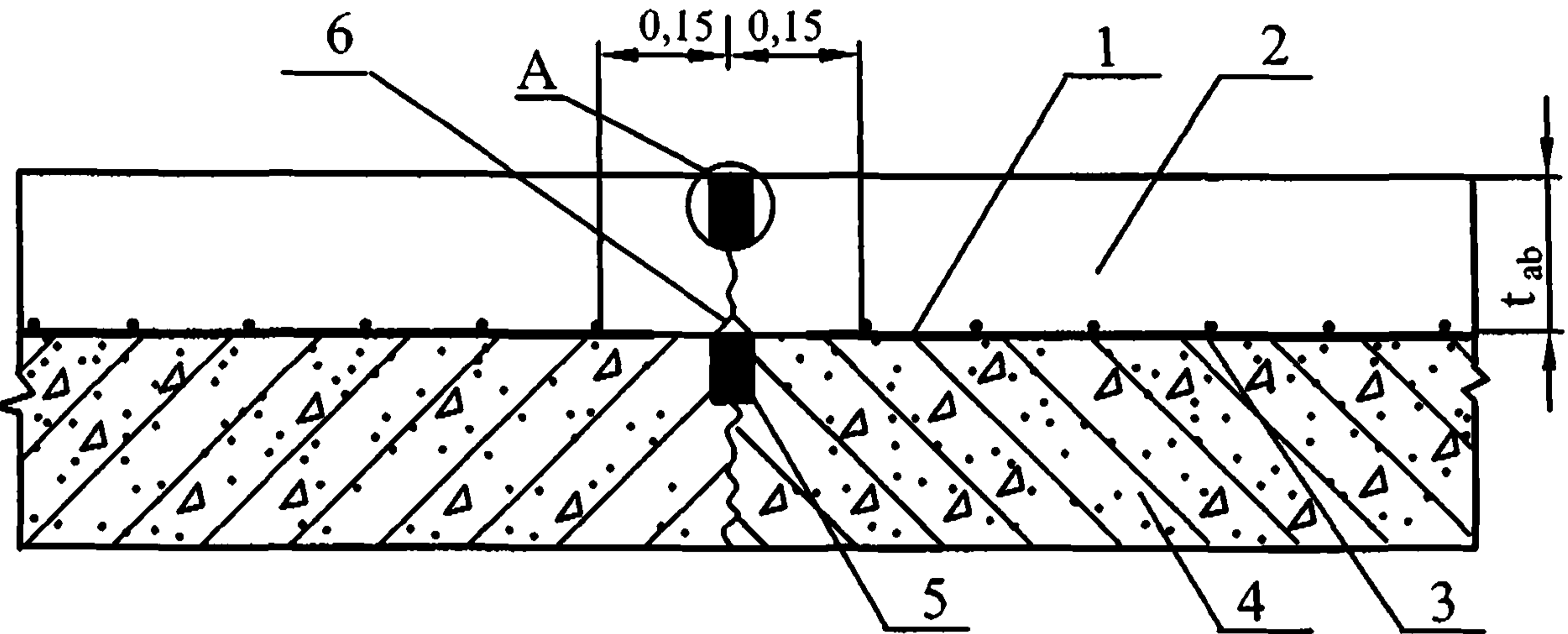
Рис.5.5. Деформационный шов в однослойном асфальтобетонном покрытии:
