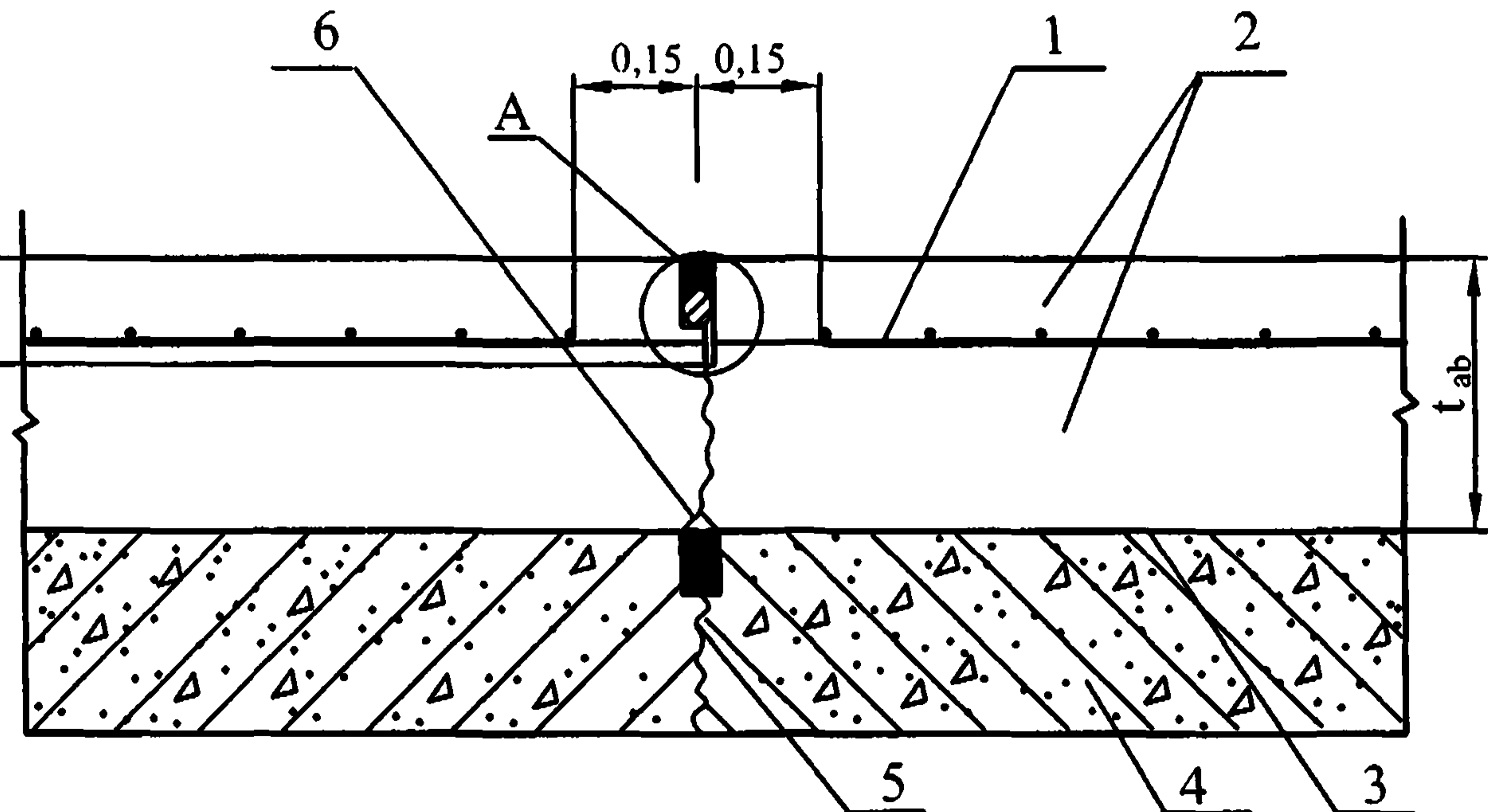
Рис.5.6. Деформационный шов в двухслойном асфальтобетонном покрытии:
