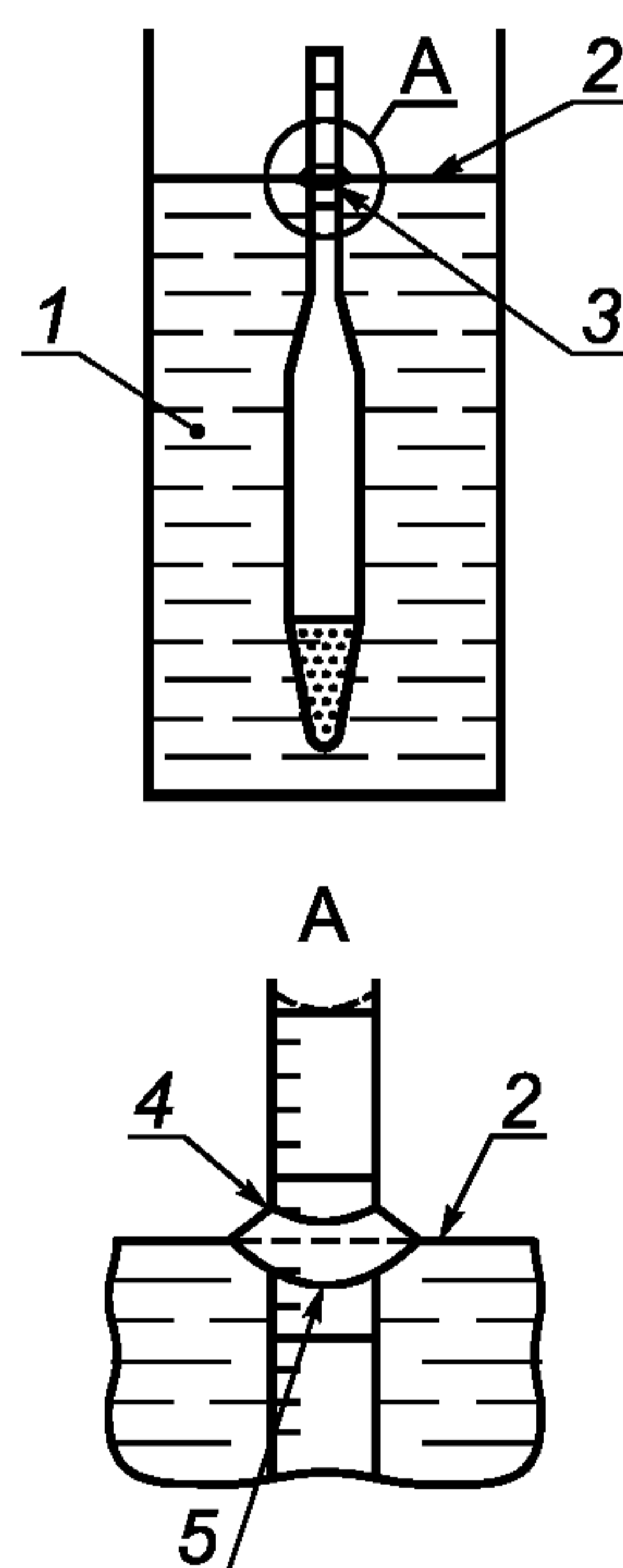
1 — жидкость; 2 — горизонтальная плоская поверхность жидкости; 3 — нижняя часть мениска; 4 — место считывания шкалы; 5 — мениск
