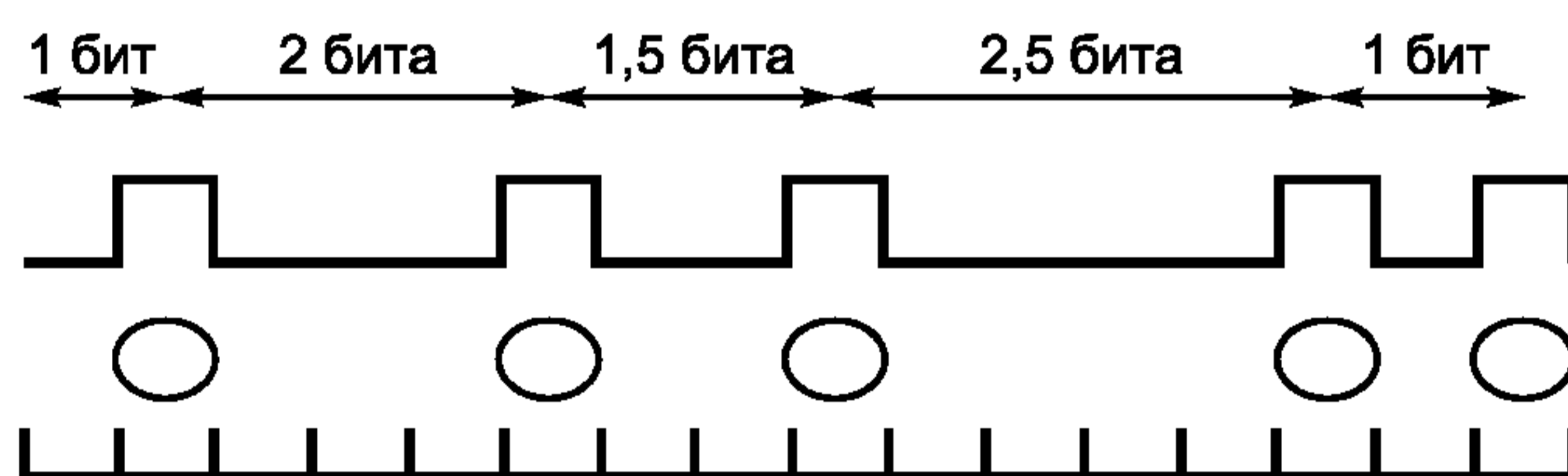
Рисунок В.2 — Структура синхронизирующей метки
