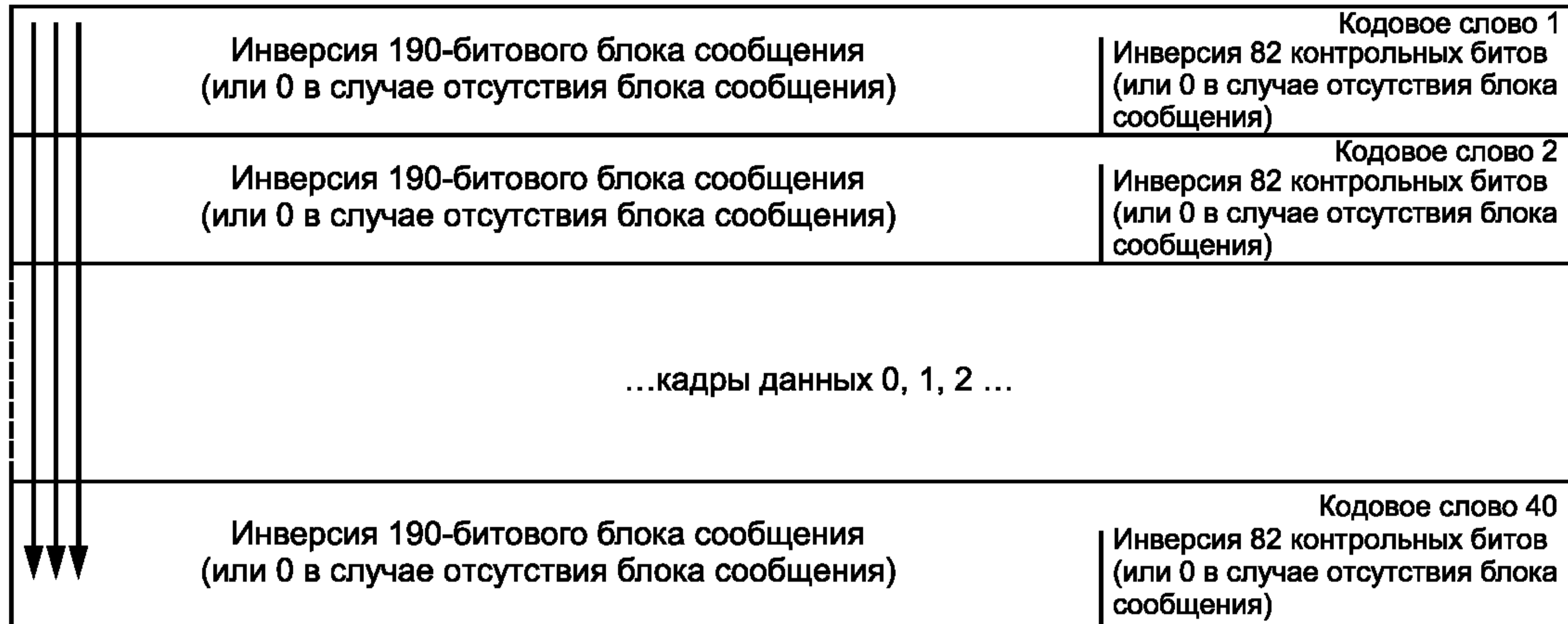
Рисунок В.15 — Перемежение данных сектора с кодом EDAC, секторы типов 7—15
