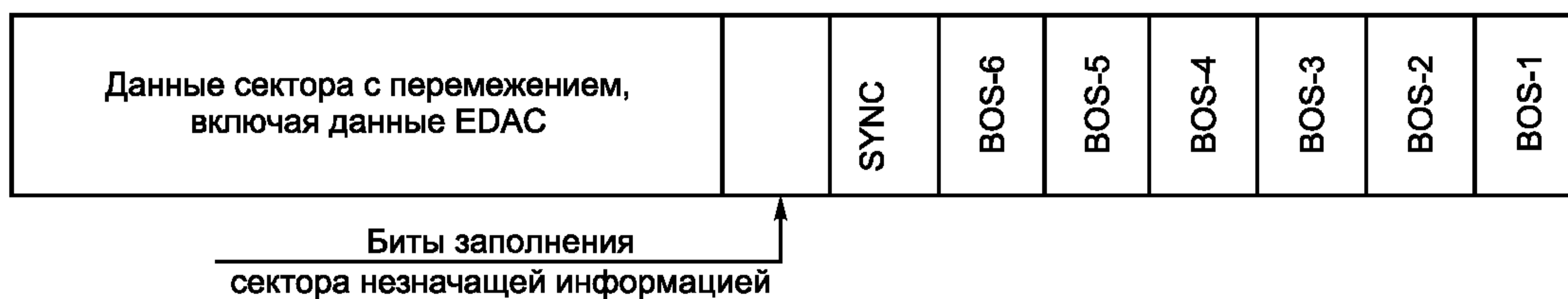
Рисунок В.8 — Структура сектора, типы 0—5
