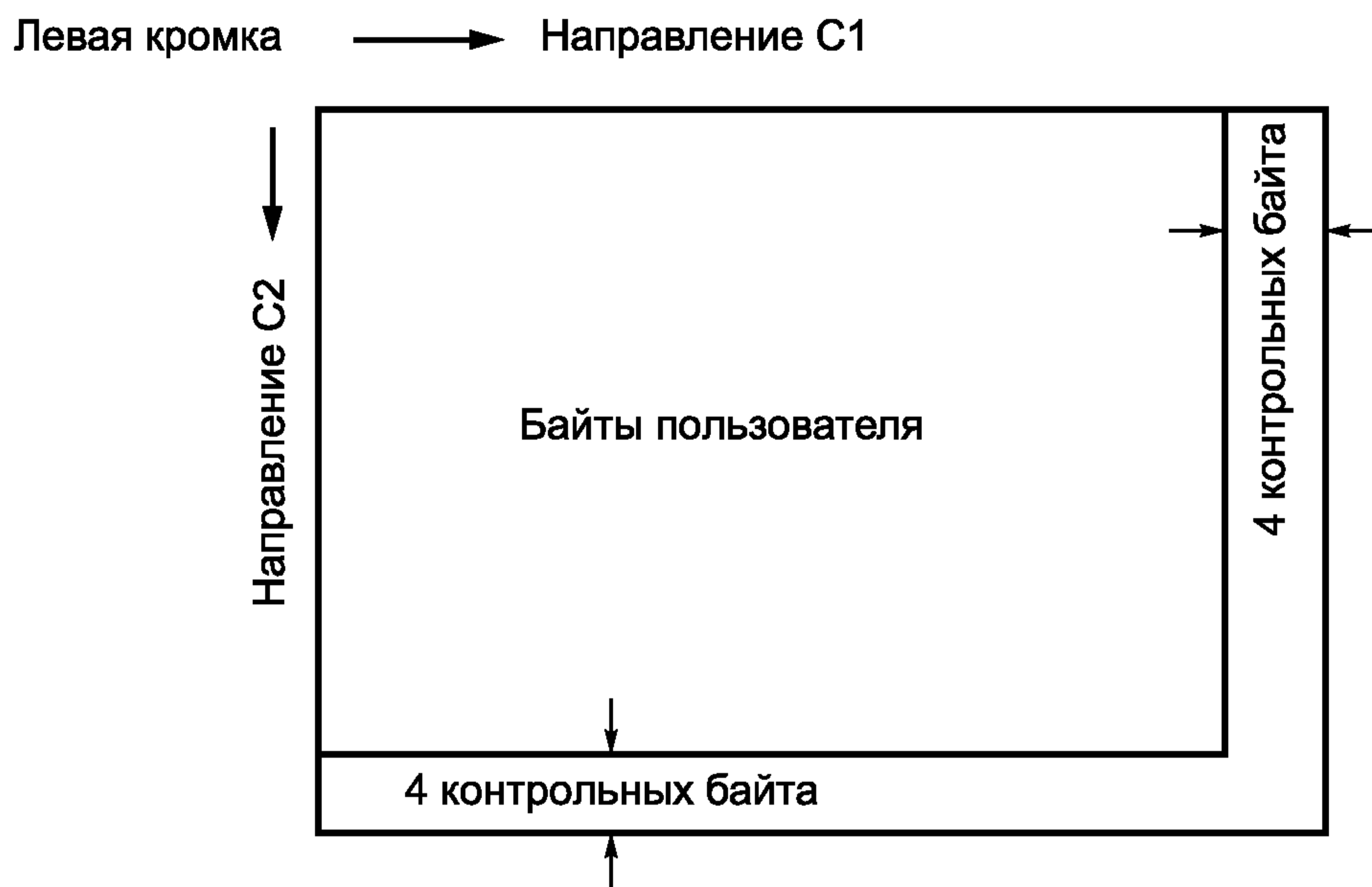
а) Компоновка сектора с добавлением ECC
