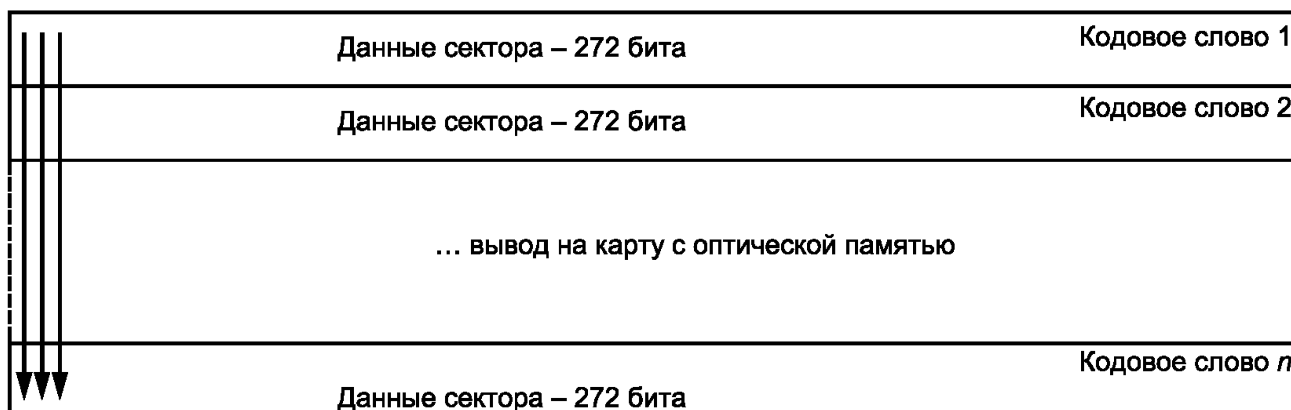
Рисунок В.14 — Перемежение данных сектора, сектор типа 5
