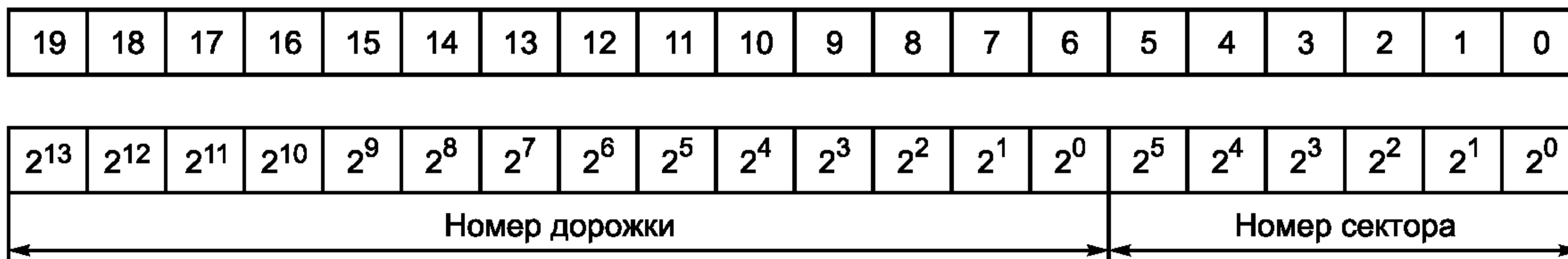
Рисунок В.4 — Формат адреса сектора и дорожки
