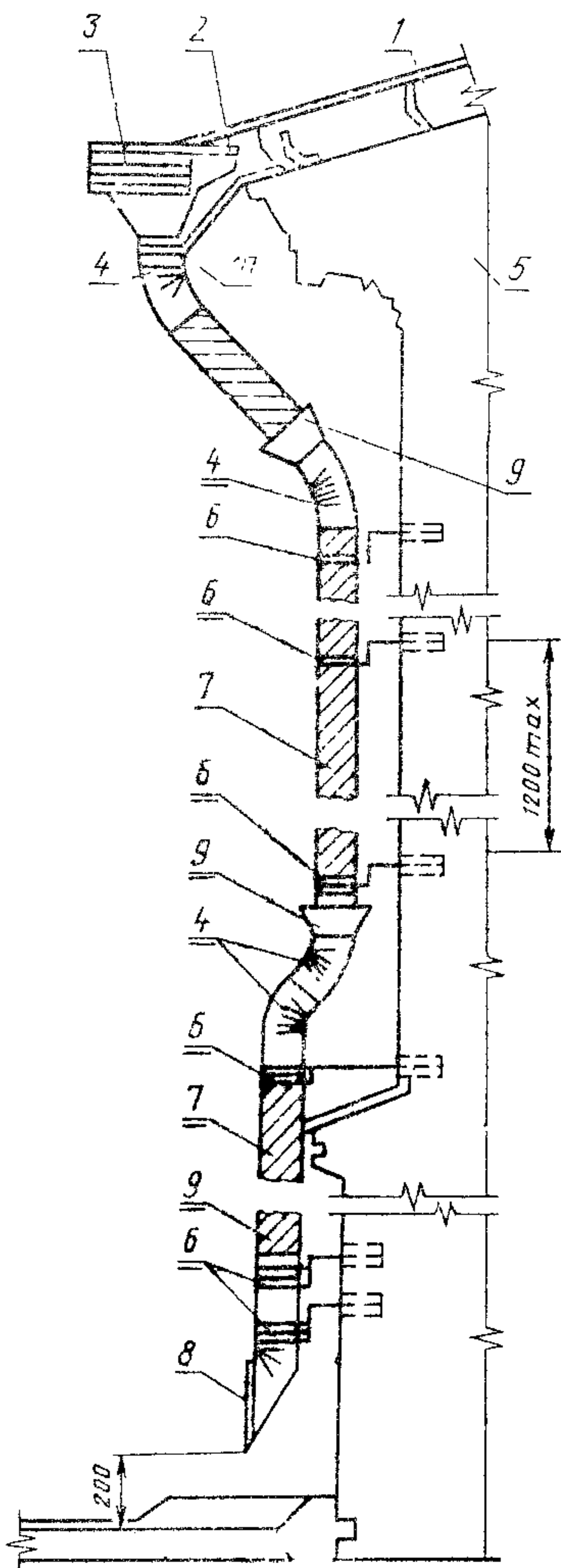
Применение звеньев труб типа ТС
