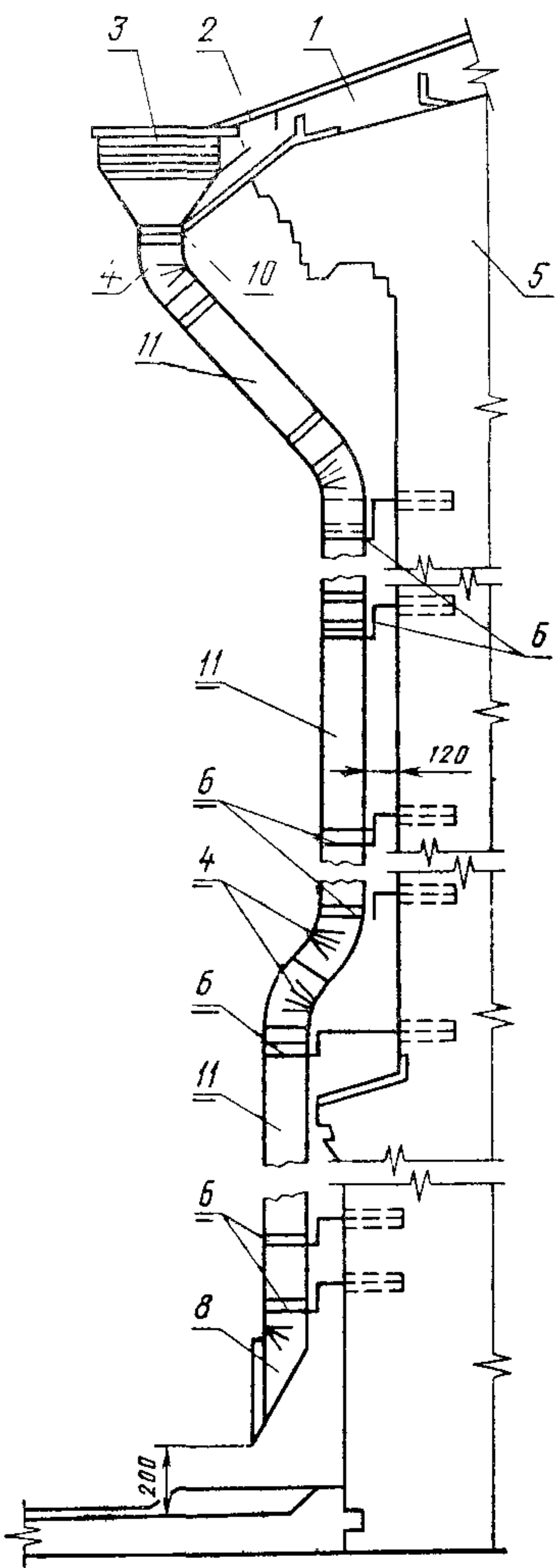
Применение звеньев труб типов ТВ1 и ТВ2
