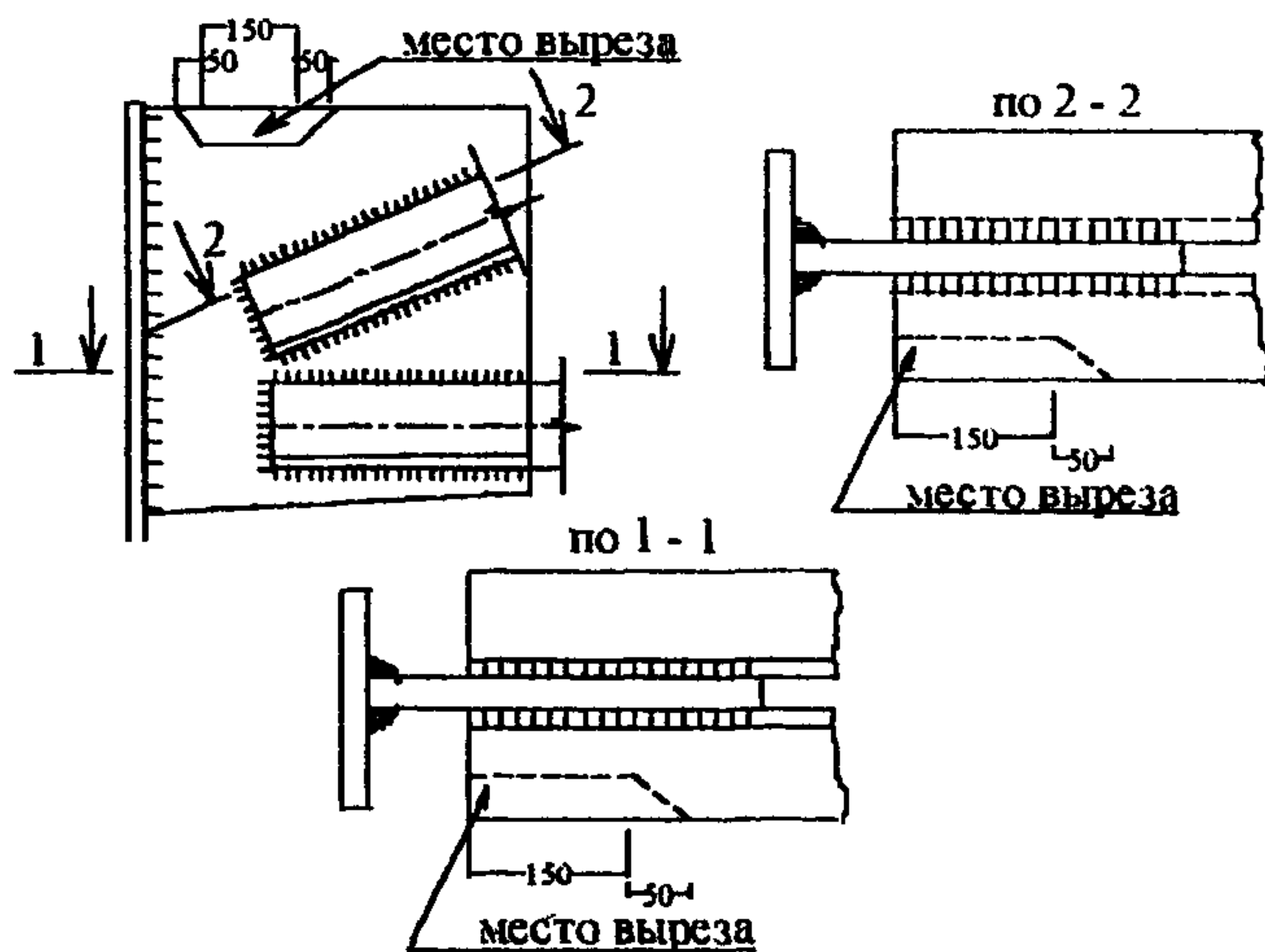
Рис. 1. Место вырезки контрольных образцов в сохранившихся фермах.
