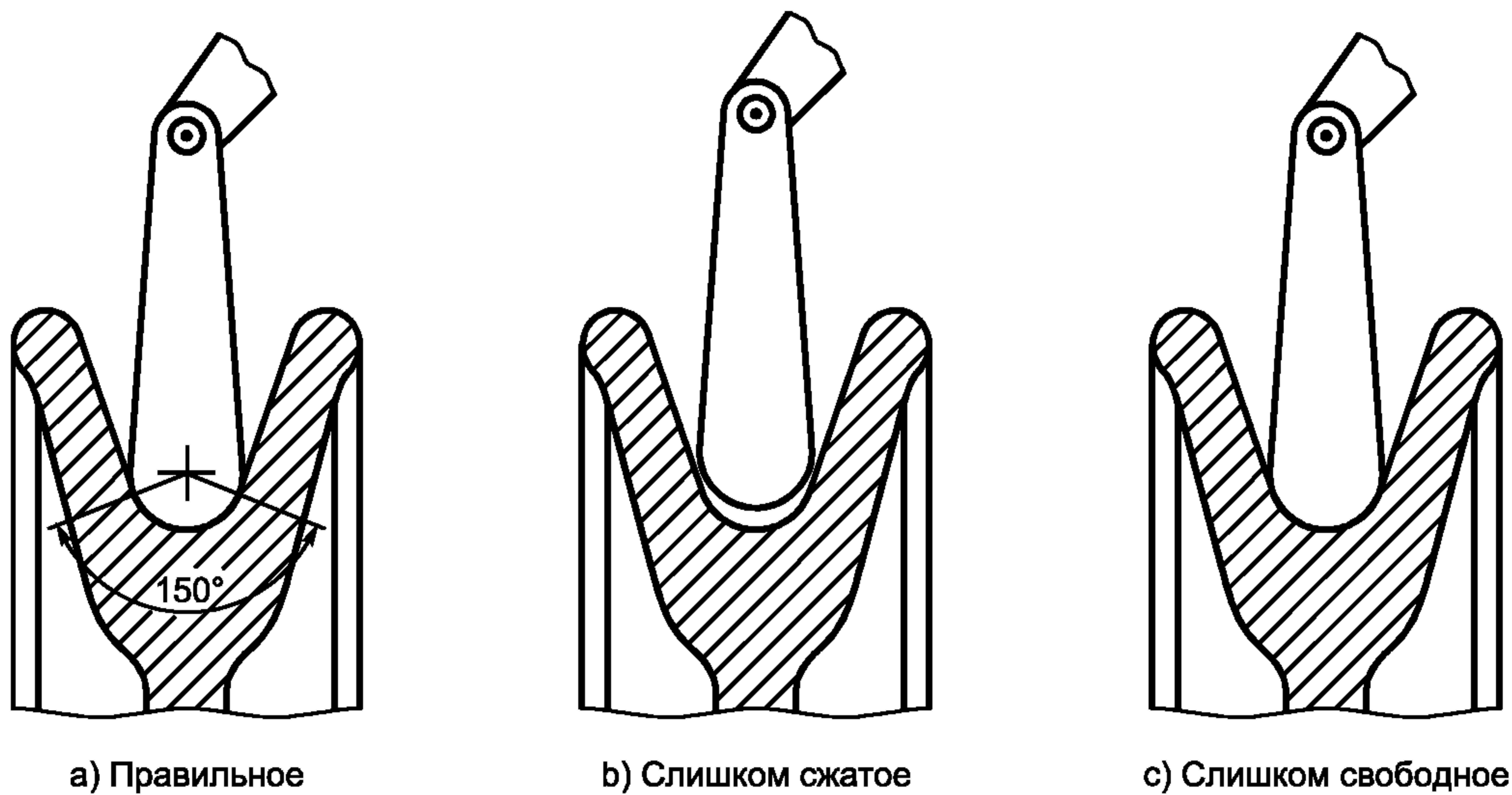
Рисунок С.4 — Проверка шкивов
