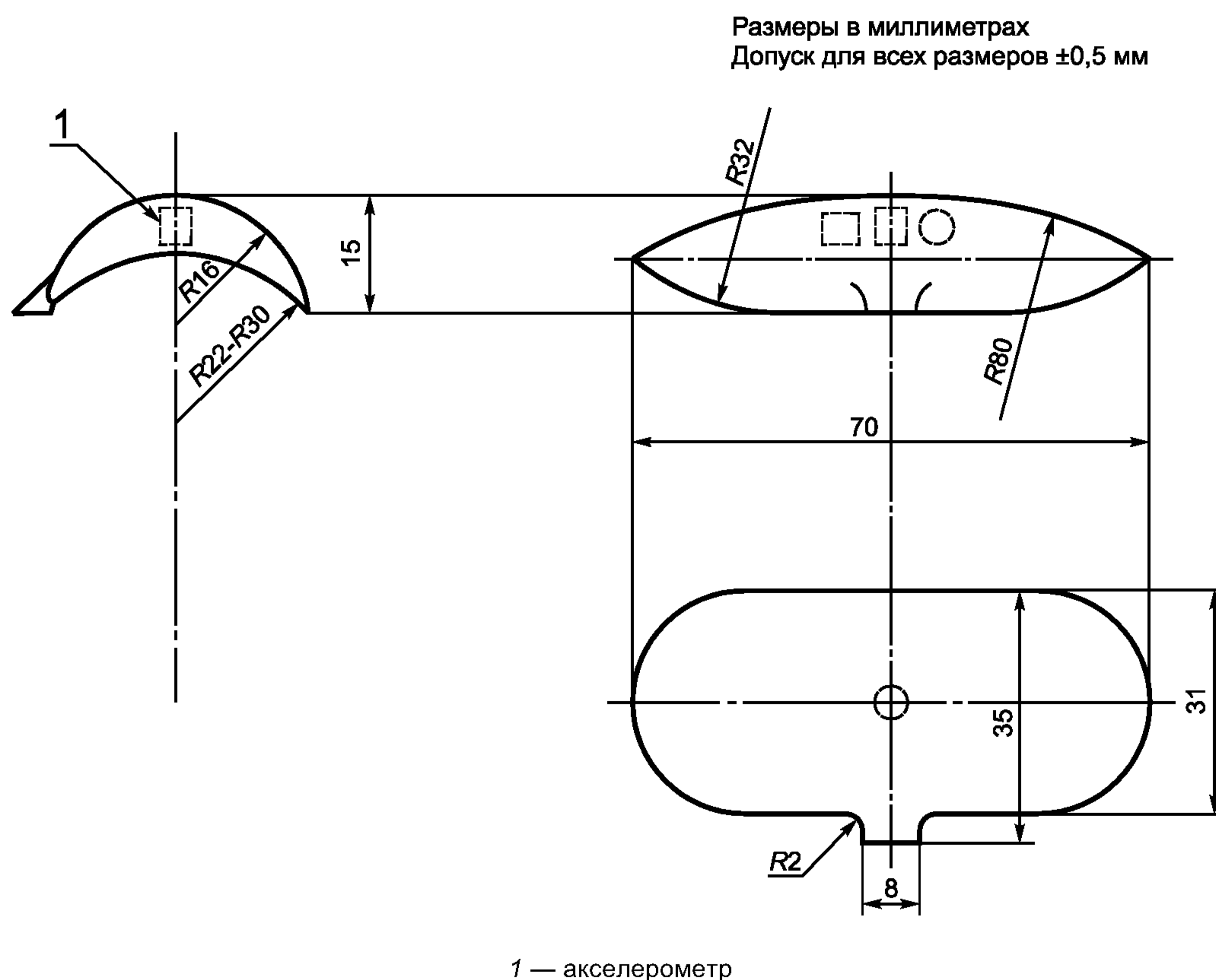
Рисунок 2 — Адаптер, позволяющий удерживать акселерометр в ладони руки
