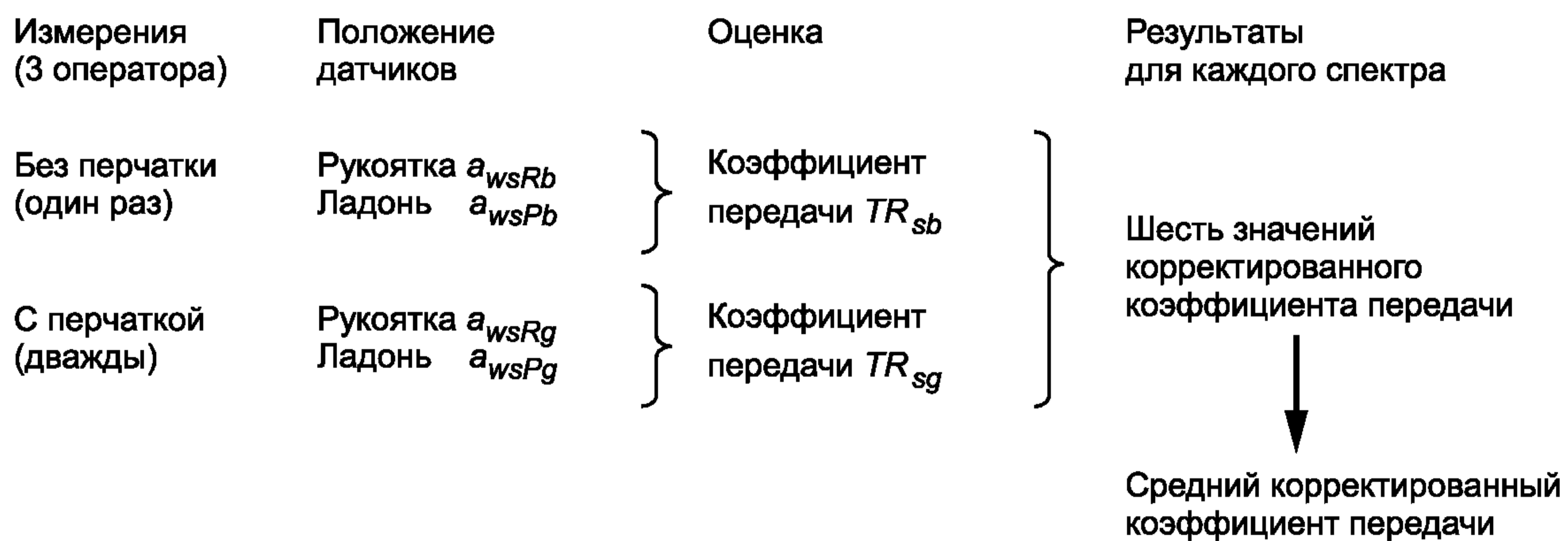
Рисунок 7 — Схема определения среднего скорректированного коэффициента передачи
