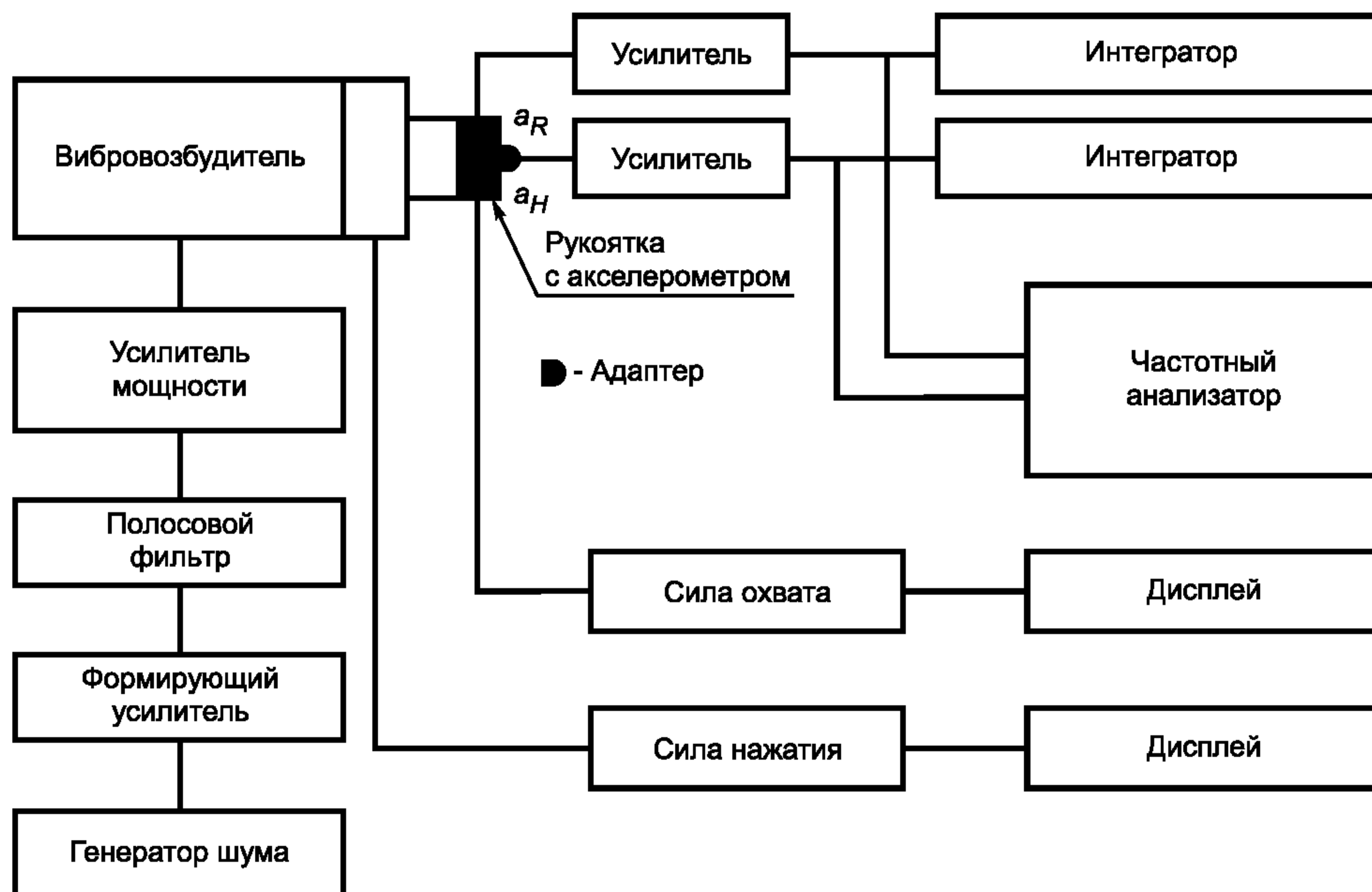
Рисунок 1 —Схема измерений вибрационной передаточной функции
