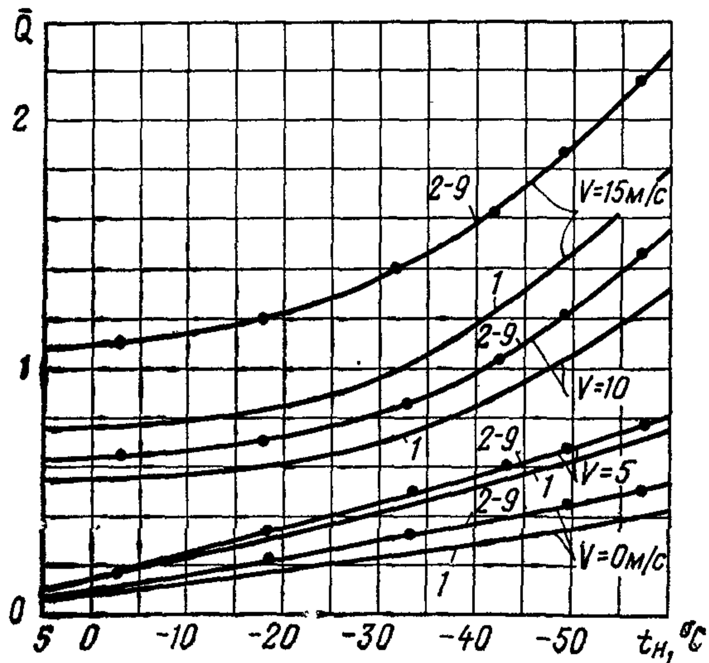
Рис. 14. Величина относительных теплотерь ( \bar{Q} ) для помещений 1—9-го этажей с избыточной вытяжкой девятиэтажного здания при работе систем вентиляции
