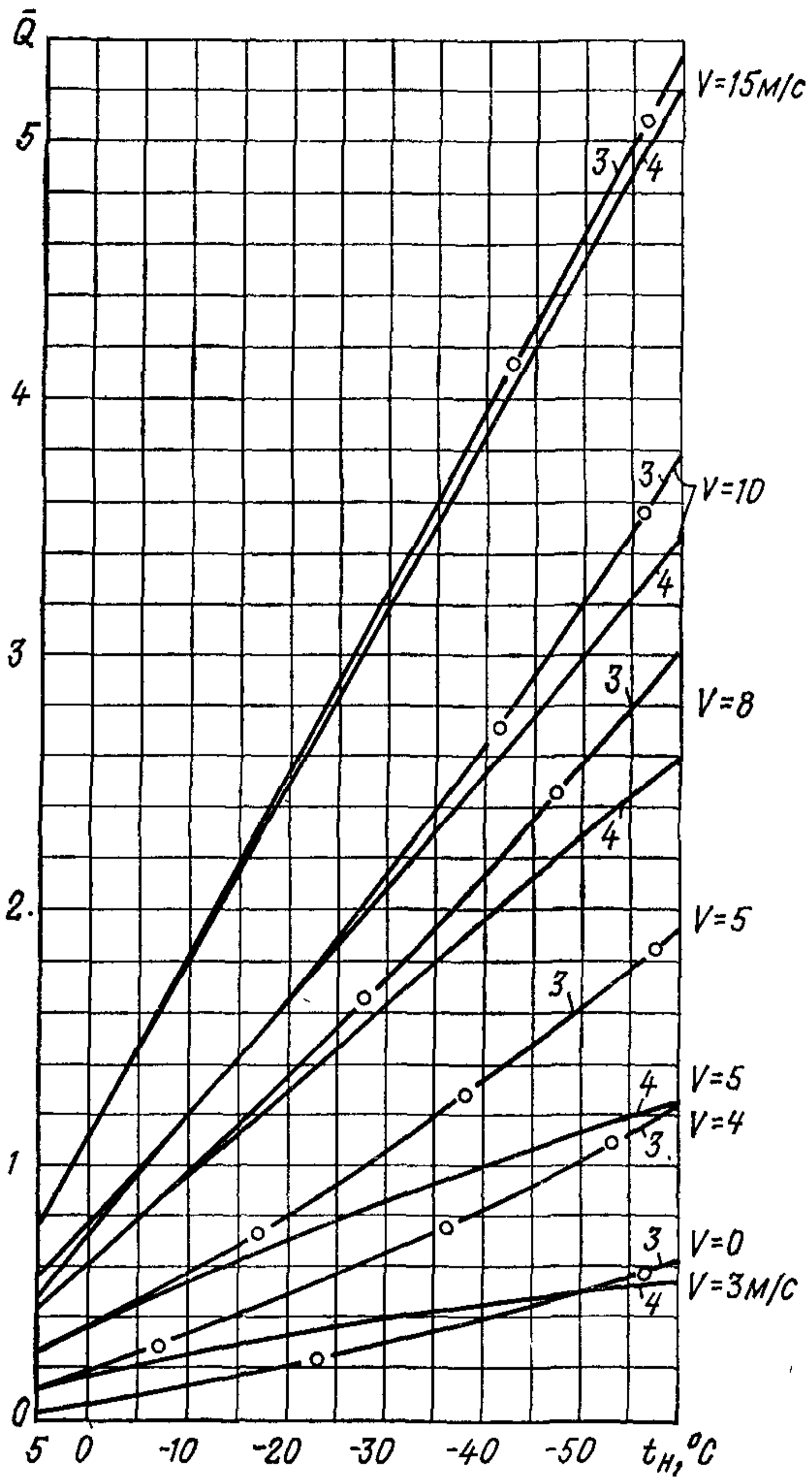
Рис. 2. Величина относительных теплотерь ( \bar{Q} ) для помещений 3—4-го этажей шестиэтажного здания в нерабочее время, а также для помещений с вытяжной вентиляцией, полностью компенсируемой притоком в рабочее время
