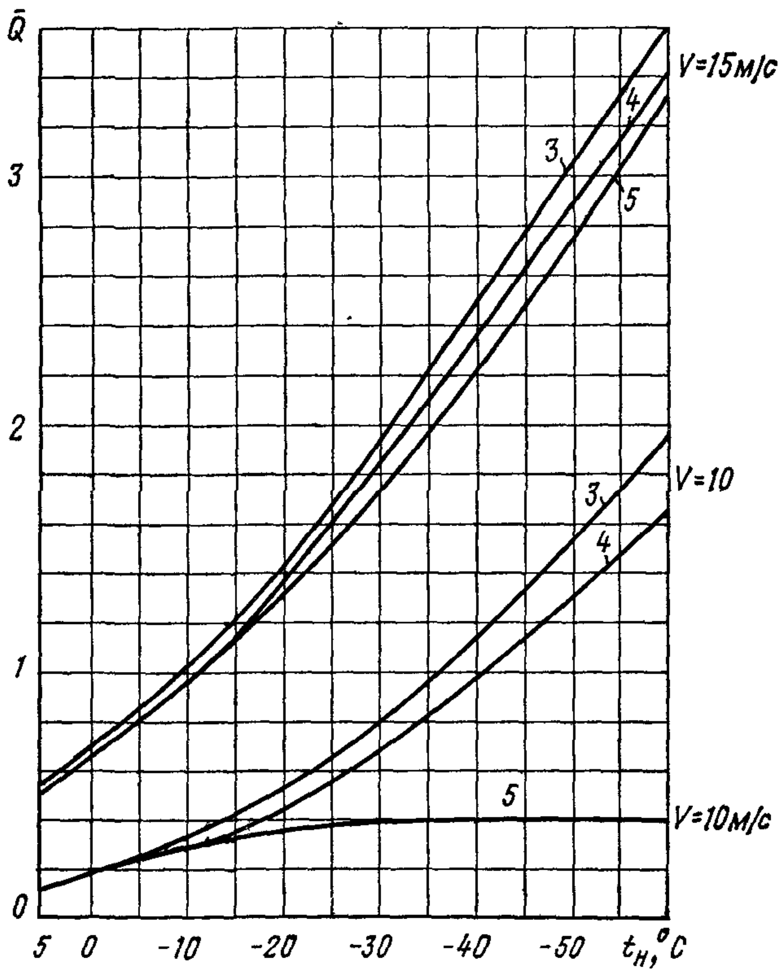
Рис. 8. Величина относительных теплопотерь ( \bar{Q} ) для помещений 3—5-го этажей шестиэтажного здания с избыточным притоком в рабочее время
