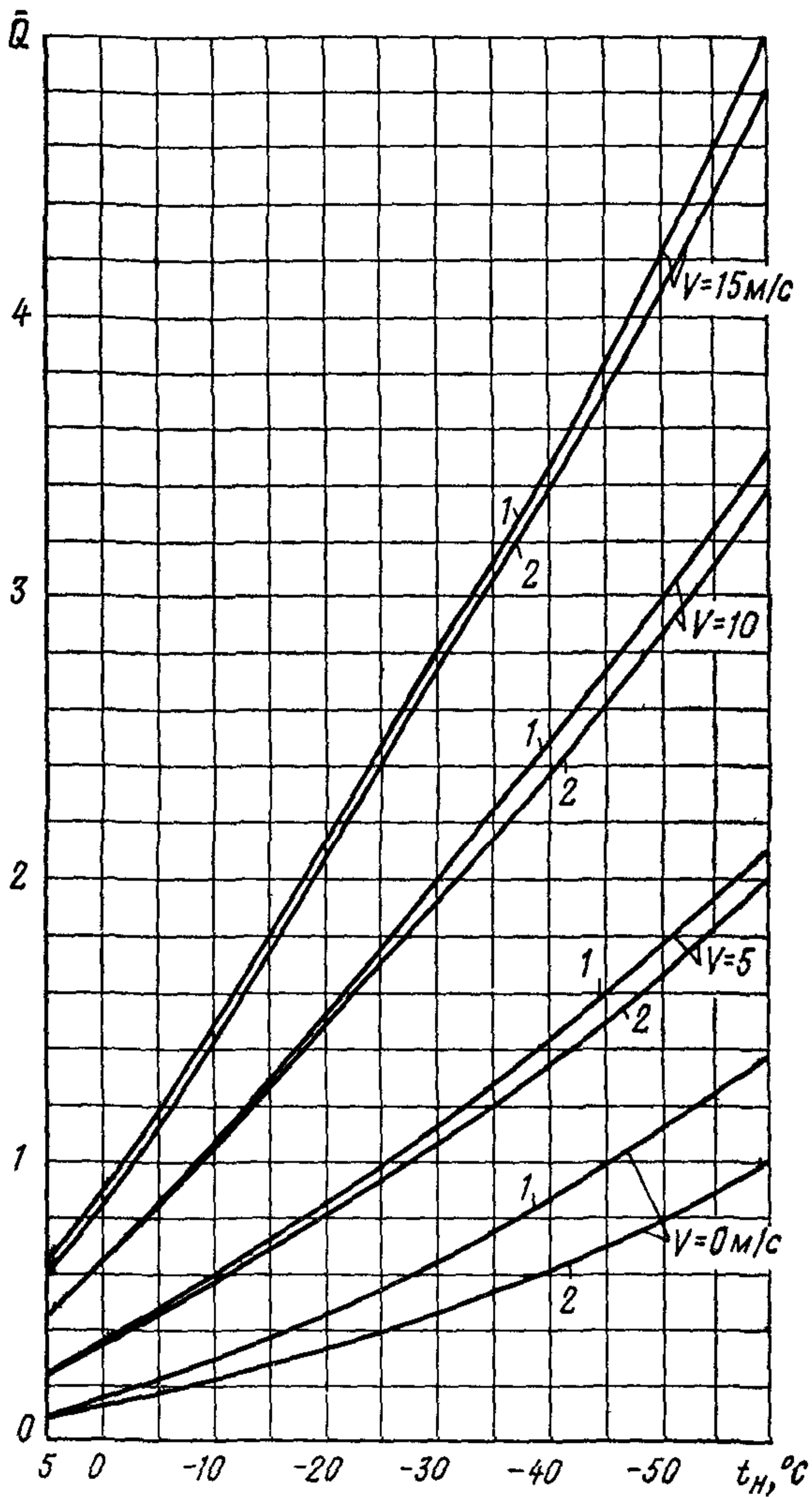
Рис. 9. Величина относительных теплопотерь ( \bar{Q} ) для помещений 1—2-го этажей девятиэтажного здания при выключенной системе вентиляции
