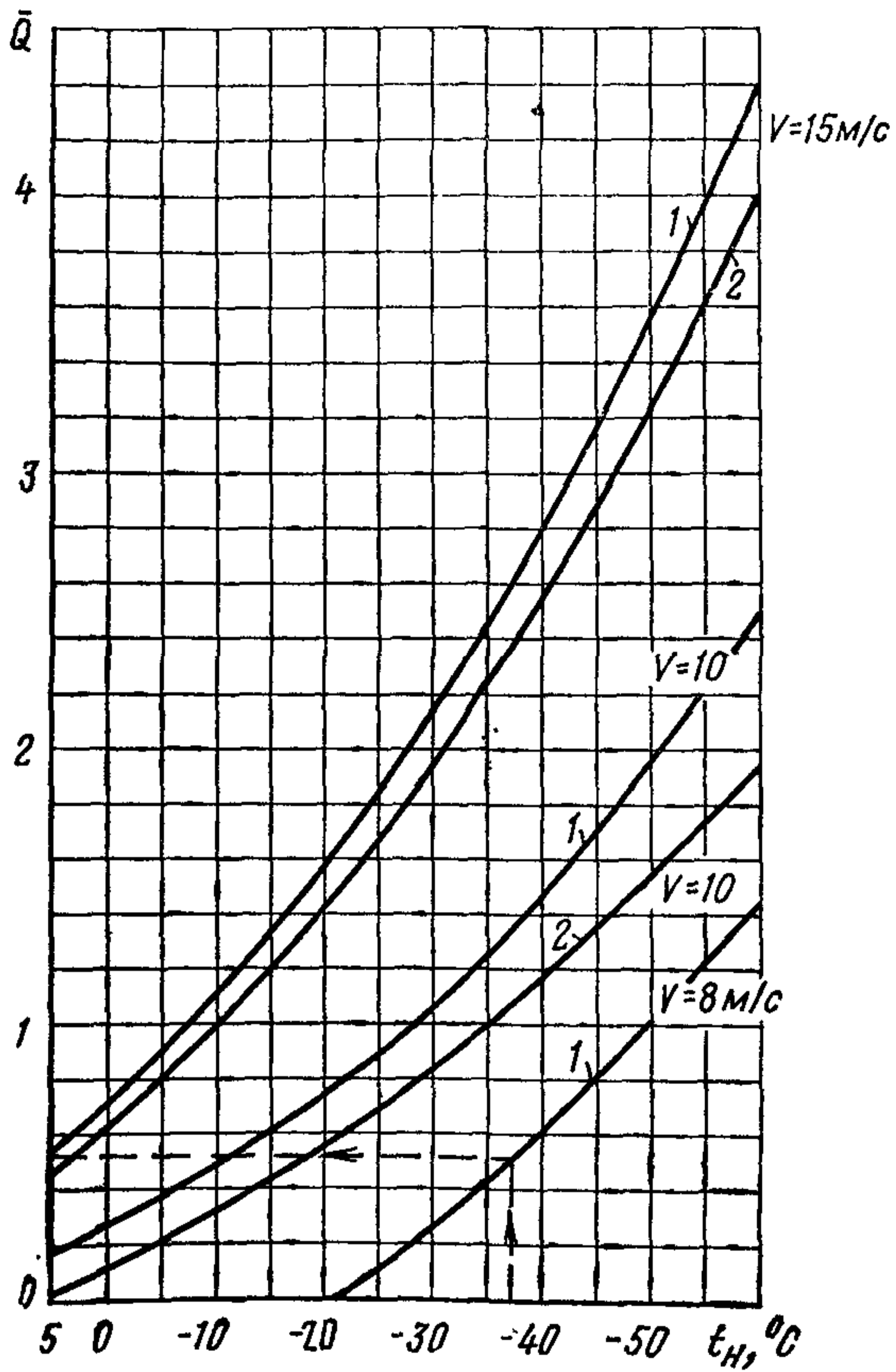
Рис. 7. Величина относительных теплотерь ( \bar{Q} ) для помещений 1—2-го этажей шестиэтажного здания с избыточным притоком в рабочее время
