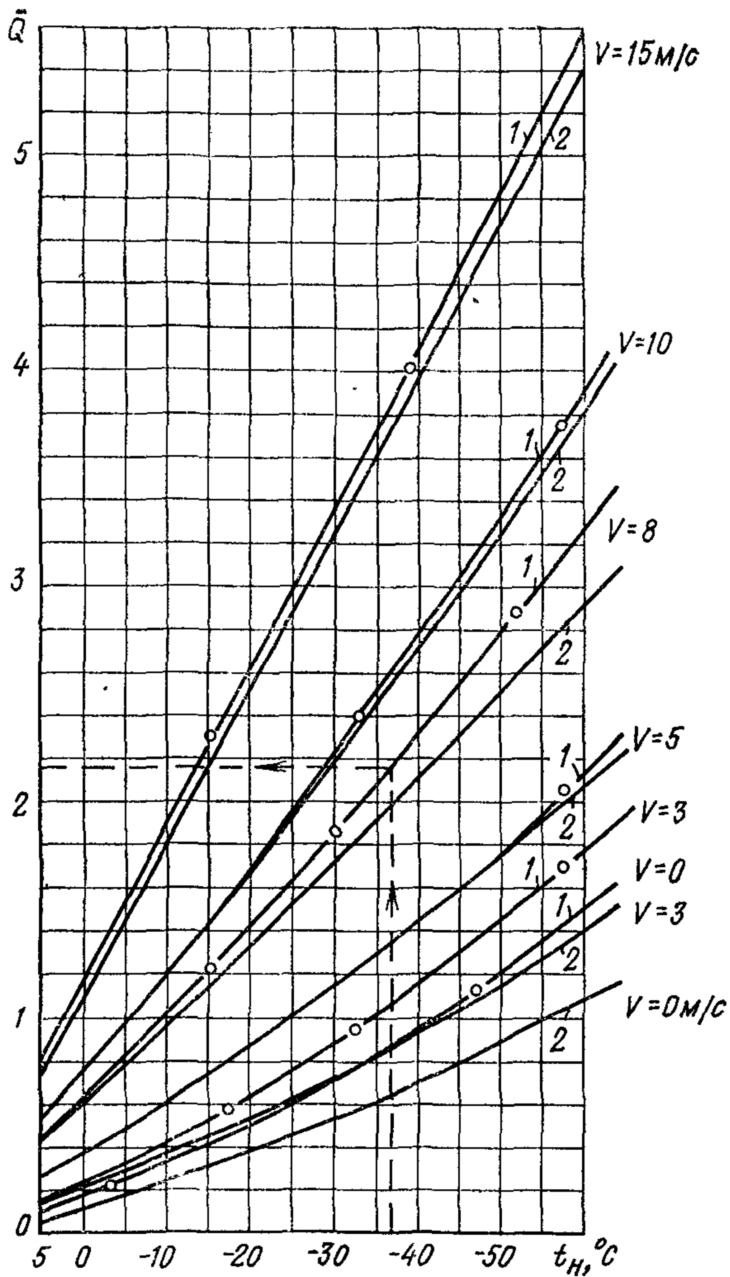
Рис 1. Величина относительных теплотерь ( \bar{Q} ) для помещений 1—2-го этажей шестиэтажного здания в нерабочее время, а также для помещений с вытяжной вентиляцией, полностью компенсируемой притоком в рабочее время
