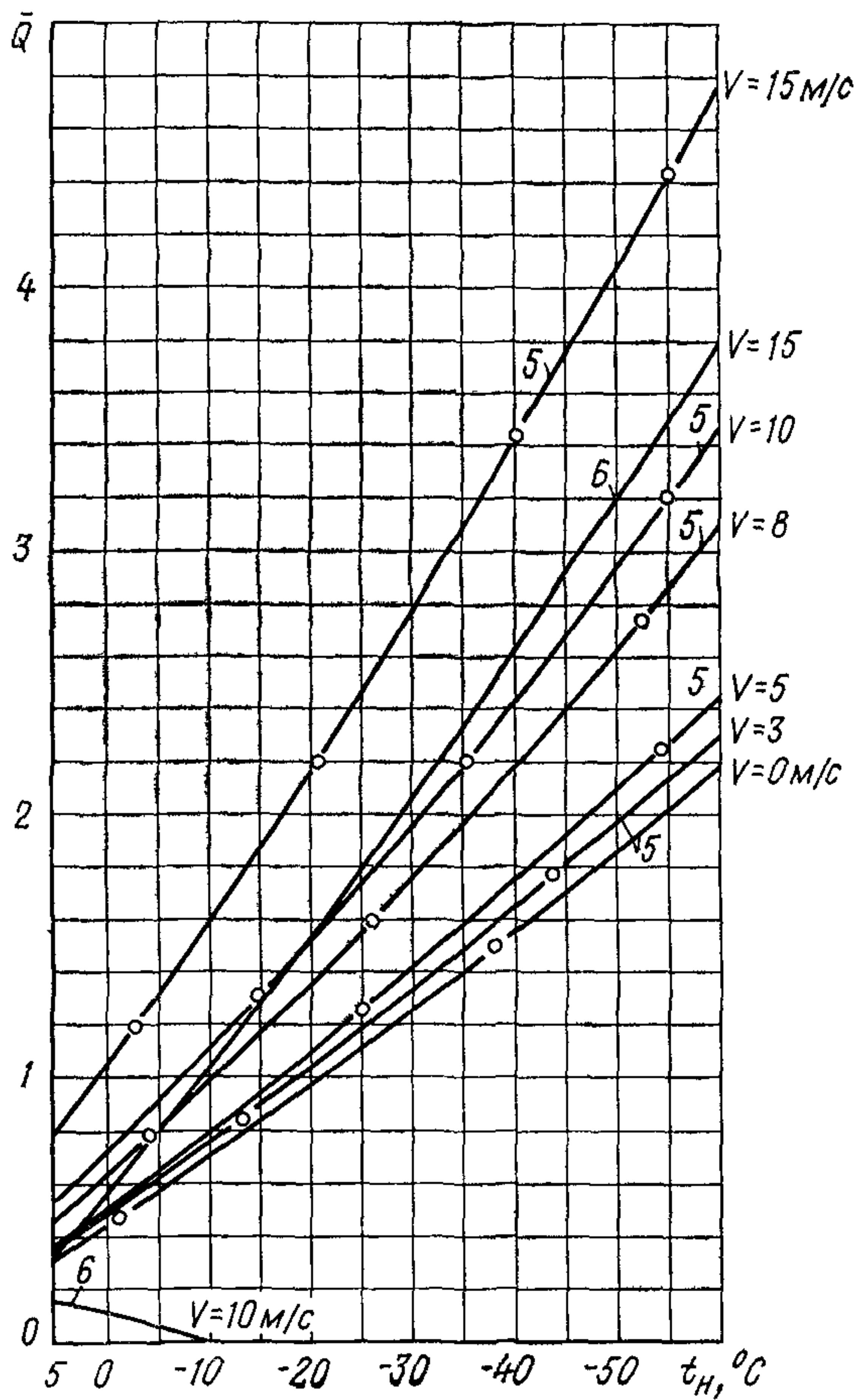
Рис. 6. Величина относительных теплопотерь ( \bar{Q} ) для помещений 5—6-го этажей шестизэтажного здания с вытяжной вентиляцией, не компенсируемой притоком в рабочее время
