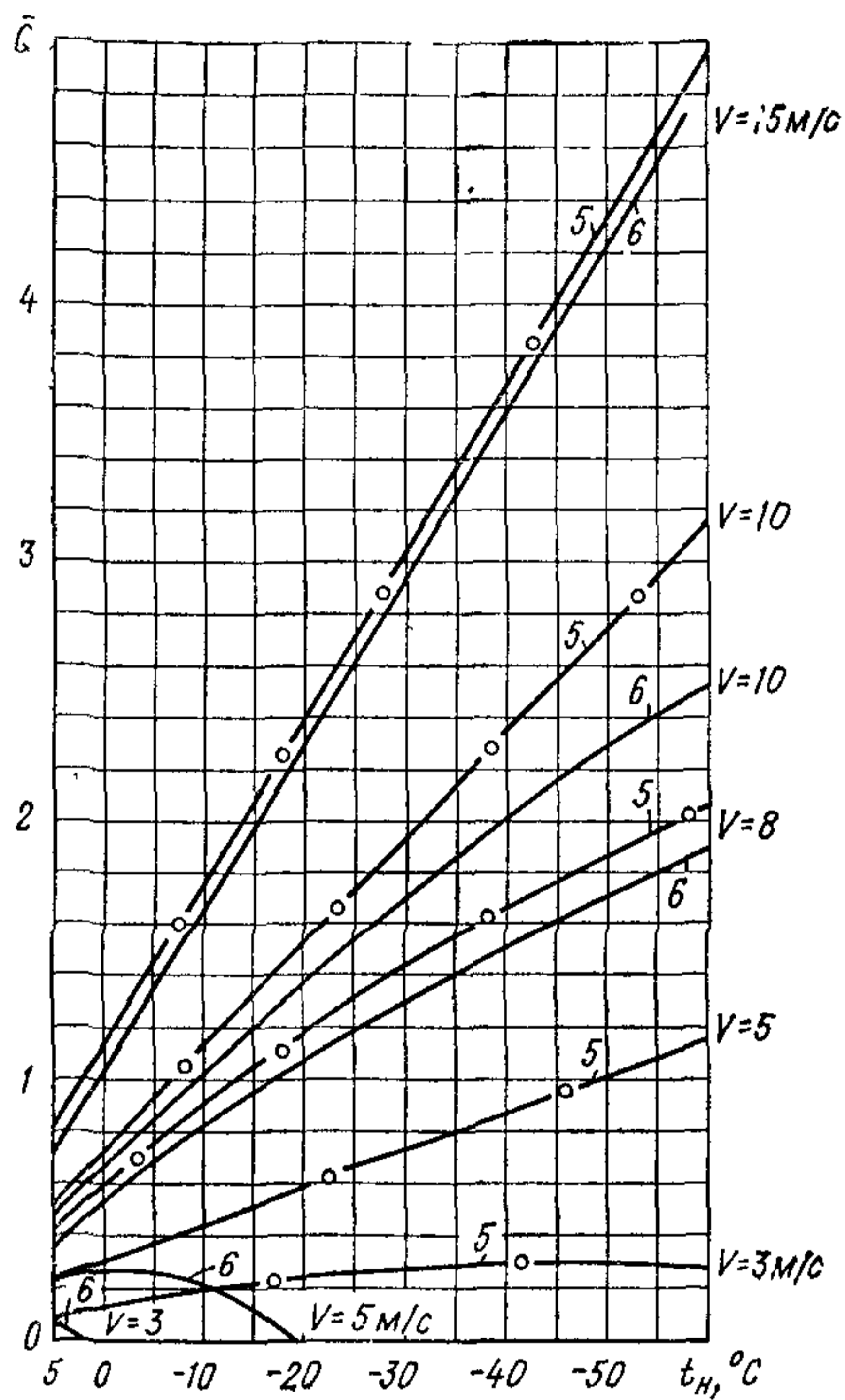
Рис. 3. Величина относительных теплотерь (\bar{Q}) для помещений 5—6-го этажей шестизэтажного здания в нерабочее время, а также для помещений с вытяжной вентиляцией, полностью компенсируемой притоком в рабочее время
