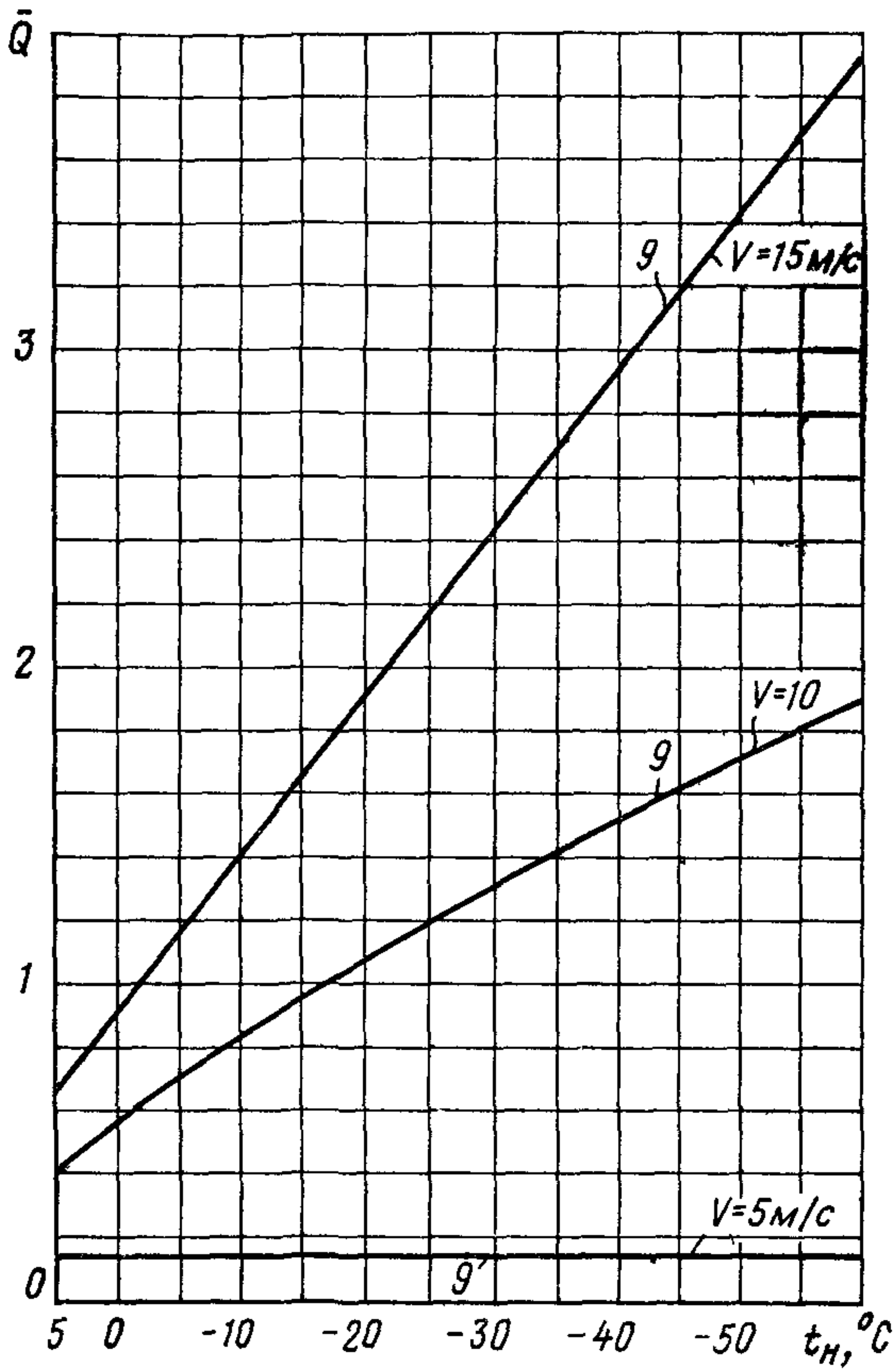
Рис. 13 Величина относительных теплопотерь ( \bar{Q} ) для помещений 9-го этажа девятиэтажного здания при выключенной системе вентиляции
