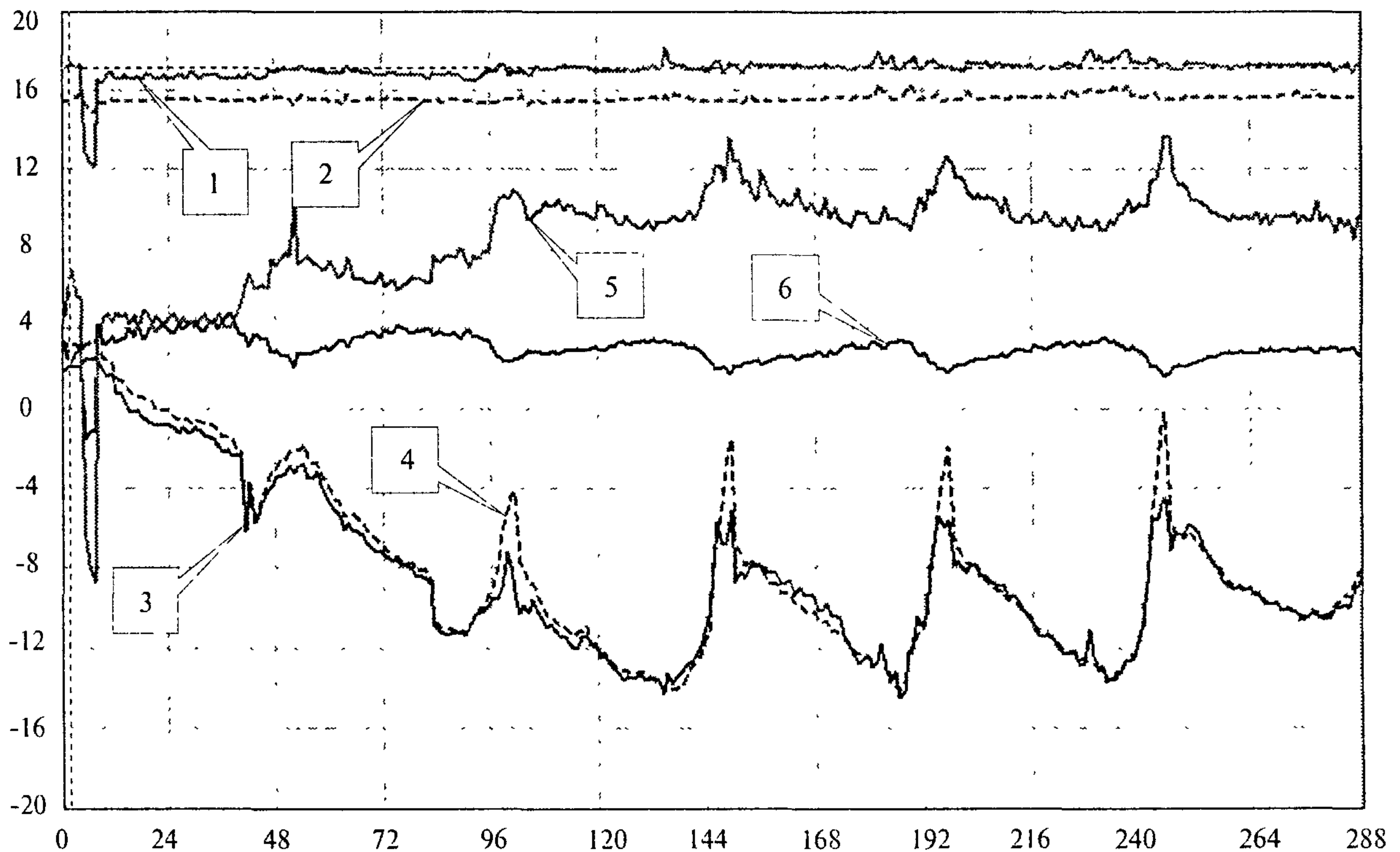
Рис.3. Графики регистрируемых величин, по оси абсцисс отложены точки измерения с интервалом 30 мин, по оси ординат — температура (°C), плотность теплового потока (Вт/м 2 ), сопротивление теплопередаче (м 2 ·°C/Вт)
