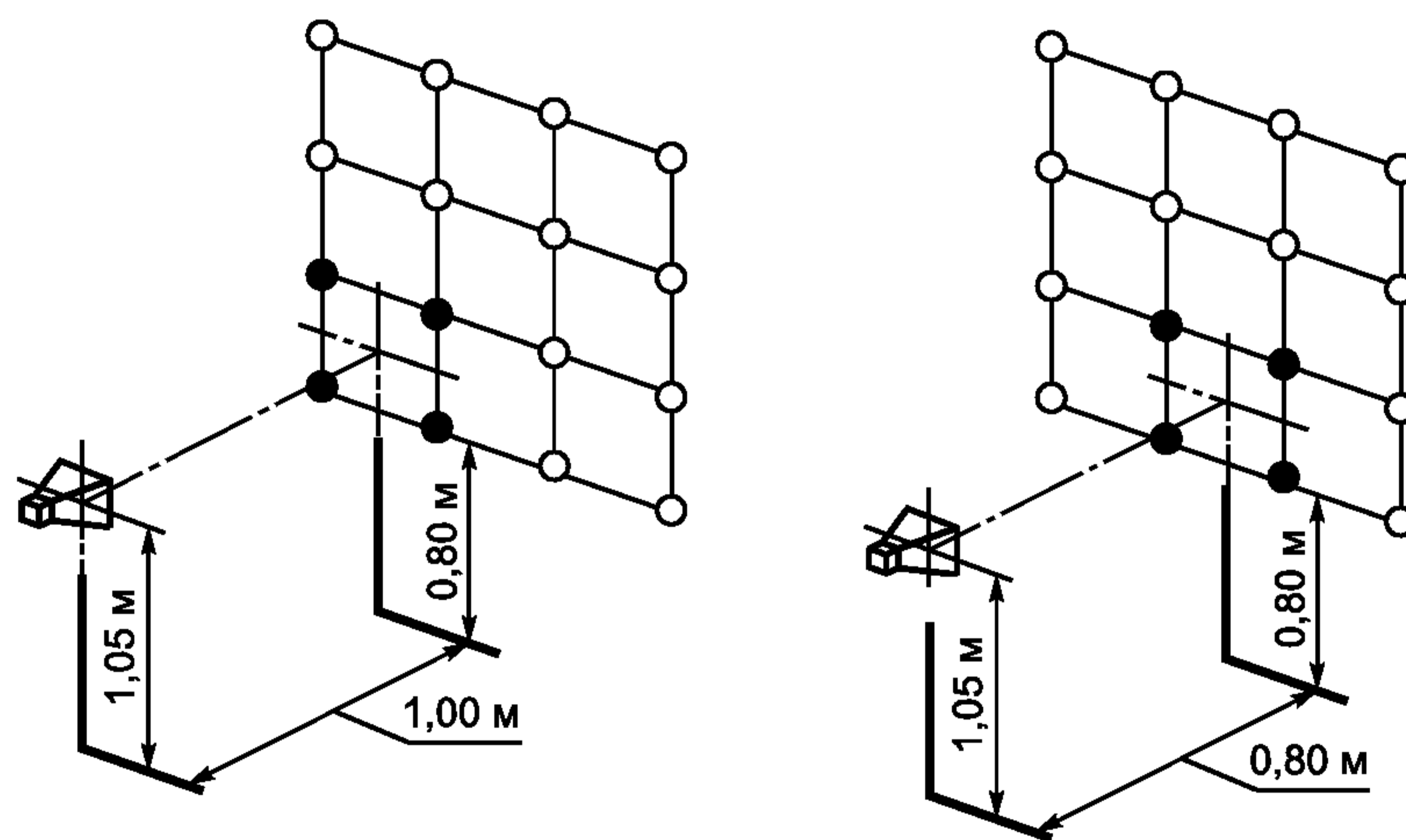
Рисунок И.2 — Пример последовательного облучения окон
