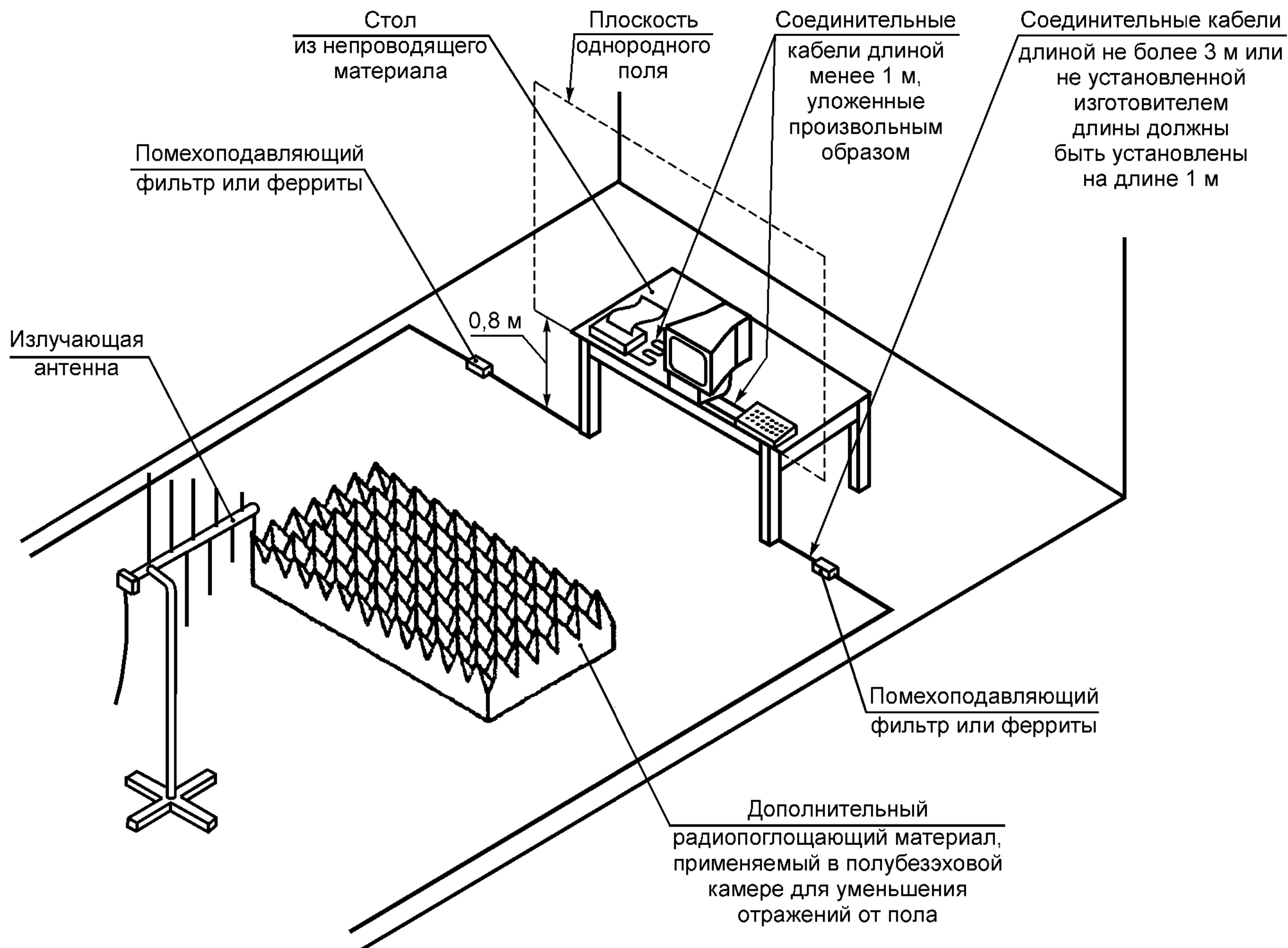
Рисунок 6 — Пример установки для испытаний настольных ТС
