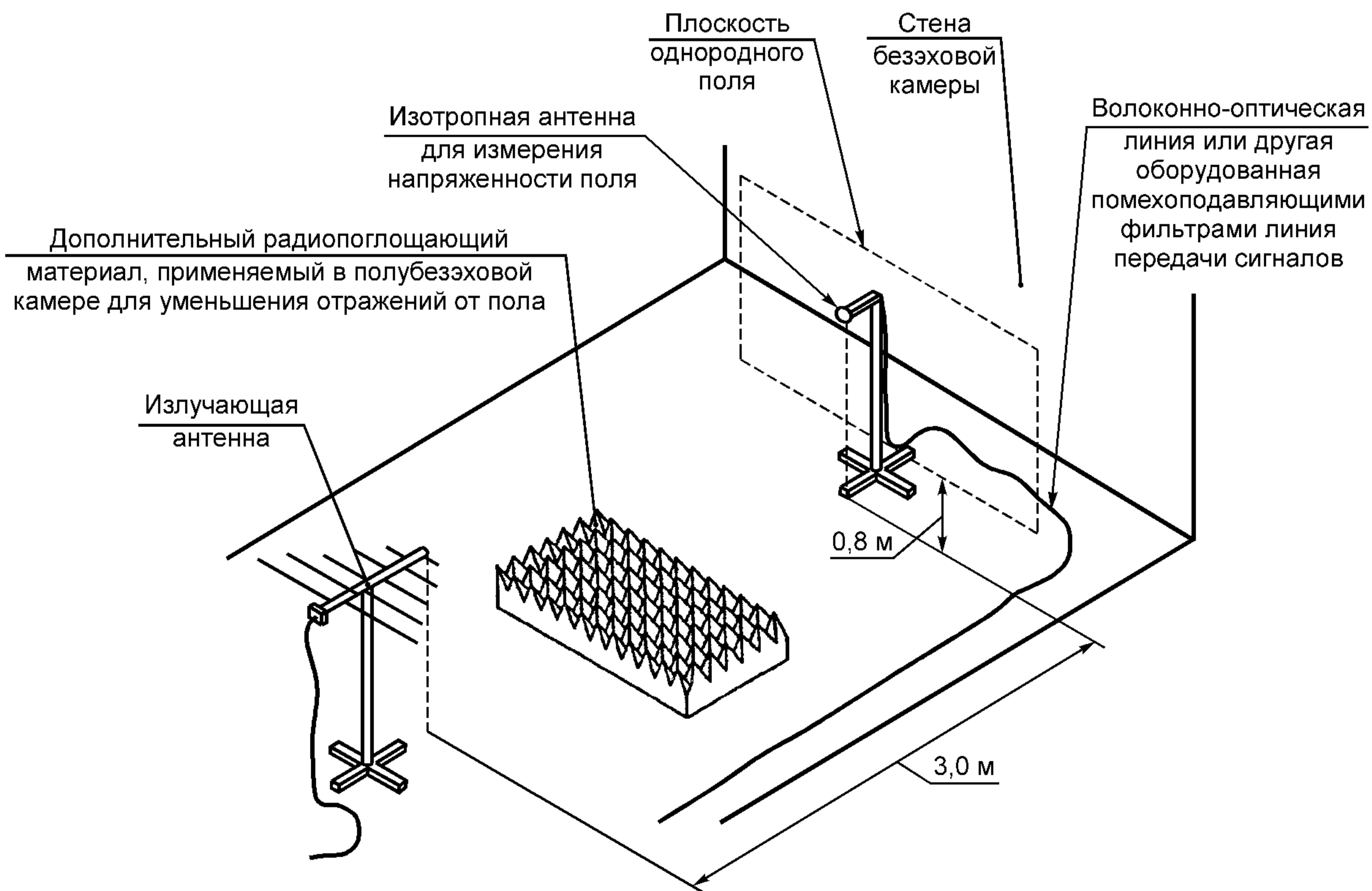
Рисунок 3 — Расположение оборудования при калибровке испытательного поля
