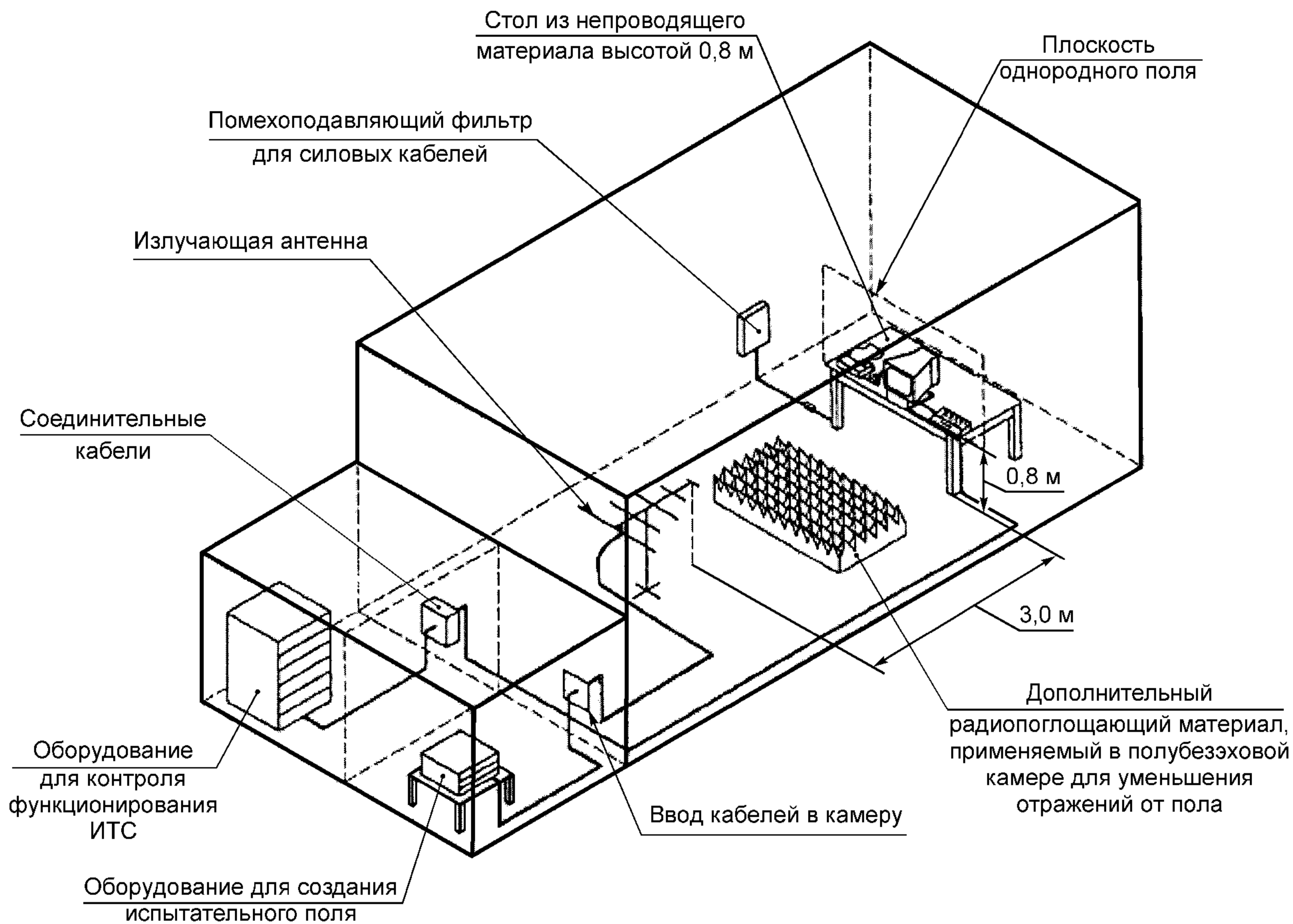
Рисунок 2 — Пример испытательной установки
