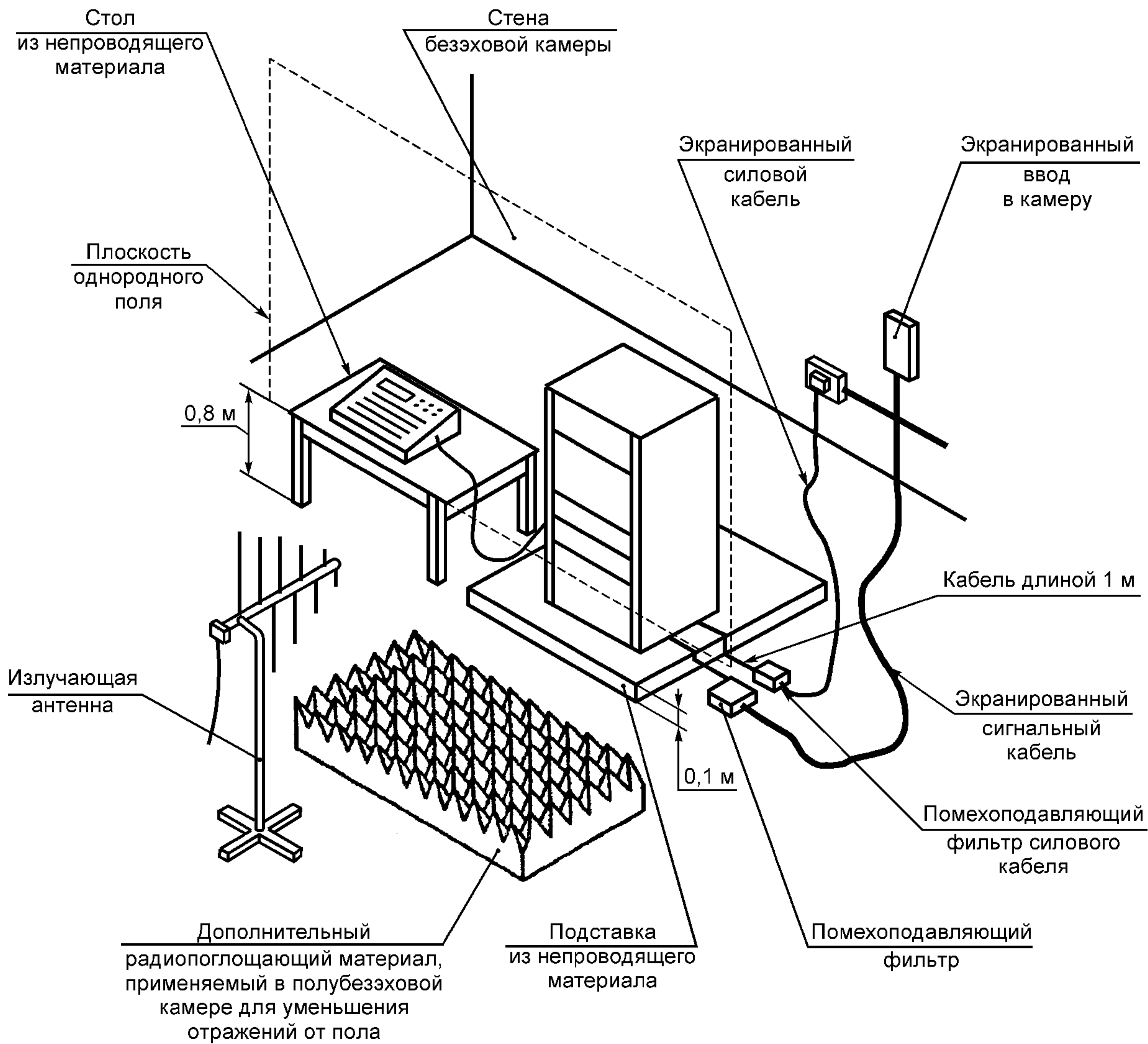
Рисунок 5 — Пример установки для испытаний напольных ТС
