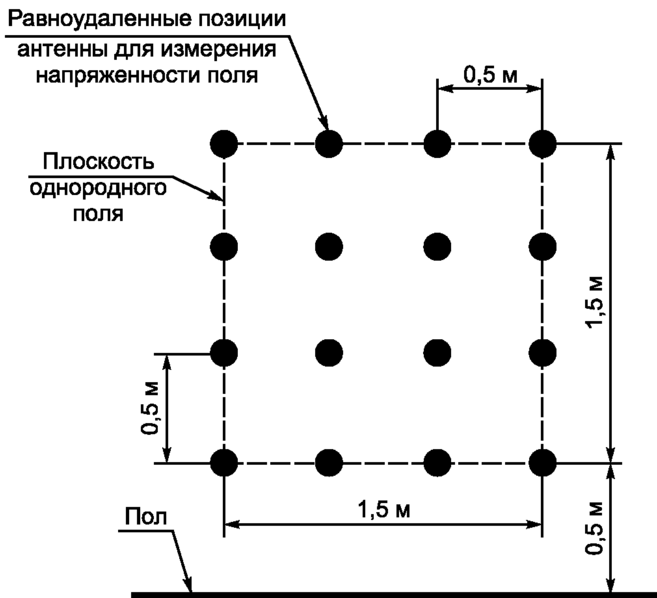
Рисунок 4 — Пример плоскости однородного поля размерами 1,5 × 1,5 м
