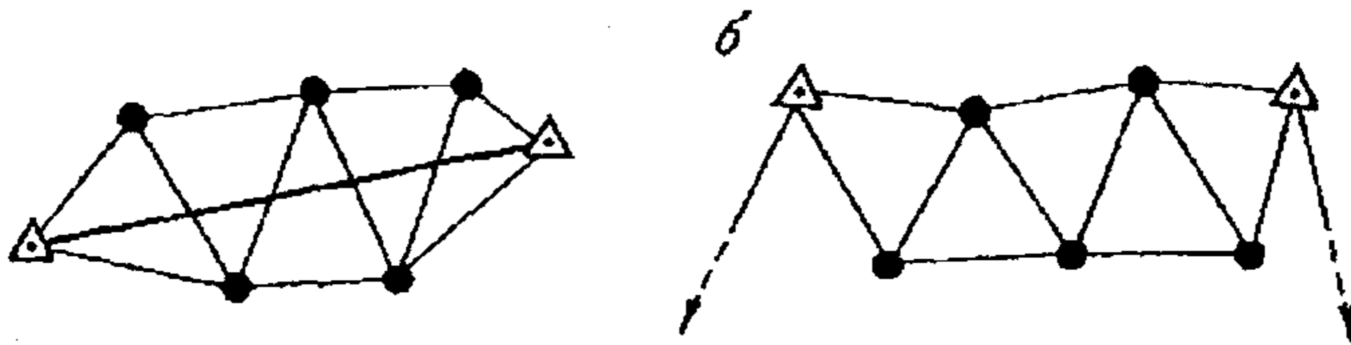
Рис. 24 Цепочки треугольников между двумя пунктами
