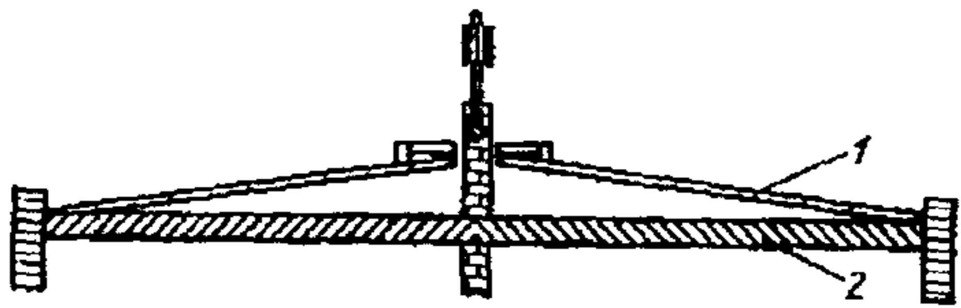
Рис. 29. Тур со съемной визирной целью 1 — крылья; 2 — перекрытие (балка)
