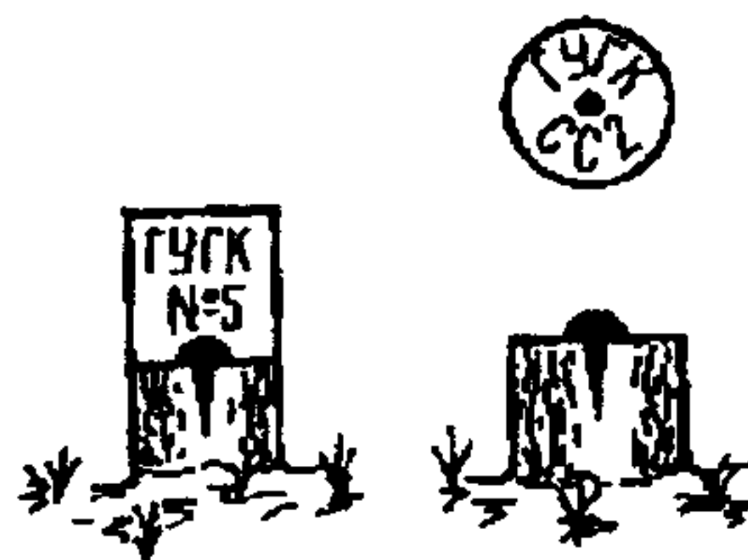
Рис. 49 Штырь, кованый гвоздь в гне
