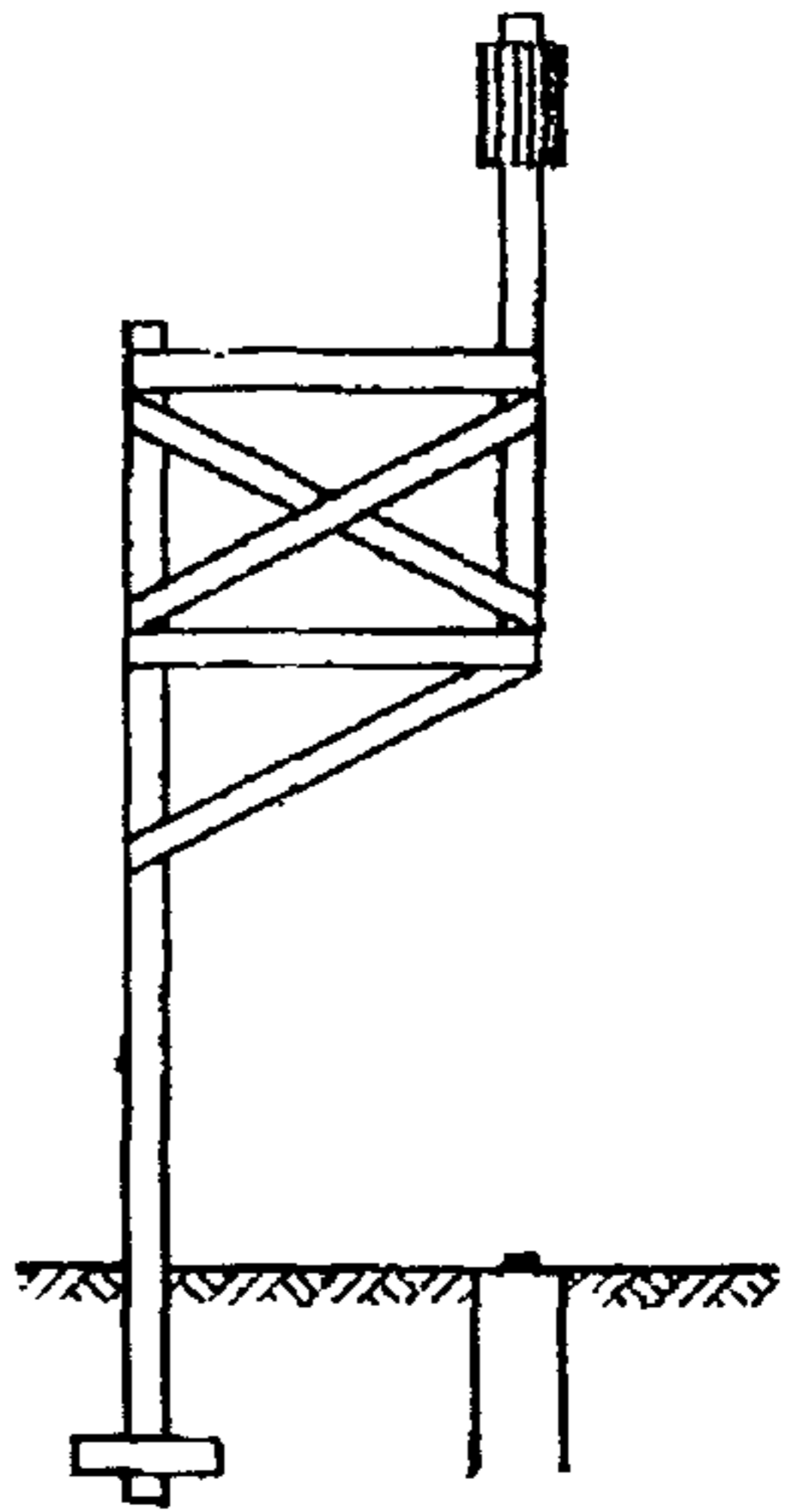
Рис. 28. Г-образная мача (деревянная или металлическая)
