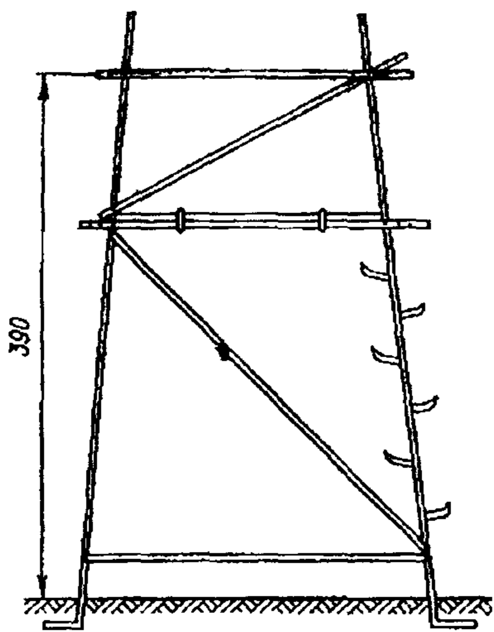
Рис. 27. Металлическая переносная площадка для наблюдения с пирамид-штативом. Изготавливается из уголковой стали (50×50×5 и 25×33×4)
