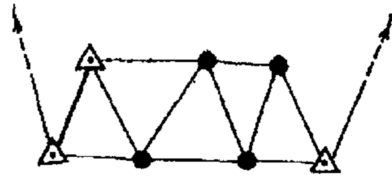
Рис. 23 Цепочка треугольников между стороной и пунктом
