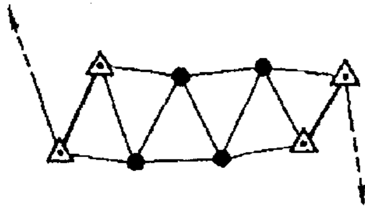
Рис. 22 Цепочка треугольников между двумя сторонами
